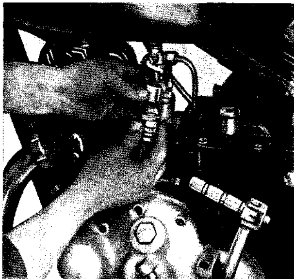
Abb. 11. Kraftstoffhahn und Reinigungssieb: Zur Reinigung des Siebes entfernt man zuerst die Schutzglocke mit einem 17-mm-Schlüssel, darauf mit der Kombinationszange die Sieb-Befestigungsmutter. Es ist alles gut in Benzin auszuwaschen, wieder in der richtigen Reihenfolge einzusetzen und gut festzuziehen. In normaler Fahrstellung steht der Hebel senkrecht nach unten. Bei dieser Hebelstellung bleibt im Tank eine Reservekraftstoffmenge von ca. 2 Liter zurück, ausreichend für eine Fahrstrecke von ca. 20 km. Eingeschaltet wird diese Reservemenge durch Nach-links-schalten des Hahnes. Man vergesse nicht, nach dem Tanken den Hebel wieder nach unten zu stellen, damit die Reservemenge wieder gesichert ist.
