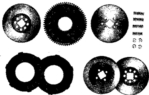
Abb. 18. Kupplung in Einzelteile zerlegt: Oben in der Mitte die zentrale Antriebsscheibe, links darunter die beiden Belaglamellen (Kork bzw. Jurid), daneben die entsprechenden Stahlscheiben. Die gesamte Kupplung arbeitet im Ölbad.
