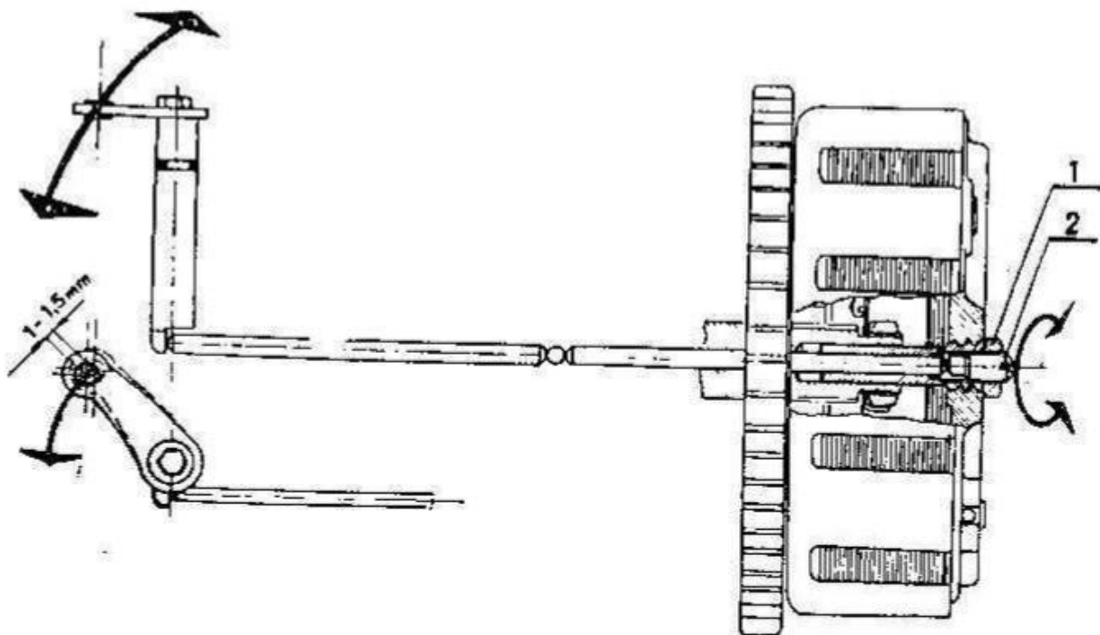
obr. 10 seřízení spojkového mechanismu
