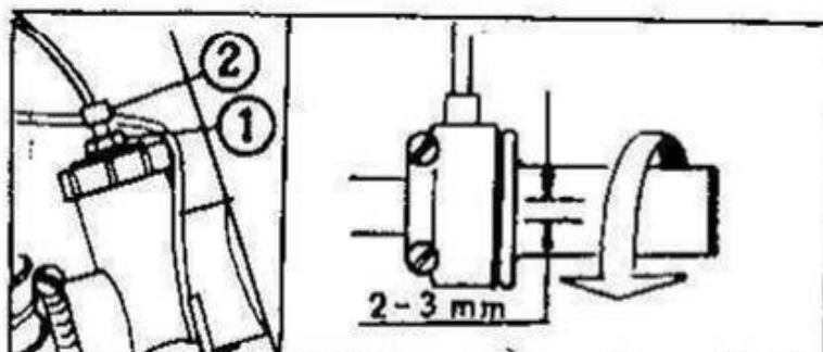
obr. 11 seřizovací šroub karburátoru - bowden plynu - plynová rukojet
