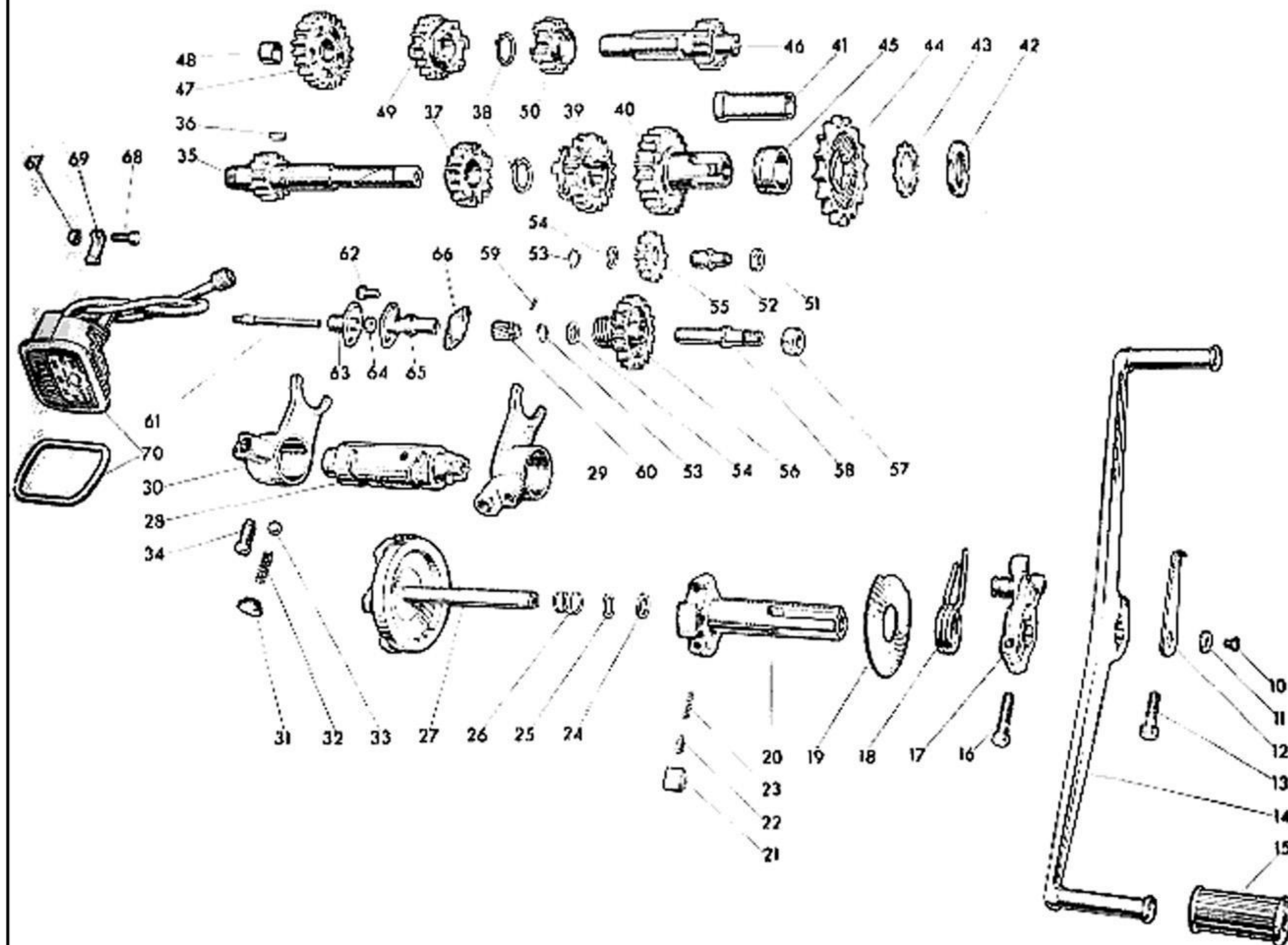
TAV. 7 COMPLESSO : Motociclo SOTTOCOMPLESSO: Trasmissione GRUPPO : Cambio SOTTOGRUPPO: Ingranaggi - Alberi e comando del cambio - Contachilometri
