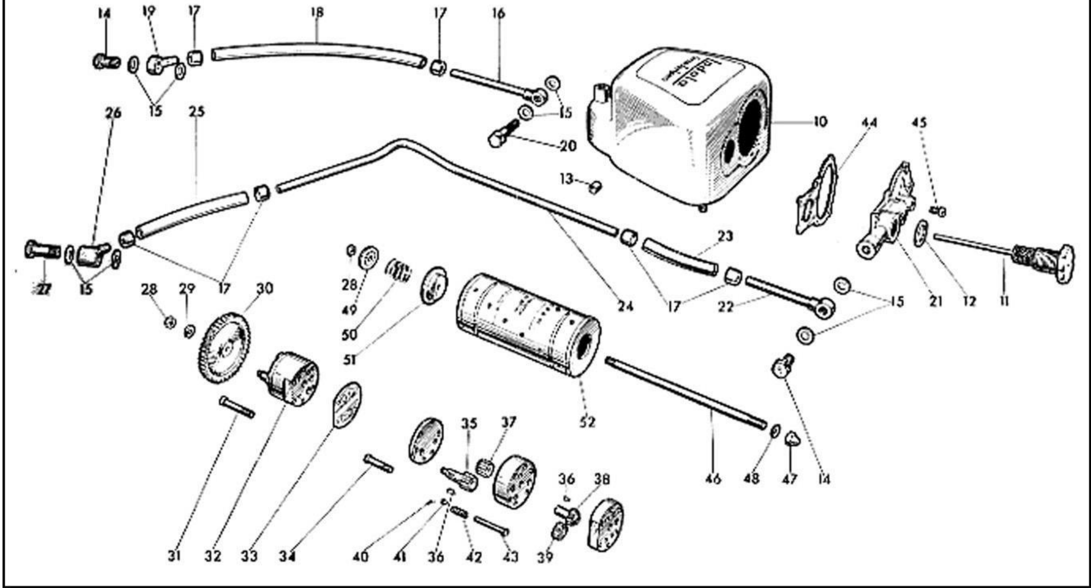
TAV. 5 COMPLESSO : Motociclo GRUPPO : Lubrificazione SOTTOCOMPLESSO: Motore SOTTOGRUPPO: Serbatoio olio - Pompa olio - Valvola automatica Tubazioni
