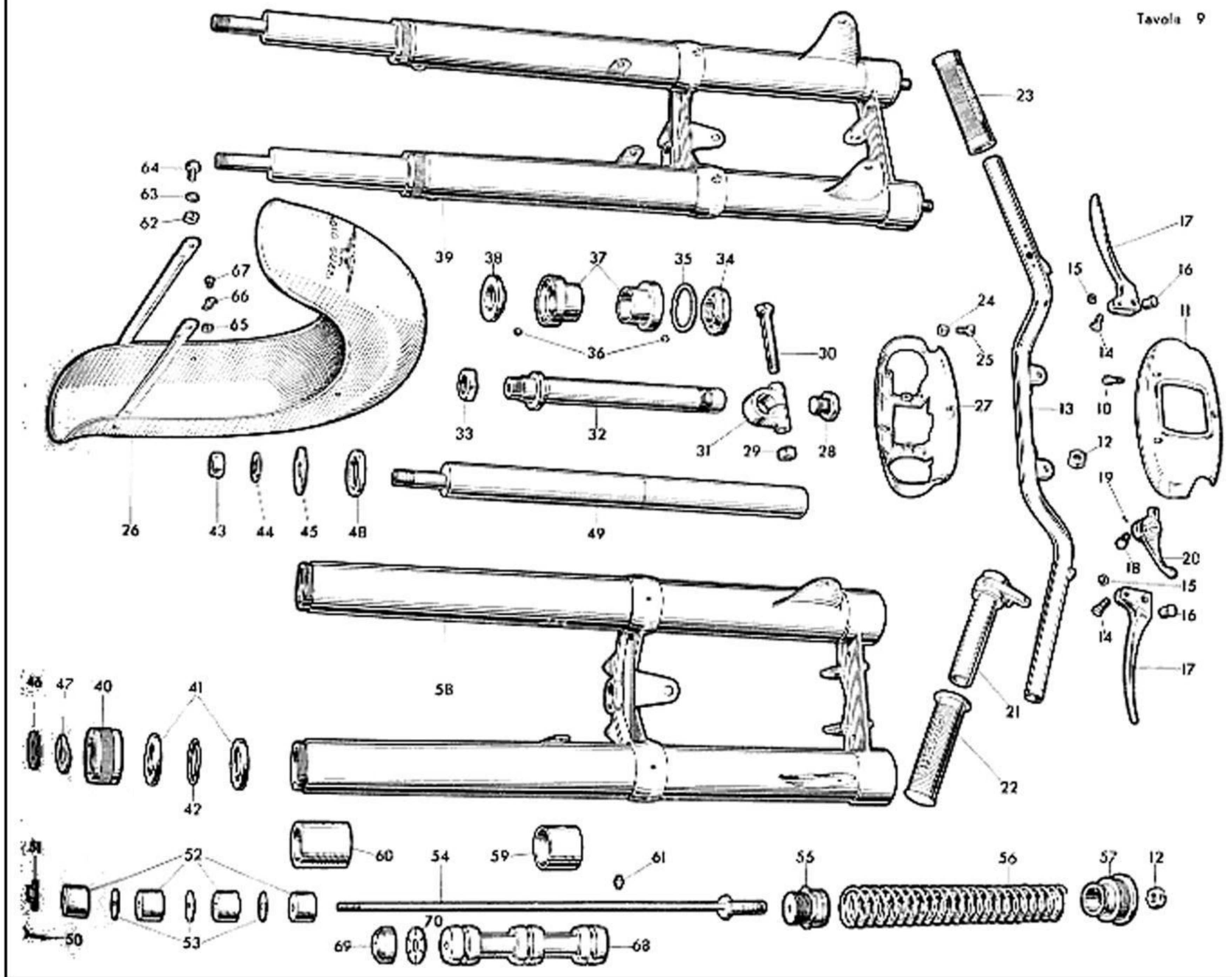
TAV. 9 COMPLESSO : Motociclo GRUPPO : Sospensione anteriore e sterzo SOTTOCOMPLESSO: Telaio - Sospensioni - Ruote SOTTOGRUPPO: Forcella anteriore - Manubrio e leve di comando Parafango anteriore
