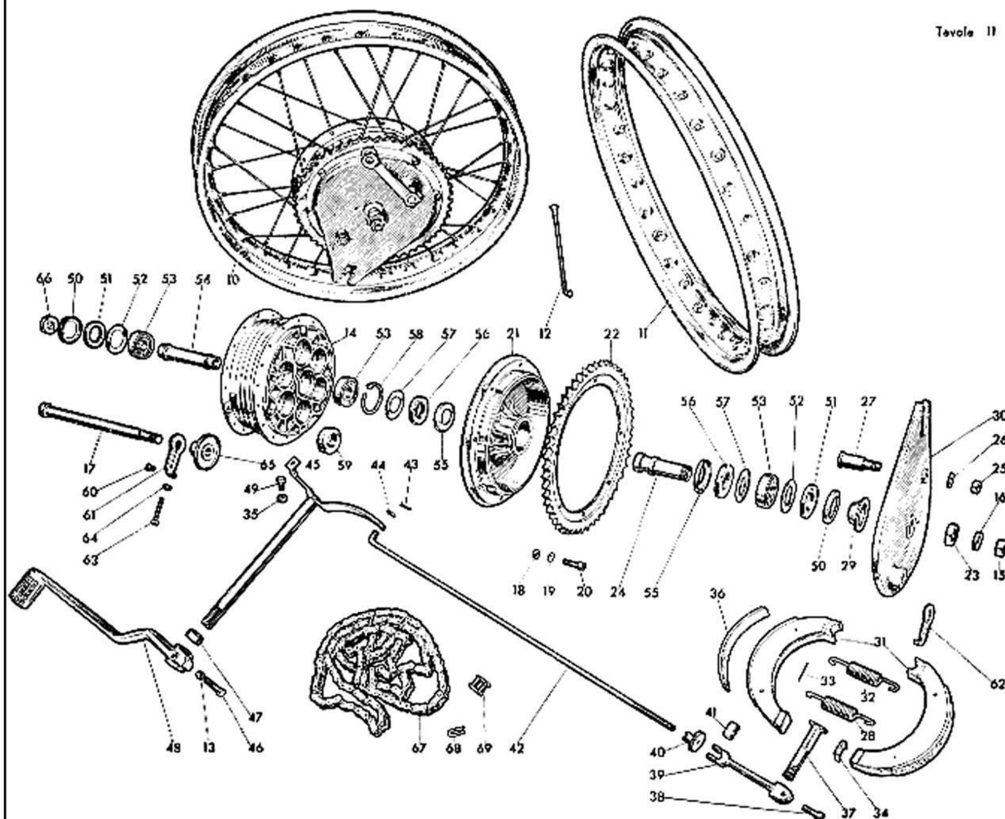
TAV. 11 COMPLESSO : Motociclo GRUPPO : Ruote SOTTOCOMPLESSO: Telaio - Sospensioni - Ruote SOTTOGRUPPO: Ruota - Mozzo - Freno anteriore e comando
