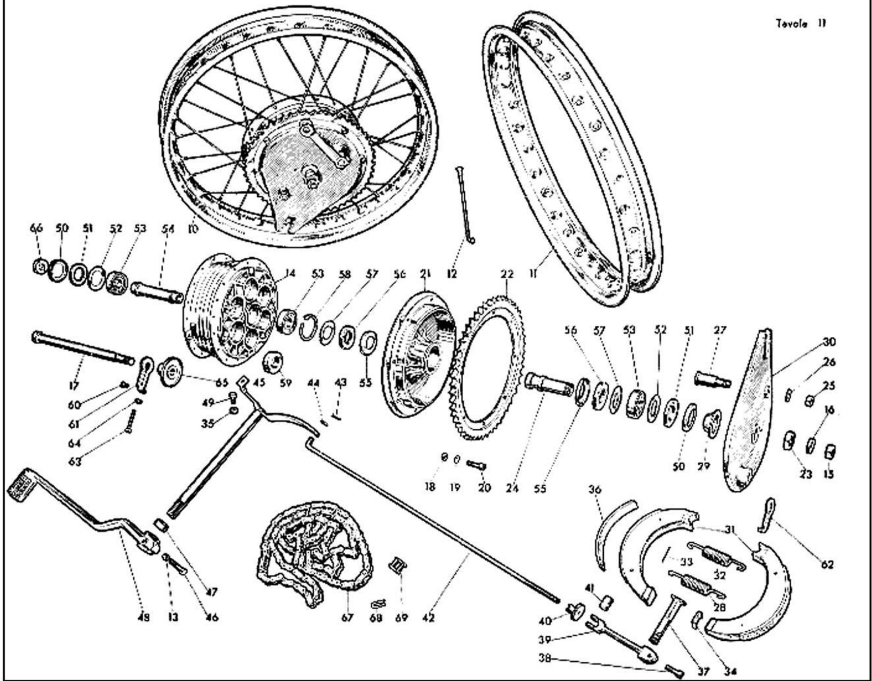
TAV. 11 COMPLESSO : Motociclo GRUPPO : Ruote SOTTOCOMPLESSO: Telaio - Sospensioni - Ruote SOTTOGRUPPO: Ruota - Mozzo - Freno anteriore e comando
