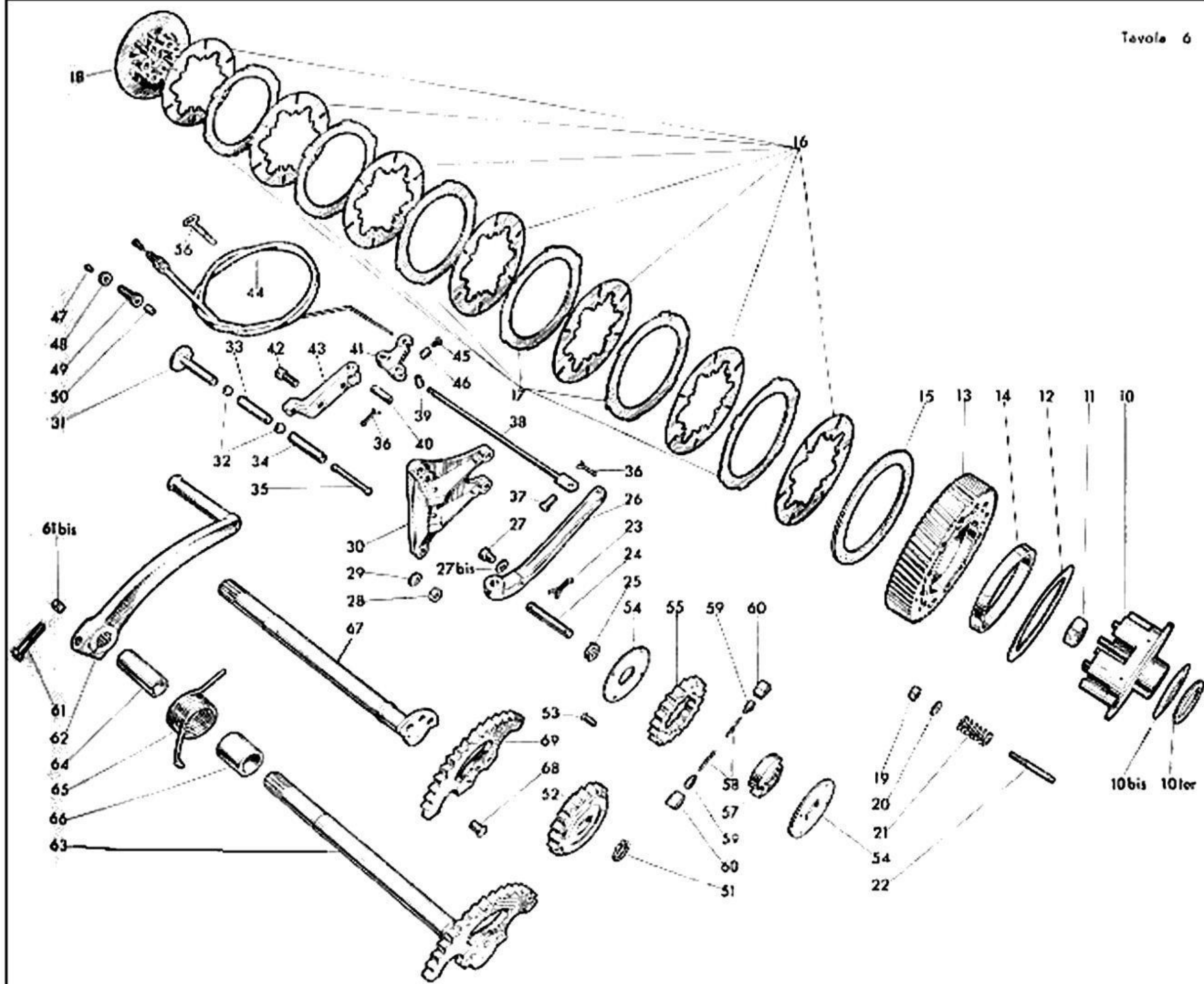
TAV. 6 COMPLESSO : Motociclo GRUPPO : Innesto e avviamento SOTTOCOMPLESSO: Trasmissione SOTTOGRUPPO: Innesto a frizione - Comando frizione - Avviamento
