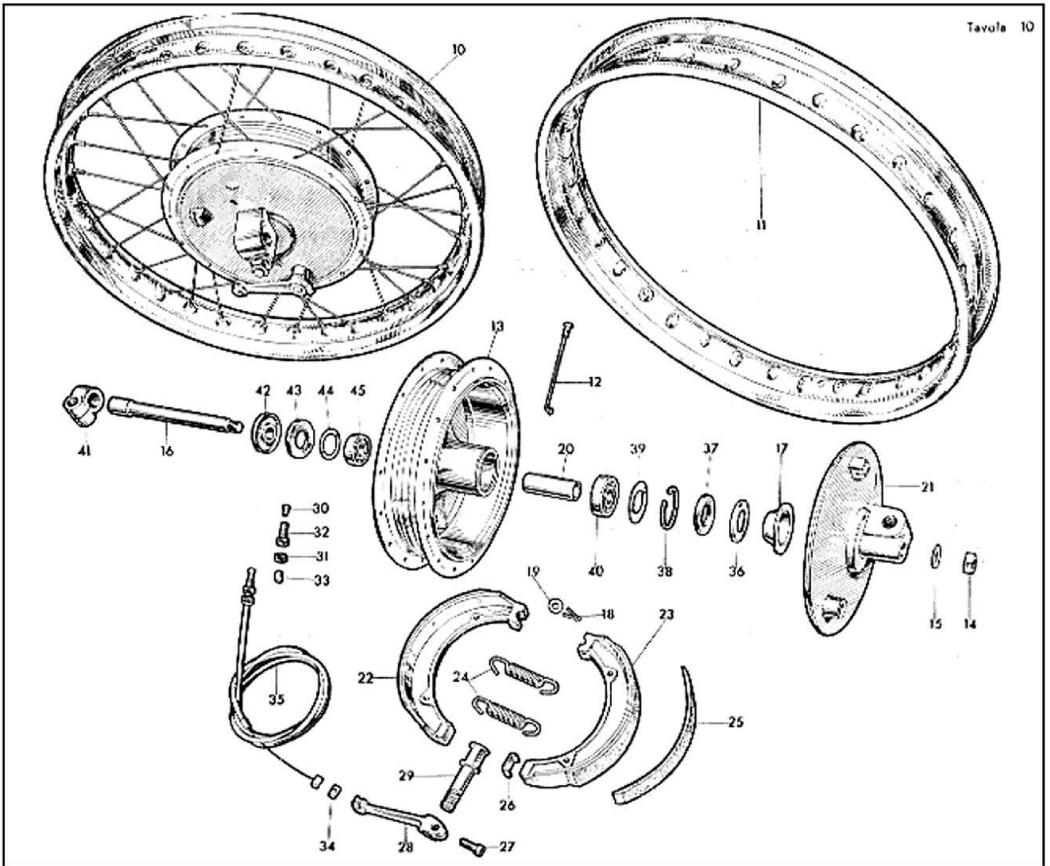
TAV. 10 COMPLESSO : Motociclo GRUPPO : Ruote SOTTOCOMPLESSO: Telaio - Sospensioni - Ruote SOTTOGRUPPO: Ruota - Mozzo - Freno anteriore e comando
