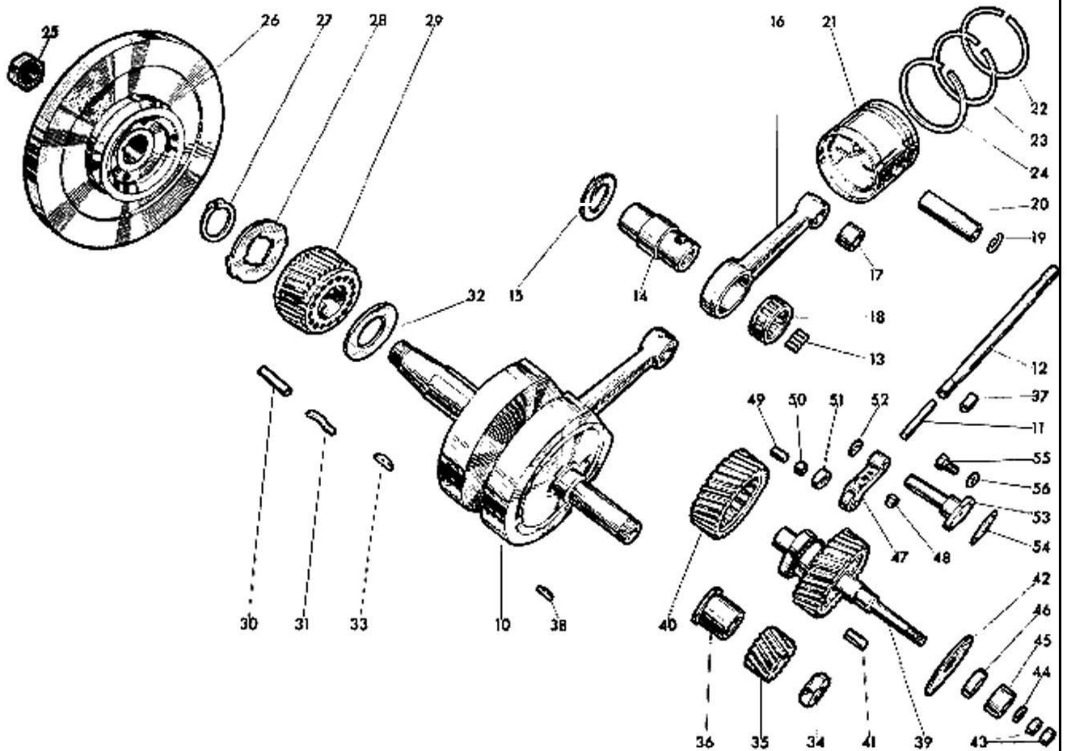
TAV. 3 COMPLESSO : Motociclo SOTTOCOMPLESSO: Motore GRUPPO : Organi principali SOTTOGRUPPO: Albero motore - Biella - Pistone - Albero camme - Gruppo distribuzione
