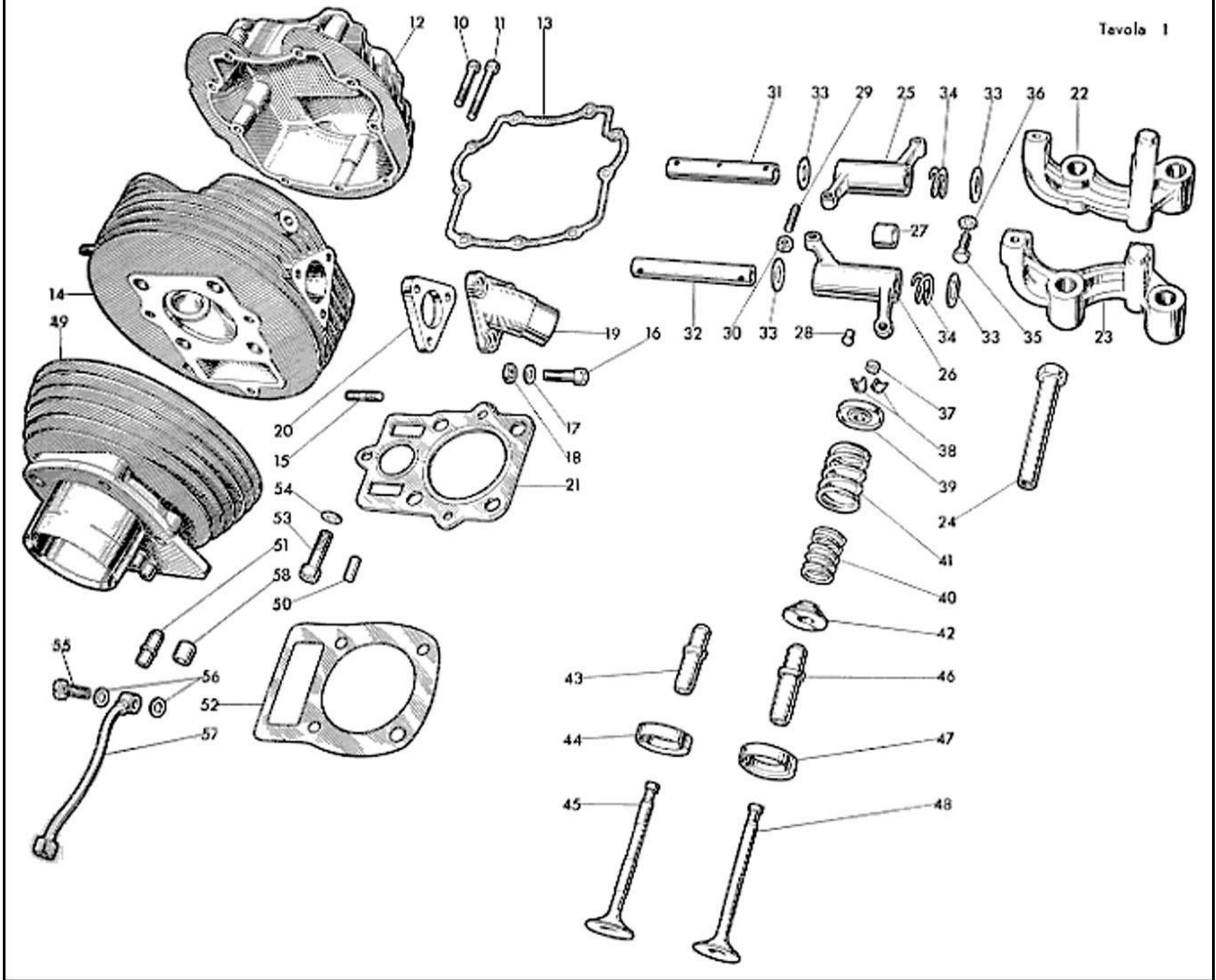
TAV. 1 COMPLESSO : Motociclo GRUPPO : Organi principali SOTTOCOMPLESSO: Motore SOTTOGRUPPO: Cilindro - Testa - Coperchio - Valvole - Bilancieri - Pipa aspirazione
