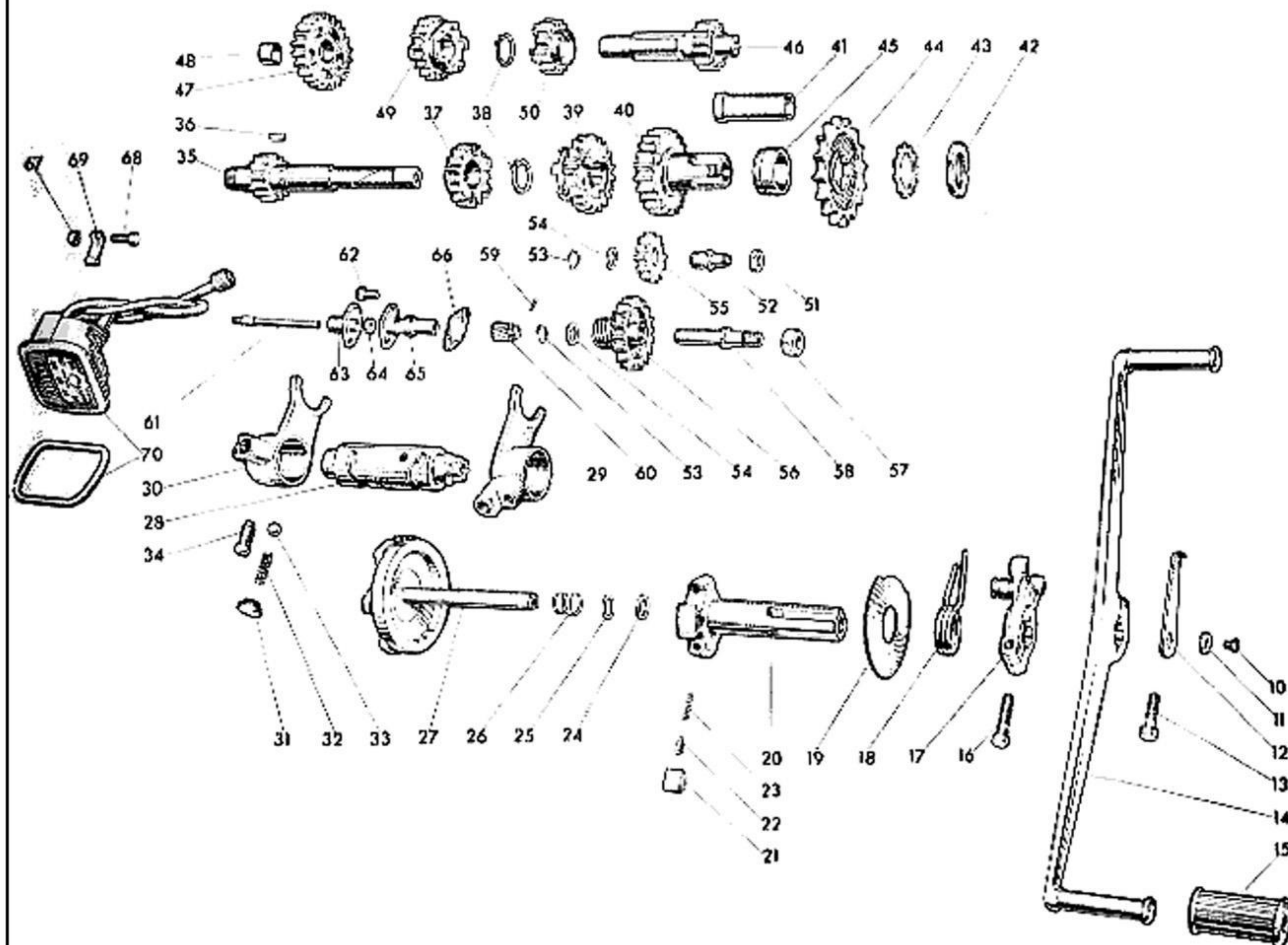
TAV. 7 COMPLESSO : Motociclo GRUPPO : Cambio SOTTOCOMPLESSO: Trasmissione SOTTOGRUPPO: Ingranaggi - Alberi e comando del cambio - Contachilometri
