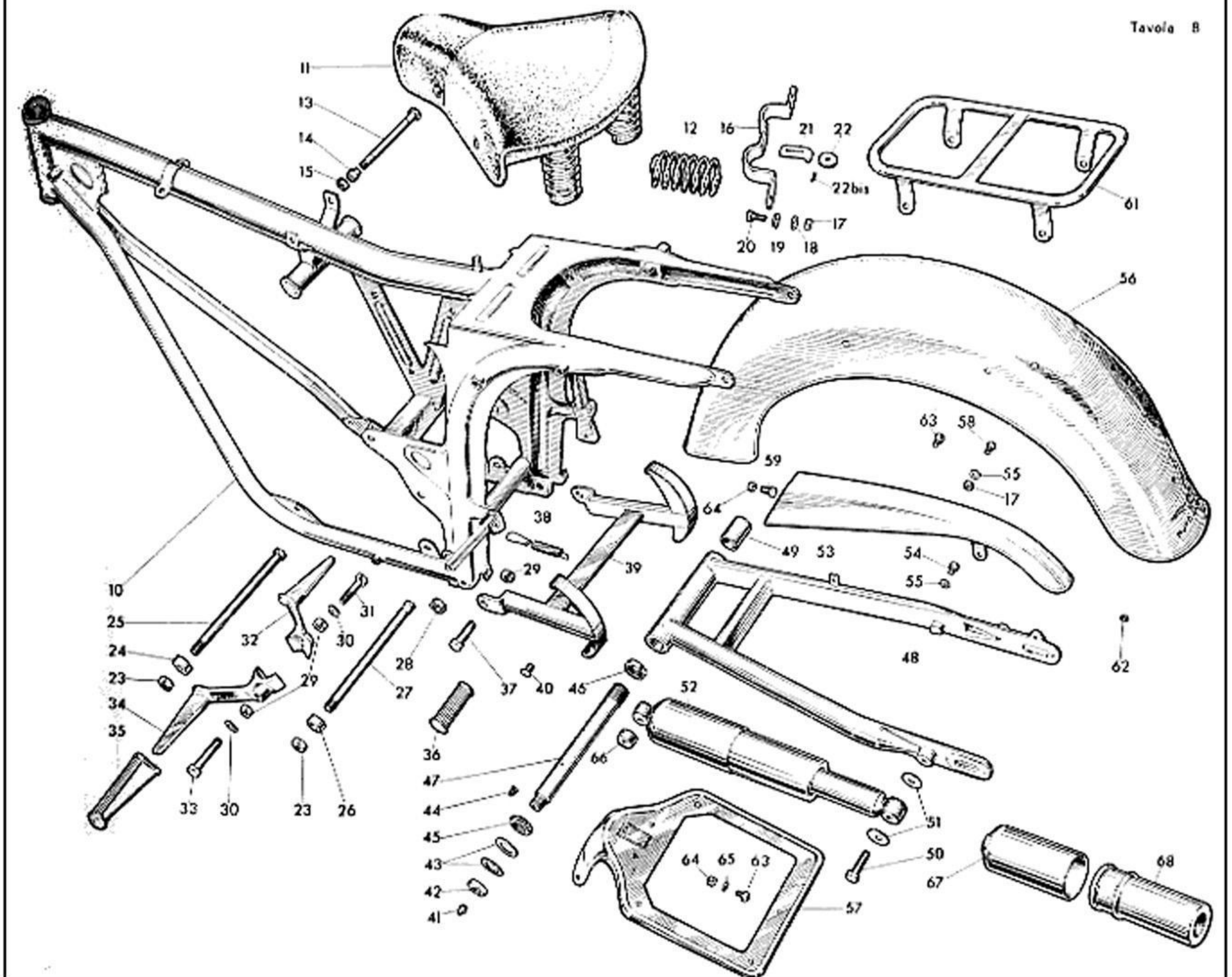
TAV. 8 COMPLESSO : Motociclo GRUPPO : Telaio SOTTOCOMPLESSO: Telaio - Sospensioni - Ruote SOTTOGRUPPO: Telaio - Parafango poster. - Sella - Portapacchi Cavall. - Forcellone oscillante - Molleggio posteriore
