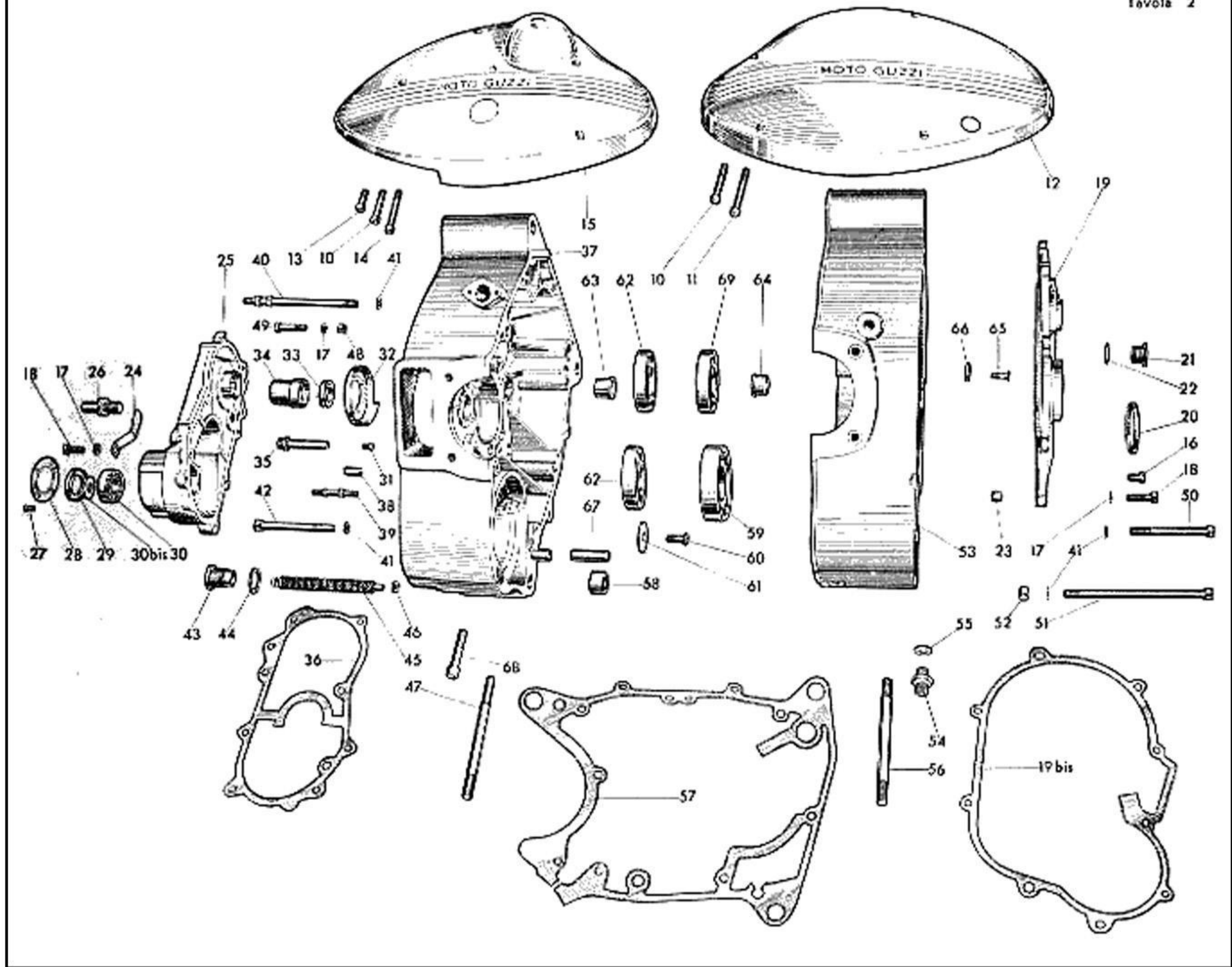
TAV. 2 COMPLESSO : Motociclo SOTTOCOMPLESSO: Motore GRUPPO : Organi principali SOTTOGRUPPO: Basamento - Coperchi
