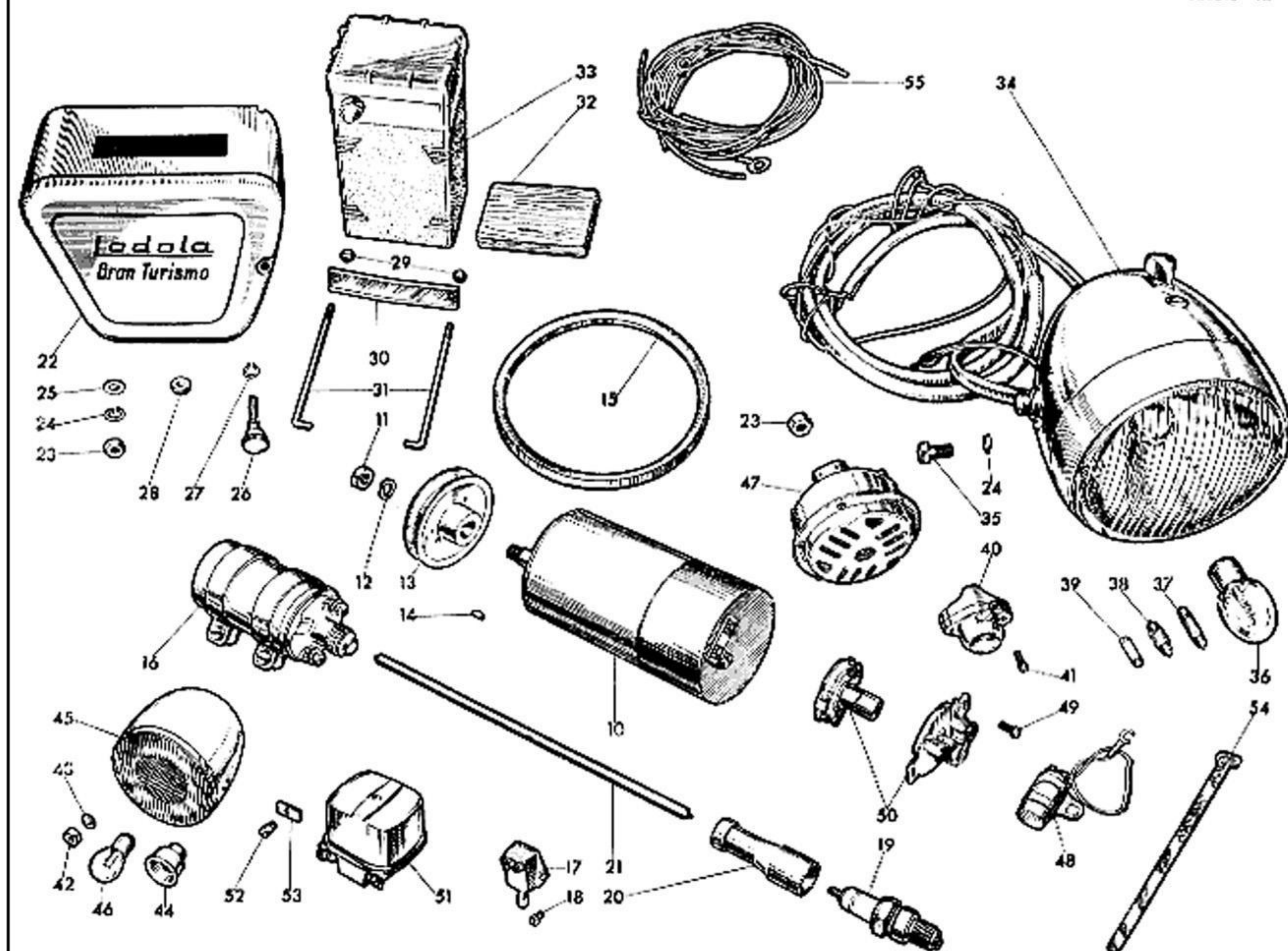
TAV. 12 COMPLESSO : Motociclo GRUPPO : Generatore - Accensione - Illuminazione ed accessori SOTTOCOMPLESSO: Impianto elettrico SOTTOGRUPPO: Dinamo - Bobina - Ruttore - Batteria - Faro anteriore - Fanalino posteriore - Tromba elettrica - Regolatore
