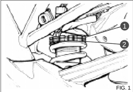
FIG. 1 1. Controghiera 1. Riug nut 1. Contre-écrou 1. Gegennutmutter 1. Contravirola 2. Ghiera di registro 2. Adjusting nut 2. Ecrou de réglage 2. Einstellungnutmutter 2. Virula de regulacón
