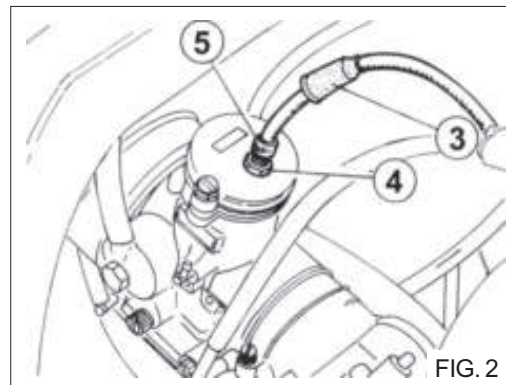
FIG. 2 3. Cappuccio 3. Rubber cap 3. Bouchon de charge et contrôle du niveau 3. Kappe 3. Casquete 4. Controdado 4. Lock nut 4. Bouchon de vidange huile 4. Gegenmutter 4. Contratuerca 5. Vite di registro 5. Adjusting screw 5. Vis de réglage 5. Einstellschraube 5. Tornillo de ajuste
