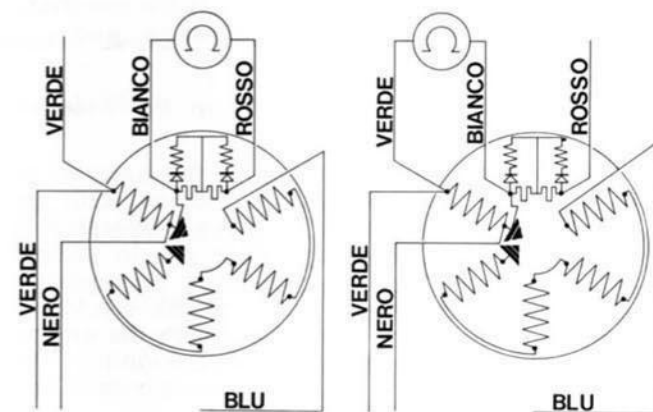
Fig. 20 6 pole flywheel magneto (equipment with turn signal lamps). Volante magnético de 6 polos (instalación con intermitentes).
