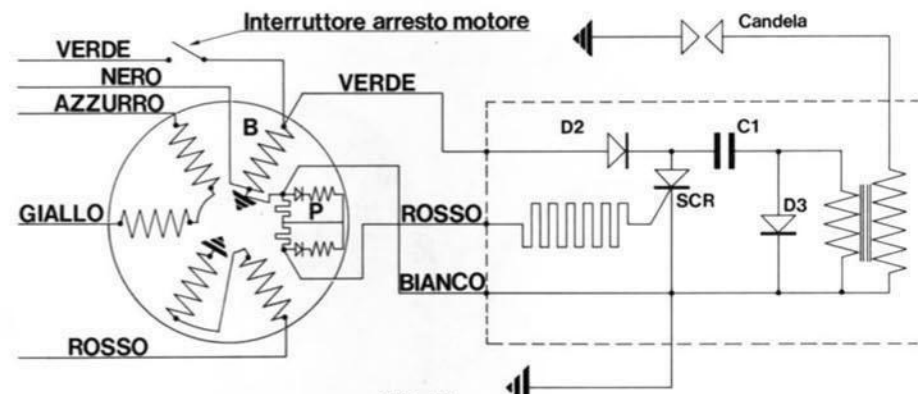
Fig. 11 6 pole flywheel magneto - Volante magnético de 6 polos (equipment without turn signal lamps) - (instalación sin intermitentes).
