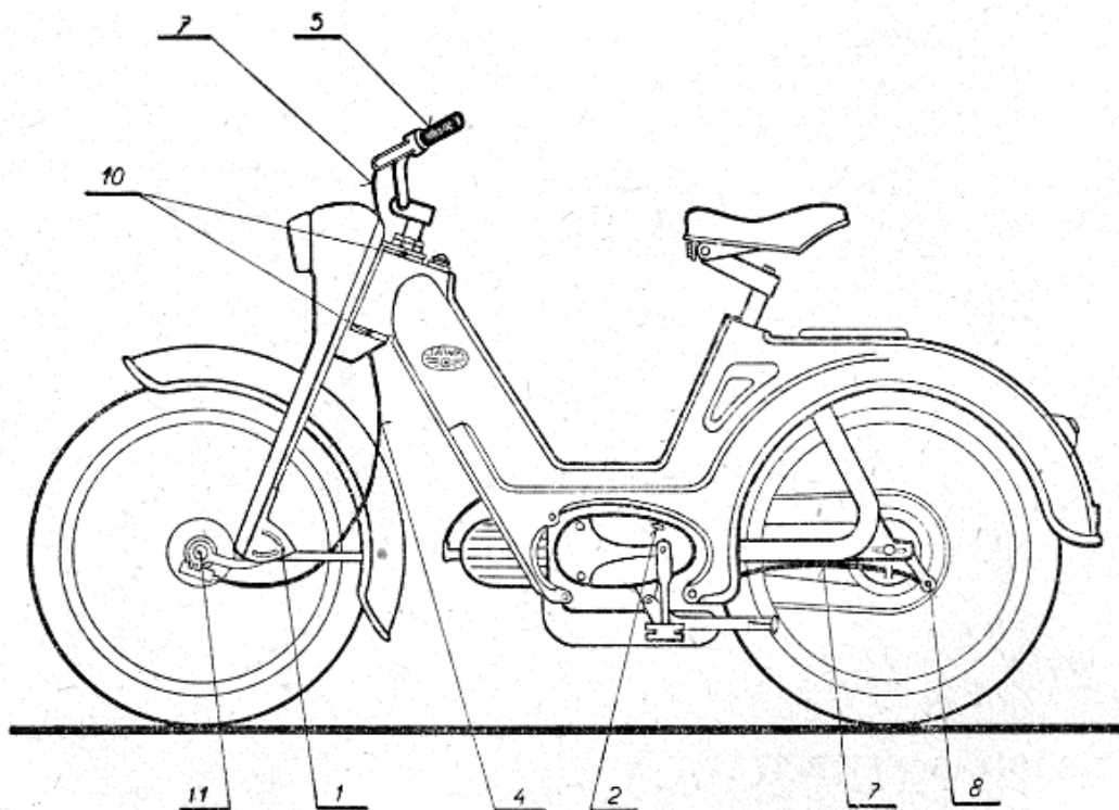
Obr. 8. Mazací plán - levá strana.
