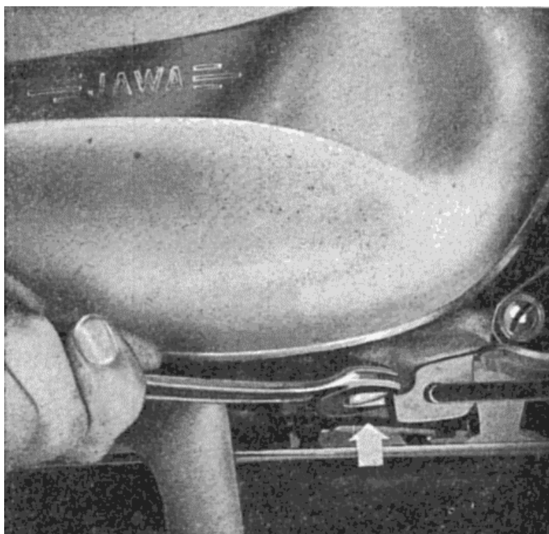
Obr. 10. Vypouštěcí šroub oleje z převodovky.
