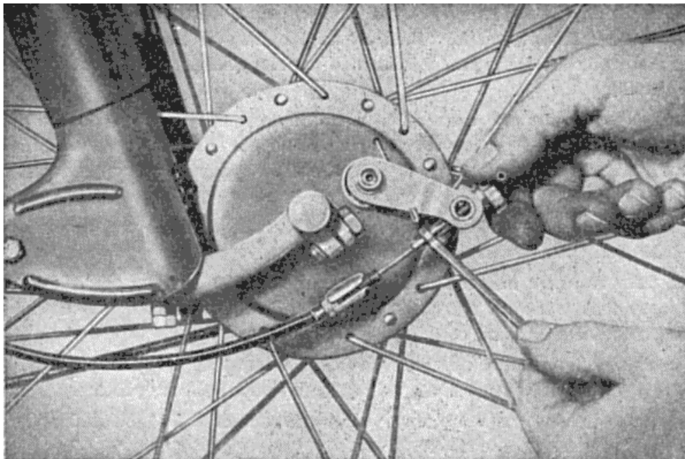
Obr. 12. Seřízení brzdy.
