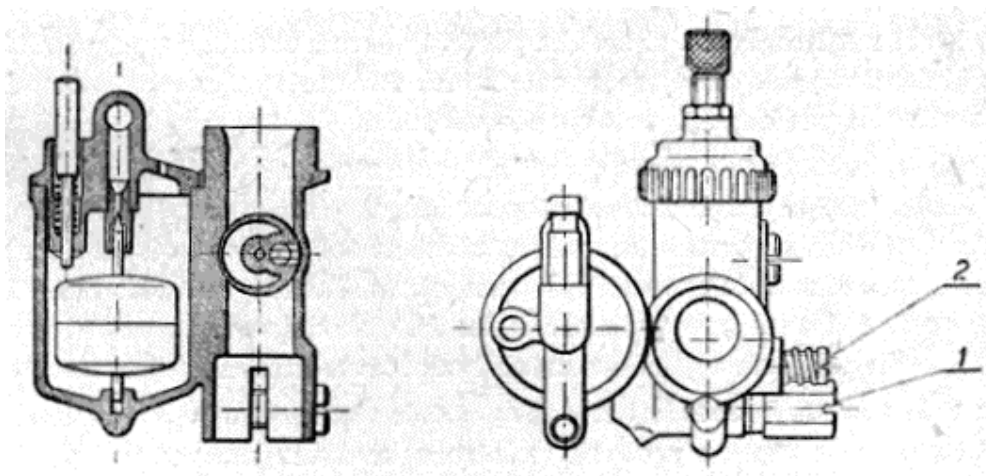
Obr. 16. Karburátor v řezu (1 - hlavní tryška; 2 - šroub volnoběhu).
