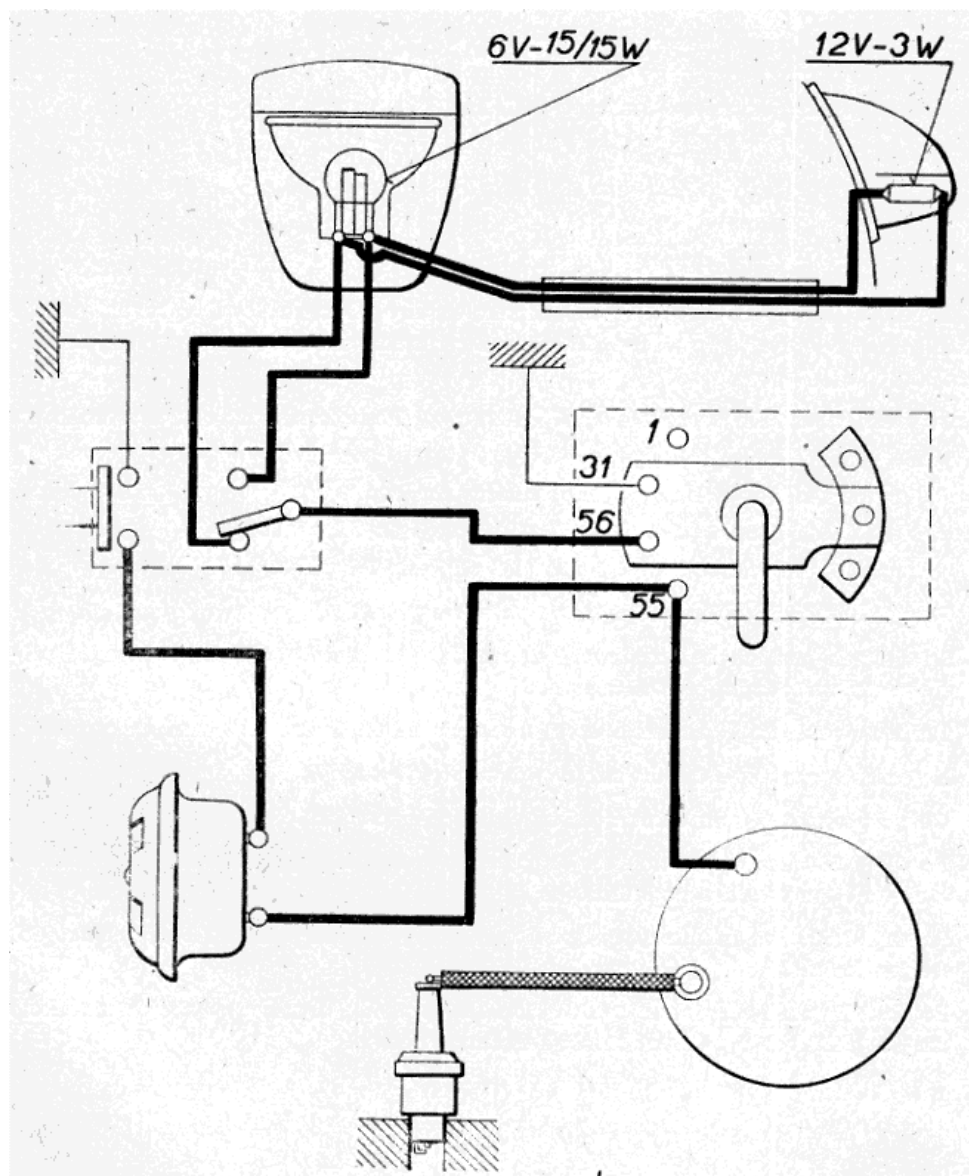
Obr. 3. Schema elektrického zapojení mopedu Jawa - 50, typ 551.
