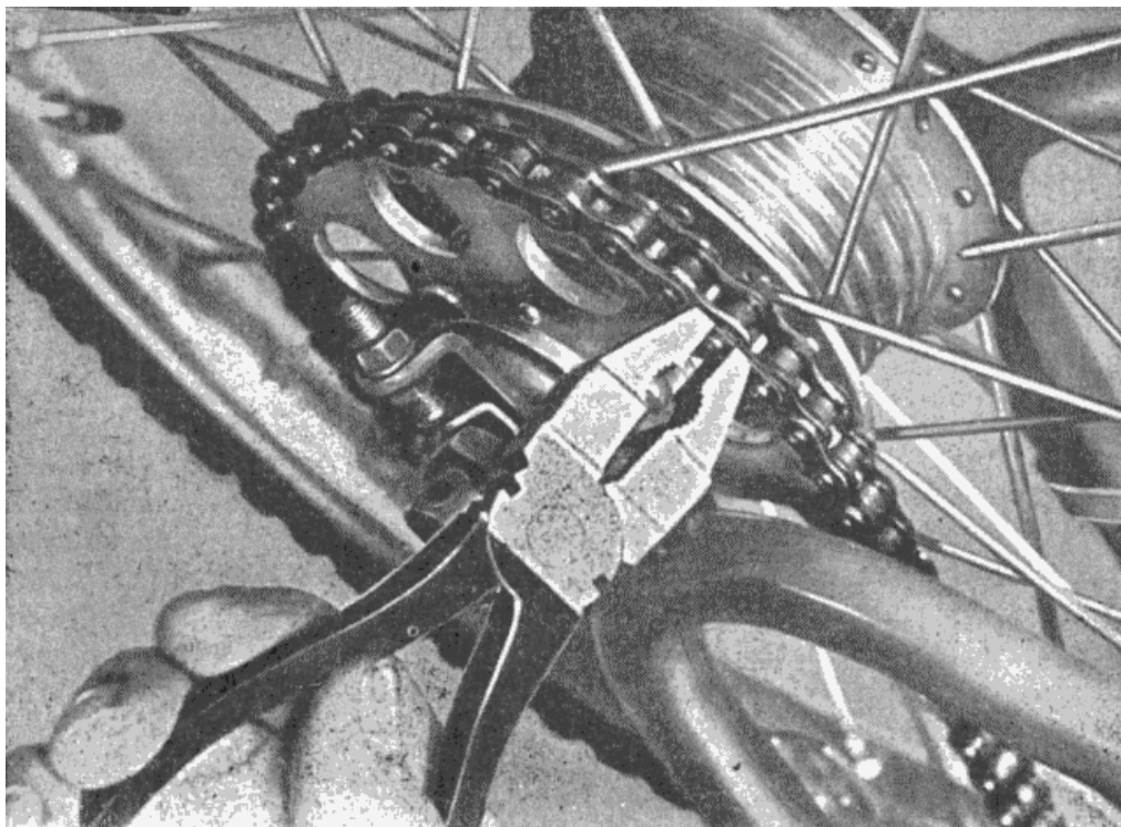
Obr. 11. Uvolnění řetězové spojky.
