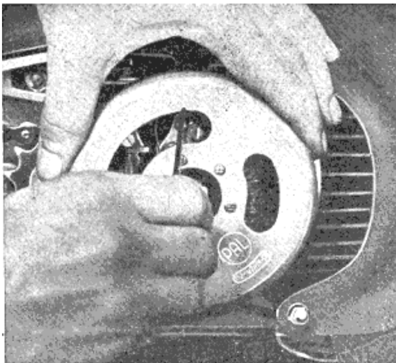
Obr. 17. Měření odtrhu přerušovače.
