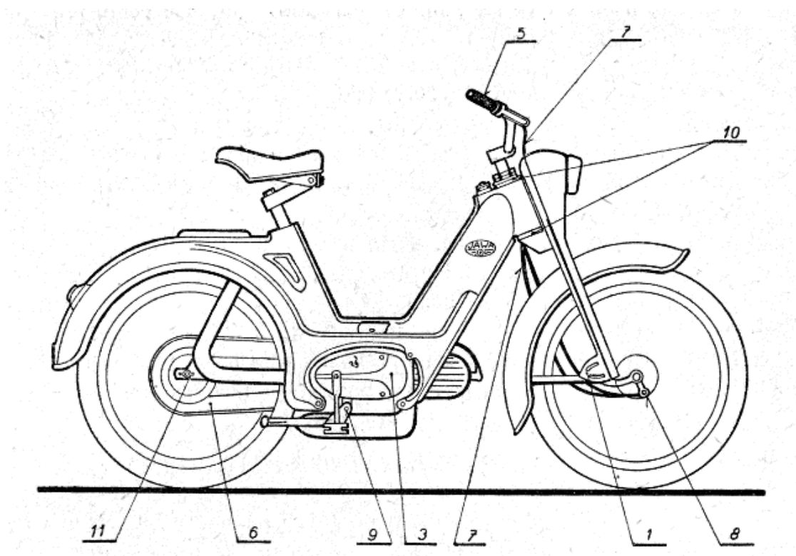
Obr. 9. Mazací plán - pravá strana.
