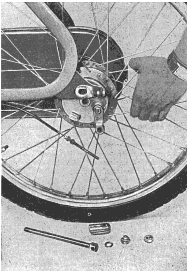
Obr. 18. Vyjmutí zadního kola.
