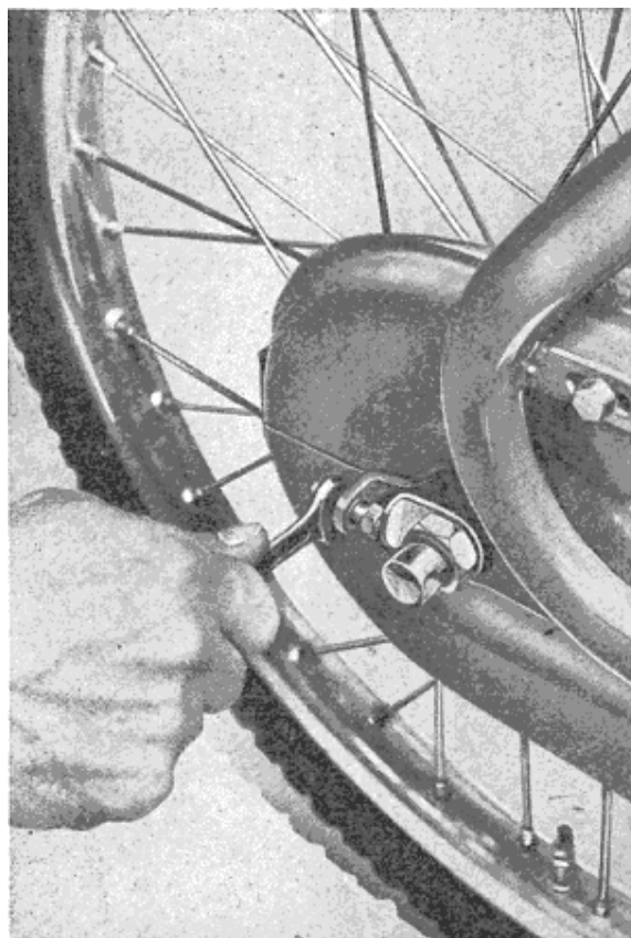
Obr. 14. Napínání řetězu.
