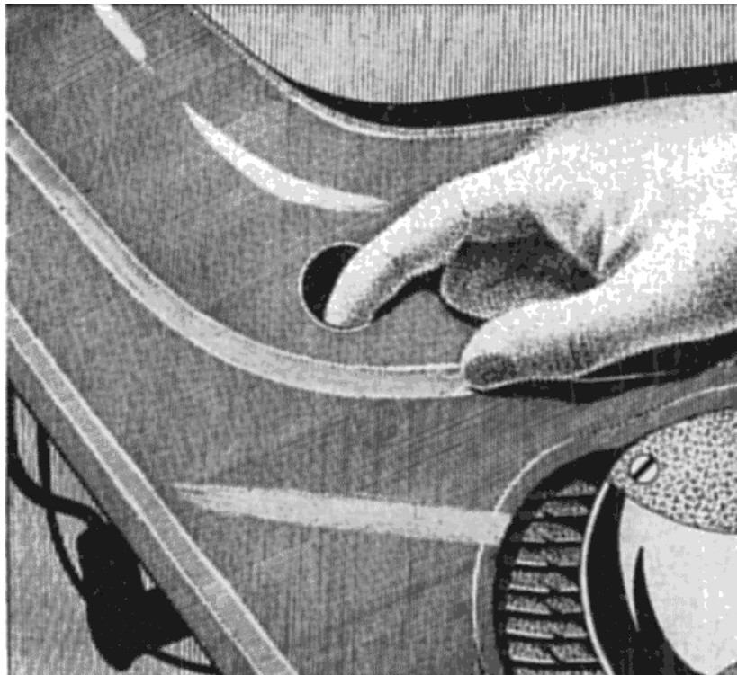
Obr. 6. Přeplavení karburátoru.
