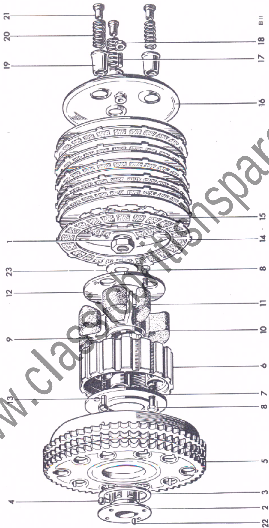
Fig. 14. CLUTCH
