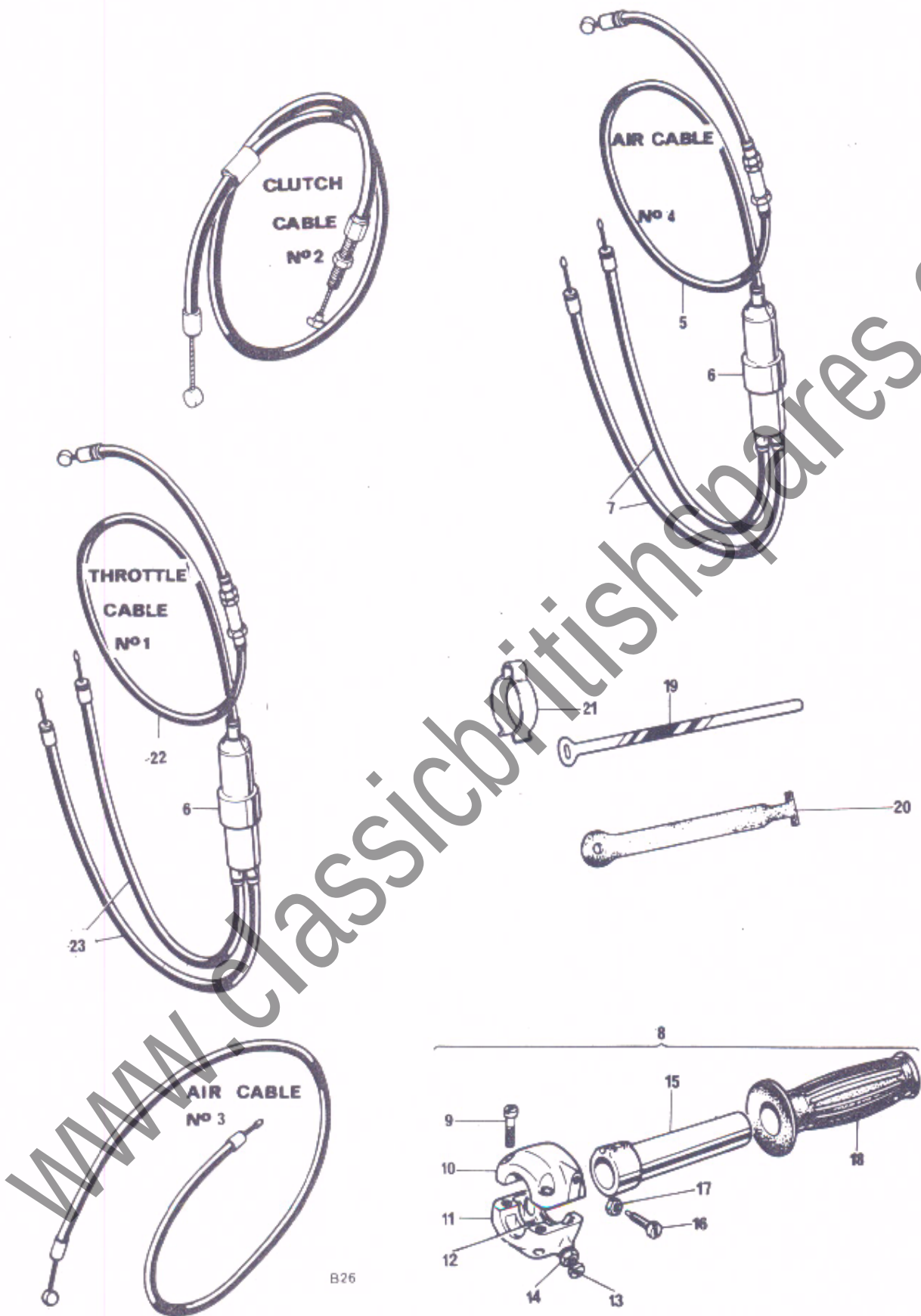
Fig. 30. CONTROL CABLES
