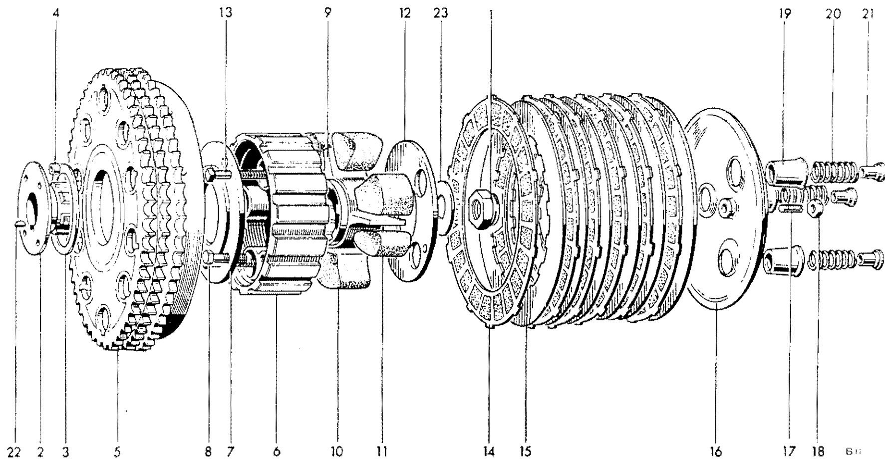
CLUTCH
