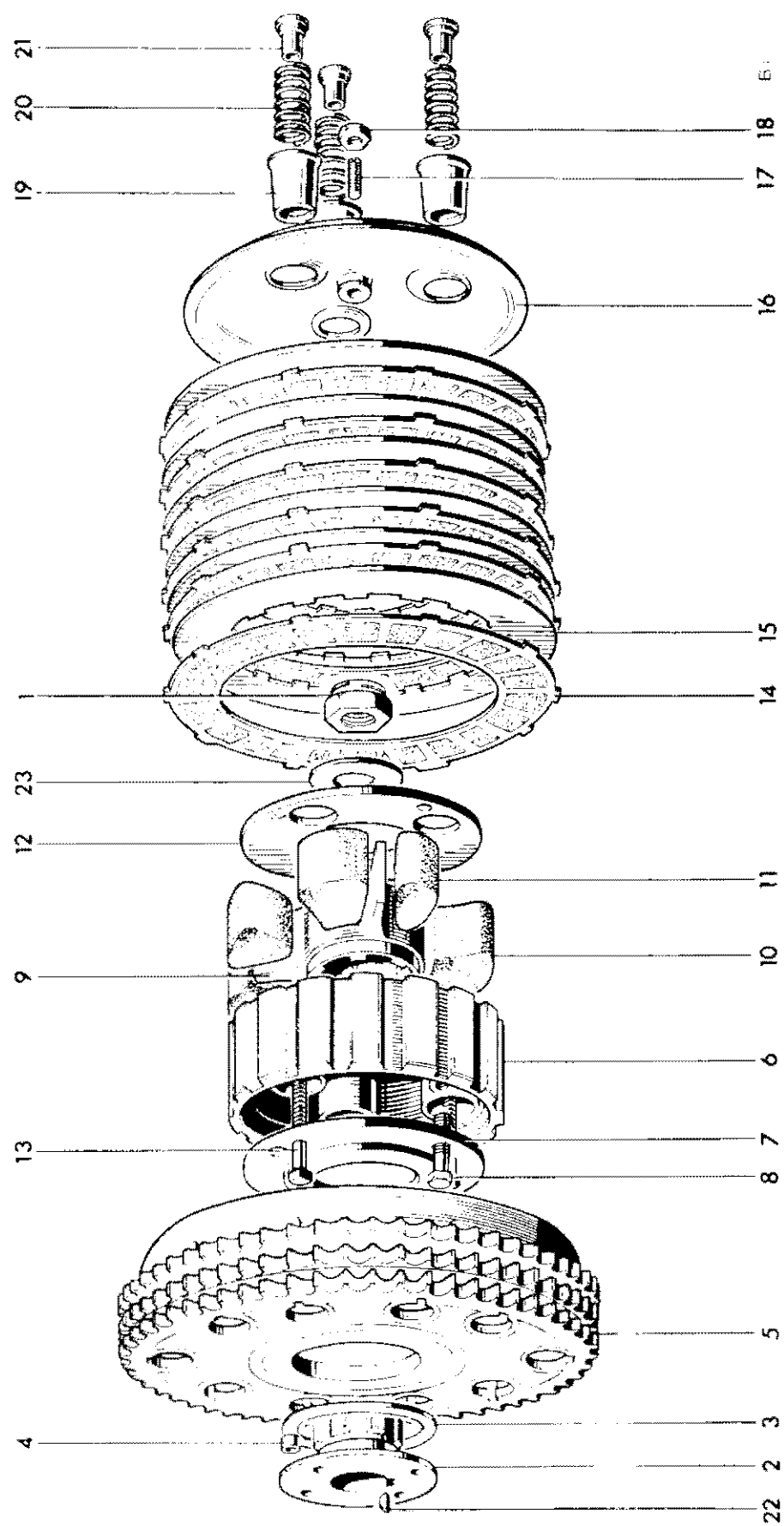
CLUTCH
