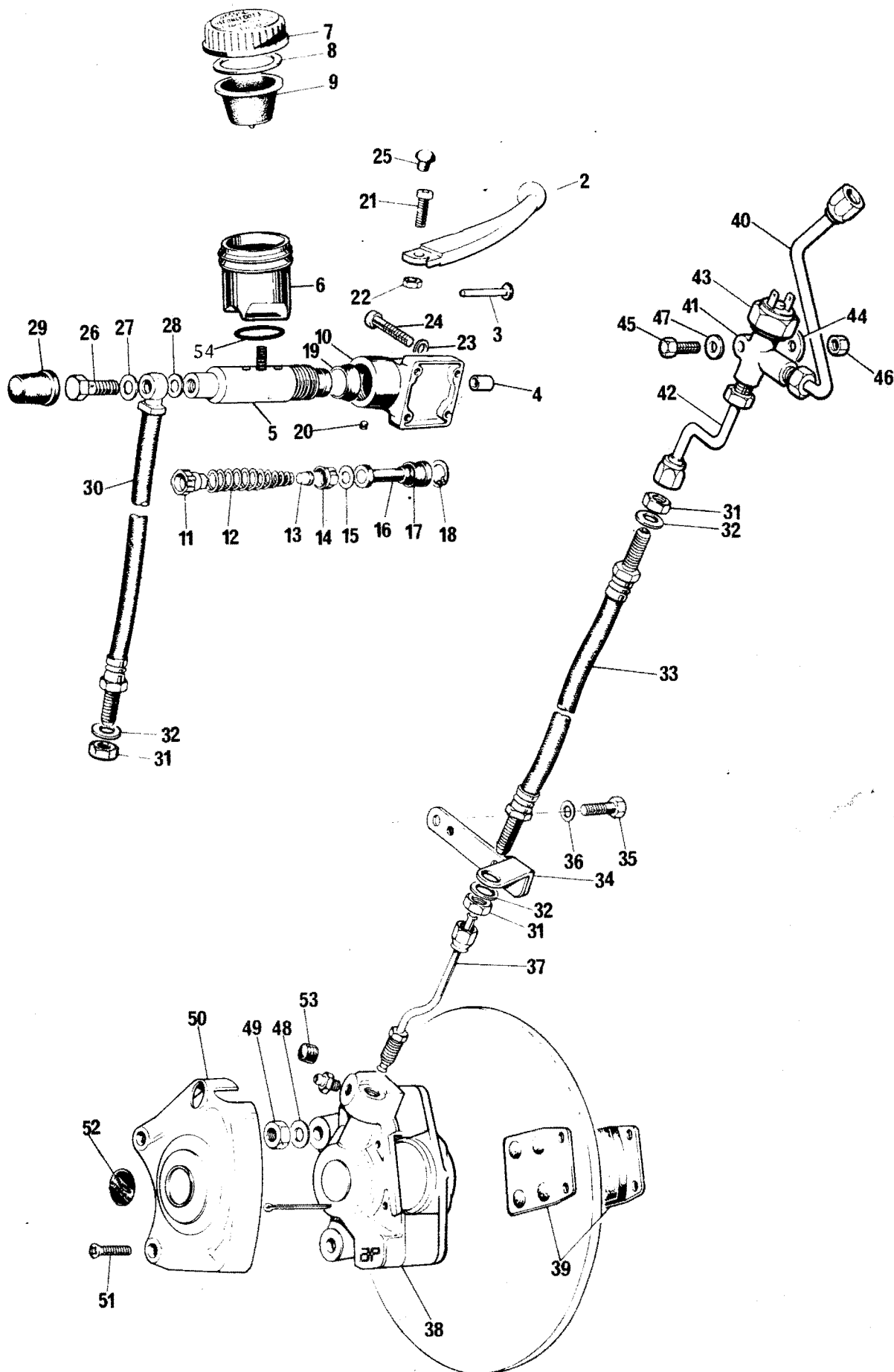
Fig. 23. FRONT BRAKE
