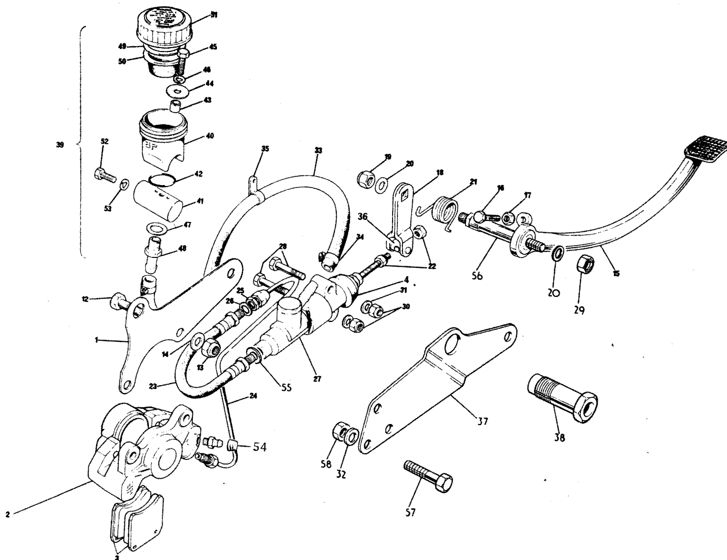
Fig. 25. REAR BRAKE
