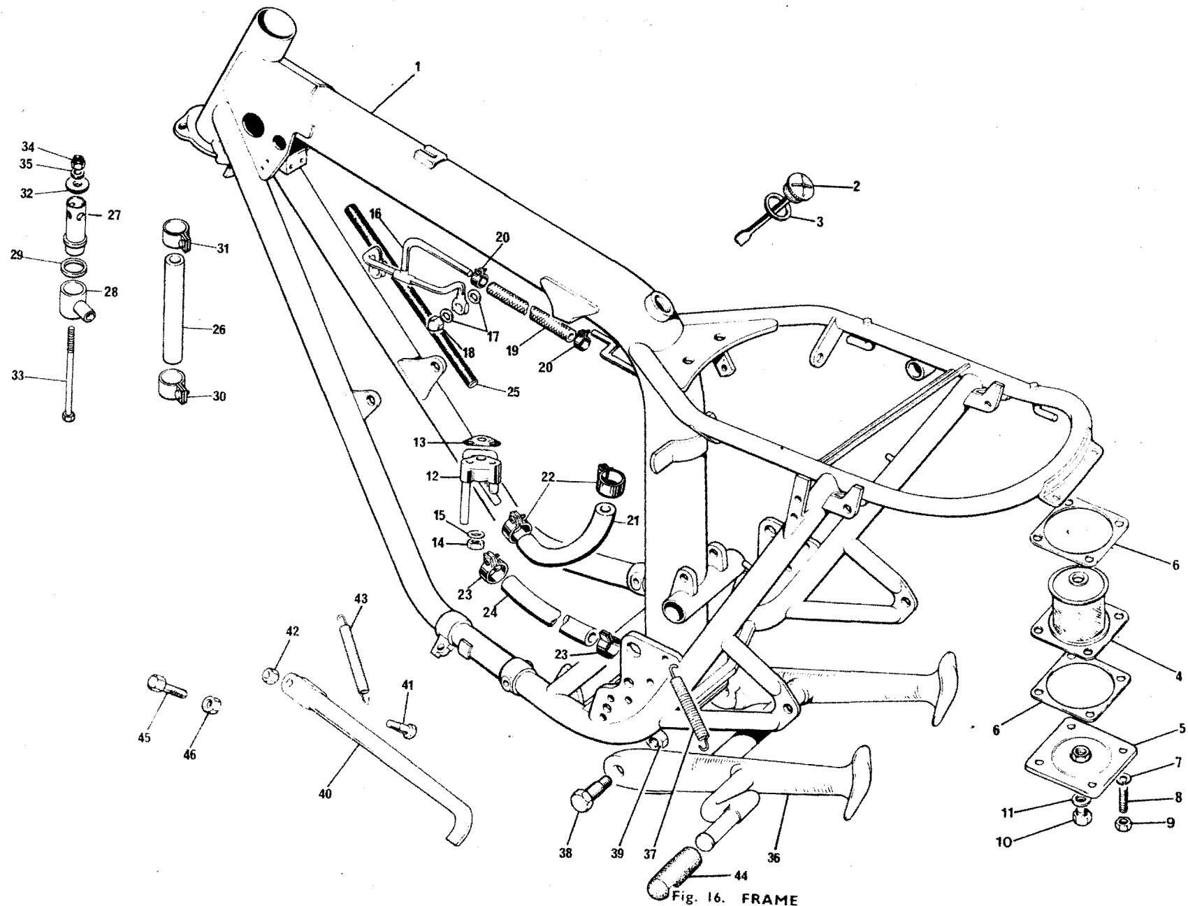
Fig. 16. FRAME
