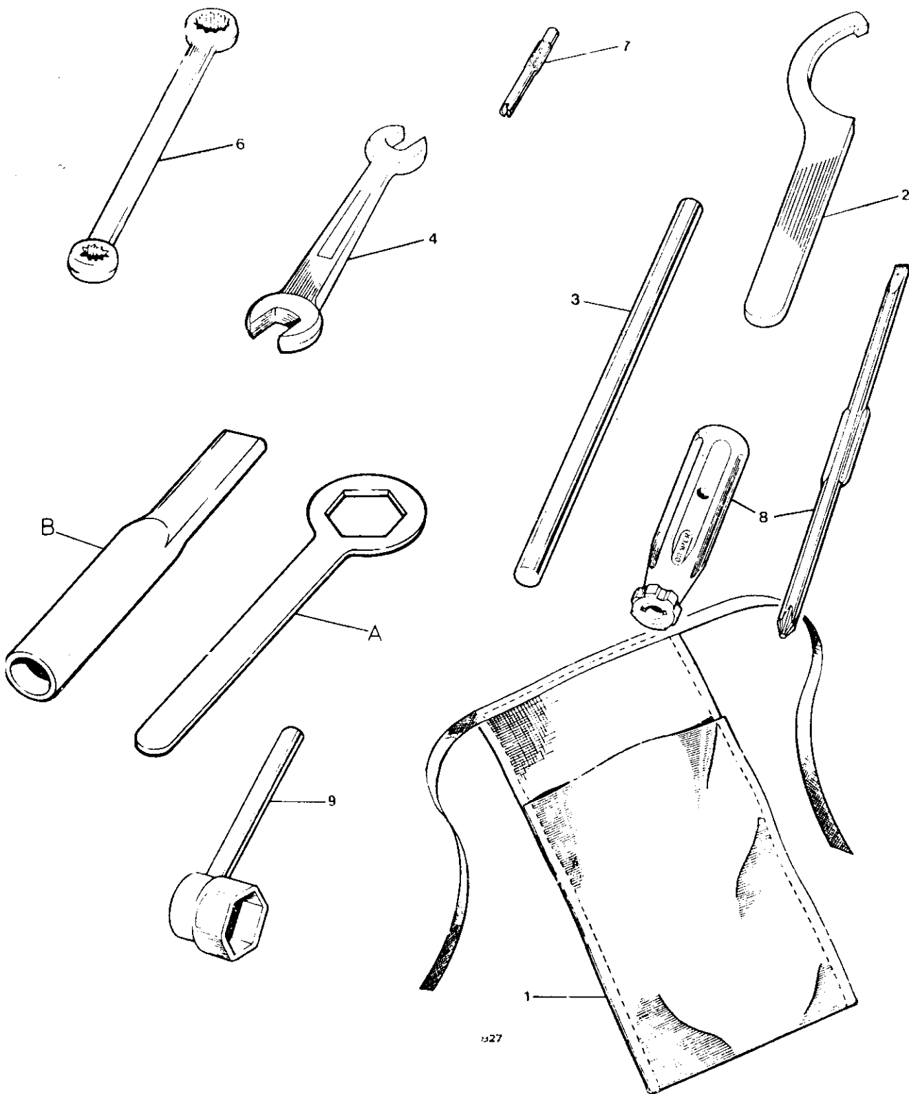
F.g. 31. TOOLKIT
