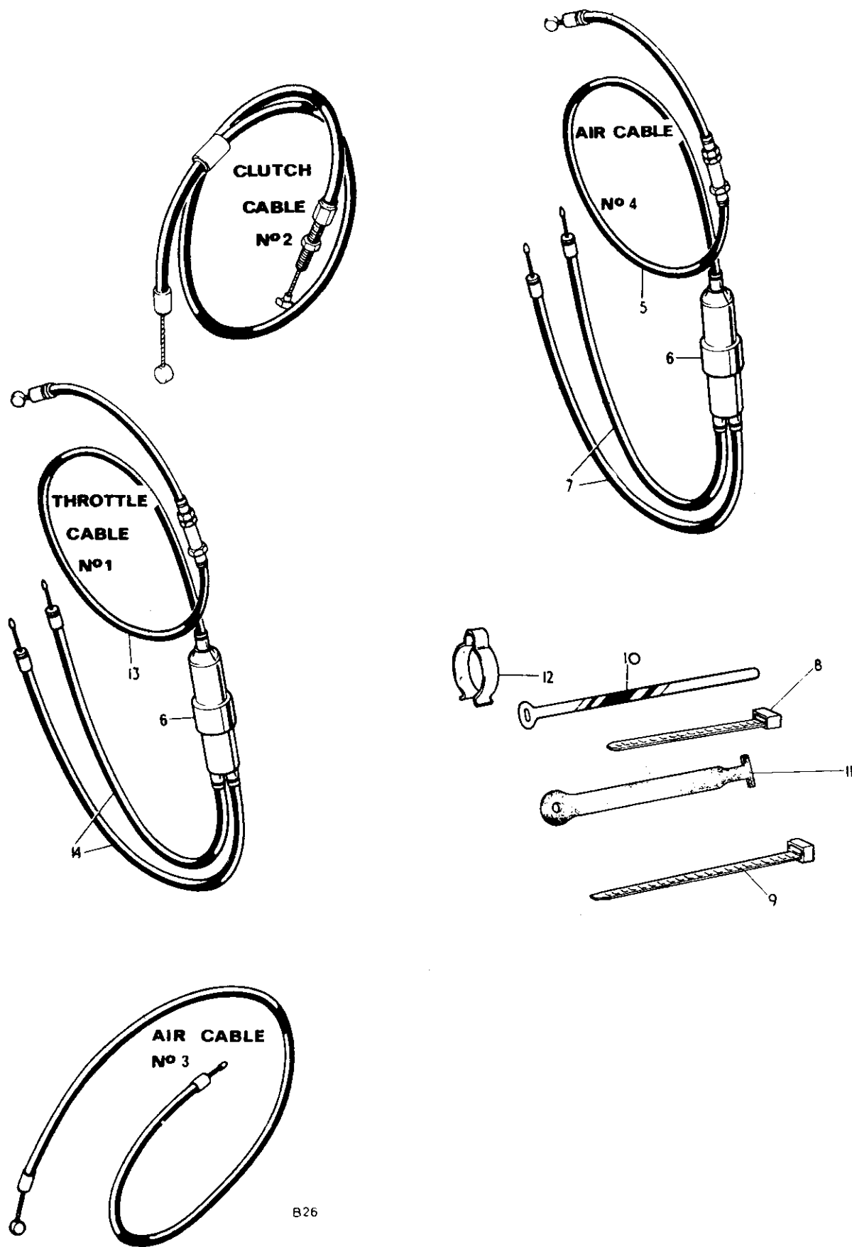
Fig. 30. CONTROL CABLES
