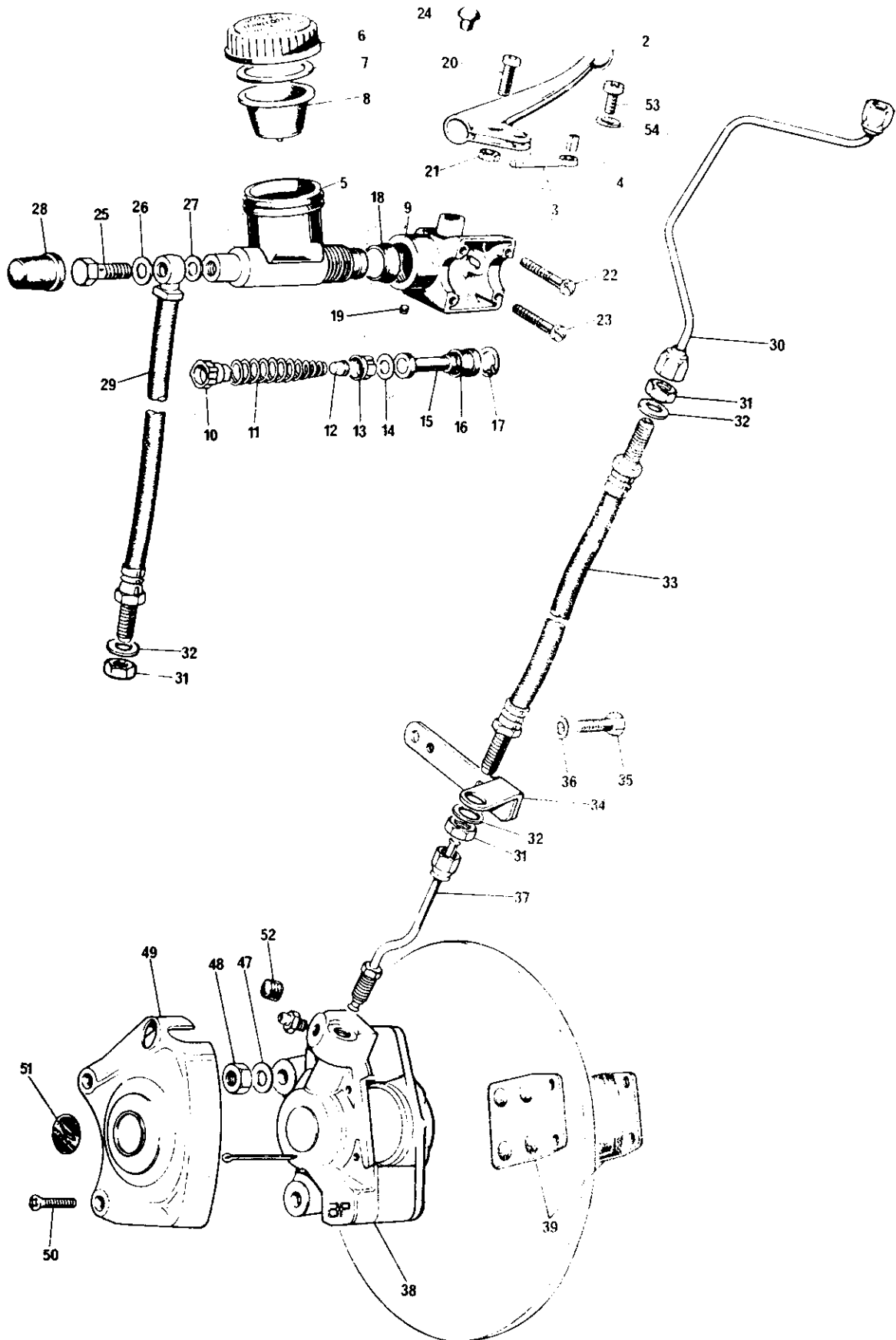
Fig. 23. FRONT BRAKE
