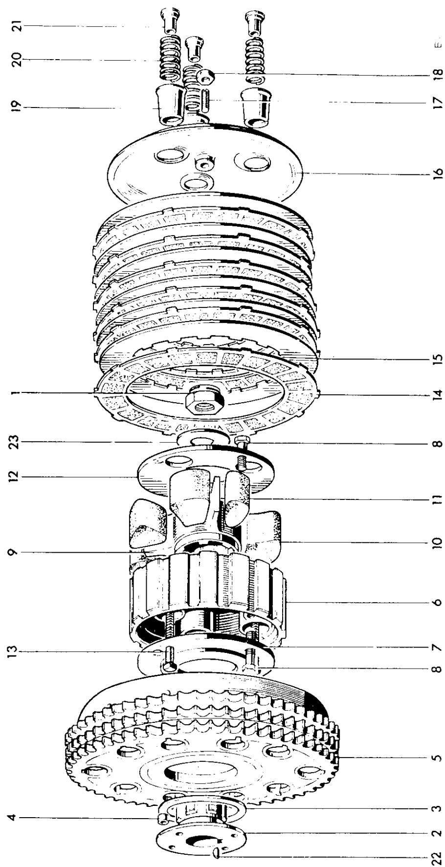
Fig. 14. CLUTCH
