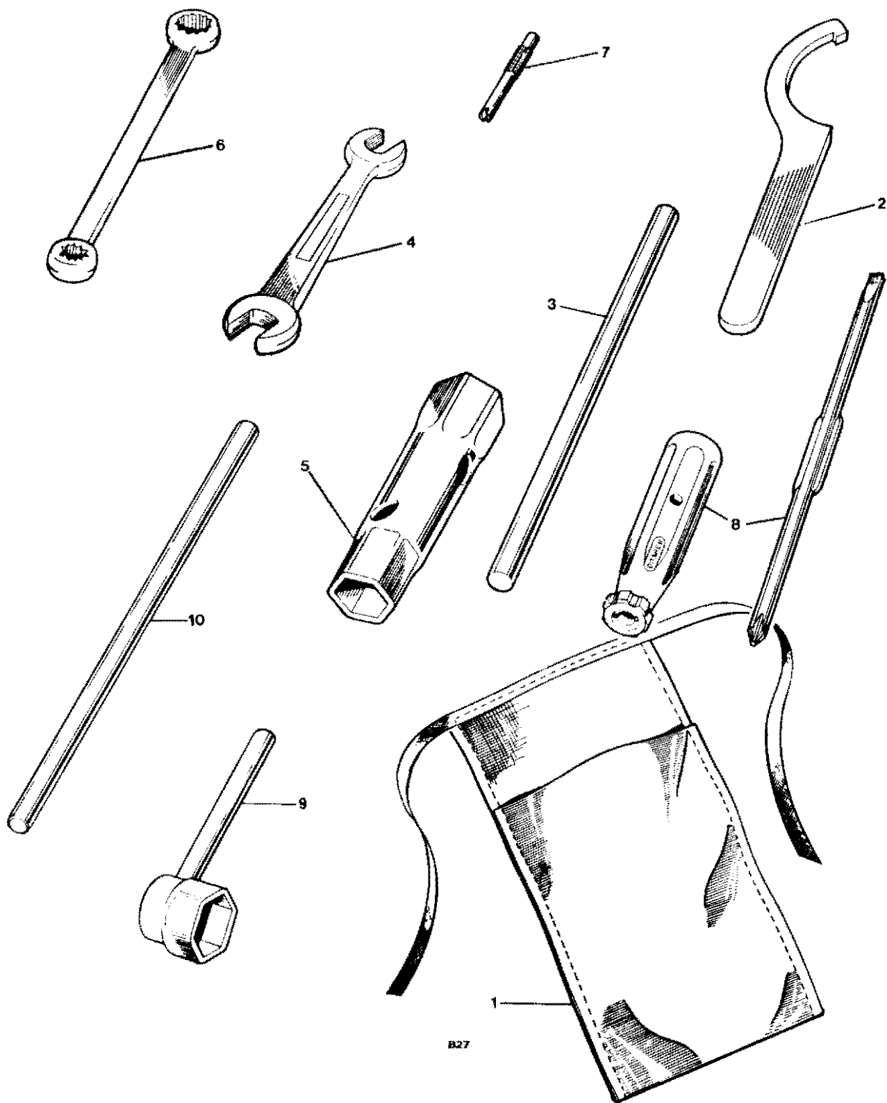
Fig. 31. TOOLKIT
