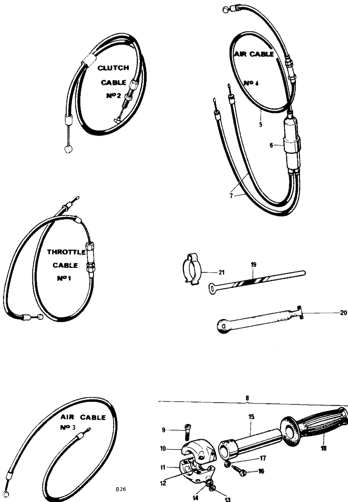
Fig. 30. CONTROL CABLES
