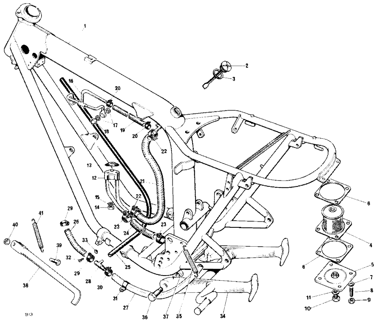
16. FRAME
