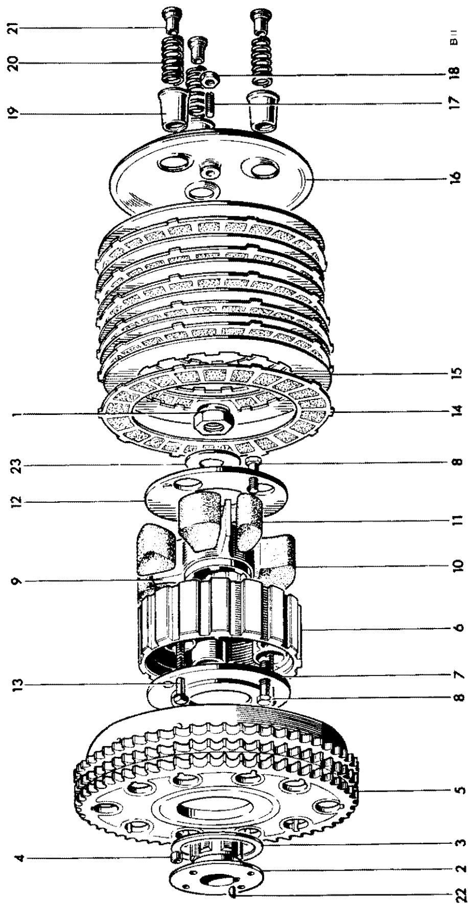
Fig. 14. CLUTCH
