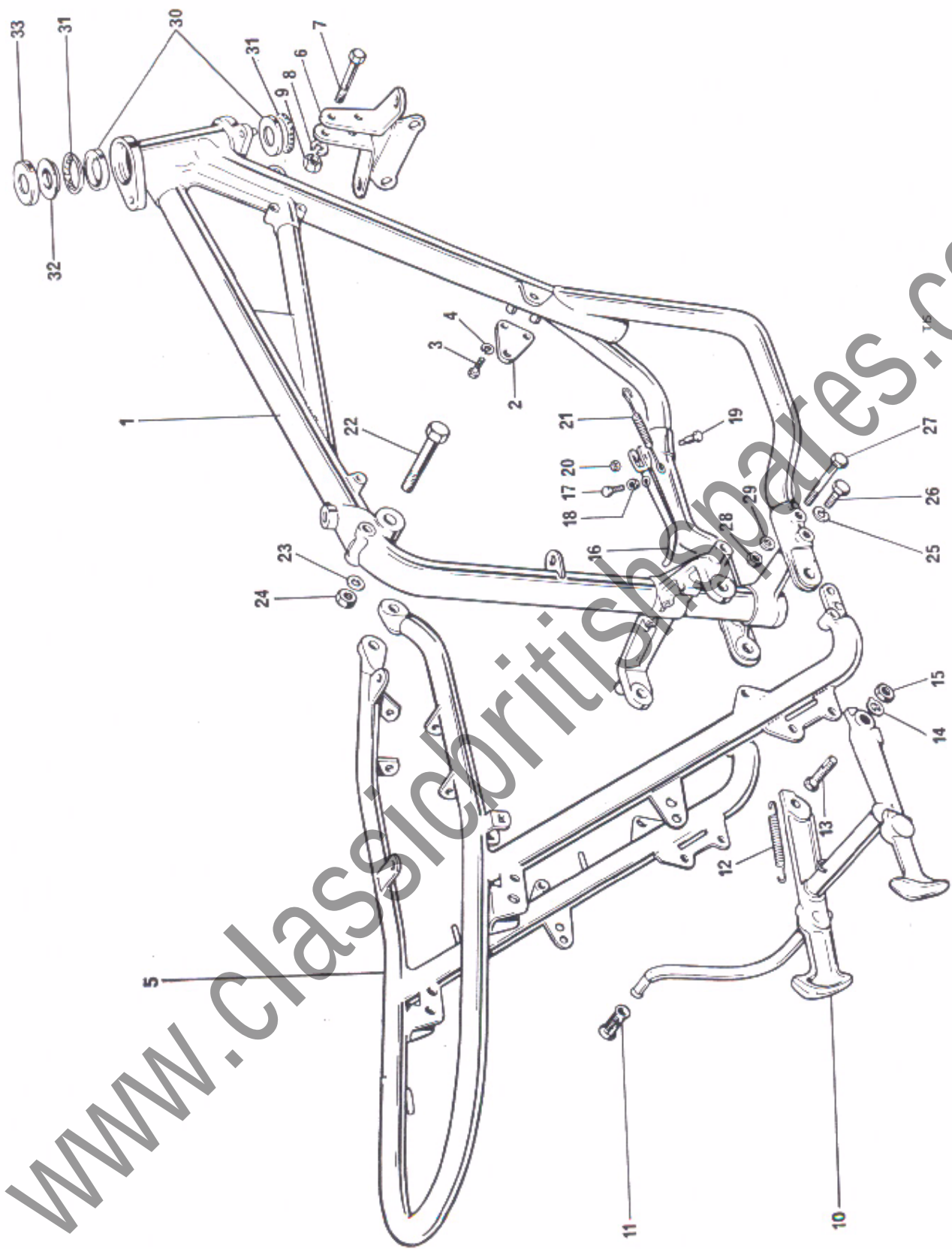
Fig. 15. FRAME
