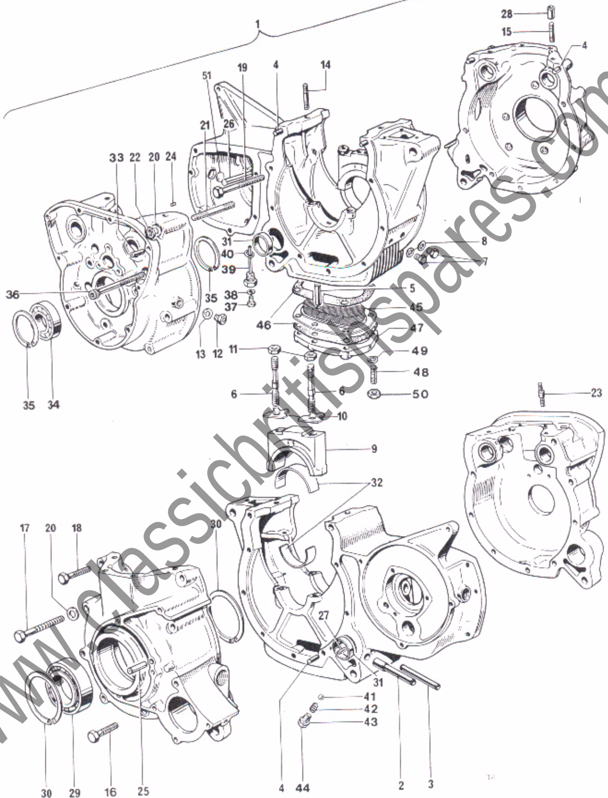
Fig. 2. CRANKCASES
