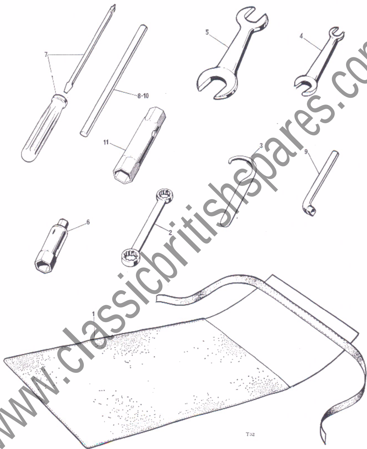
Fig. 32. TOOLKIT
