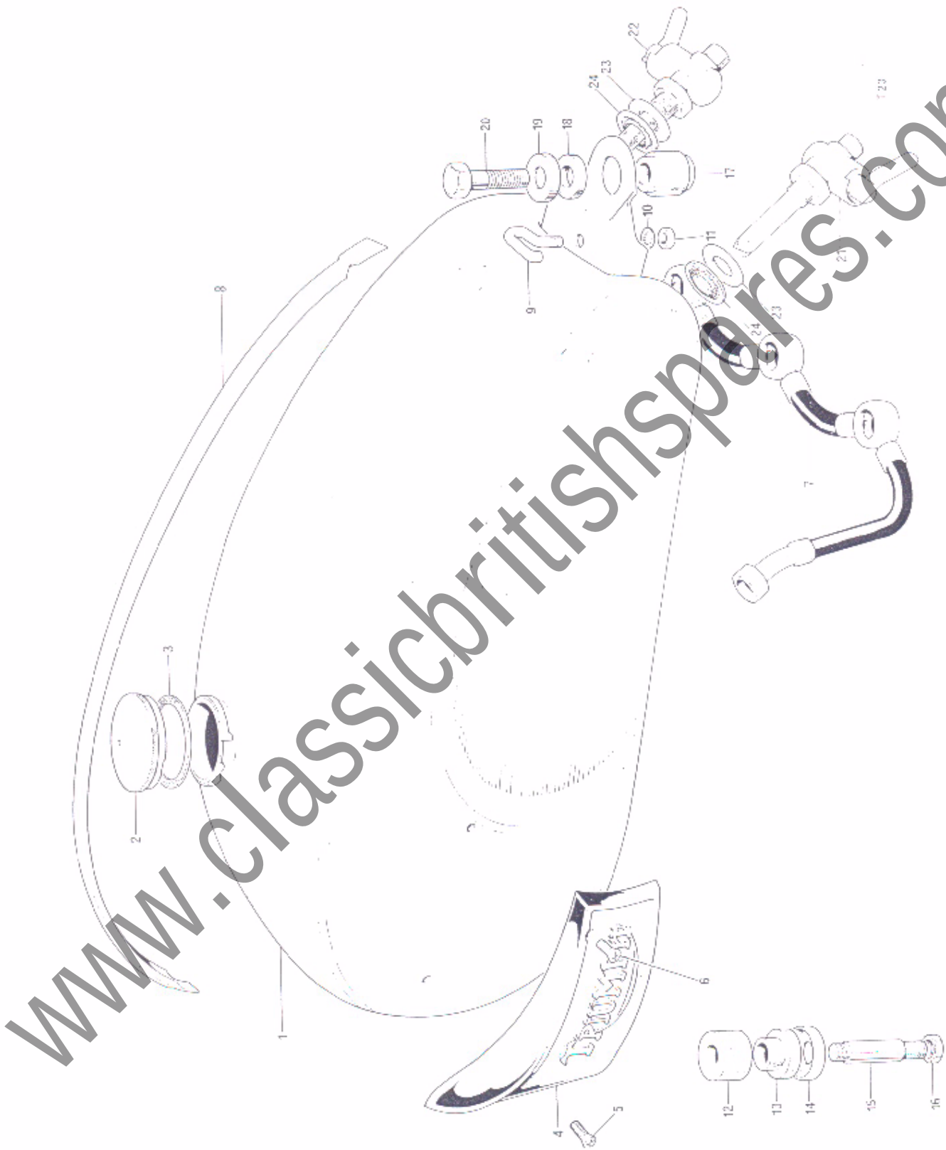
Fig. 25. GAS TANK
