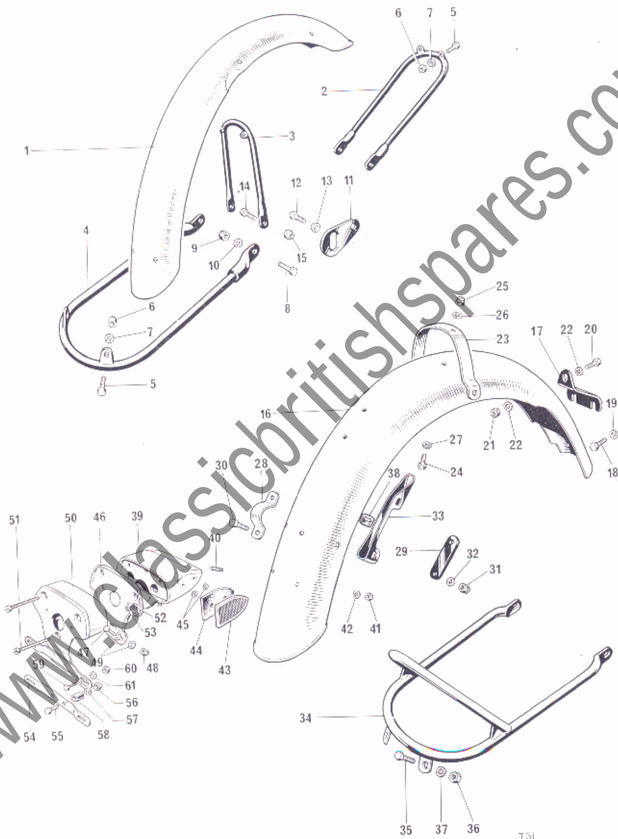
Fig. 27. MUDGUARDS (FENDERS)
