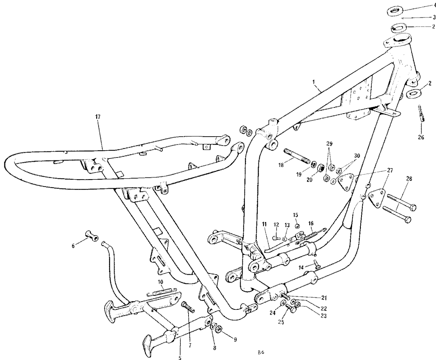
Fig. 12. FRAME
