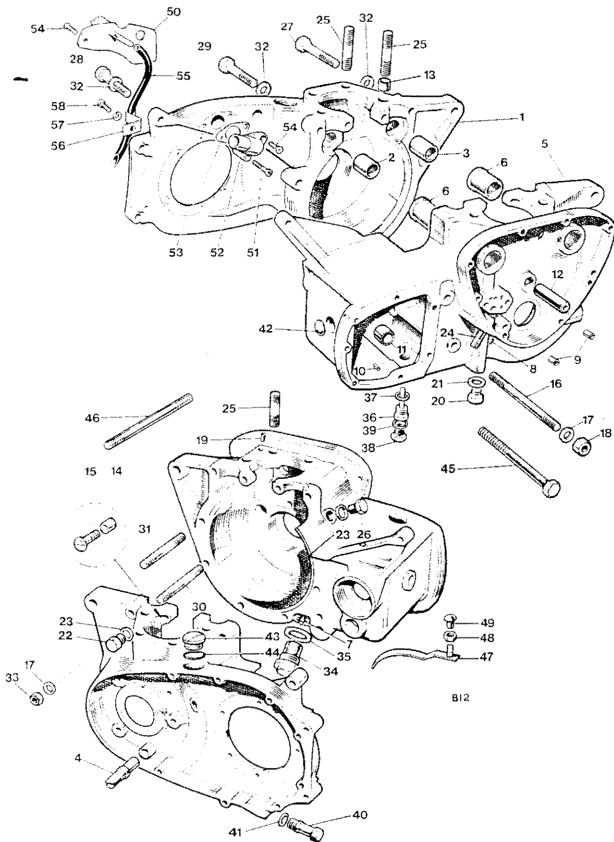
Fig. 2. CRANKCASE
