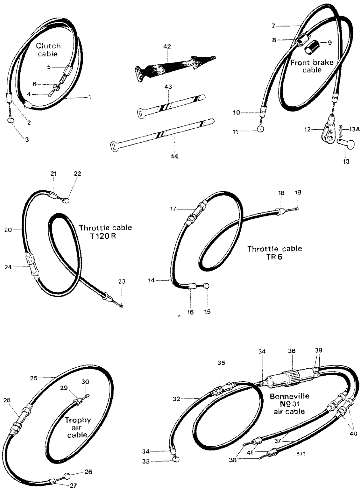
Fig. 27. CONTROL CABLES
