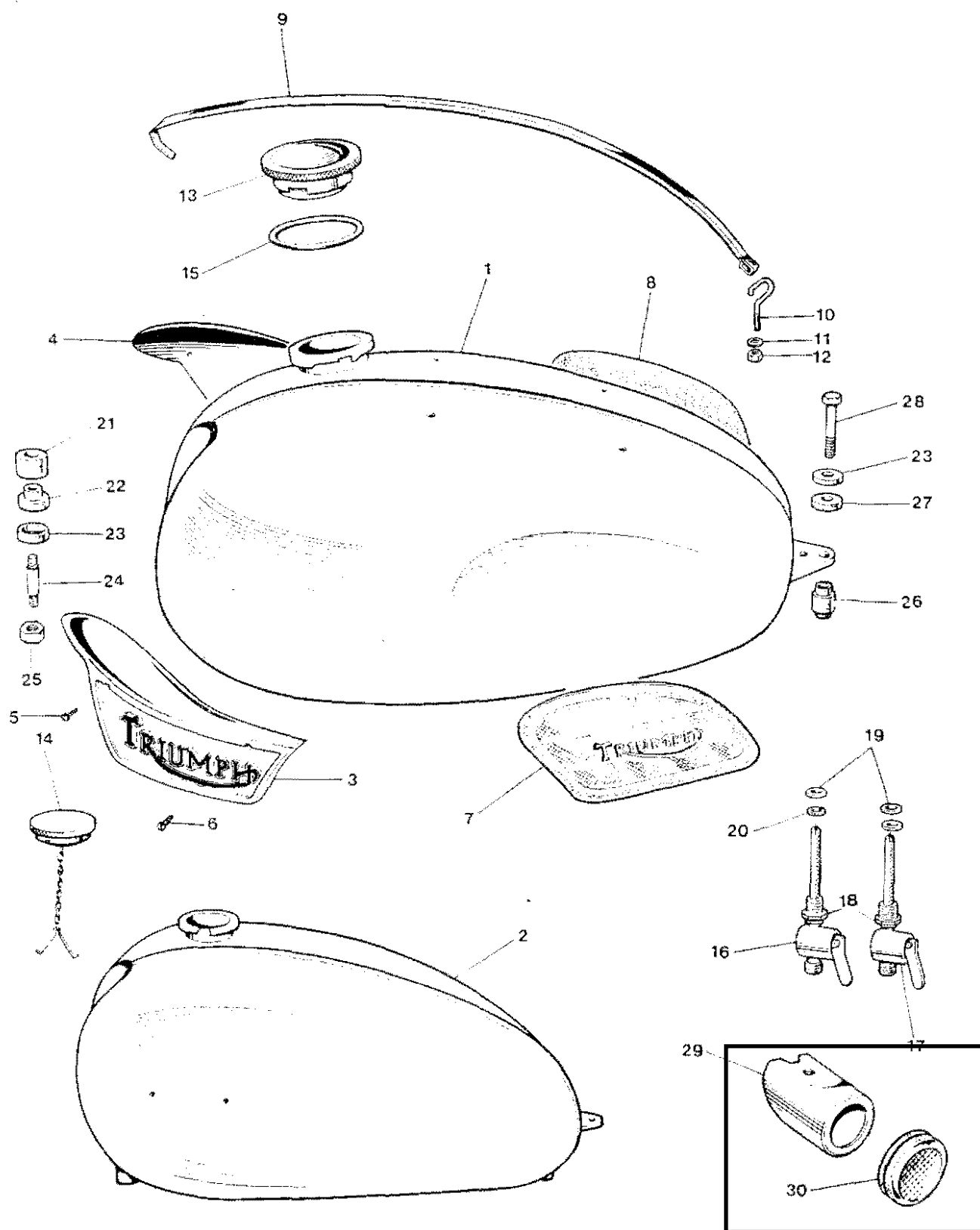
Fig. 21. GAS TANKS
