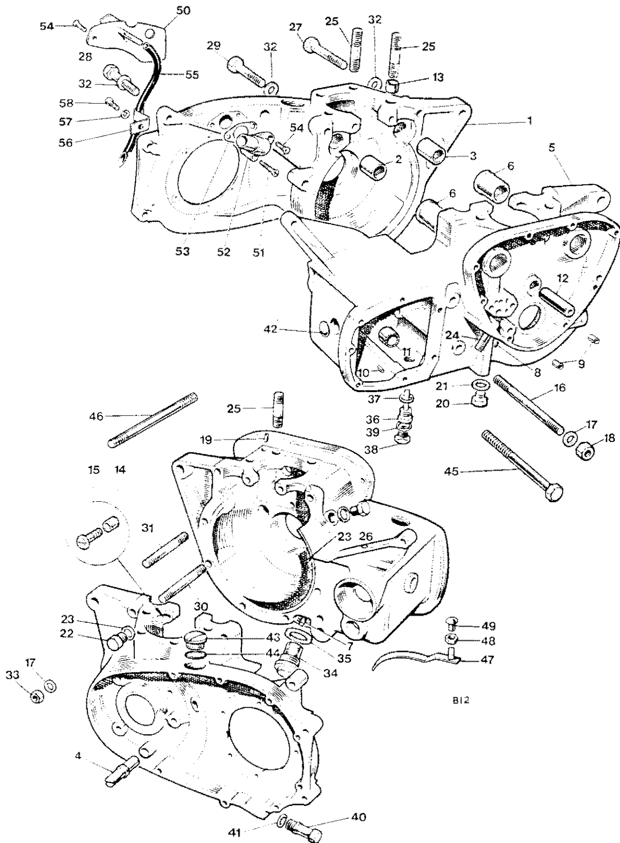
Fig. 2. CRANKCASE
