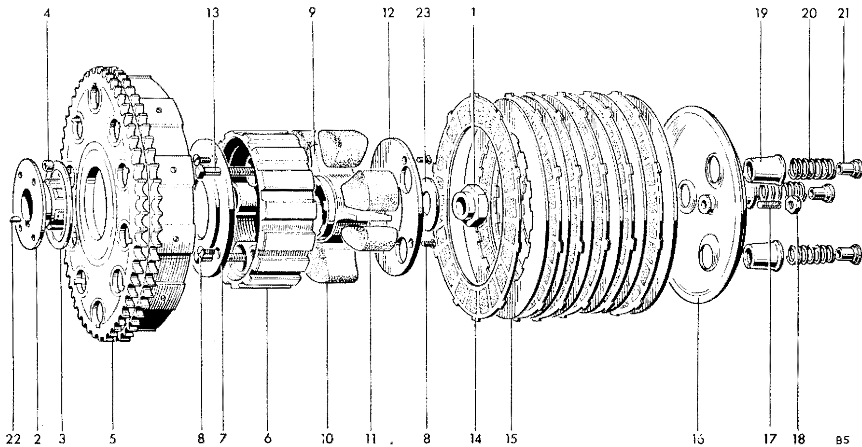
Fig. 10. CLUTCH
