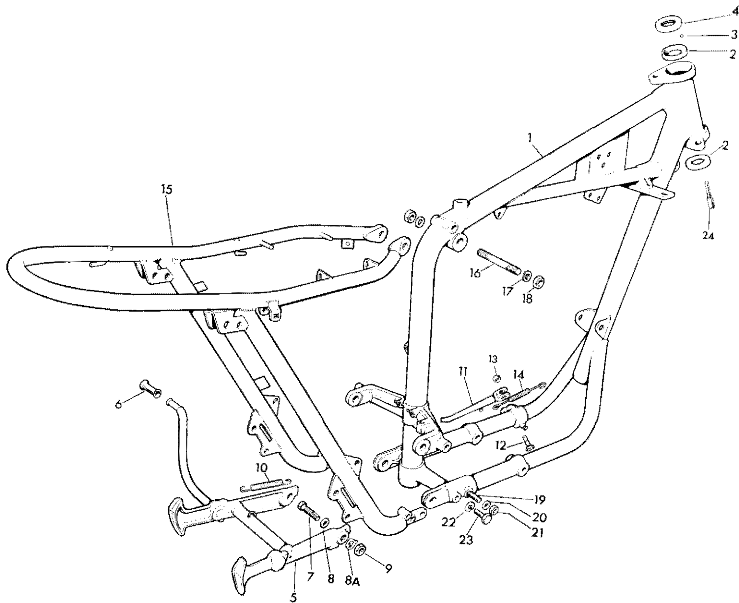
Fig. 12. FRAME
