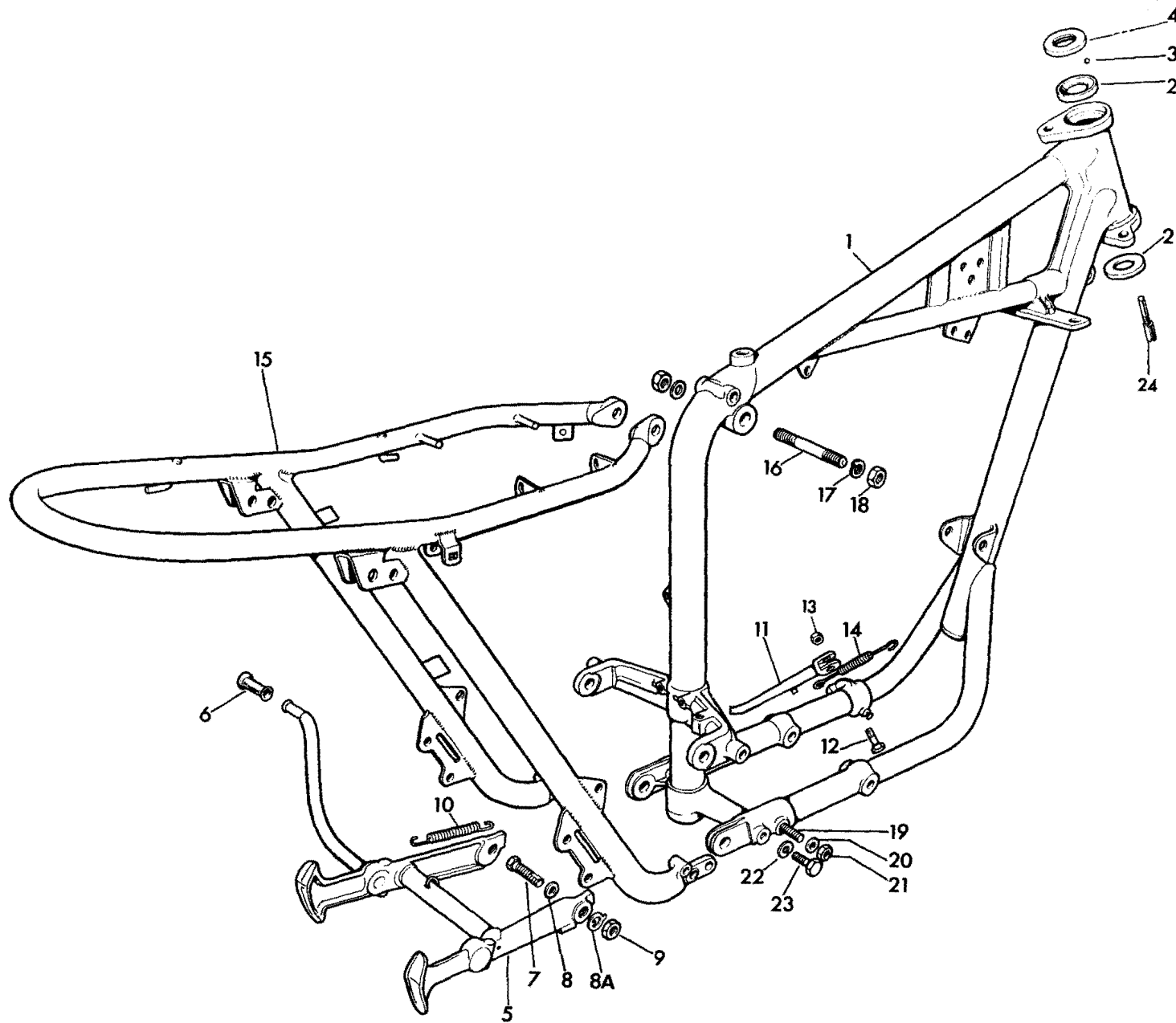
Fig. 12. FRAME
