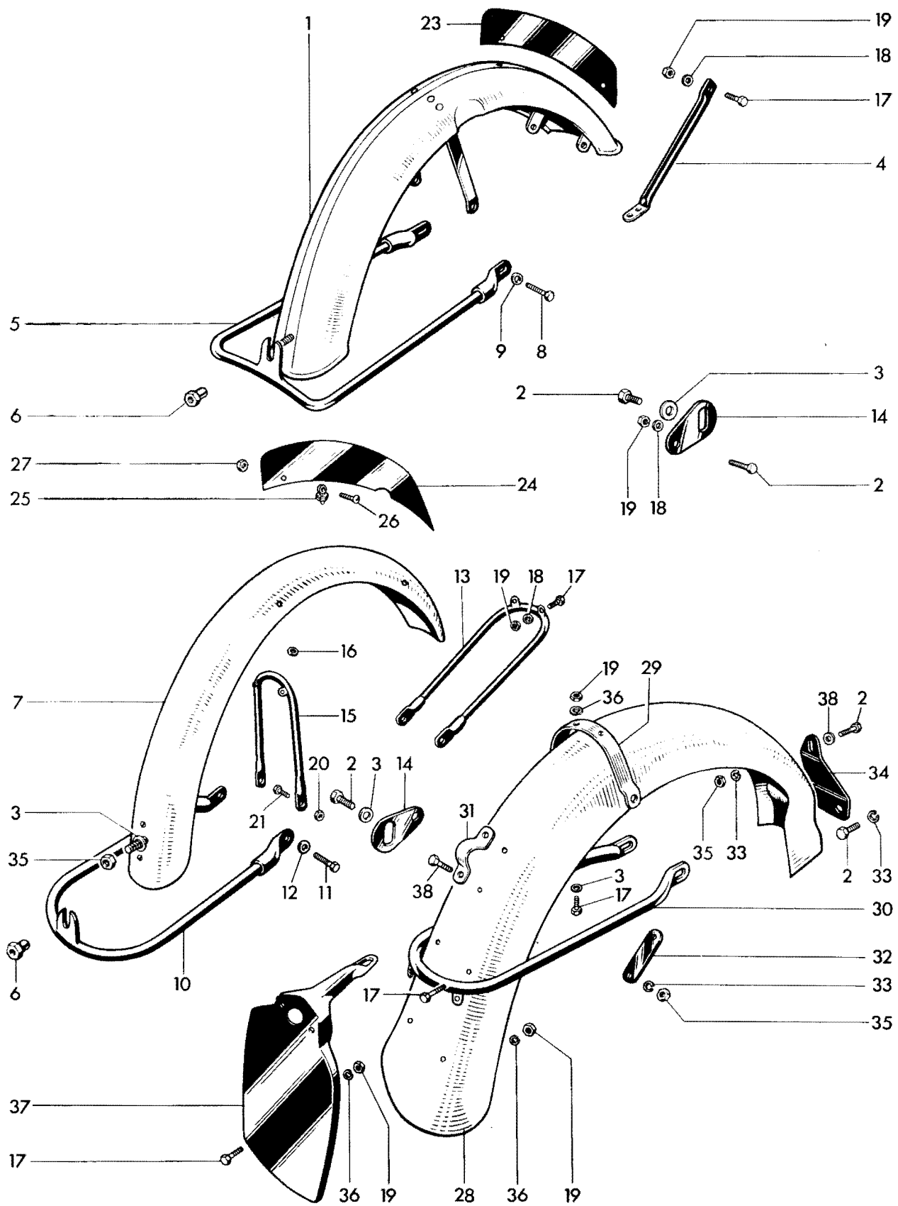
Fig. 29. MUDGUARDS (STANDARD)
