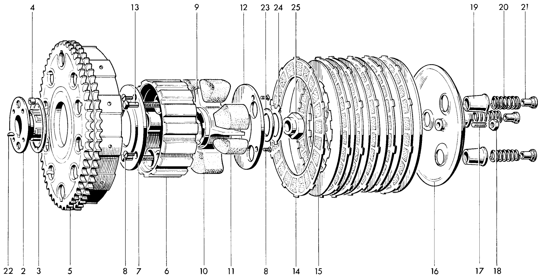
Fig. 10. CLUTCH
