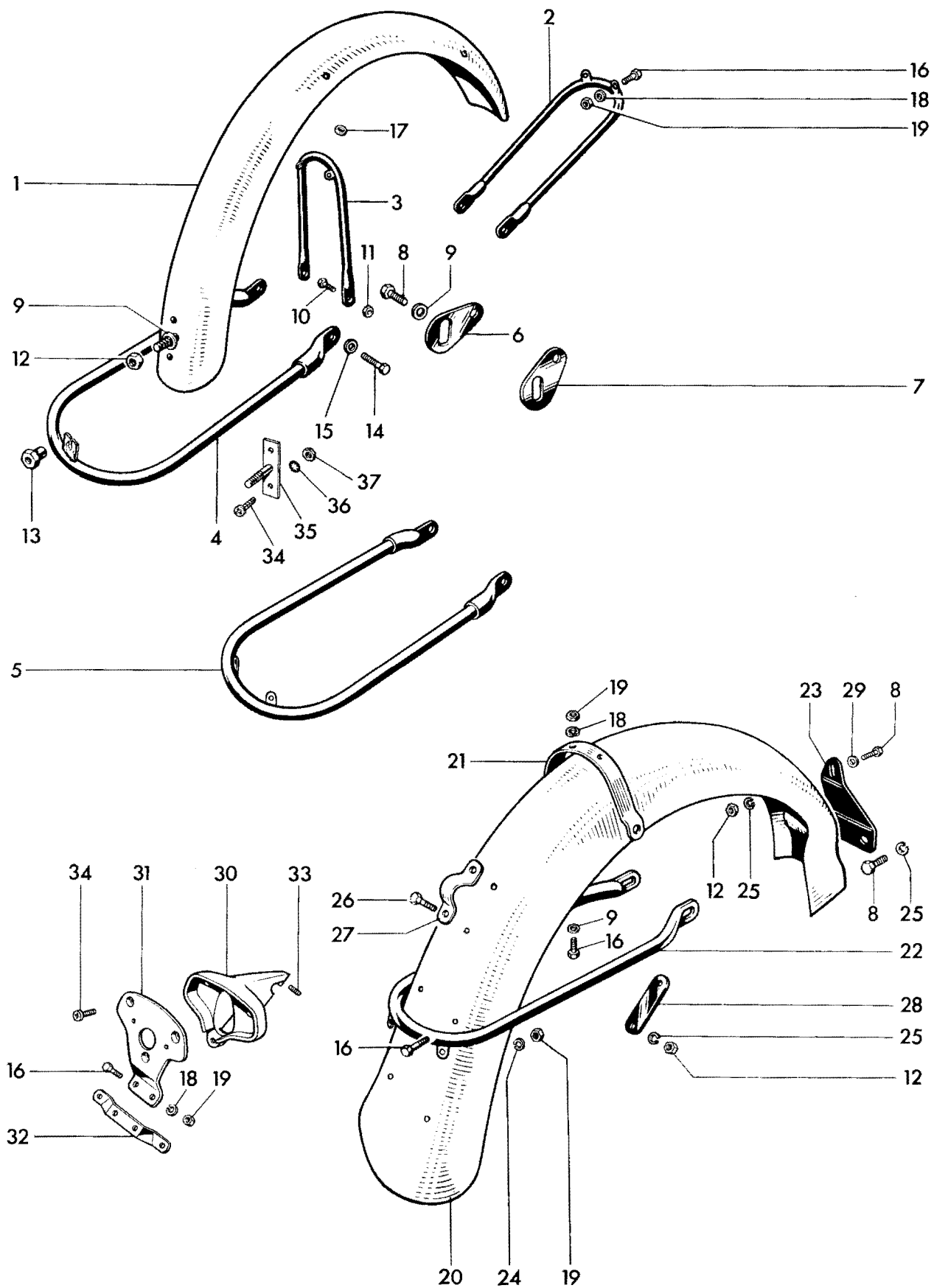
Fig. 30. FENDERS (U.S.A.)
