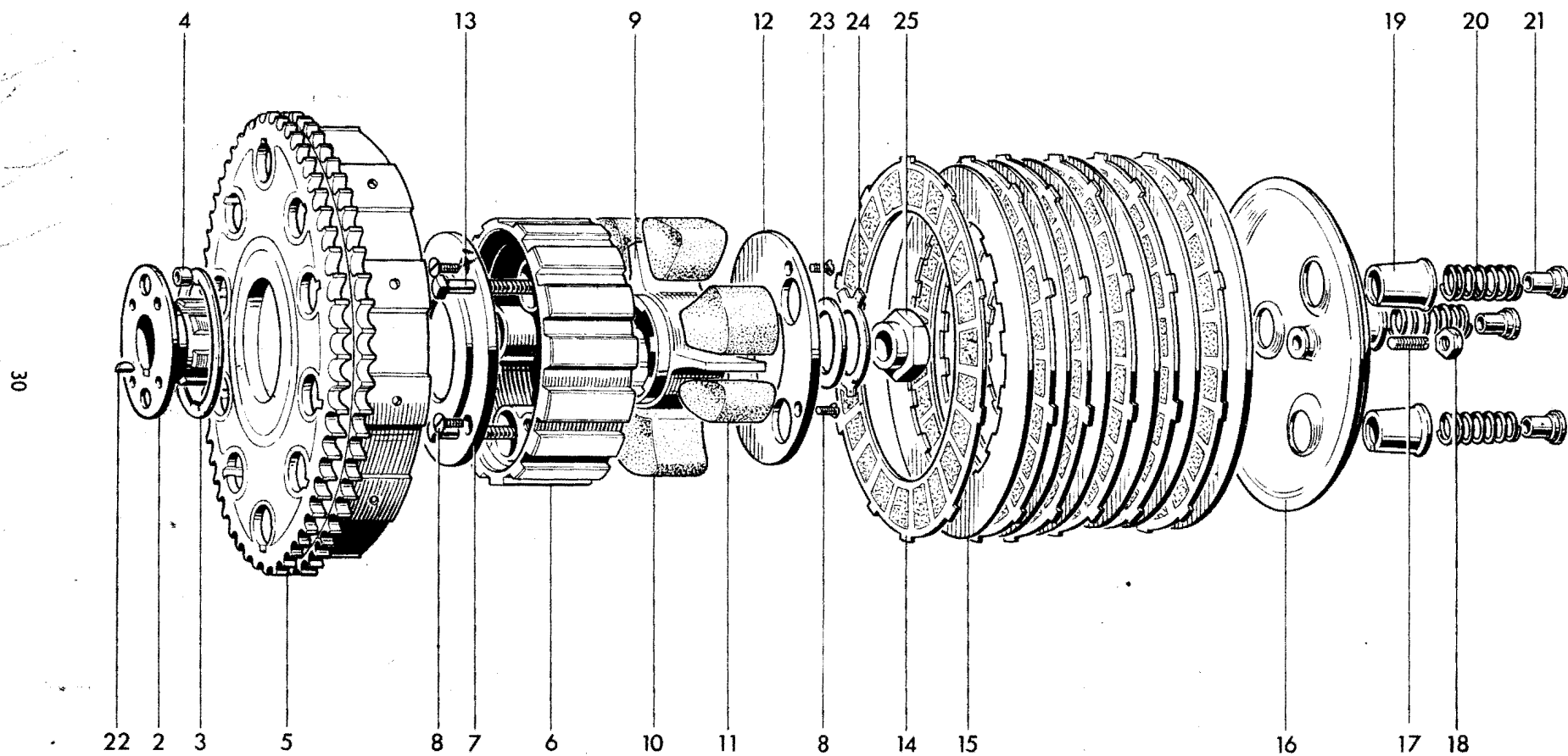
Fig. 10. CLUTCH
