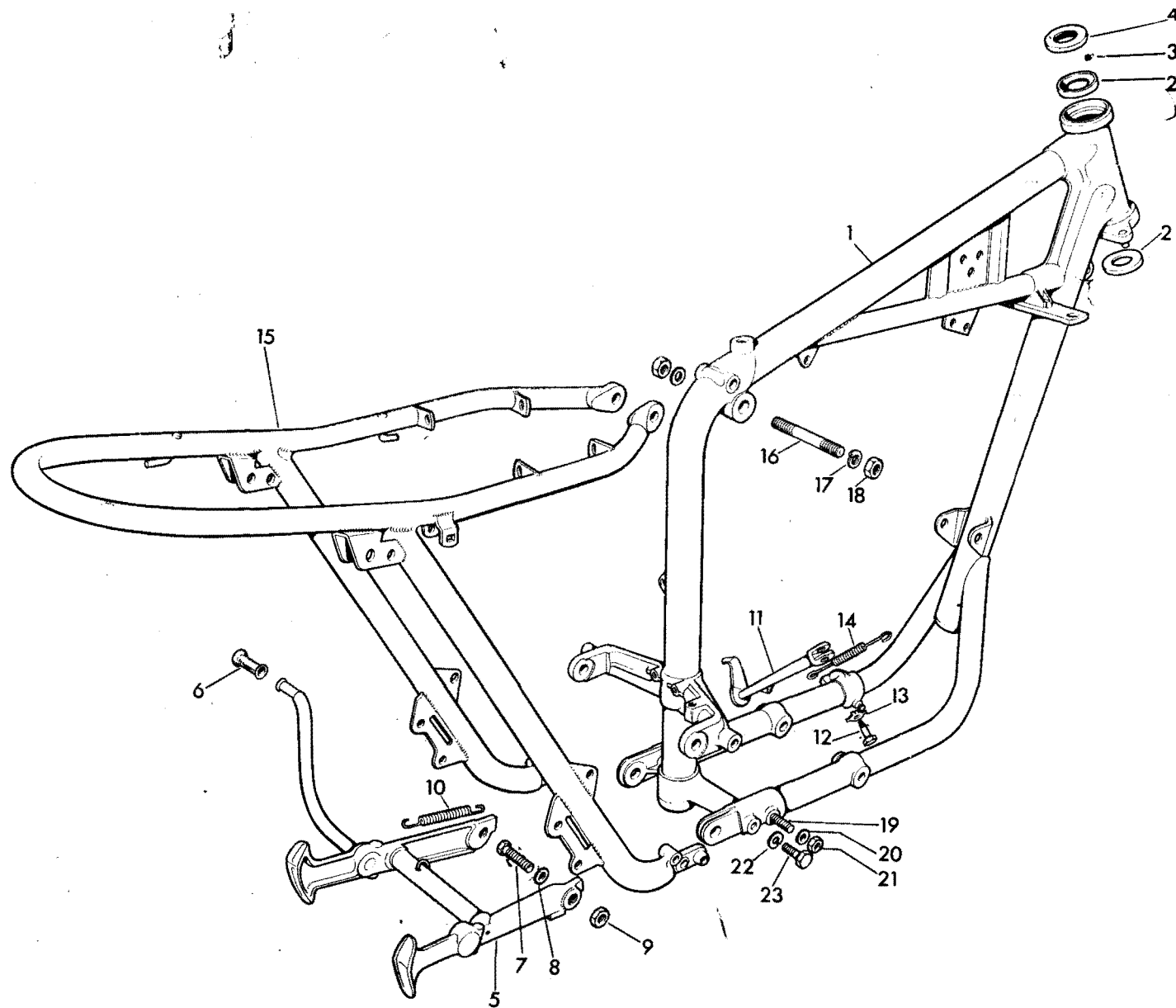
Fig. 12. FRAME
