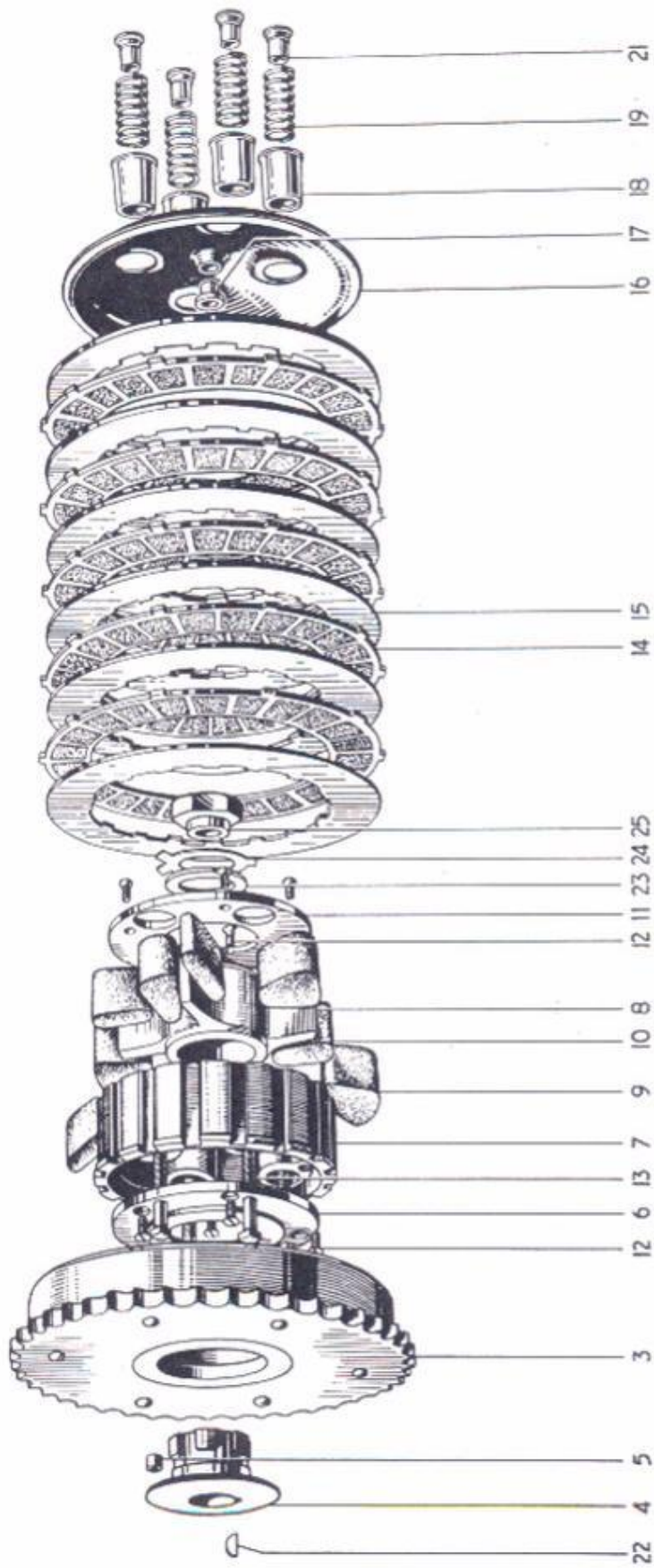
FIG. 10 CLUTCH
