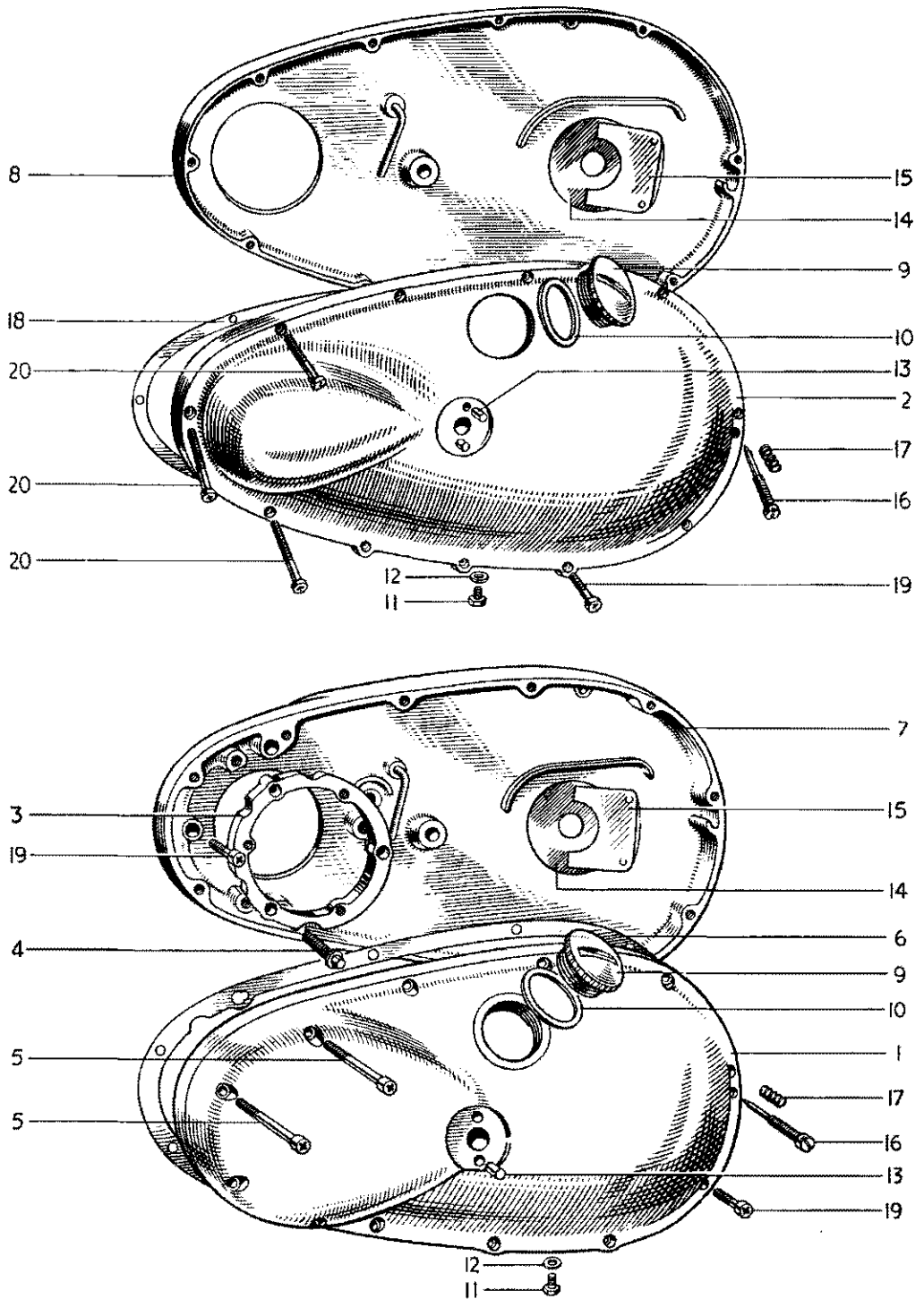
FIG. 24. PRIMARY CHAINCASE
