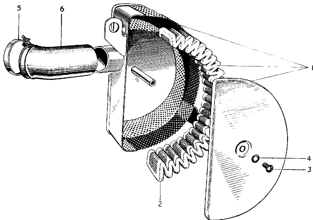
FIG. 28. AIR FILTER
