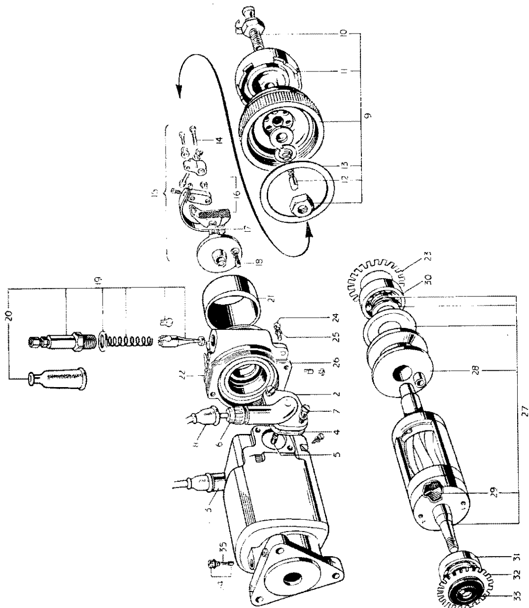
FIG. 31. LUCAS MAGNETO
