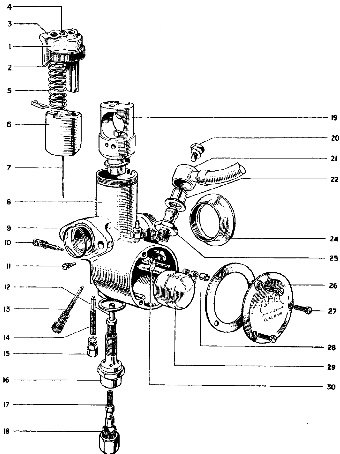
FIG. 29. AMAL CARBURETTER
