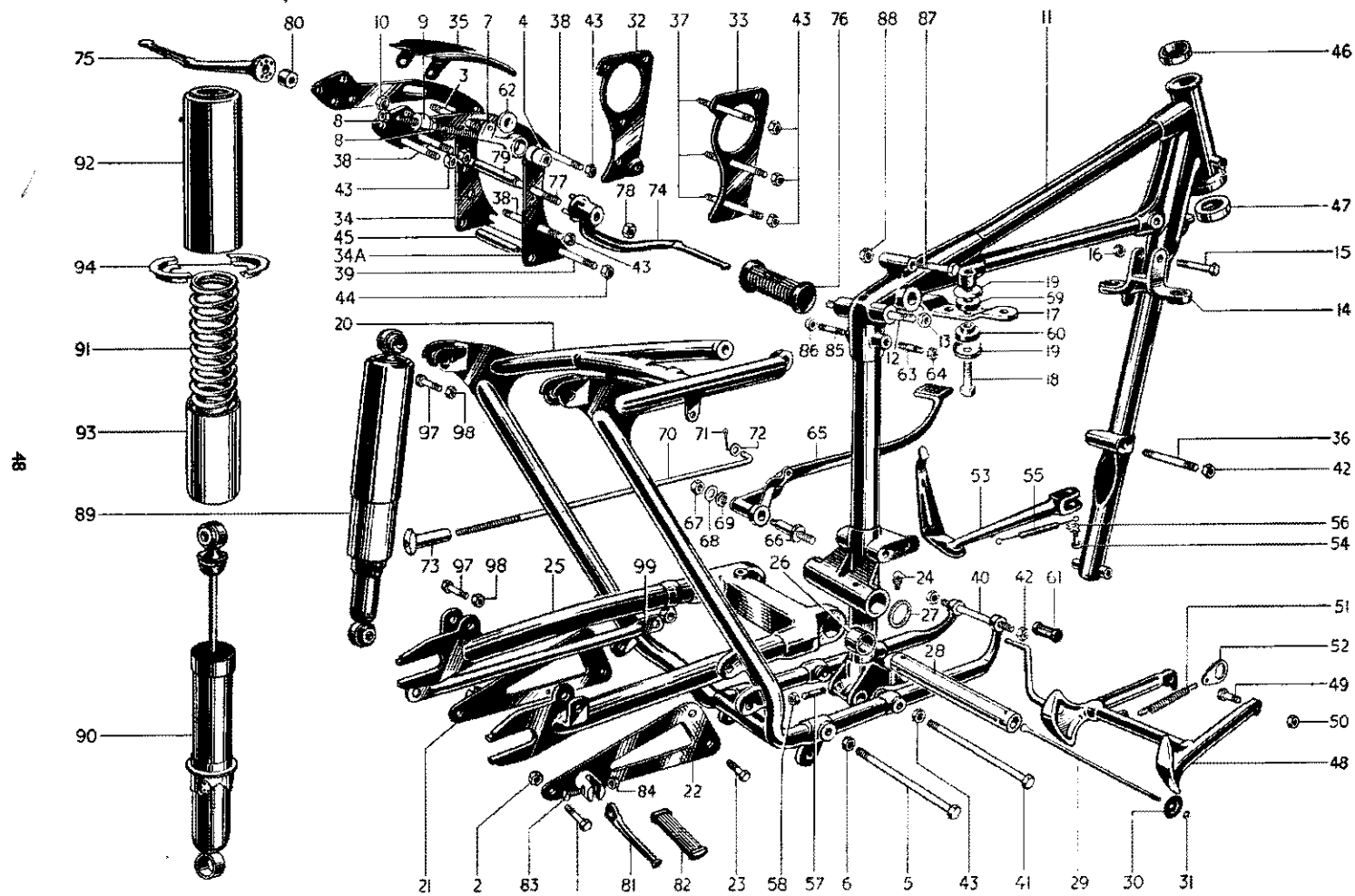
FIG. 13. FRAME
