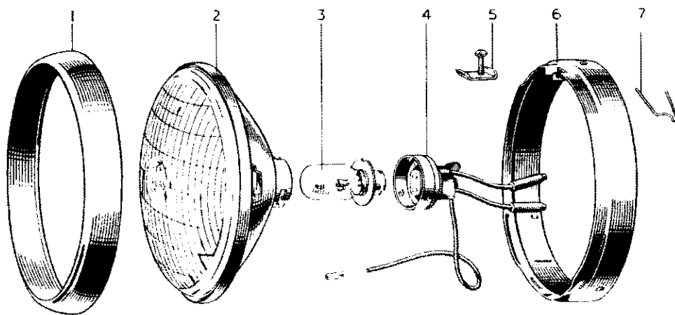
FIG. 30. HEAD LAMP
