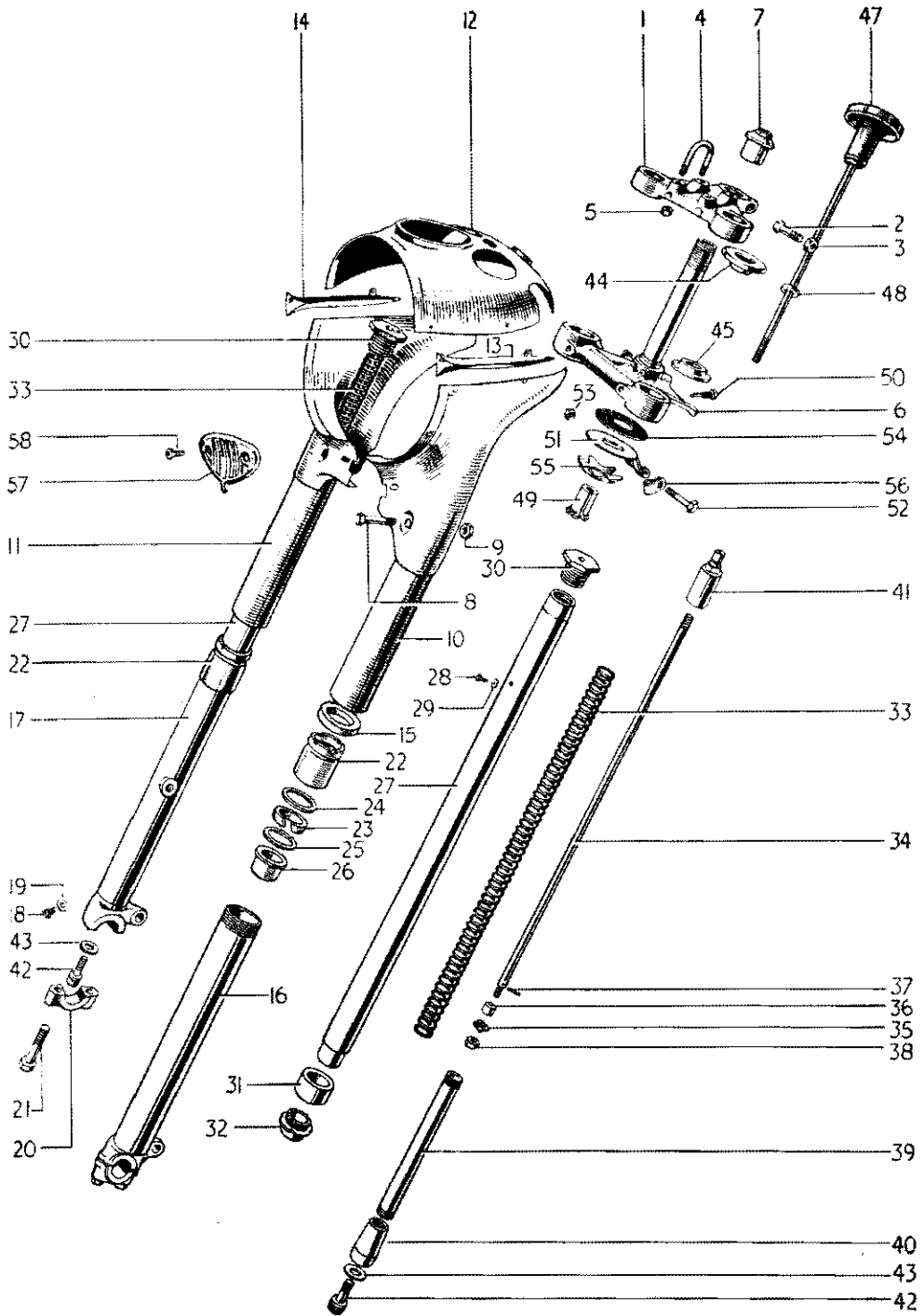
FIG. 15. TELESCOPIC FORK
