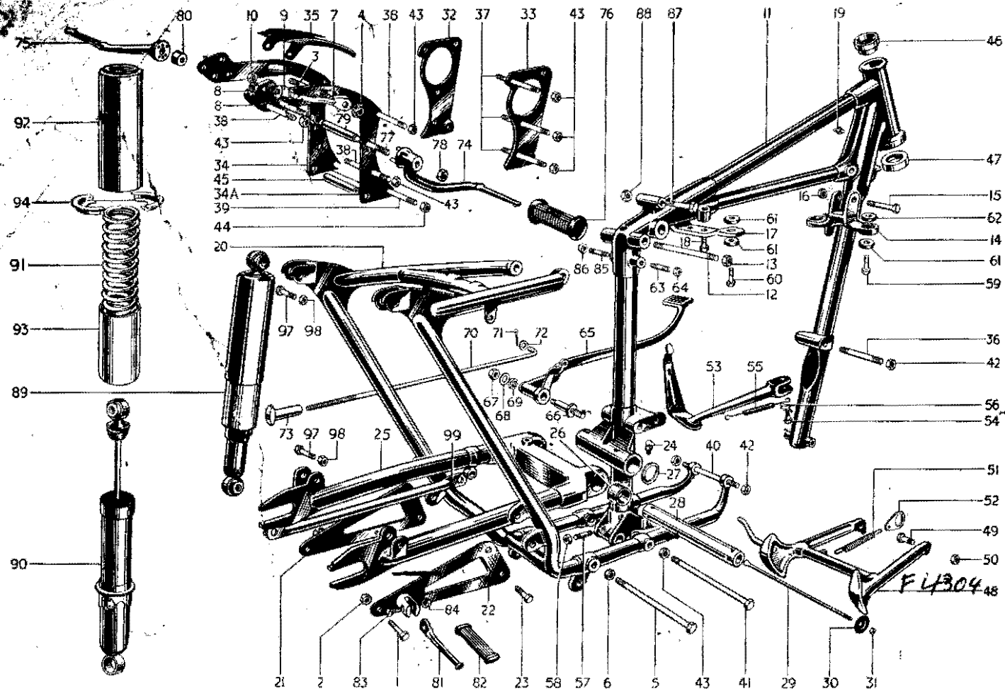
FIG. 13. FRAME
