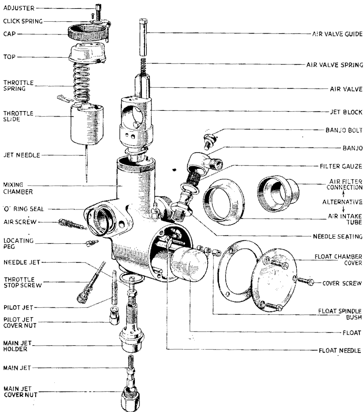
FIG. 29. AMAL CARBURETTER
