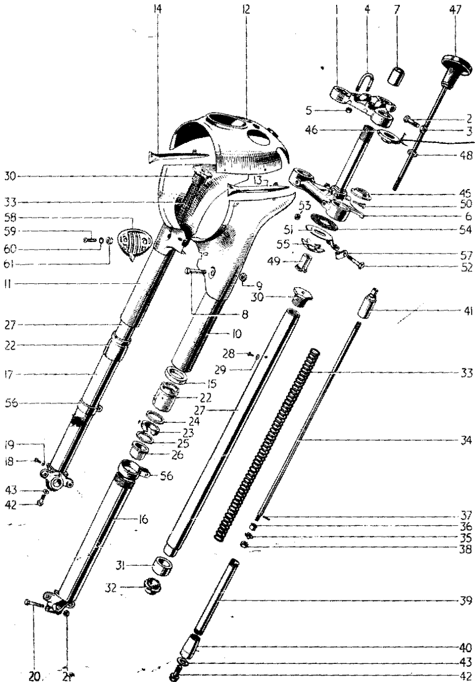
FIG. 15. TELESCOPIC FORK
