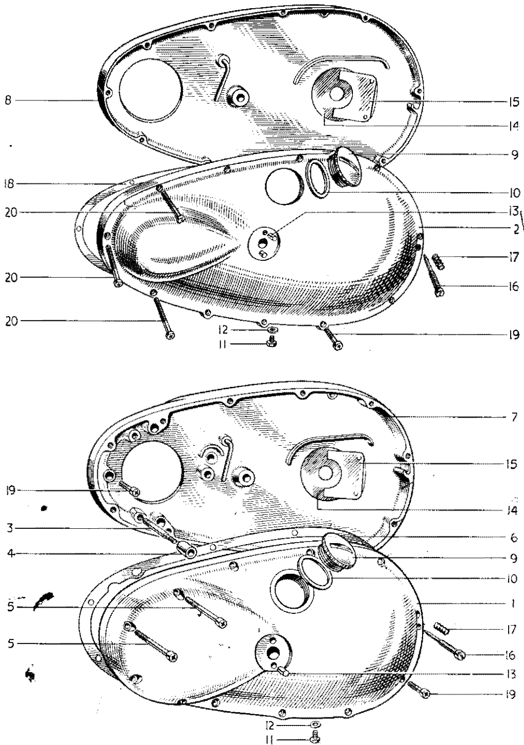
FIG. 24. PRIMARY CHAINCASE
