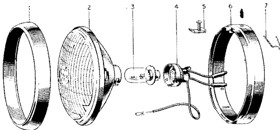
FIG. 31. HEAD LAMP
