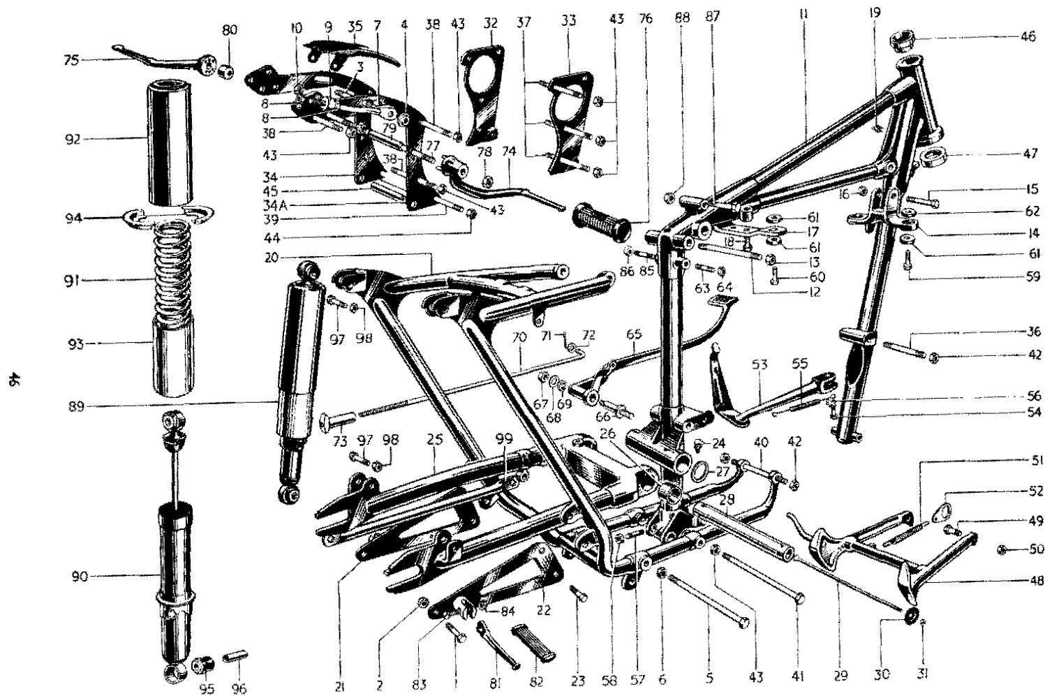
FIG. 13. FRAME
