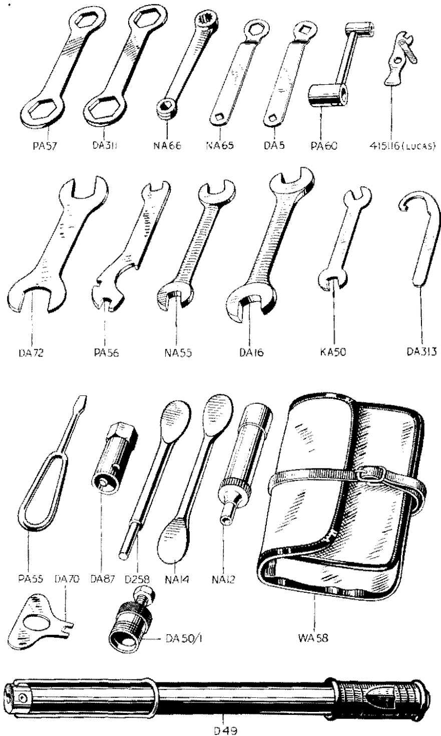
FIG. 28. TOOL KIT
