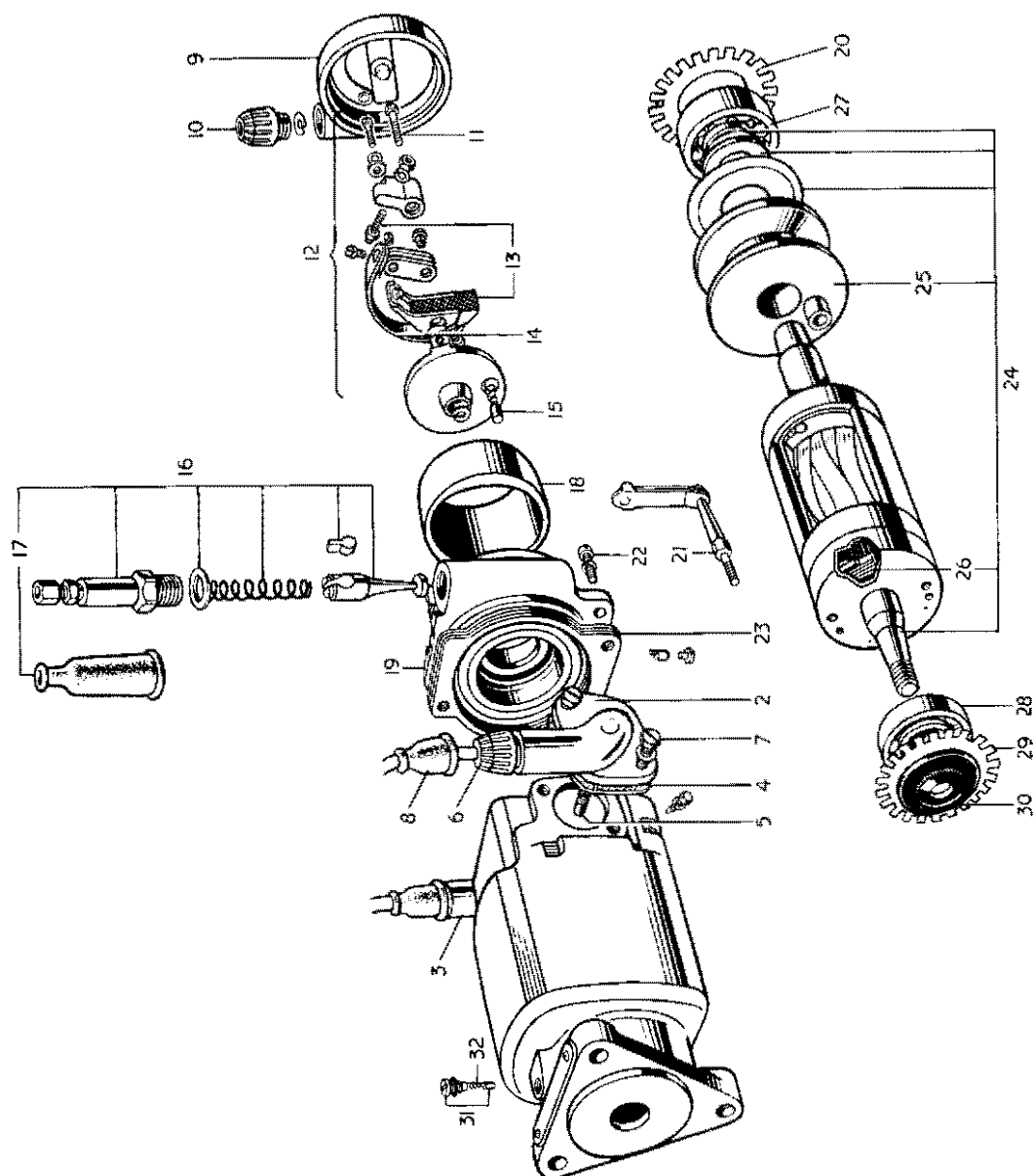
FIG. 33. LUCAS MAGNETO
