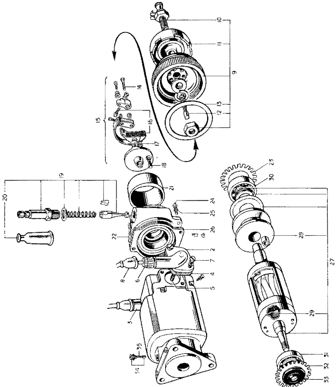
FIG. 34. LUCAS MAGNETO
