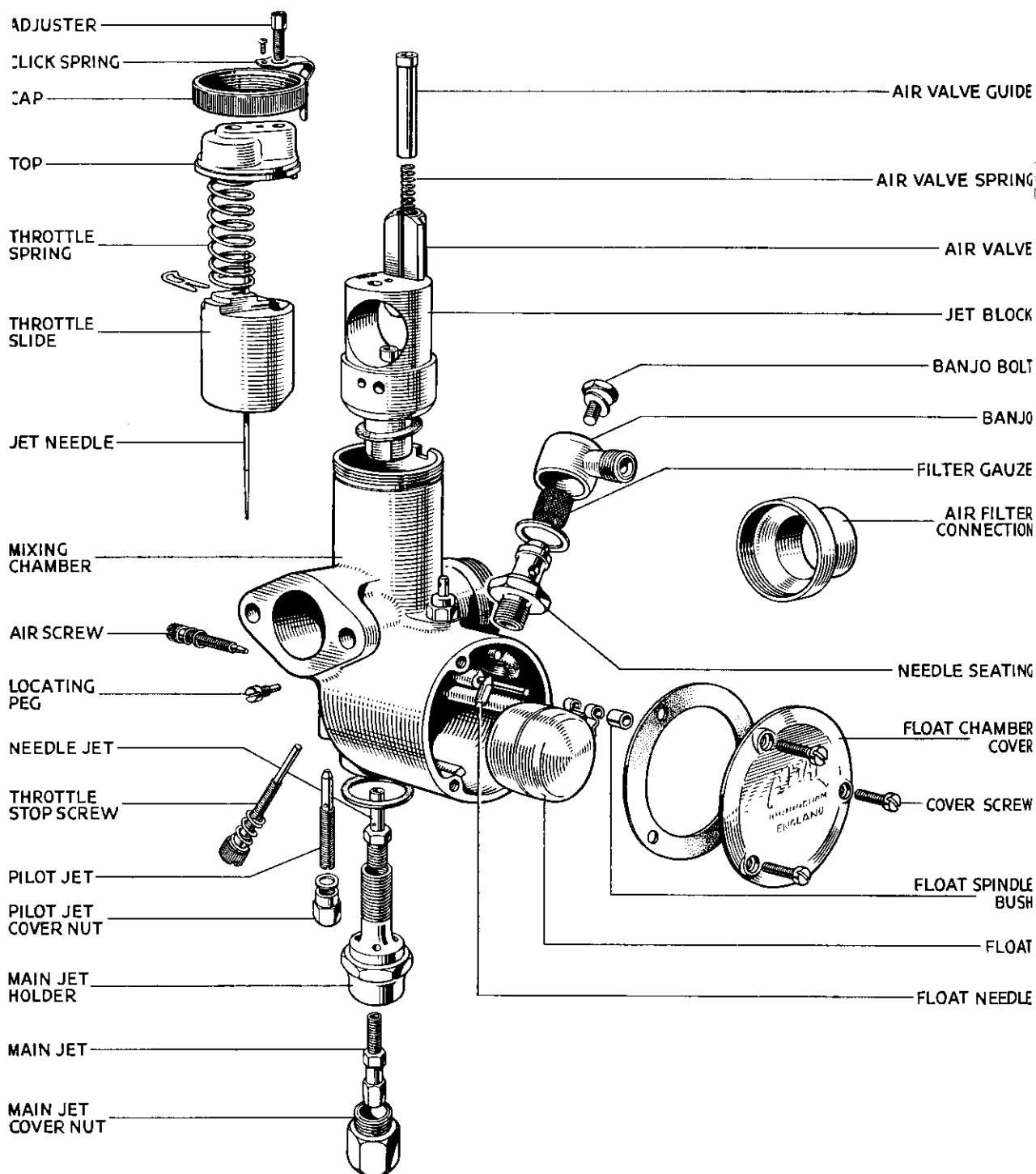
FIG. 30. AMAL CARBURETTER
