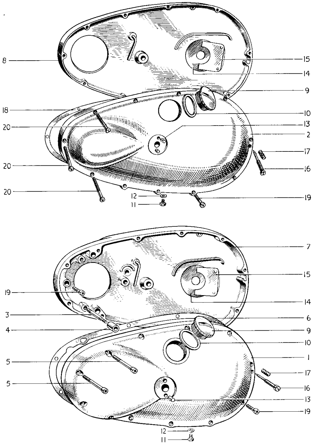
FIG. 25. PRIMARY CHAINCASE
