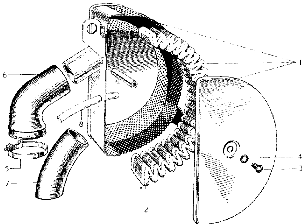
FIG. 29. AIR FILTER
