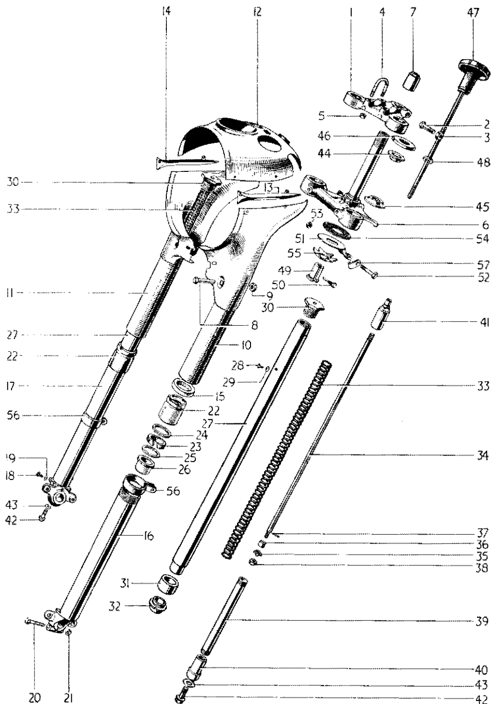
FIG. 16. TELESCOPIC FORK
