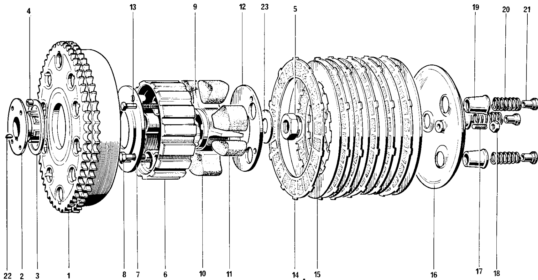
Fig. 10. CLUTCH
