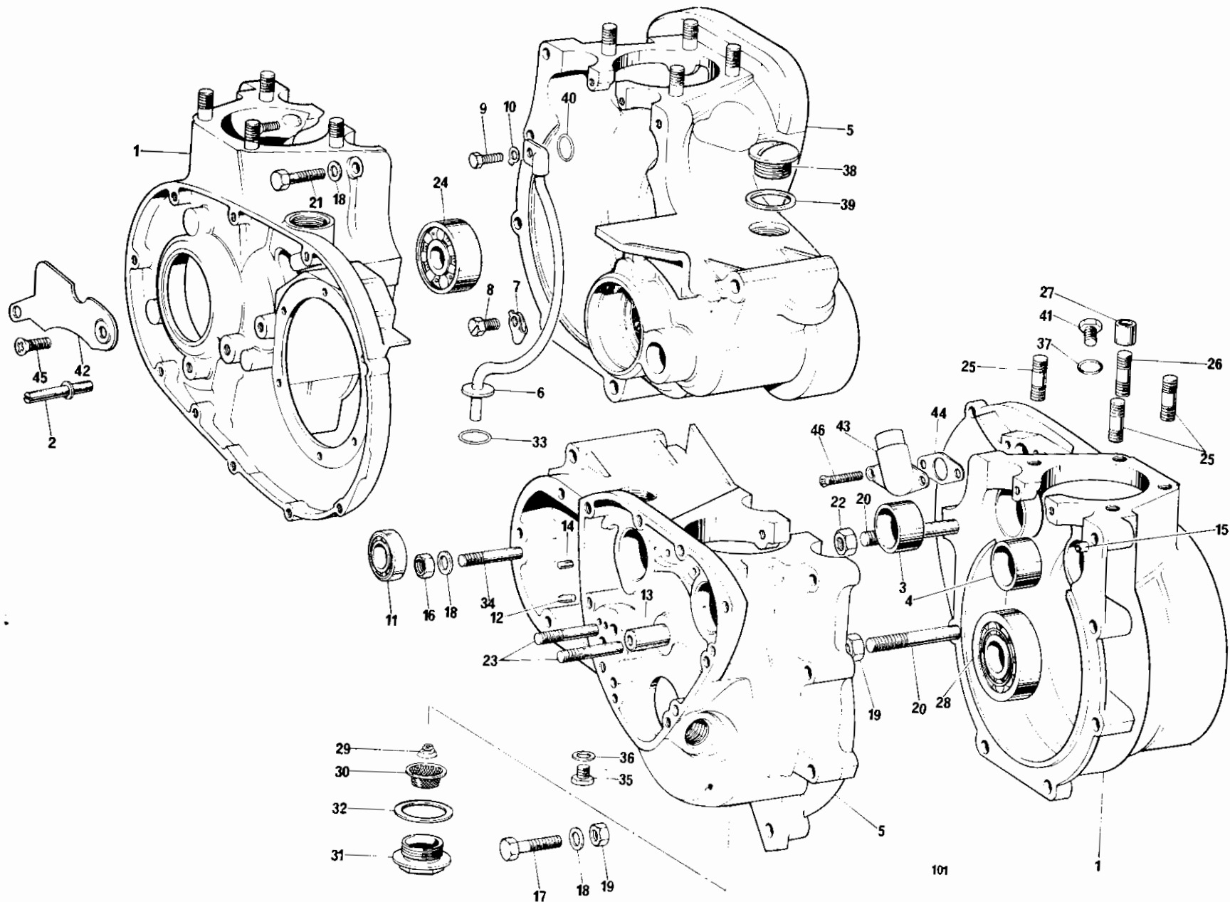
Fig. 2. CRANKCASE
