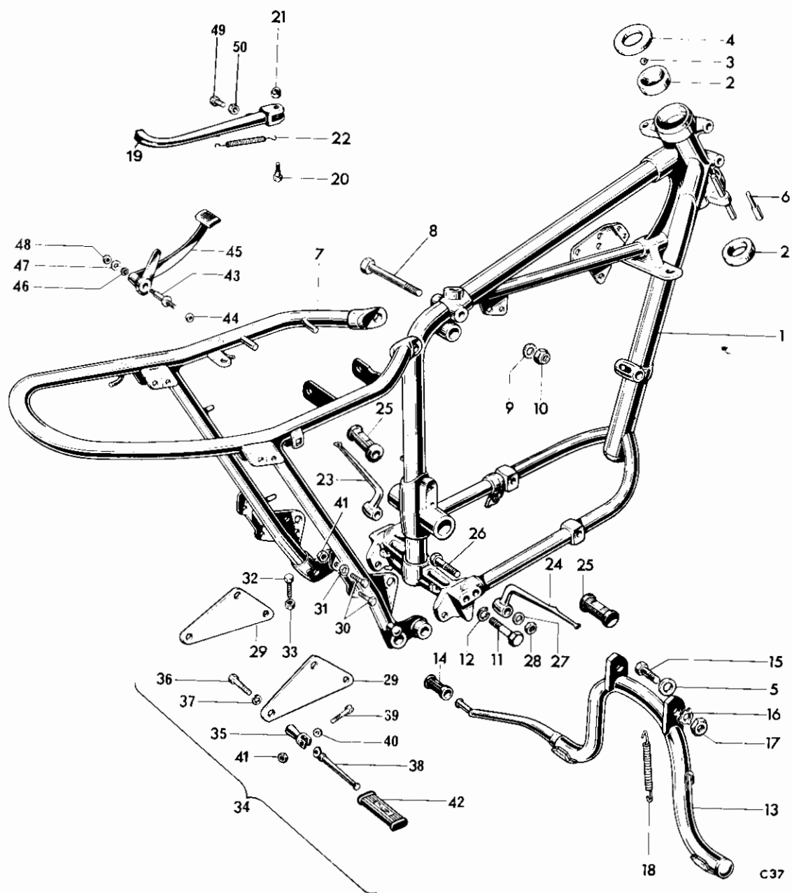
Fig. 14. FRAME
