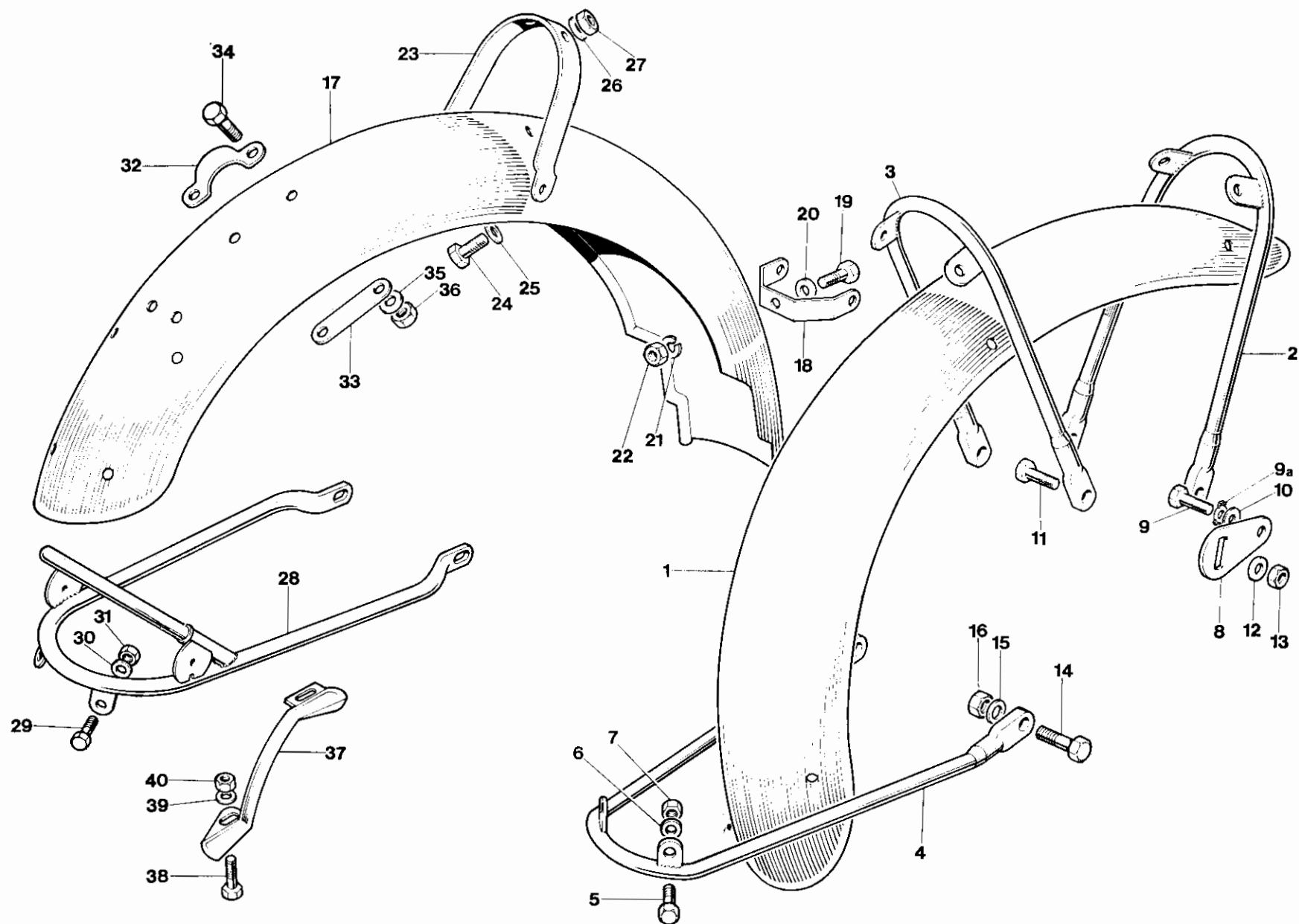
Fig. 19. FENDERS
