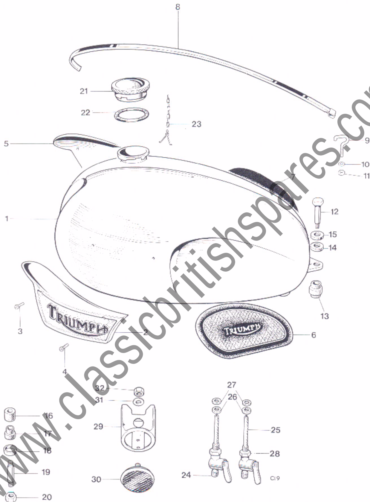
Fig. 27. GAS TANK
