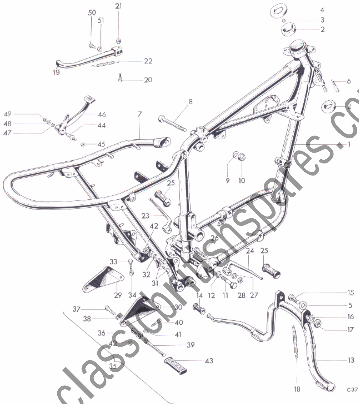
Fig. 18. FRAME
