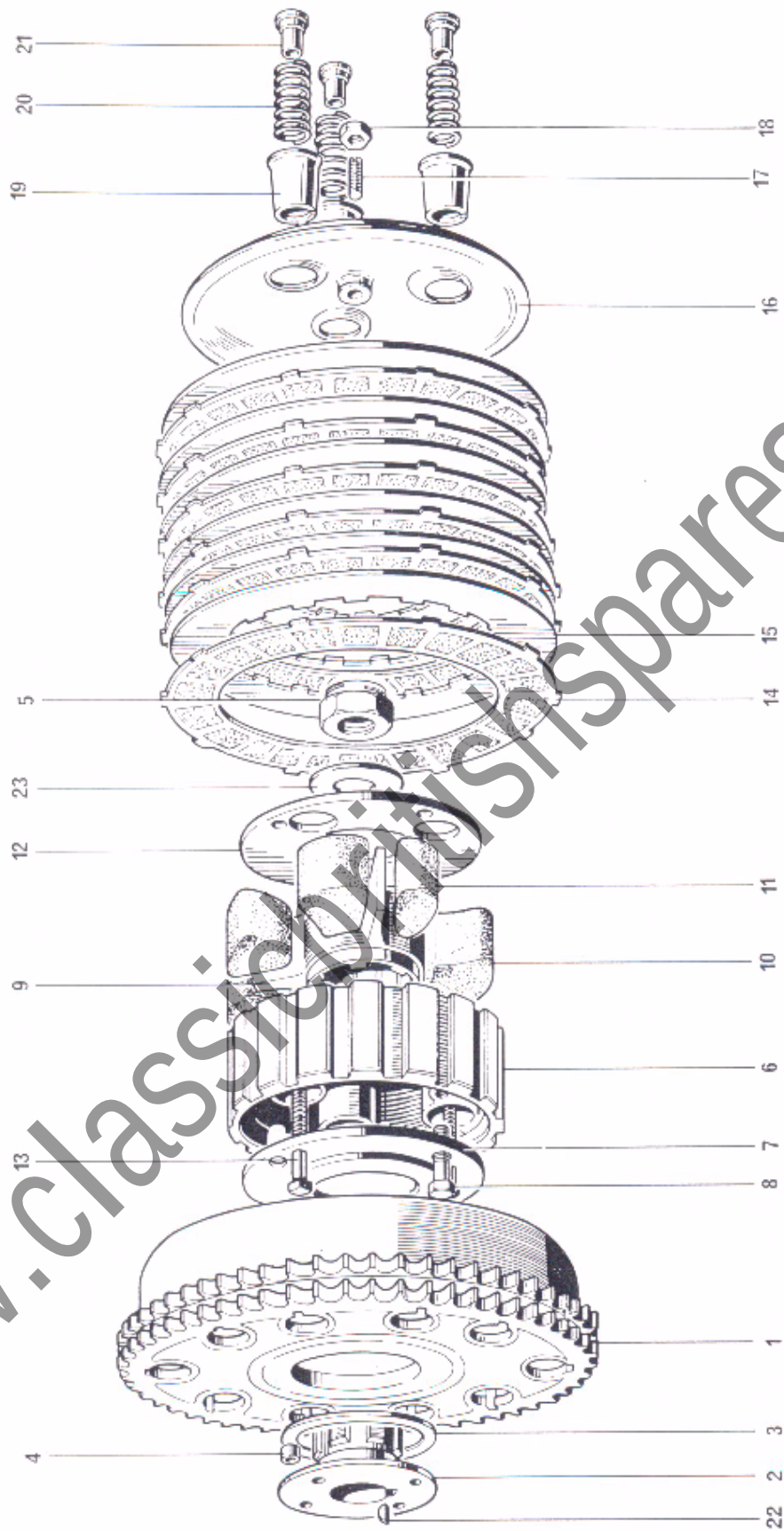
Fig. 13. CLUTCH
