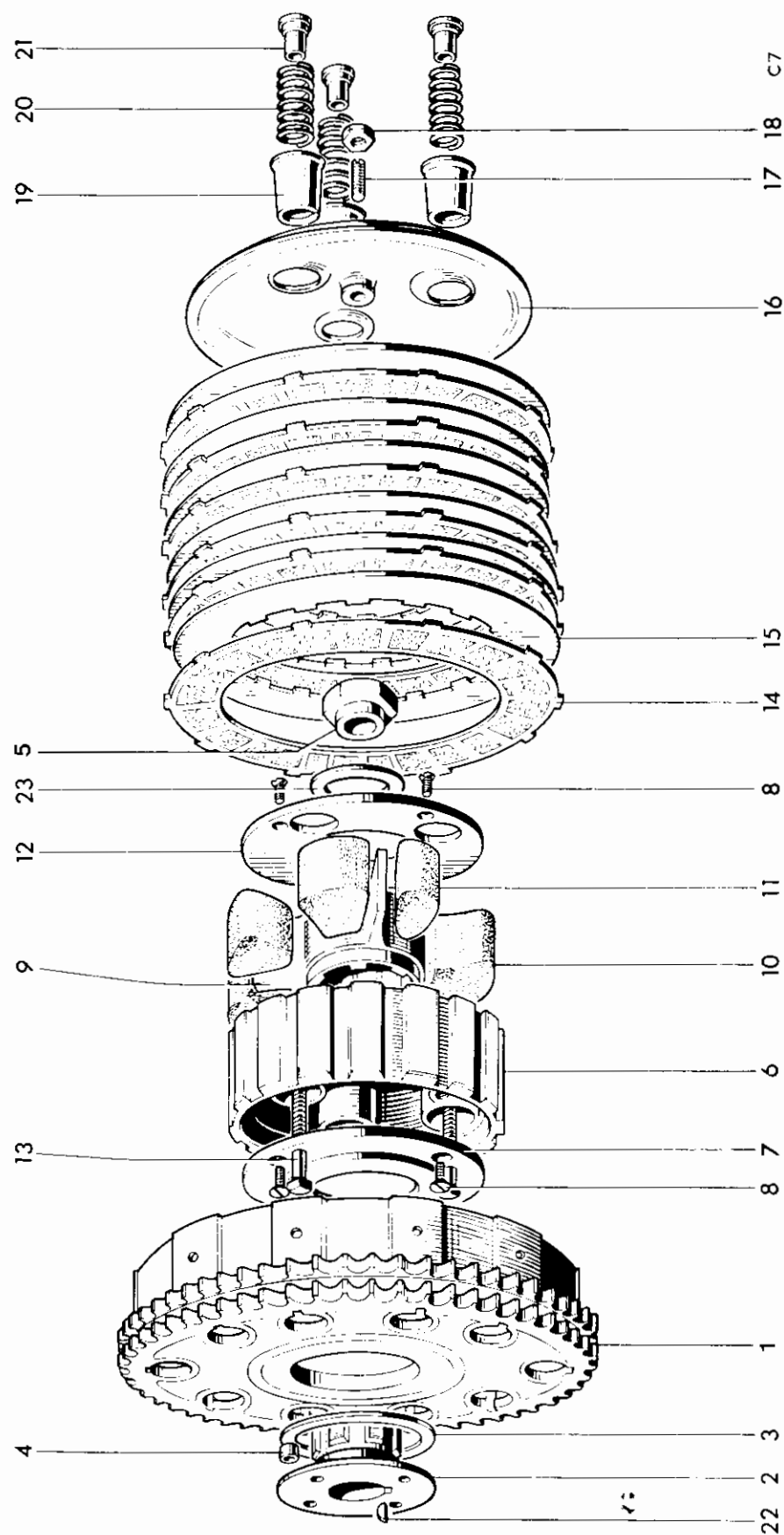
Fig. 13. CLUTCH
