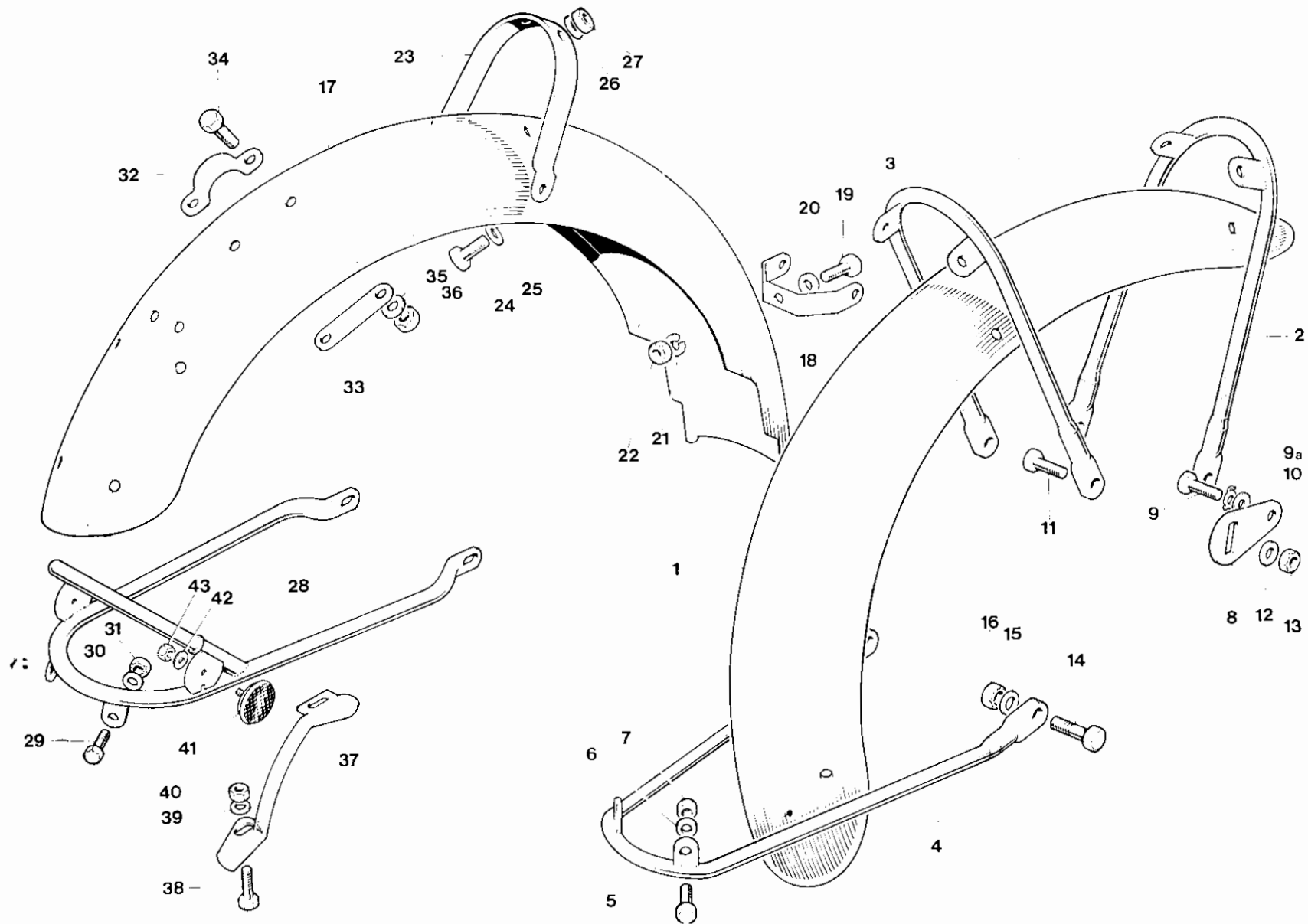
Fig. 24. FENDERS
