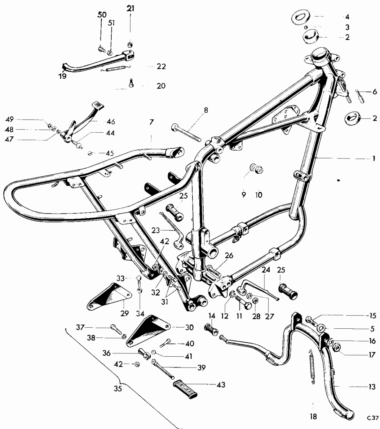
Fig. 18. FRAME
