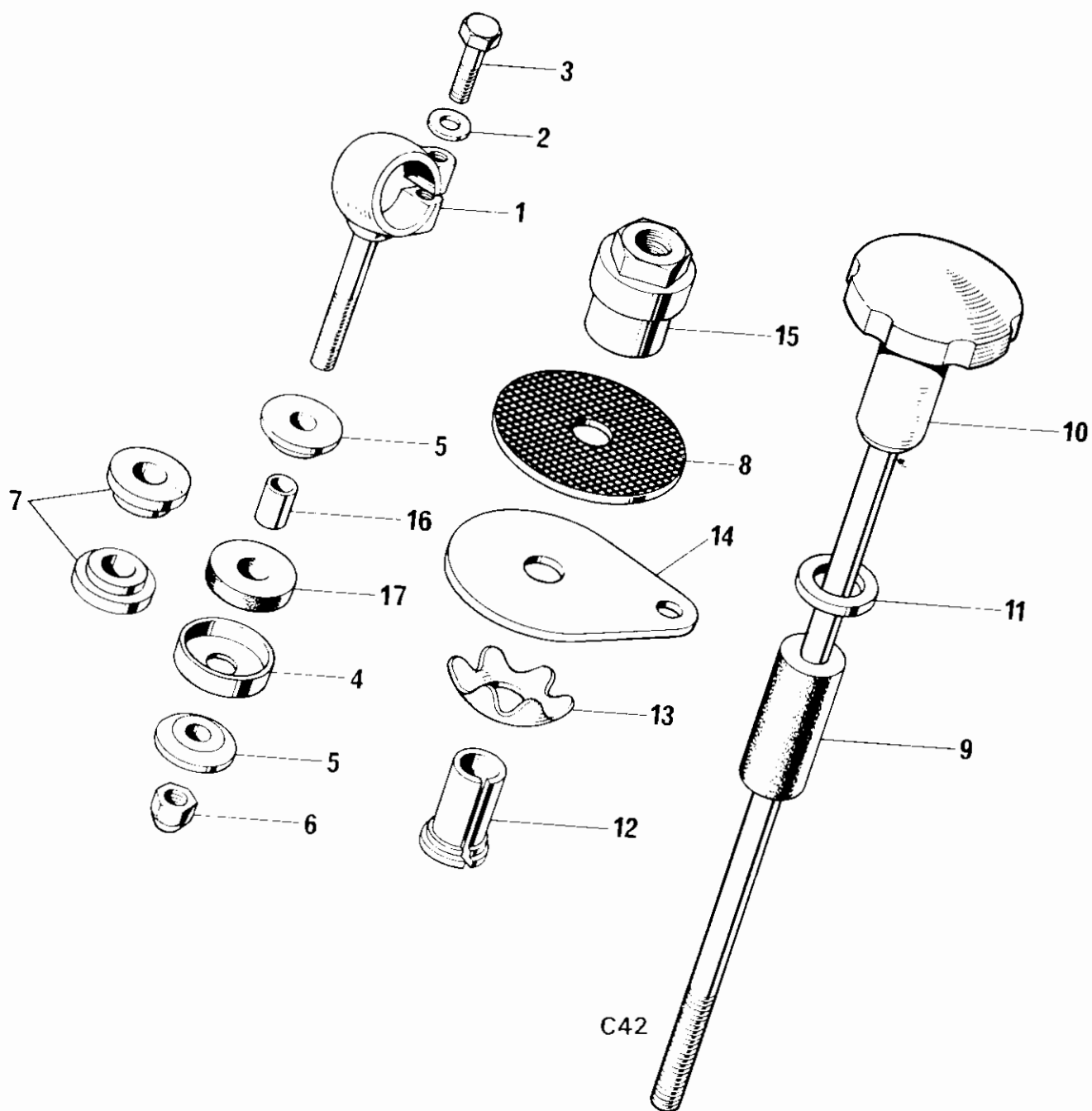
Fig. 30. STEERING DAMPER
