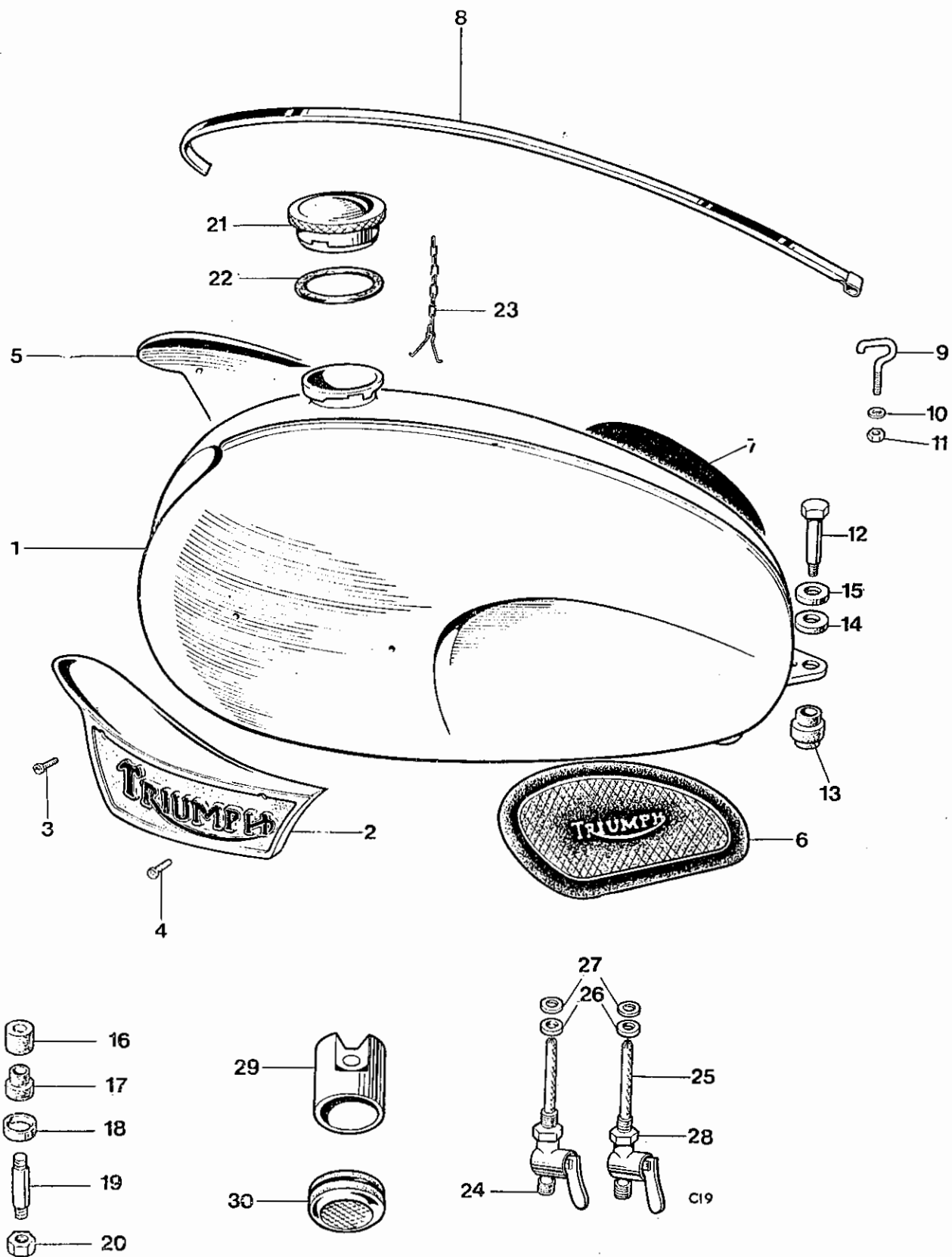
Fig. 25. GAS TANK
