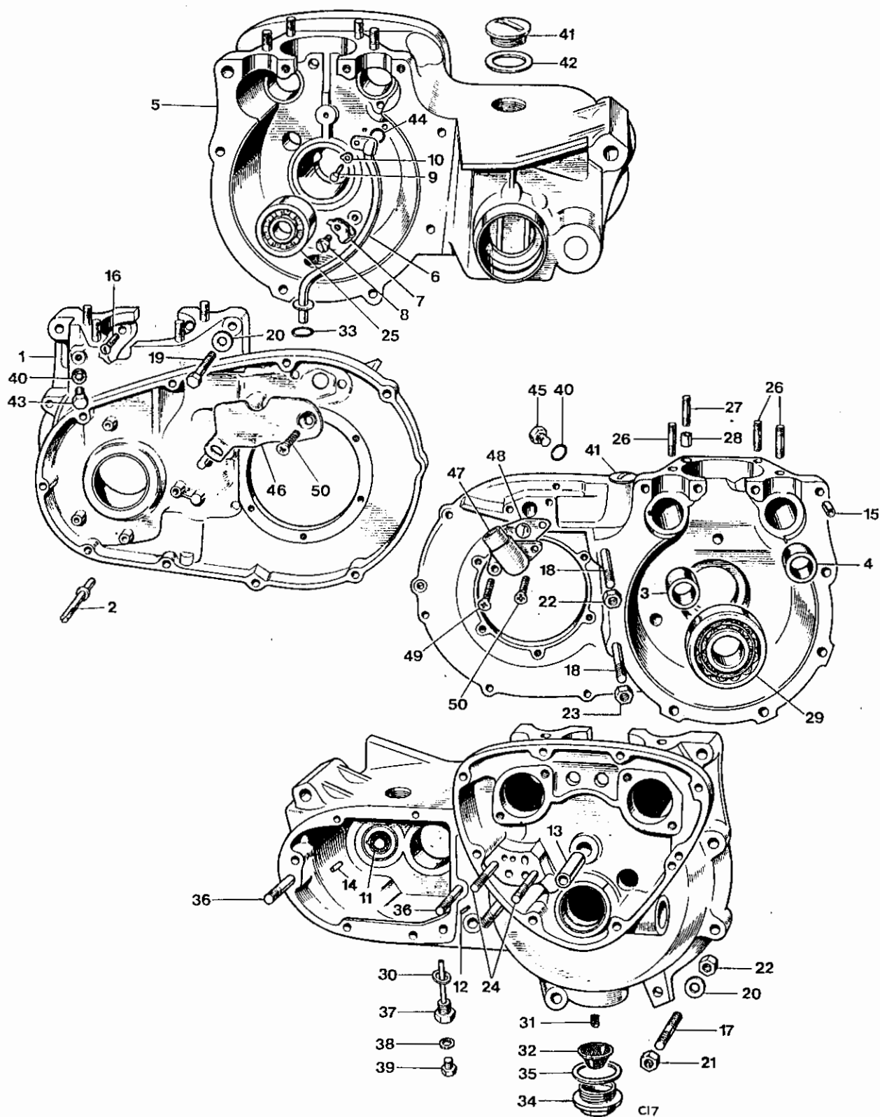
Fig. 2. CRANKCASE
