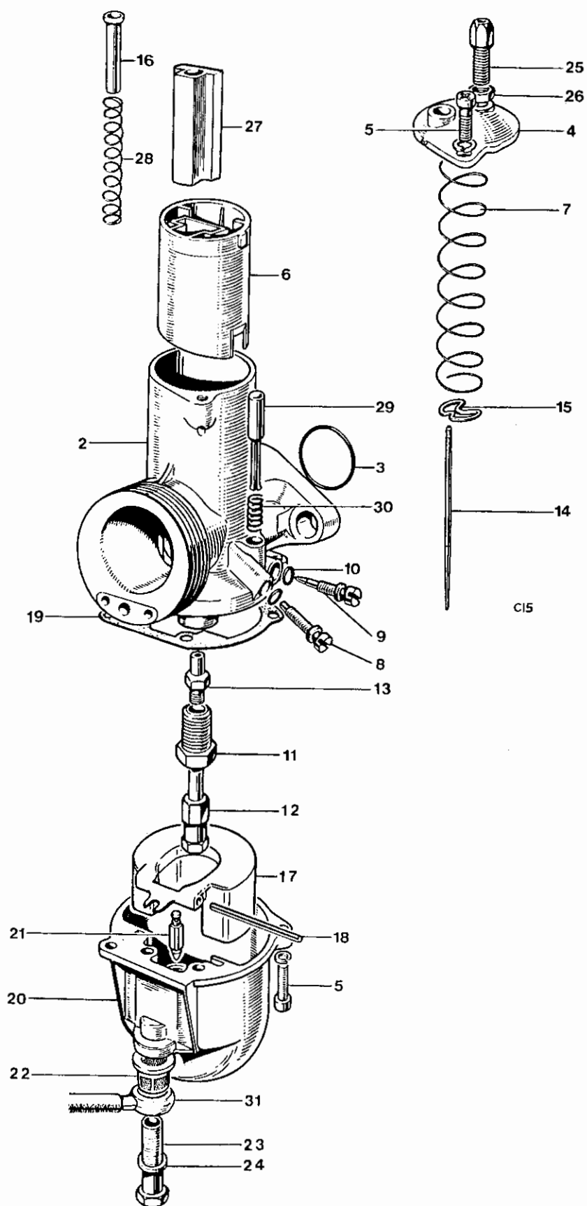
Fig. 31. CARBURETOR T100R
