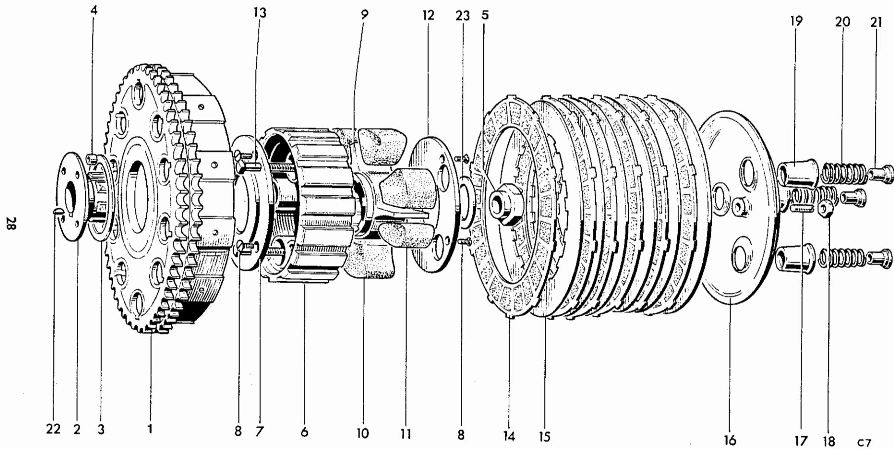
Fig. 11. CLUTCH
