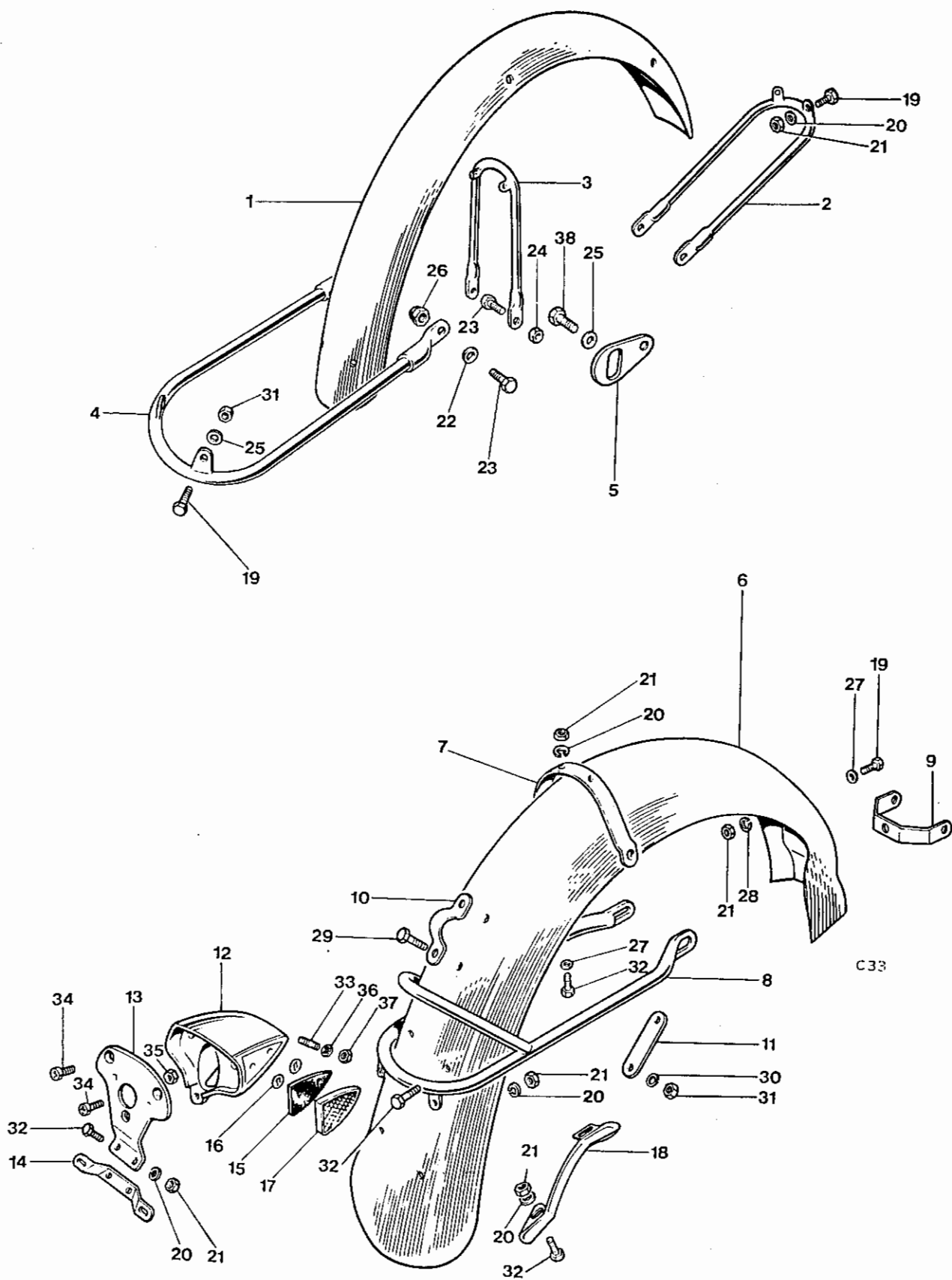
Fig. 23. FENDERS
