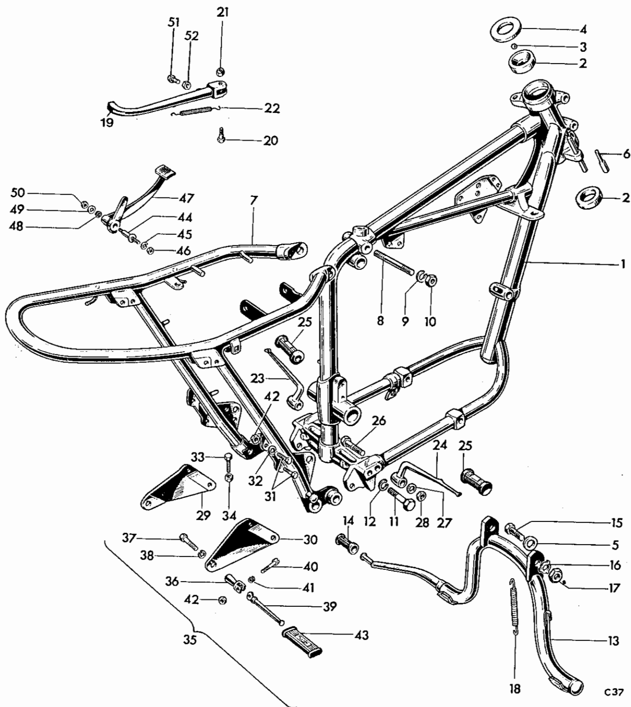
Fig. 15. FRAME
