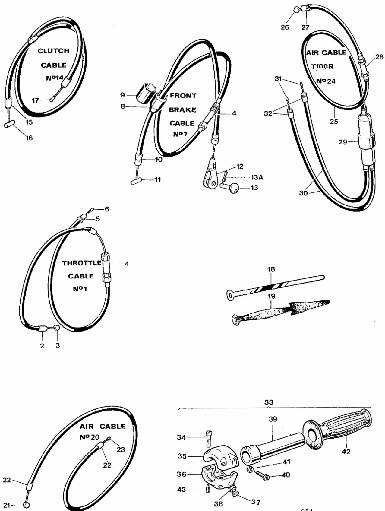
Fig. 29. CONTROL CABLES
