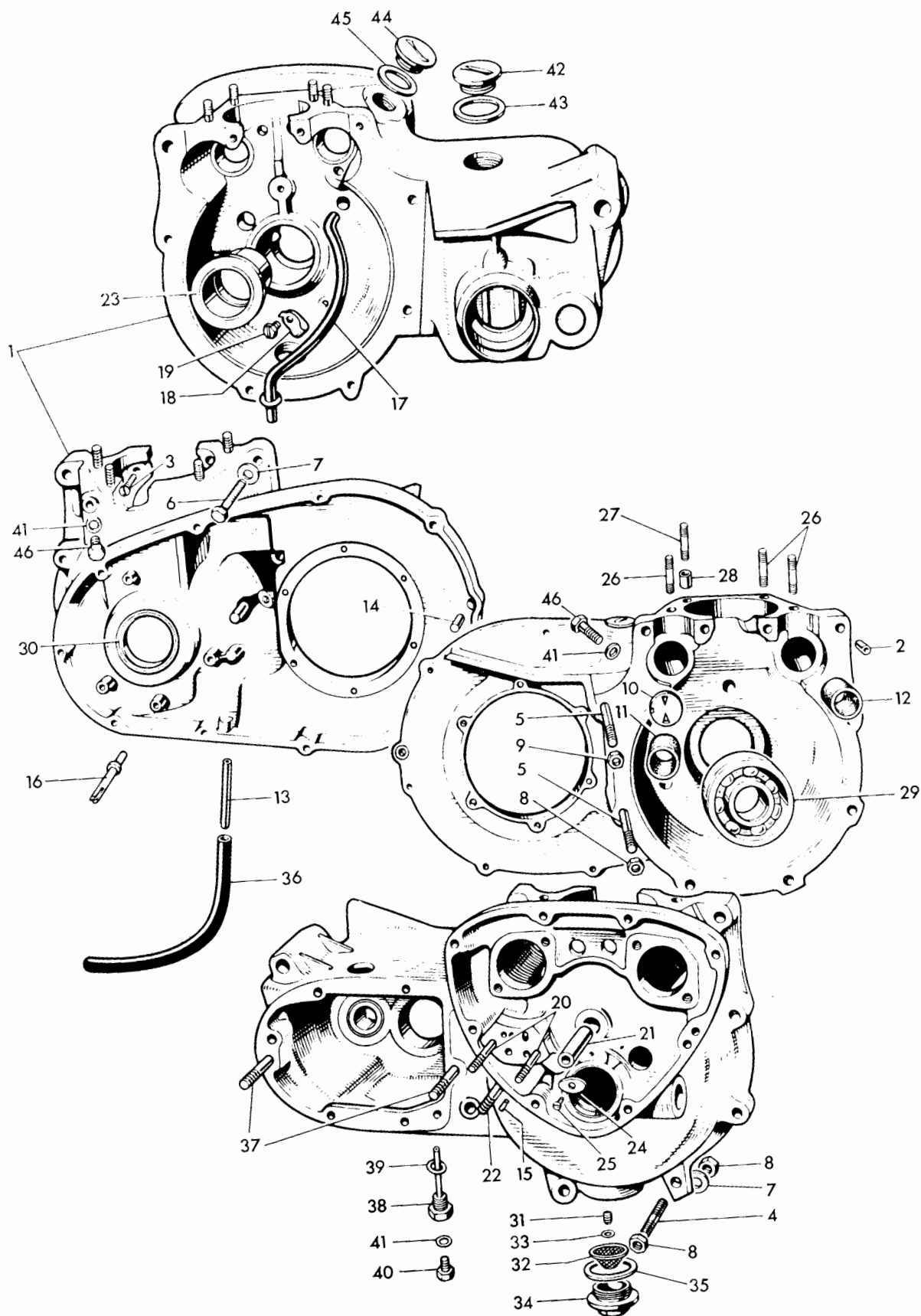
Fig. 2. CRANKCASE
