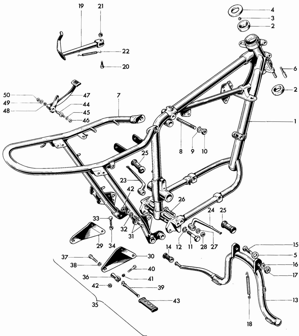
Fig. 15. FRAME
