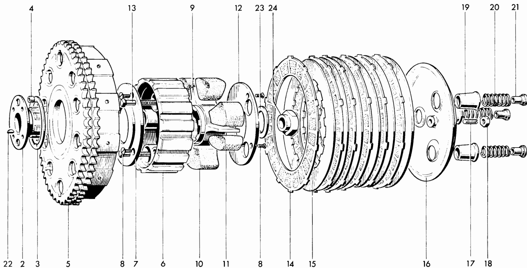
Fig. 11. CLUTCH
