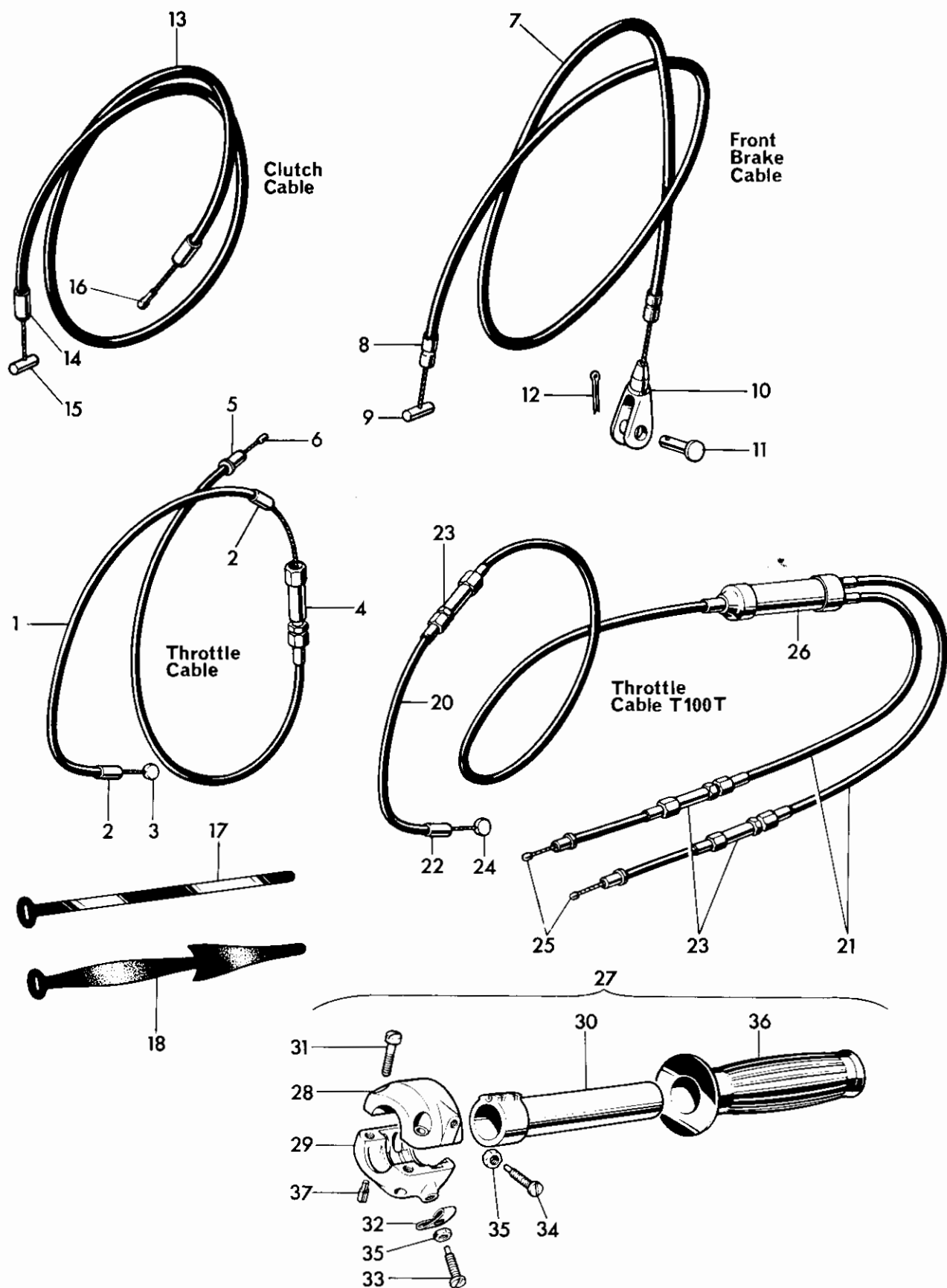
Fig. 28. CONTROL CABLES
