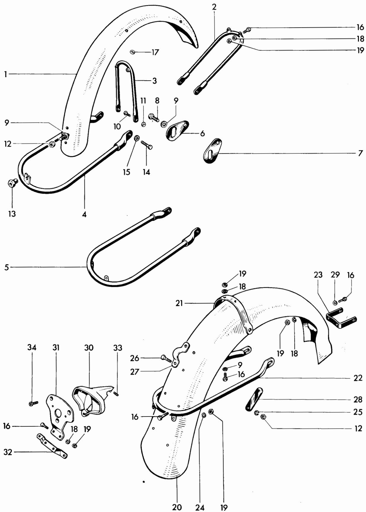
Fig. 23. FENDERS (U.S.A.)
