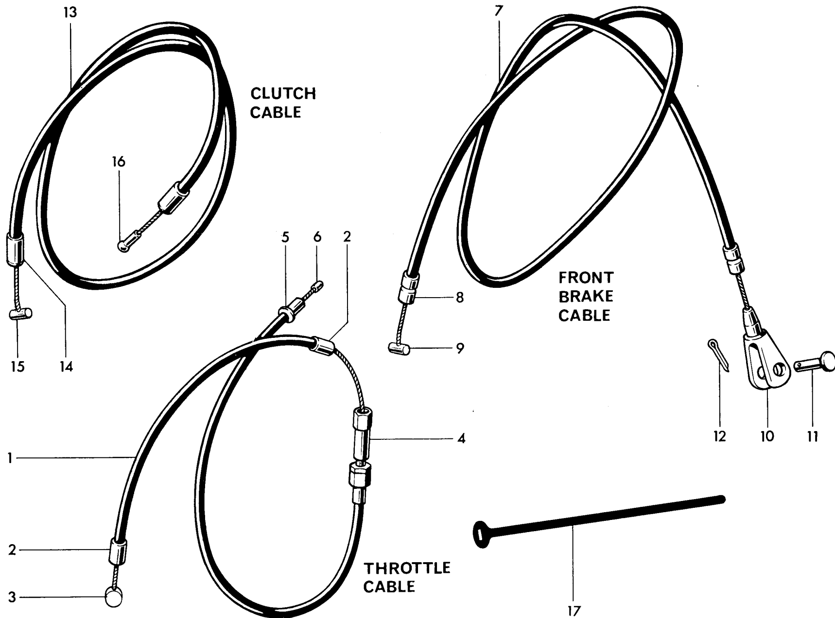
Fig. 29. CONTROL CABLES
