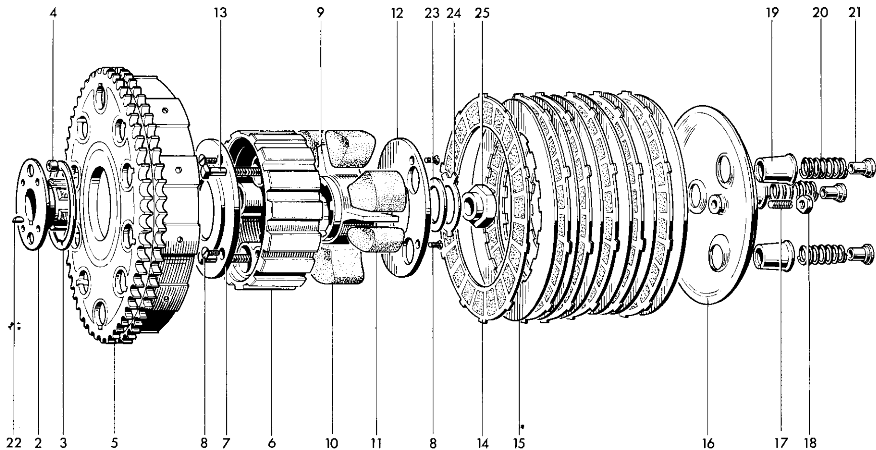
Fig. 9. CLUTCH
