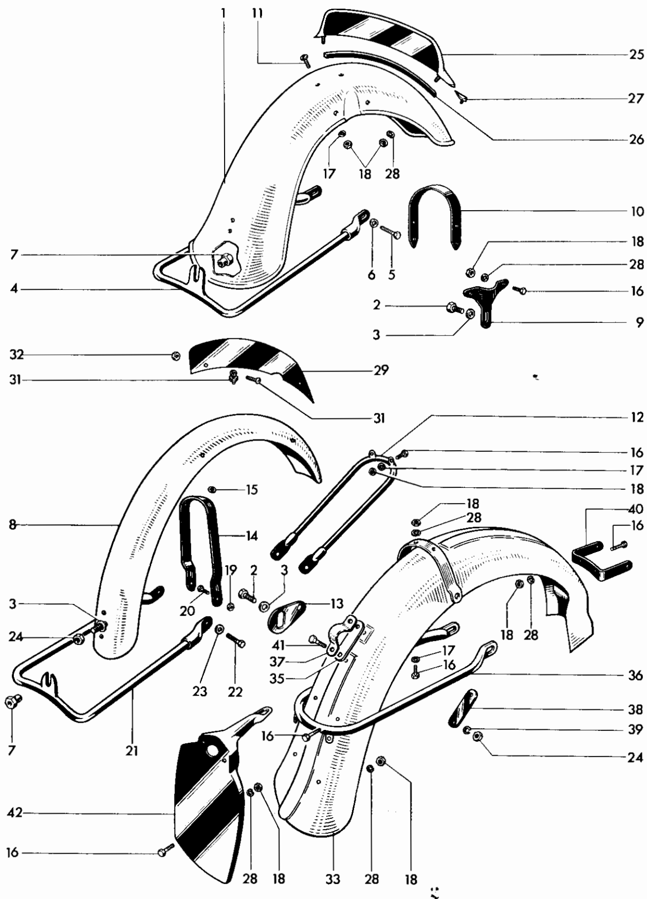
Fig. 20. MUDGUARDS
