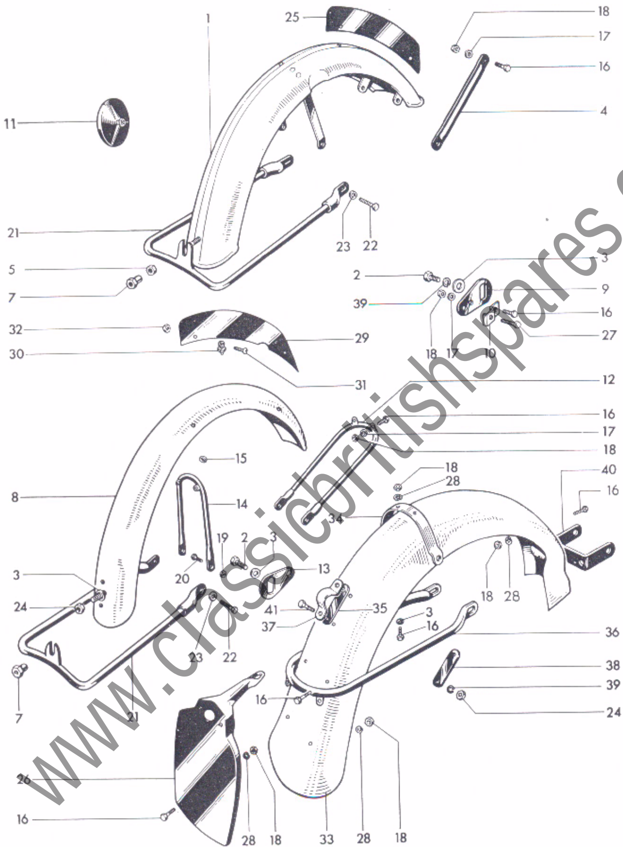
Fig. 20. MUDGUARDS
