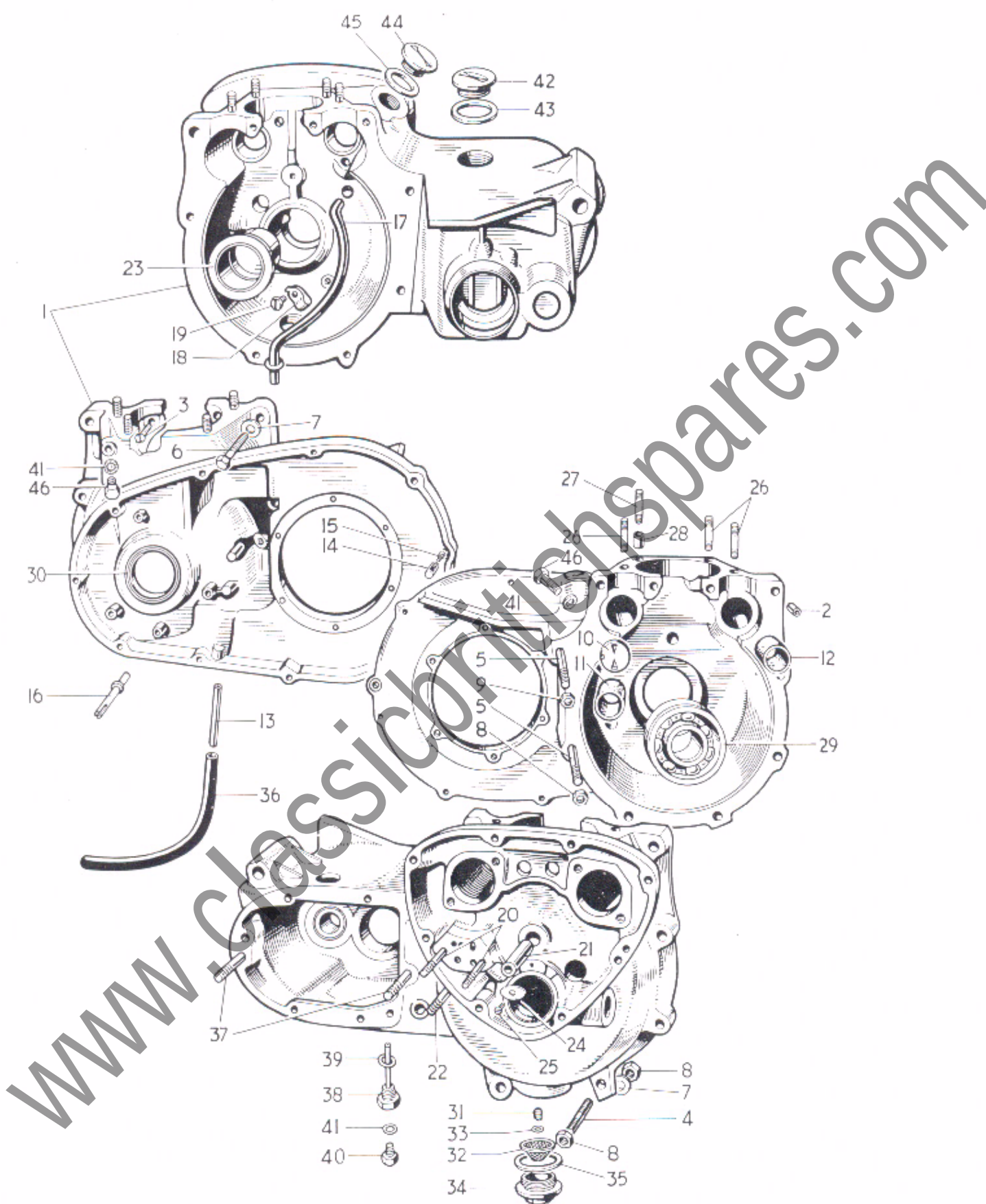
Fig. 2. CRANKCASE
