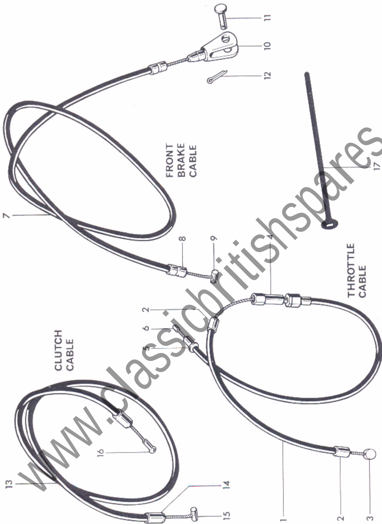
Fig. 26. CONTROL CABLES
