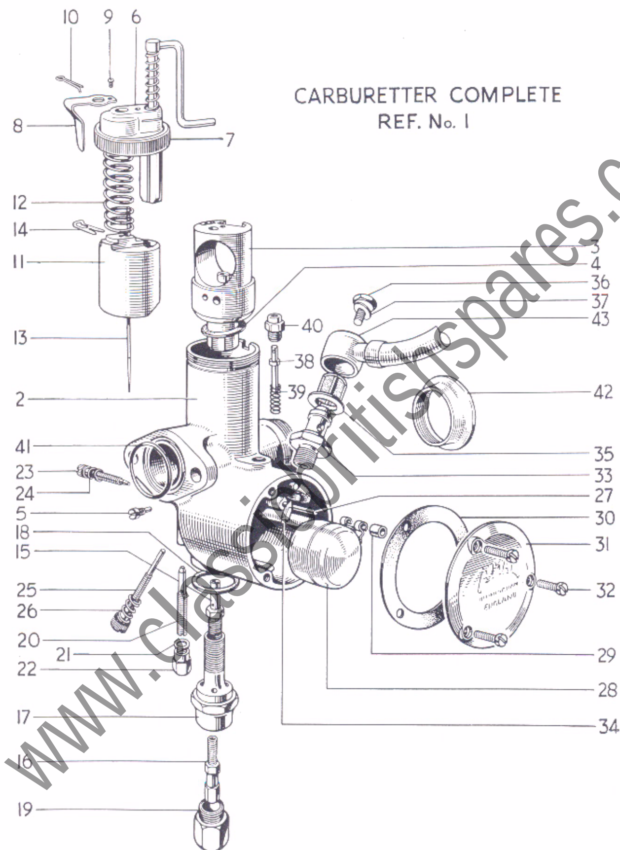
Fig. 23. CARBURETTER.
