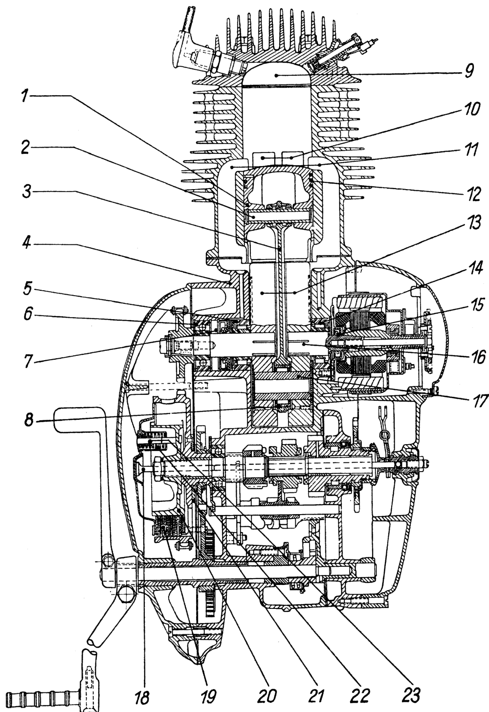
Bild 5. Triebwerkblock im Schnitt
