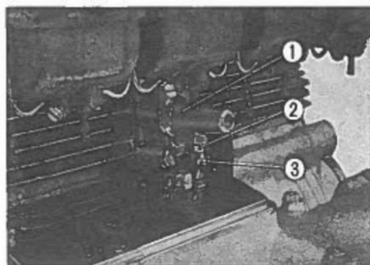
Fig. 2-46 • CB 750. ① Contenitore del tendicatena. ② Controdamo. ③ Vite di fissaggio.
