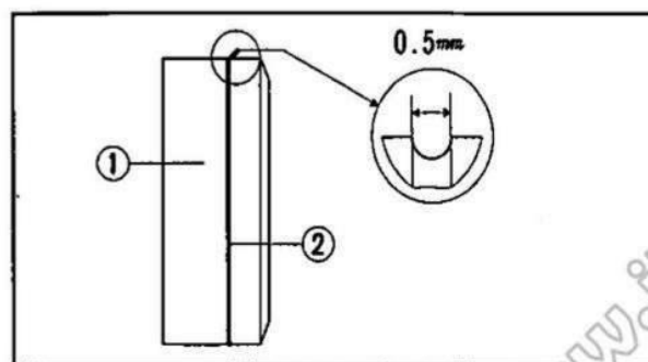
Fig. 4-8 ① Pasticca. ② Solco con linea rossa.
