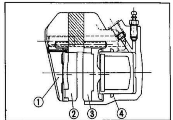
Fig. 4-22 ① Pinza B. ③ Pasticca A. ② Pasticca B. ④ Pinza A.
