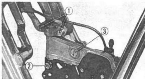
Fig. 4-1 ① Bulloni da 6 mm. ③ Bullone di registro della pinza del freno. ② Dado da 8 mm.
