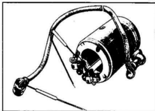
Fig. 5-59 Controllo dell'avvolgimento dello statore.
