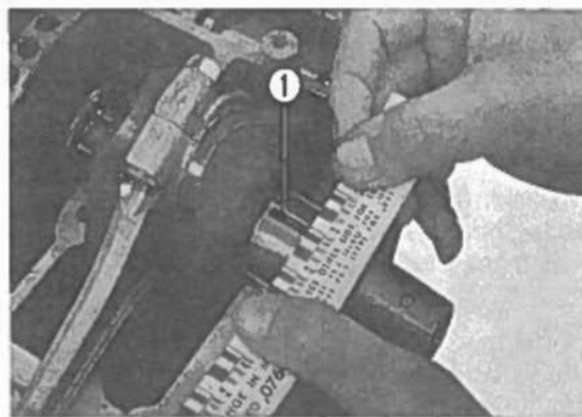
Fig. 3-151 ① Plastigage.
