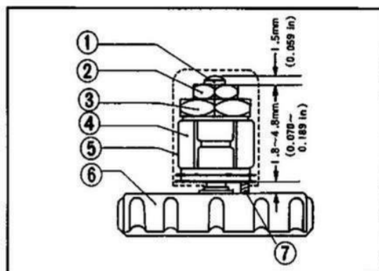
Fig. 2-29 ① Astina filettata. ② Controdado. ③ Dado di regolazione. ④ Braccetto di comando. ⑤ Guaina di gomma. ⑥ Parte superiore del carburatore. ⑦ Spessimetro.
