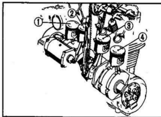
Fig. 2-2 ① Pistone nr 1. ③ Pistone nr 3. ② Pistone nr 2. ④ Pistone nr 4.
