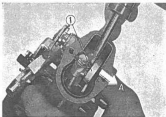
Fig. 3-109 ① Braccetto di unione.
