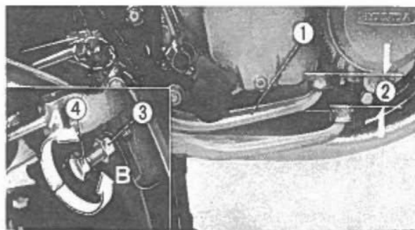
Fig. 2-59 ① Pedale freno posteriore. ② Corsa a vuoto. ③ Controdado. ④ Bullone di registro.
