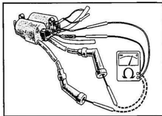
Fig. 5-68 Prova della continuità della bobina.
