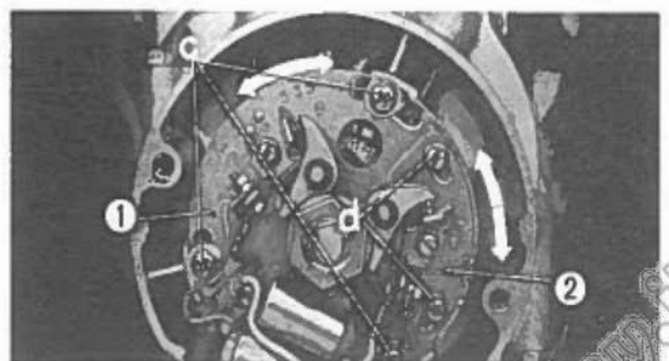
Fig. 2-7 ① Piatto di base delle puntine "e". ② Piatto di base delle puntine "f"
