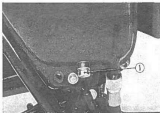
Fig. 2-51 ① Bullone di scarico olio.
