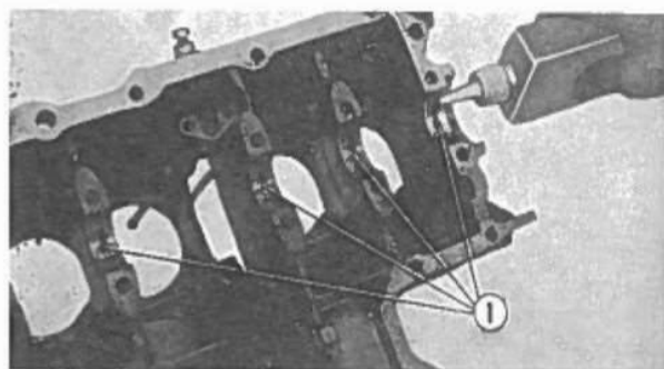
Fig. 3-40 ① Cuscinetti.
