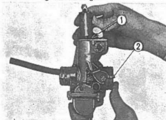
Fig. 3-119 ① Lato smussato. ② Valvola dello starter.
