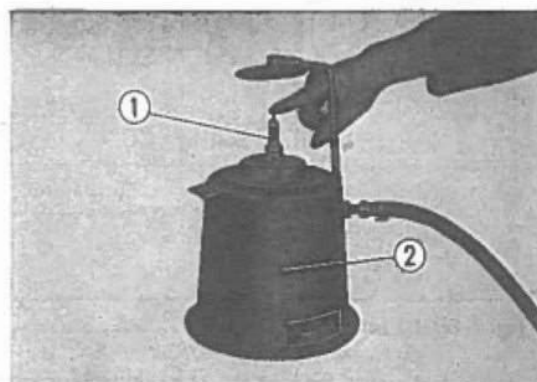
Fig. 5-71 ① Candela. ② Apparecchio per pulizia candele.
