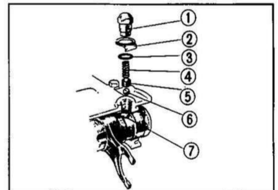
Fig. 3-83 ④ Molla. ① Bullone di fissaggio. ⑤ Cappello della molla. ② Rondella di sicurezza. ⑥ Sfera di acciaio. ③ Gommino di tenuta. ⑦ Parte incavata.
