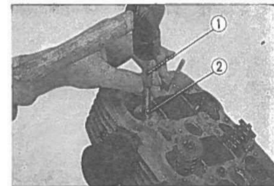
Fig. 3-127 ① Attrezzo per la messa in posto della guida. ② Guidavalvola.
