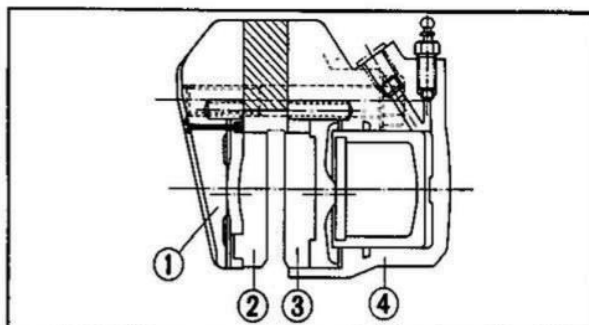
Fig. 4-9 ① Pinza B. ③ Pasticca A. ② Pasticca B. ④ Pinza A.
