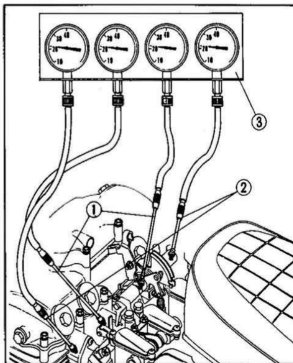
Fig. 2-10 ① tubicino a vite di collegamento "A". ② tubicino a vite di collegamento "B". ③ vacuometro.
