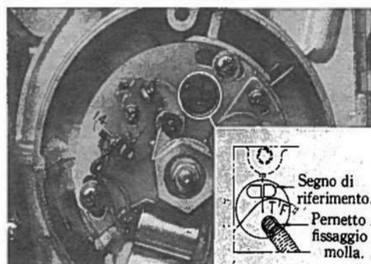
Fig. 2-44 Posizione delle punterie a 15° DPMS.
