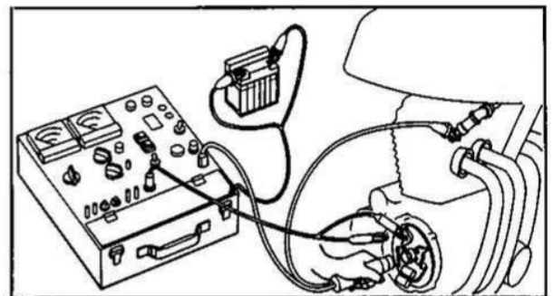
Fig. 2-5 Controllo dell'anticipo di accensione.
