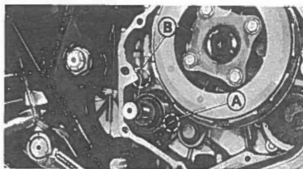
Fig. 3-16 Installazione della molla della messa in moto.
