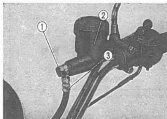
Fig. 4-28 ① Bullone olio. ② Cilindro principale. ③ Cavo dell'olio.
