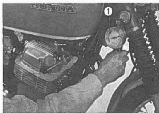
Fig. 2-68 ① Manometro per misurare la compressione.
