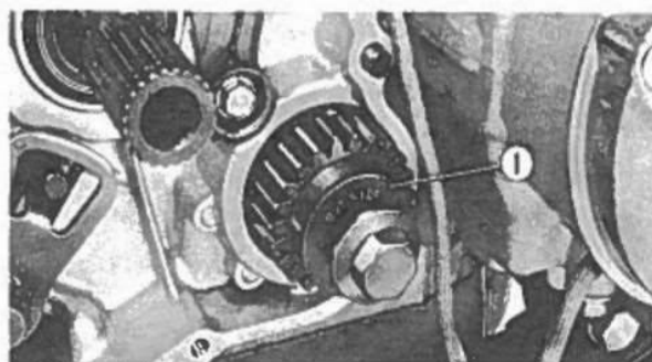
Fig. 3-31 ① Rondella speciale.
