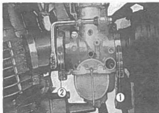
Fig. 3-159 ① Fascetta del filtro aria. ② Fascetta di fissaggio dei carburatori.
