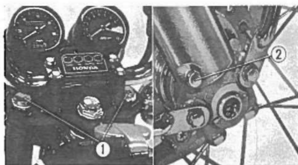
Fig. 2-67 ① Bulloni della forcella anteriore. ② Bulloncini di scarico olio.
