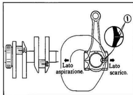
Fig. 3-97 ① Orecchiette di fissaggio del cuscinetto.
