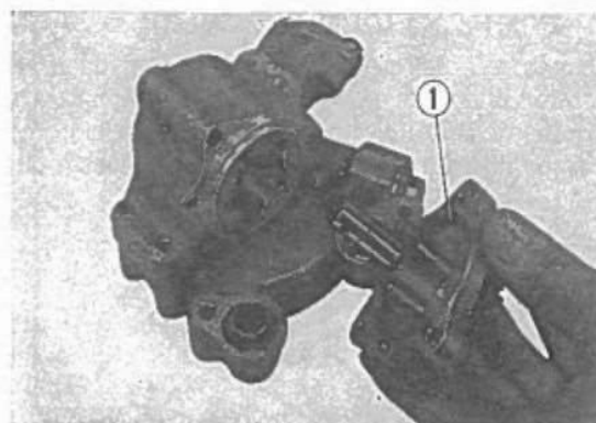
Fig. 3-134 ① Anello di gomma.
