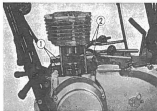
Fig. 3-66 ① Basi dei pistoni. ② Pinze di compressione dei segmenti.
