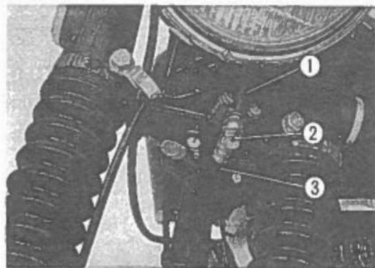
Fig. 4-25 ① Attacco. ② Bullone dell'olio. ③ Cavo del liquido del freno.
