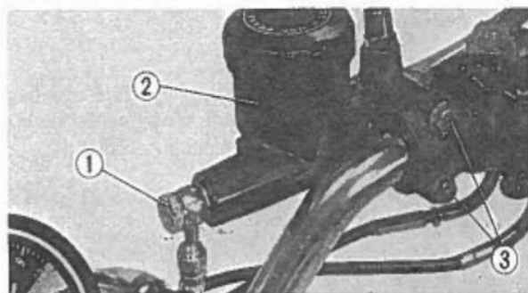
① Bullone dell'olio. ② Cilindro principale. ③ Bulloni esagonali.
