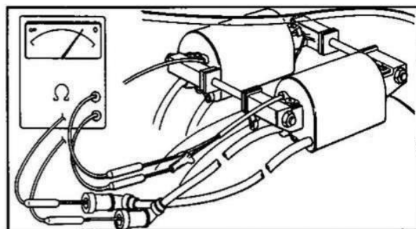
Fig. 5-3 Controllo della continuità dell'avvolgimento della bobina.
