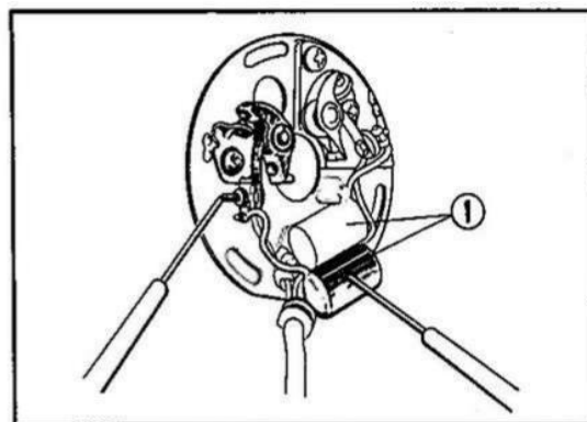
Fig. 5-73 ① Condensatore.
