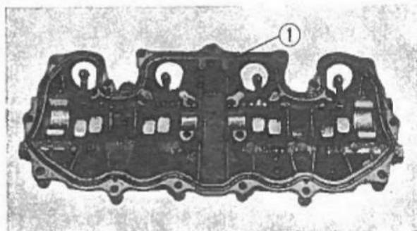
Fig. 3-10 Ordine di serraggio dei bulloni del coperchio della testa.
