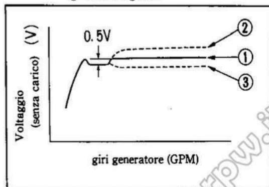
Fig. 5-83 ① Standard. ② Grande apertura del nucleo. ③ Piccola apertura del nucleo.
