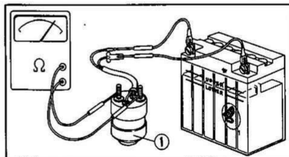
Fig. 5-30 ① Interruttore magnetico di avviamento.
