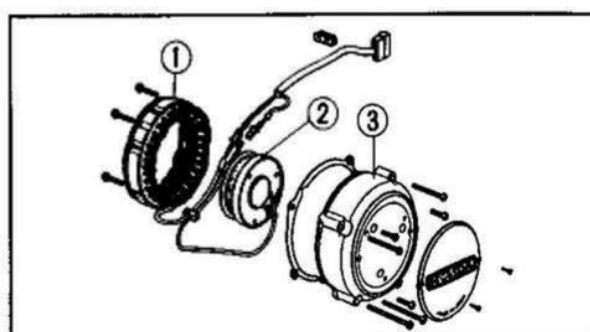
Fig. 5-13 ① Avvolgimento dello statore. ② Avvolgimento di campo. ③ Coperchio del generatore.
