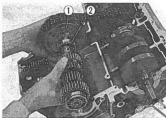
Fig. 3-142 ① Corona della trasmissione primaria. ② Albero primario del carter.
