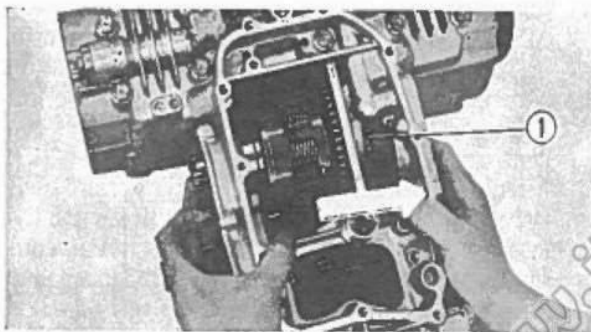
Fig. 3-21 ① Contralbero.
