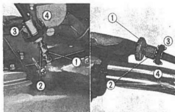
Fig. 2-40 ① Controdado. ② Registro. ③ Aumento della corsa a vuoto. ④ Diminuzione della corsa a vuoto.
