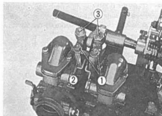
Fig.3-105 ① Dadi esagonali. ② Piastrina parapolvere B. ③ Dadi a cappello.
