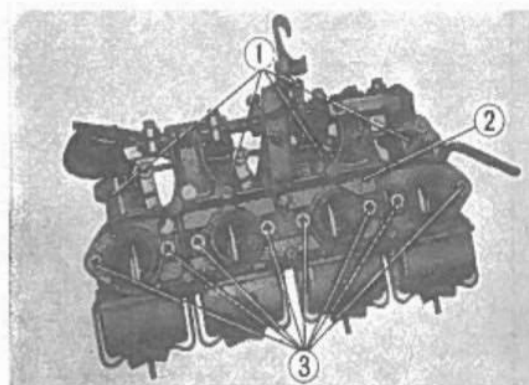
Fig. 3-160 ① Carburatori. ③ Viti. ② Piastra di fissaggio.
