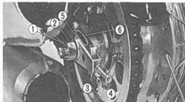
Fig. 2-65 ① Coppiglia. ④ Bullone di registro. ② Dado asse ruota. ⑤ Segno di riferimento. ③ Controdado. ⑥ Tacche del forcellone.
