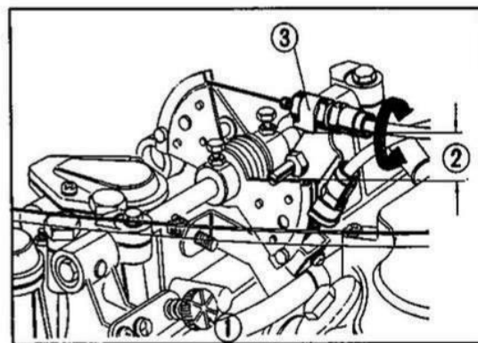
Fig. 2-20 ① Vite di registro del minimo. ② 49 \pm 1 mm. ③ Supporto del registro del cavo del gas.
