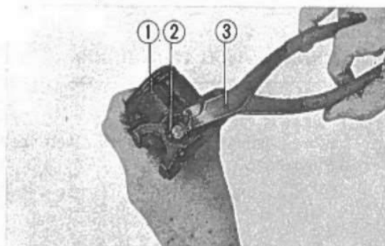
Fig. 4-18 ① Corpo del cilindro principale. ② Anello Seeger. ③ Pinze speciali.
