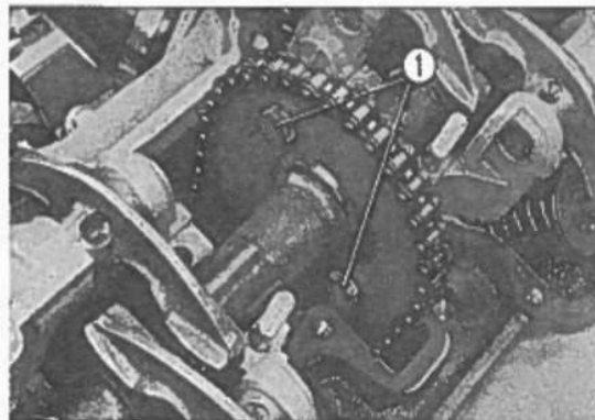
Fig. 3-131 ① Bulloncini di fissaggio del pignone dell'asse a camme.
