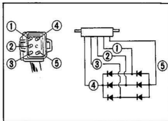
Fig. 5-51 ①, ②, ③ Giallo ⑤ Verde. ④ Giallo/Bianco.
