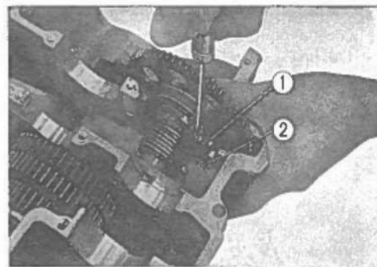
Fig. 3-138 ① Flangia della ruota libera. ② Molla di ritorno.
