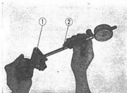
Fig. 4-32 ① Corpo del cilindro principale. ② Alesametro.
