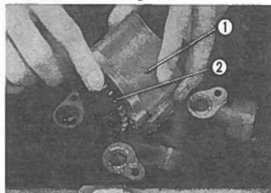
Fig. 3-135 ① Complesso della pompa dell'olio. ② Ingranaggio di comando della pompa.
