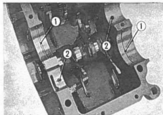
Fig. 3-87 ① Semianelli di fermo dei cuscinetti. ② Grani di fissaggio.
