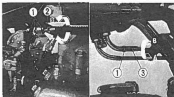
Fig. 2-16 ① Controdado. ② Dado di registro. ③ Registro del cavetto del gas.
