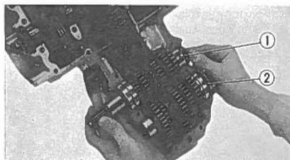
Fig. 3-23 ① Albero primario. ② Albero secondario.
