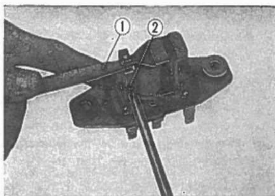
Fig. 5-84 ① Spessoremetro. ② Vite di regolazione della distanza dal nucleo.
