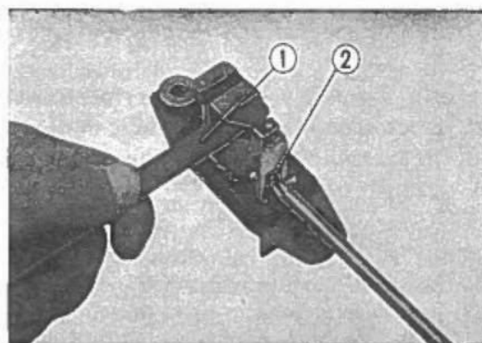
Fig. 5-85 ① Spessoremetro. ② Vite di fissaggio della apertura delle puntine.
