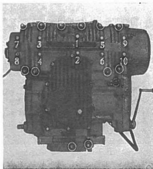
Fig. 3-156 Ordine di serraggio.
