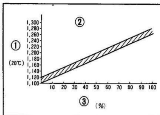
Fig. 5-64 ① Densità. ② Relazione tra densità e carica. ③ Carica residua (%).
