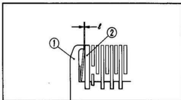
Fig. 3-13 ① Centro frizione. ② Disco B.
