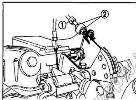
Fig. 2-34 Registrazione del cavetto del gas.
