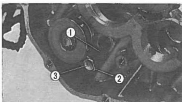
Fig. 3-25 ① Piastrina di fermo del perno dei forcellini. ② Rondella di sicurezza. ③ Bullone da 8 mm.
