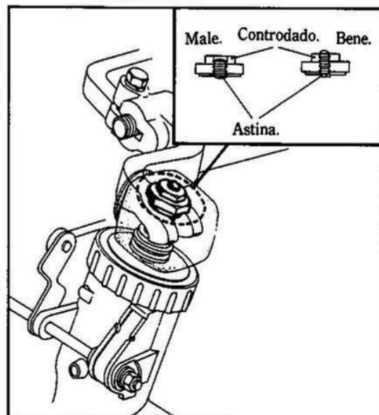
Fig. 2-30 CONTRODADO
