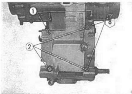
Fig. 3-103 ① Bulloni da 6 mm. ② Bulloni da 8 mm.
