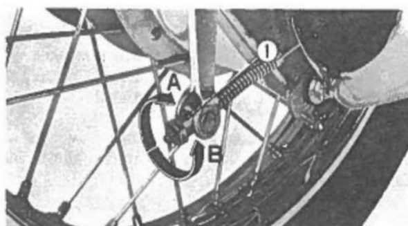
Fig. 2-60 ① Bullone di registro.
