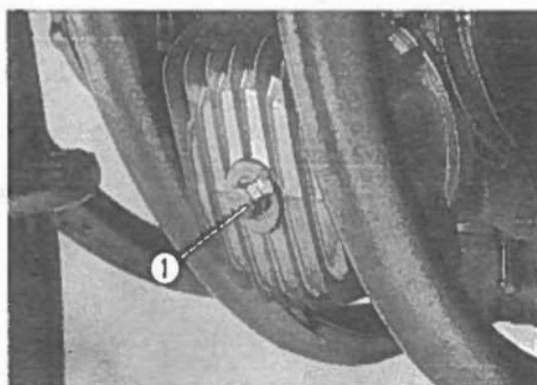
Fig. 2-53 ① Bullone centrale del filtro dell'olio.
