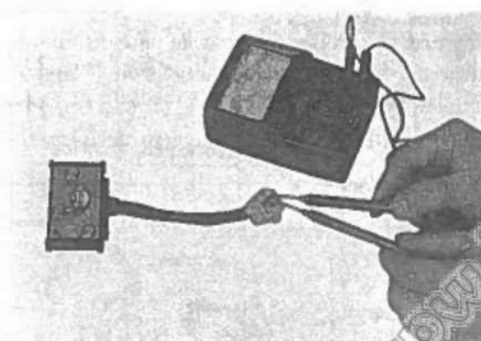
Fig. 5-50 Controllo del raddrizzatore al silicio.
