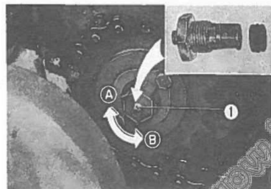
Fig. 2-66 ① Vite di registro. A Flusso dell'olio diminuisce. B Flusso dell'olio aumenta.
