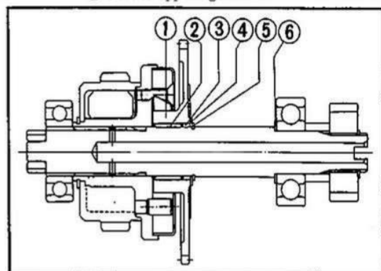
Fig. 3-90 ① Ingranaggio messa in moto. ② Cuscinetto ad aghi (25 x 29 x 17) ③ Collarino da 25 mm. ④ Rondella da 25 mm. ⑤ Anello Seeger da 25 mm. ⑥ Rondella da 22 mm.
