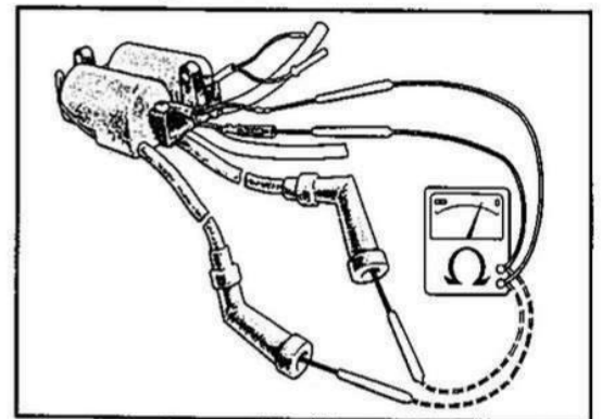
Fig. 5-37 Controllo della continuità della bobina di accensione.
