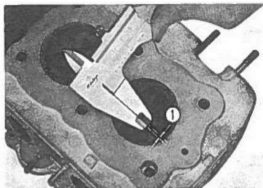
Fig. 3-61 ① Larghezza della sede valvola.
