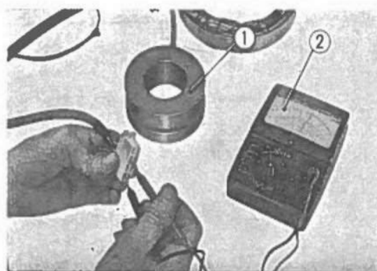
Fig. 5-78 ① Avvolgimento di campo. ② Tester.
