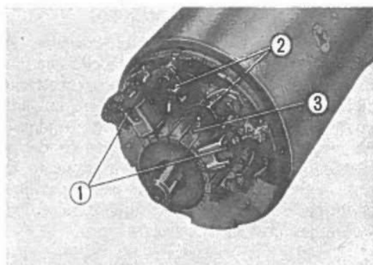
Fig. 5-58 ① Spazzole. ② Molle. ③ Commutatore.
