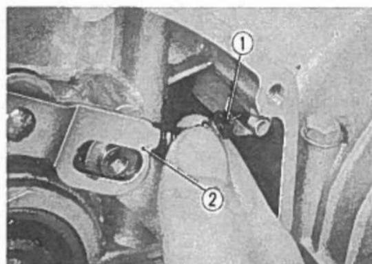
Fig. 3-86 ① Molla. ② Braccetto di fermo del tamburo selettore.
