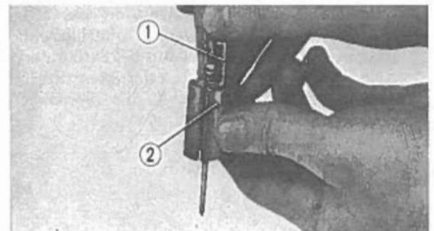
Fig. 3-55 ① Piastrina della valvola. ② Valvola del gas.
