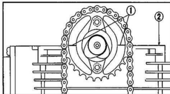
Fig. 3-8 ① Linea di riferimento del pignone dell'asse a cammes. ② Superficie superiore della testata.
