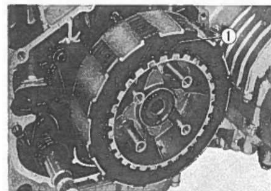
Fig. 3-75 ① Solchi per l'olio.
