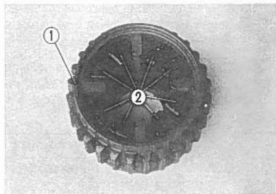
Fig. 3-89 ① Corona della trasmissione primaria. ② Parastrappi in gomma.
