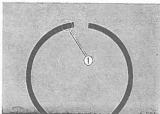
Fig. 3-124 ① Lettera stampigliata.
