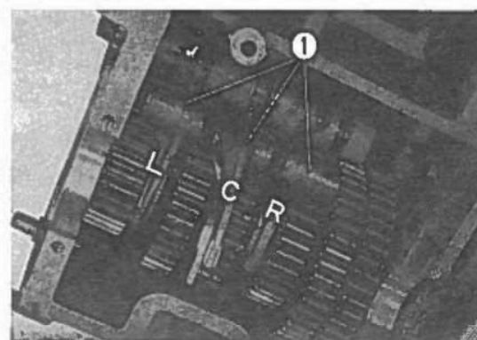
Fig. 3-145 ① Forchette del cambio.
