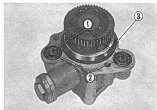
Fig. 3-74 ① Boccoletta di passaggio olio. ② Gommino da 14 mm. ③ Gommino da 47 mm.
