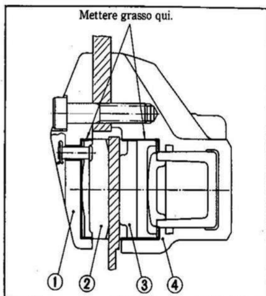
Fig. 4-33 ① Pinza B. ③ Pasticca A. ② Pasticca B. ④ Pinza A.
