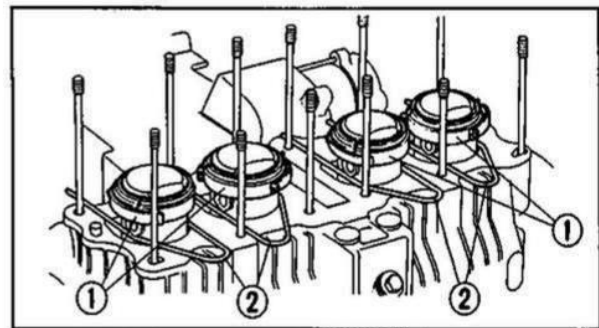
Fig. 3-5 ① Compressori dei segmenti. ② Basi dei pistoni.
