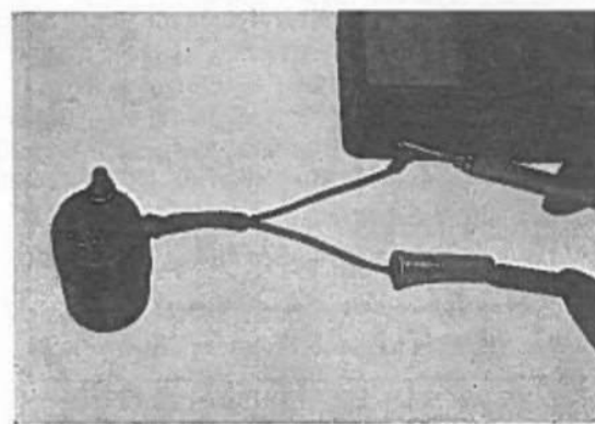
Fig. 5-62 Prova della continuità dell'avvolgimento primario.
