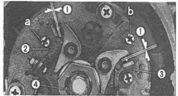
Fig. 2-4 ① Apertura delle puntine. ③ Base delle puntine 2,3. ② Base delle puntine 1,4. ④ Dado speciale.
