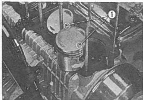
Fig. 3-64 ① Freccie stampigliate sul cielo dei pistoni.
