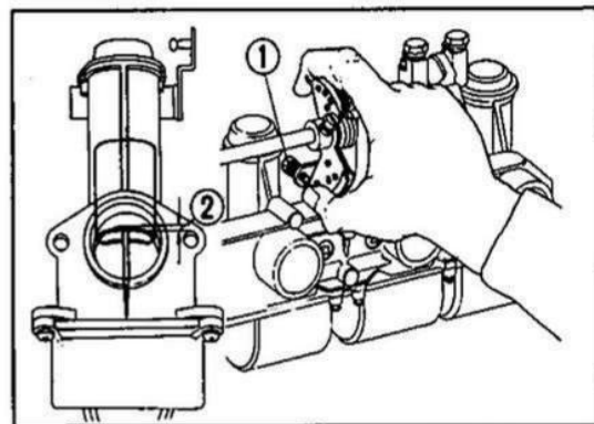
Fig. 2-26 ① Vite di fondocorsa. ② 0-1,0 mm.
