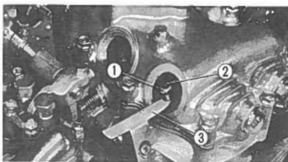
Fig. 2-3 ① Controdado. ③ Spessimetro. ② Vite di registro.
