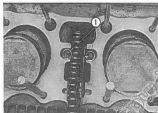
Fig. 3-149 ① Blocchetti di gomma.
