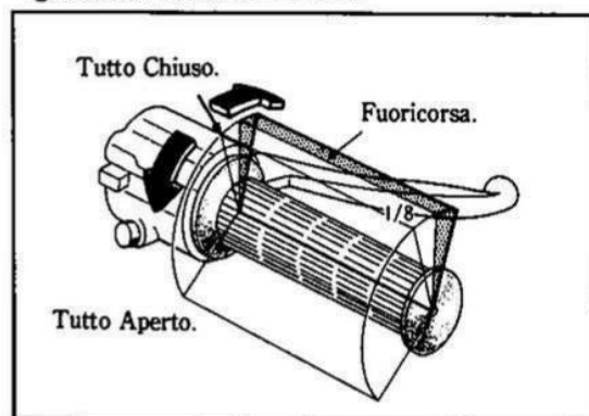
Fig. 2-32 Spostamento di fuoricorsa.
