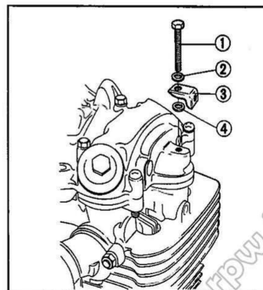
Fig. 3-71 ① Vite da 6 mm. ② Rondella di rame cromato. ③ Piastrina laterale del coperchio testa. ④ Rondella di alluminio.
