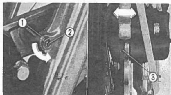
Fig. 2-56 ① Controdado. ② Bullone di registro. ③ Pasticca B.
