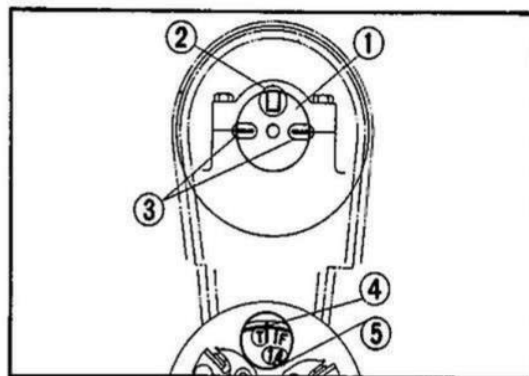
Fig. 3-130 ① Asse a camme. ④ Segno "T". ② Tacca. ⑤ Segno 1,4. ③ Linee di riferimento.
