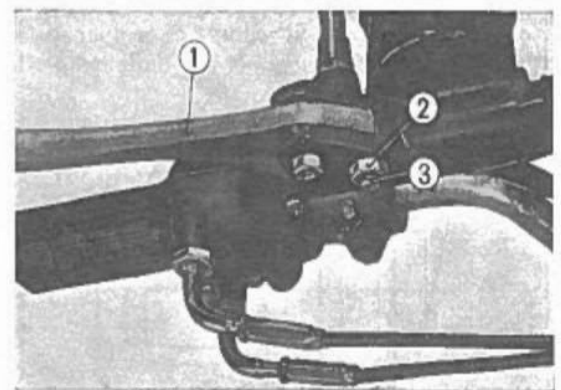
Fig. 4-30 ① Leva del freno anteriore. ② Controdado. ③ Bullone di registro della leva.
