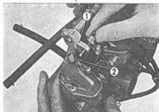
Fig.3-106 ① Braccetto di unione. ② Portaregistri.
