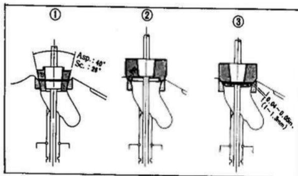
Fig. 3-123 ① Fresetta interna. ② Fresetta per la parte superiore della sede. ③ Fresetta 90°
