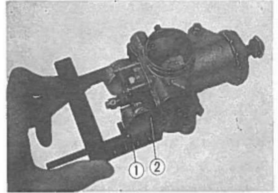
Fig. 3-163 ① galleggiante. ② mascherina di misura del livello.
