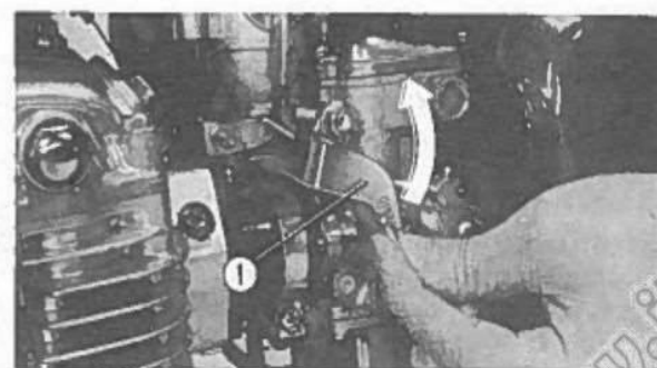
Fig. 2-14 ① Leva dello starter.
