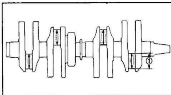
Fig. 3-36 Diametro esterno dei perni di biella.
