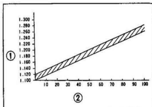
Fig. 5-94 ① Densità (a 20°C). ② Capacità residua (%).
