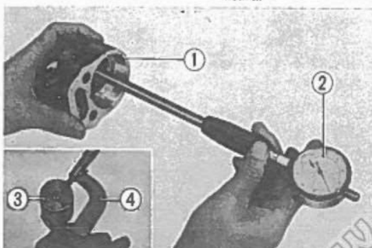
Fig. 4-20 ① Cilindro delle pinze. ③ Pistone. ② Alesametro. ④ Micrometro.
