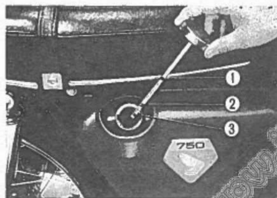
Fig. 2-50 ① Astina di controllo livello olio. ② Tacca del livello superiore ③ Tacca del livello inferiore.
