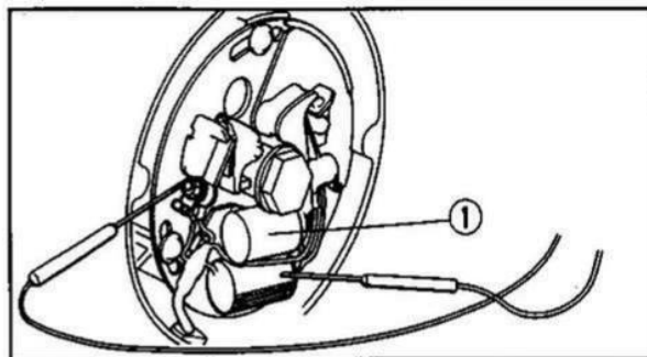
Fig. 5-8 ① Condensatori.
