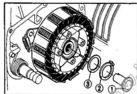
Fig. 3-76 ② Rondella di rasamento. ① Anello Seeger da 25 mm.
