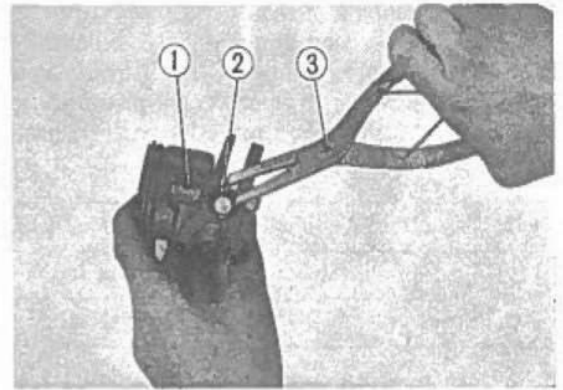
Fig. 4-29 ① Corpo del cilindro principale. ② Anello Seeger. ③ Pinze speciali.
