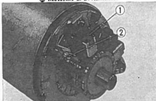
Fig. 5-88 ① Spazzola. ② Vite montaggio spazzola.
