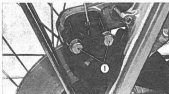
Fig. 4-2 ① Bulloni di fissaggio della pinza.
