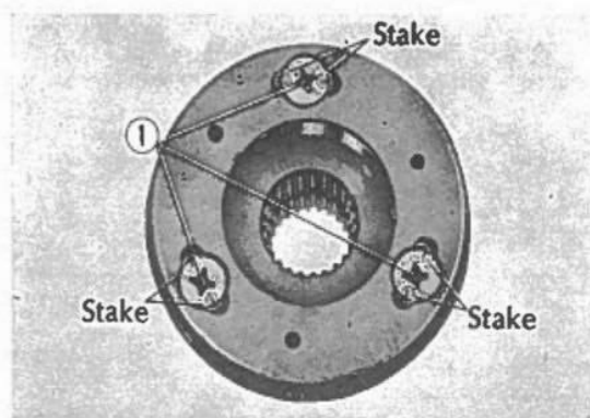
Fig. 3-88 ① Vite da 6 mm. a testa piana. STAKE = Punzonatura.
