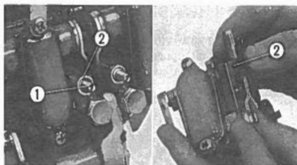
Fig. 3-50 ① Vite di registro. ② Portaregistro.
