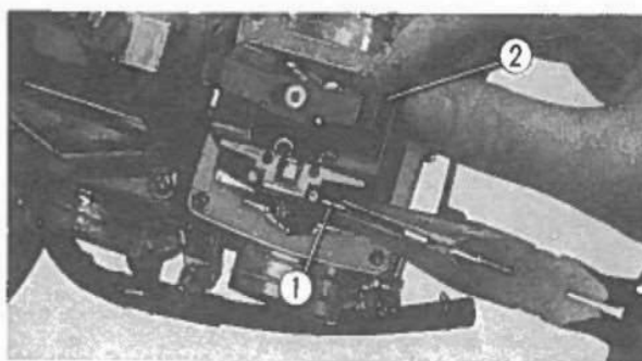
Fig. 3-52 ① Pernetto del galleggiante. ② Galleggiante.
