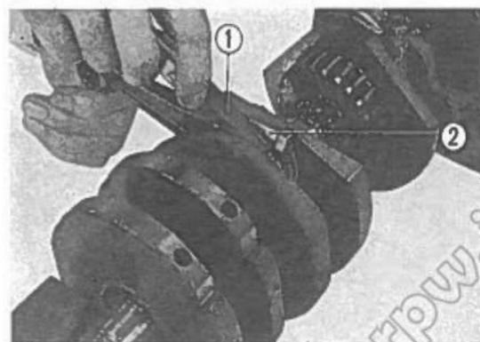
Fig. 3-99 ① Spessimetro. ② Biella.
