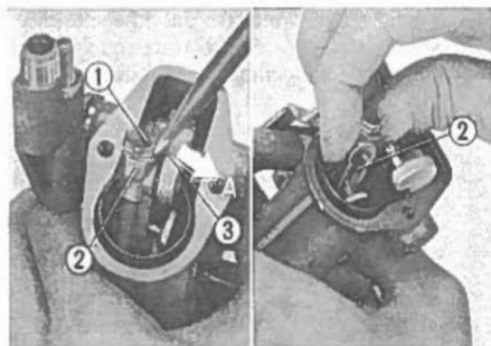
Fig. 3-110 ① Bullone da 6 mm. ② Astina della valvola del gas. ③ Braccetto di unione.
