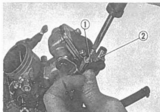
Fig. 3-112 ① Vite di registro. ② Portaregistro.
