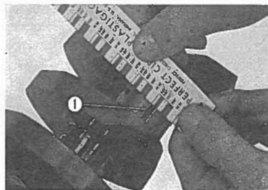
Fig. 3-154 ① Plastigage.
