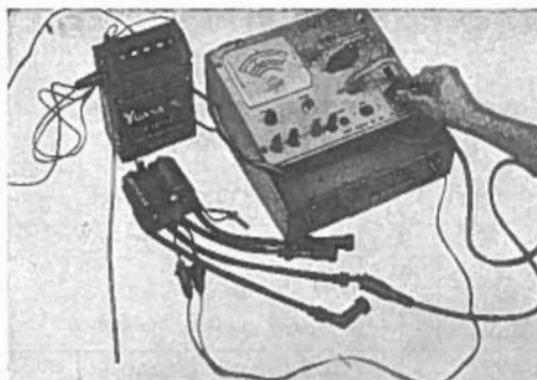
Fig. 5-69 Prova della bobina di accensione.
