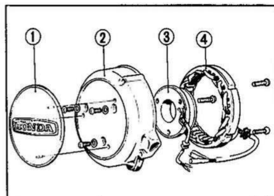
Fig. 5-47 ① Coperchio laterale. ② Coperchio del generatore. ③ Avvolgimento di campo. ④ Avvolgimento dello statore.
