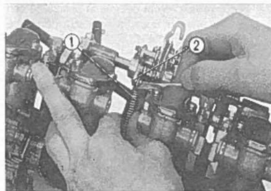
Fig.3-104 ① Molla di ritorno della leva del gas.
