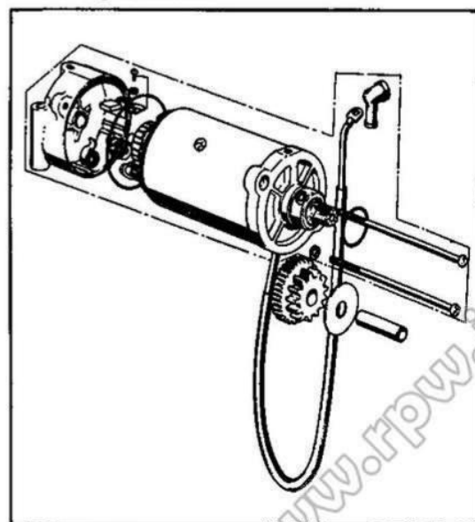
Fig. 5-57 Disegno dello smontaggio del motorino di avviamento.
