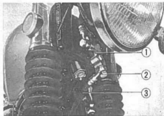
Fig. 4-14 ① Attacco del cavetto. ② Bullone dell'attacco. ③ Cavetto del liquido del freno.
