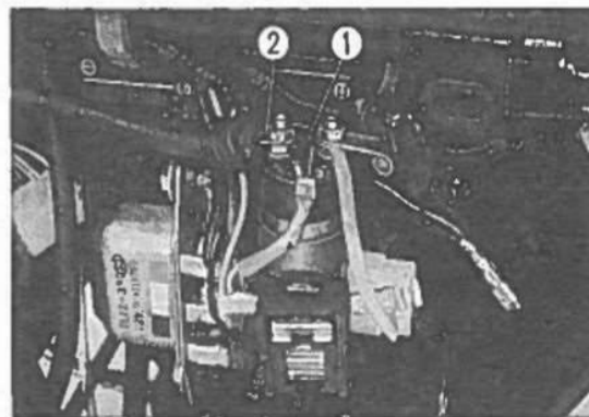
Fig. 5-91 ① Interruttore magnetico. ② Cavetto del motore di avviamento.
