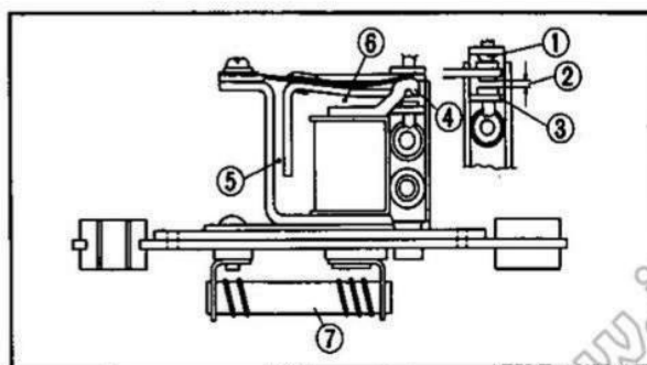
Fig. 5-18 ① Puntine (contatto superiore). ② Apertura delle puntine. ③ Puntine (contatto inferiore). ④ Braccetto di regolazione. ⑤ Apertura angolare. ⑥ Apertura dell'armatura. ⑦ Resistenza.
