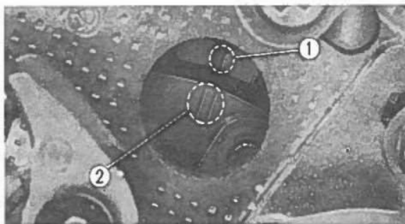
Fig. 2-8 ① segno fisso di riferimento. ② segni dell'anticipo massimo.
