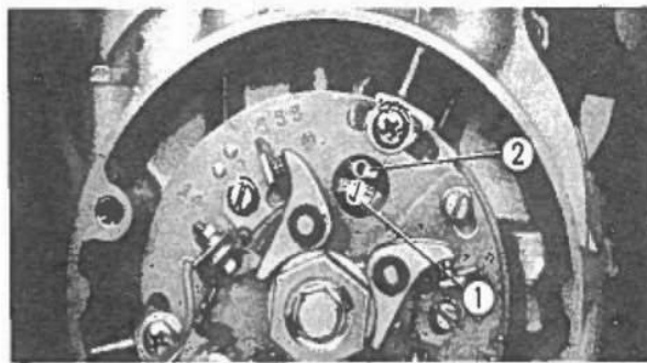
Fig. 3-7 ① Indice "T" 1,4 ② Indice fisso di riferimento.
