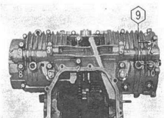
Fig. 3-101 Bulloni da 8 mm.
