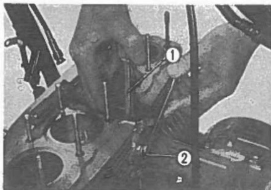
Fig. 3-67 ① Tendicatena. ② Controdado.
