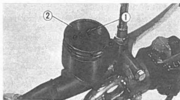
Fig. 2-55 ① Linea di livello. ② Serbatoio liquido freni.
