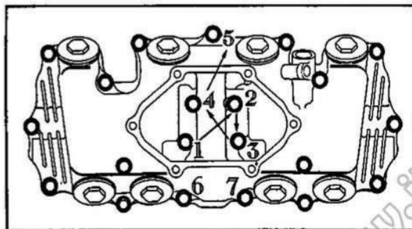
Fig. 3-9 Guarnizione coperchio testa.
