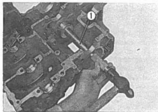
Fig. 3-146 ① Attrezzo per il montaggio del cuscinetto.
