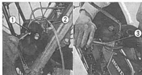
Fig. 2-57 ① Valvolina di spurgo. ② Tubetto di Plastica trasparente. ③ Leva del freno.
