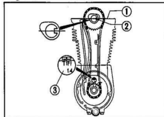
Fig. ① Superficie di appoggio del coperchio testa. 3-69 ② Tacca di riferimento. ③ Piatto dell'anticipo.
