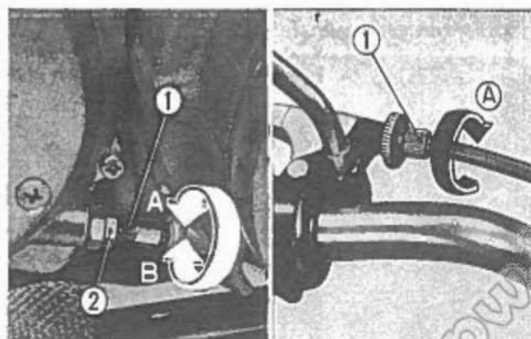
Fig. 2-42 ① Bullone di registro del cavetto della frizione. ② Controdado.
