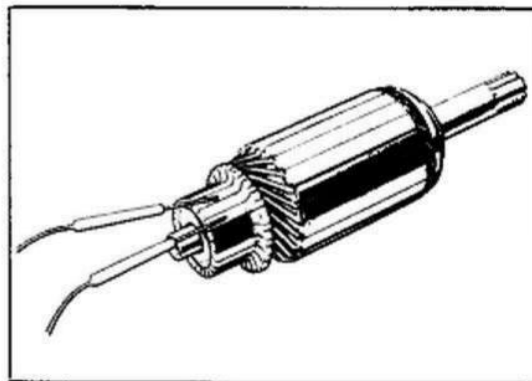
Fig. 5-60 Controllo dell'avvolgimento della armatura.
