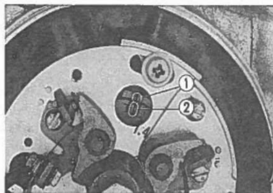
Fig. 3-129 ① Segno fisso di riferimento. ② Segno "T".
