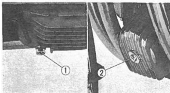
Fig. 2-48 ① Bullone scarico olio. • CB 350 F. ② Bullone centrale del filtro dell'olio.
