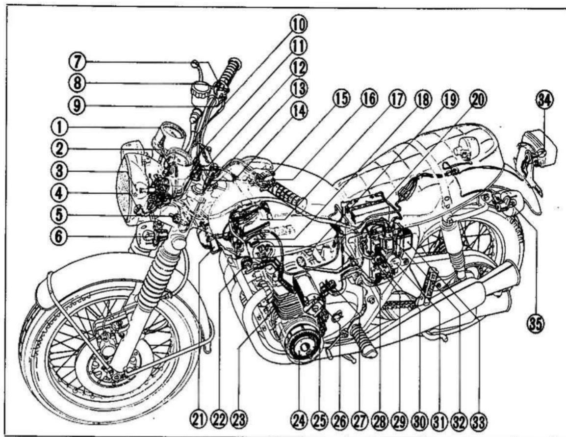
Fig. 5-34 Diagramma completo del sistema elettrico.
