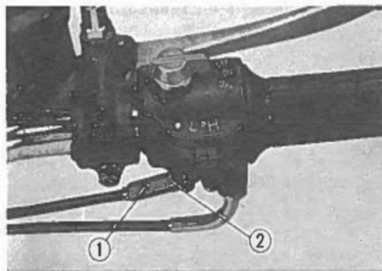
Fig. 2-23 ① Registro. ② Controdado.
