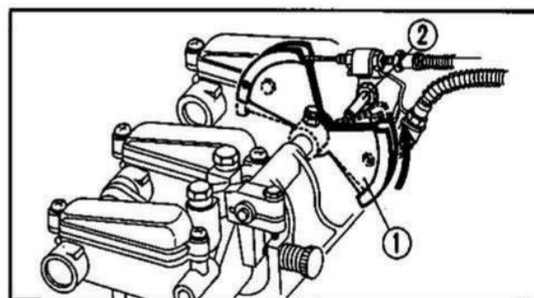
Fig. 2-17 ① Leva del gas. ② Pernetto di fermo.
