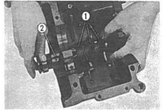
Fig. 3-81 ① Forcellini del cambio. ② Tamburo selettore
