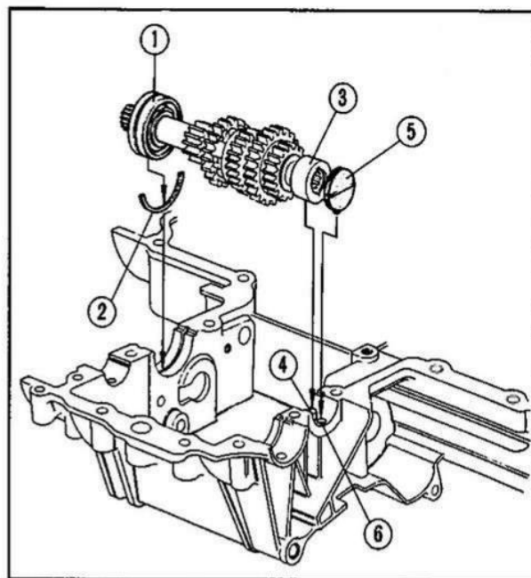
Fig. 3-26 ① Cuscinetto a sfera 5205 HS. ② Semianello di fermo da 52 mm. ③ Cuscinetto ad aghi da 20 mm. ④ Spina di fermo da 6 mm. ⑤ Paraolio. ⑥ Foro di fermo.
