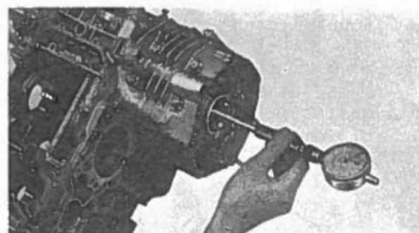
Fig. 3-34 Controllo del diametro interno dei supporti di banco.
