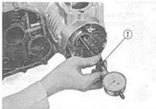
Fig. 3-93 ① Alesametro.
