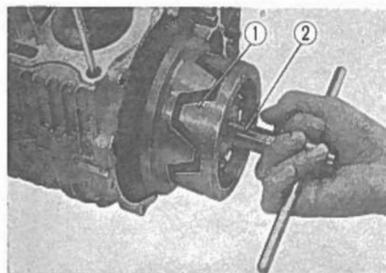
Fig. 3-139 ① Rotore del generatore. ② Estrattore del generatore.
