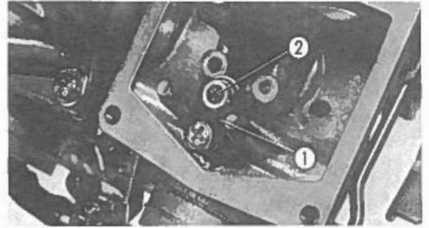
Fig. 3-35 ① Piastrina di fermo. ② Sede della valvolina.
