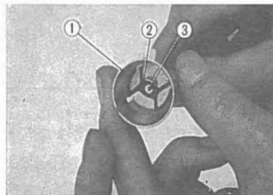
Fig. 3-161 ① Valvola del gas. ③ Spillo conico. ② Piastrina di fissaggio dello spillo.
