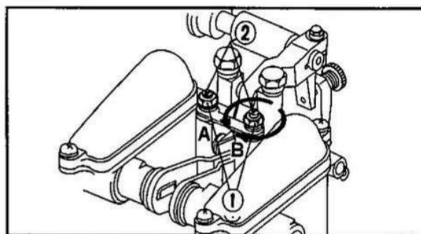
Fig. 2-12 ① Controdado. ② Vite di registro.
