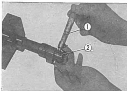
Fig. 3-122 ① Micrometro. ② Perno dell'asse a cammes.
