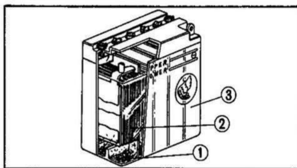
Fig. 5-32 ① Sedimento. ② Piastra. ③ Involucro della batteria.
