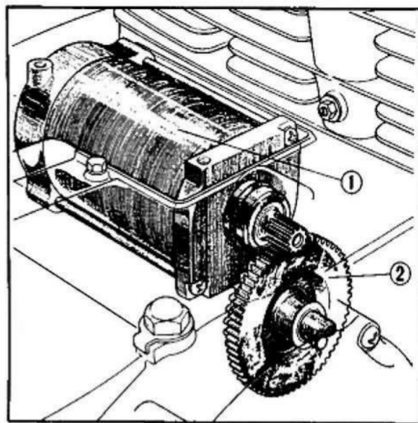
Fig. 5-55 Installazione del motorino di avviamento.
