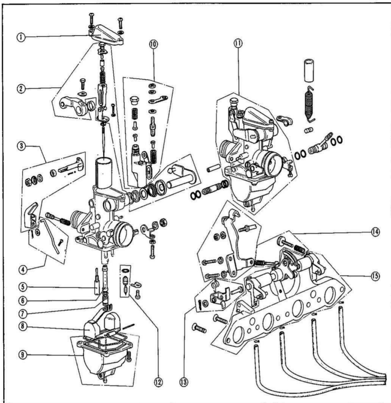
Fig. 3-43 ① Cappellotto. ② Gruppo braccetto di unione A. ③ " " di unione. ④ Astina dello starter. ⑤ Getto del minimo. ⑥ Portagetto del massimo. ⑦ Getto del massimo. ⑧ Galleggiante. ⑨ Gruppo vaschetta A. ⑩ Gruppo alloggiamento registro A. ⑪ Carburatore completo. ⑫ Gruppo valvolina della vaschetta. ⑬ Gruppo di unione. ⑭ Gruppo viti di registro B. ⑮ Piastra alloggiamento carburatore.
