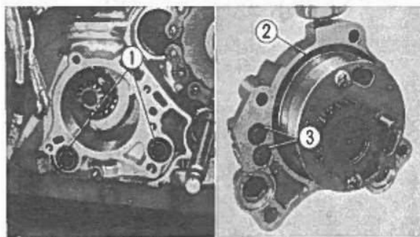
Fig. 3-12 ① Gommino 15×2,5 ② Gommino 63×2,5 ③ Gommino 9,9×1,5
