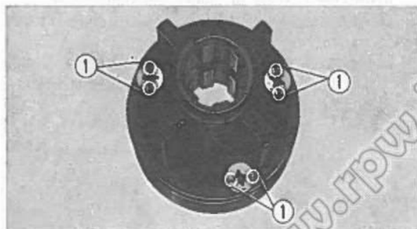
Fig. 3-28 ① Punzonatura.
