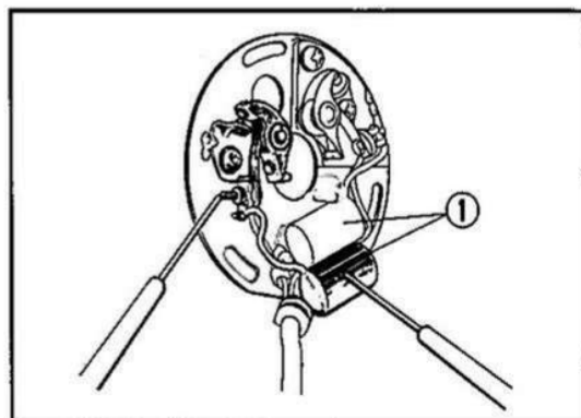
Fig. 5-42 ① Condensatore.
