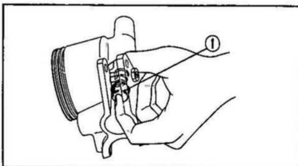
Fig. 4-11 ① Cappellotto.
