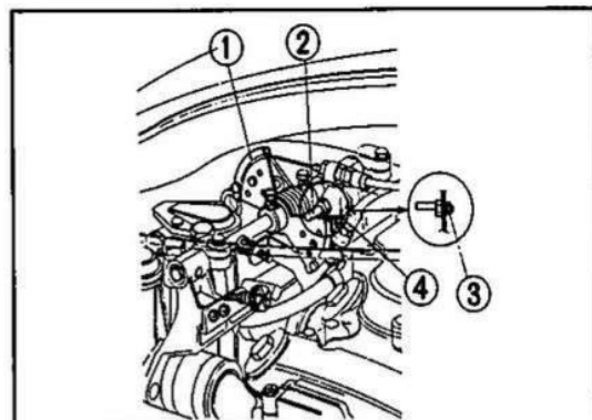
Fig. 2-25 ① Leva del gas. ③ Controdato. ② Pernetto eccentrico. ④ 2-3 mm.
