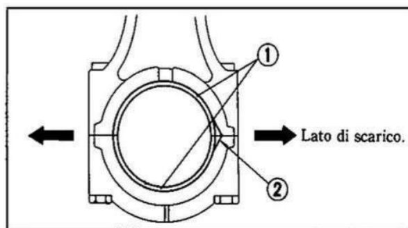
Fig. 3-38 ① Cuscinetto. ② Orecchietta di fermo.
