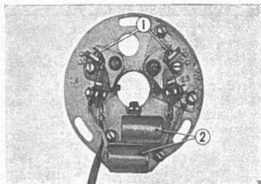
Fig. 5-72 ① Puntine platinat. ② Condensatore.
