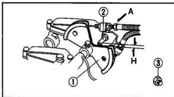
Fig. 2-15 ① Leva del gas. ② Pernetto del fermo. ③ Controdado.
