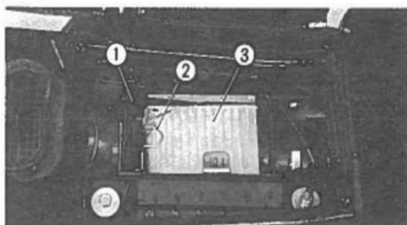
Fig. 2-61 ① Contenitore del filtro dell'aria. ② Molla di fissaggio. ③ Filtro dell'aria.
