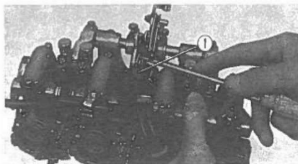
Fig. 3-44 ① Molletta di ritorno della valvola del gas.
