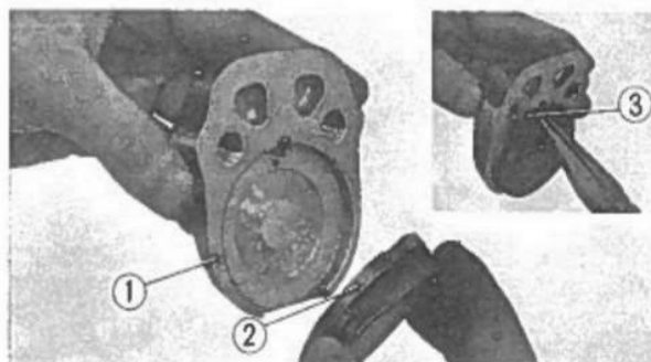
Fig. 4-3 ① Pinza B. ② Pasticca B. ③ Coppiglia.
