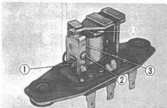
Fig. 5-54 (A) Apertura del nucleo. (B) Apertura delle puntine. ① Vite registro apertura nucleo. ② Vite registro apertura puntine. ③ Contatto inferiore.
