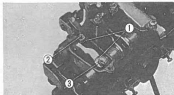
Fig. 3-47 ① Rondella di sicurezza. ② Bullone da 4 mm. ③ Bullone da 6 mm.
