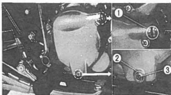
Fig. 2-35 ① Segno di riferimento. ② Controdado. ③ Registro della frizione.
