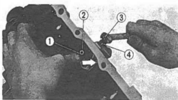
Fig. 3-32 ① Astina di spinta. ② Segno di riferimento. ③ Bullone di registro del tendicatena. ④ Controdado.
