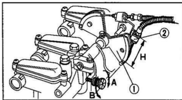
Fig. 2-11 ① Leva del Gas. ② Fermo della guaina del cavetto di comando.
