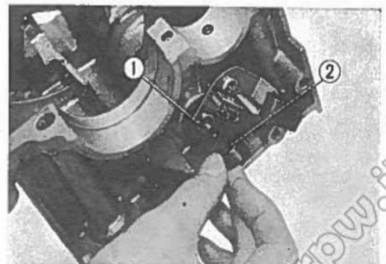
Fig. 3-84 ① Tamburo selettore. ② Spia del folle.
