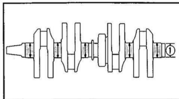
Fig. 3-35 ① Diametro esterno dei perni di banco.
