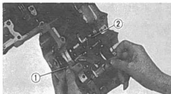
Fig. 3-24 ① Perno dei forcellini. ② Tamburo del selettore.
