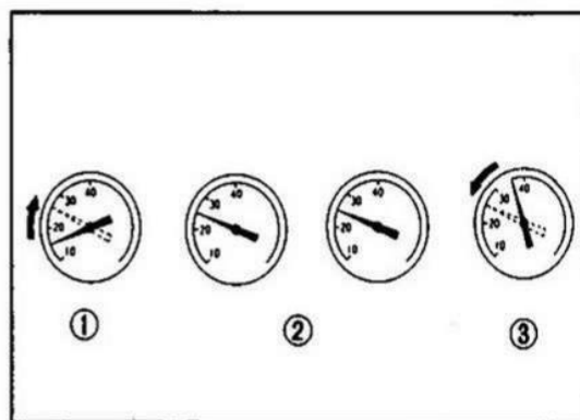
Fig. 2-22 ① Bassa depressione. ② Normale. ③ Alta depressione.
