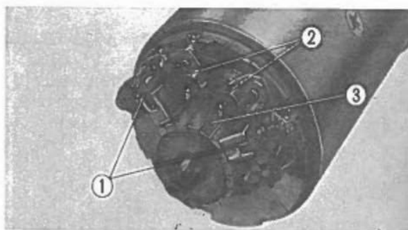
Fig. 5-25 ① Spazzole. ② Molle. ③ Commutatore.
