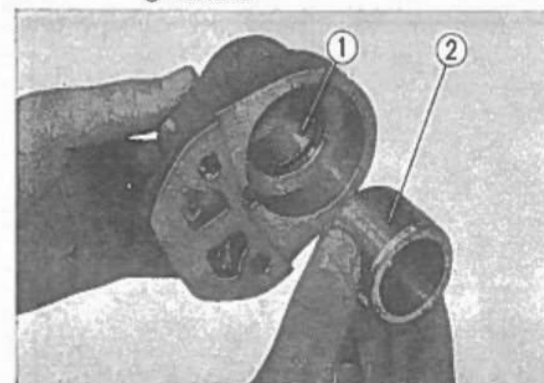
Fig. 4-27 ① Pinza A. ② Pistone.
