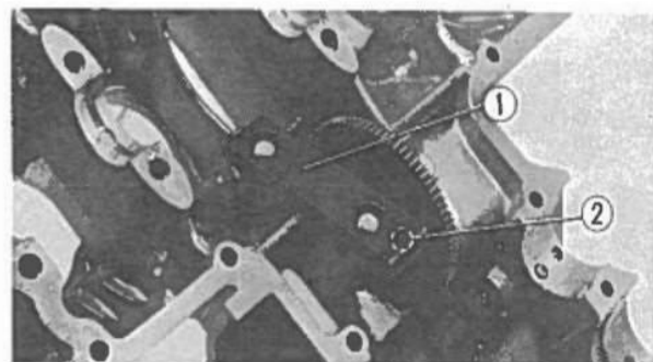
Fig. 3-41 ① Guida della catena primaria. ② Segno di riferimento.
