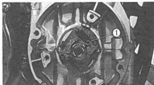
Fig. 5-9 ① Anticipo Automatico.
