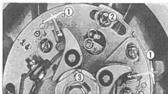
Fig. 5-7 ① Puntine. ② Segno fisso di riferimento. ③ Segno "F".
