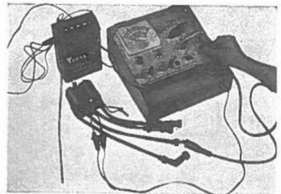
Fig. 5-38 Prova del funzionamento della bobina.
