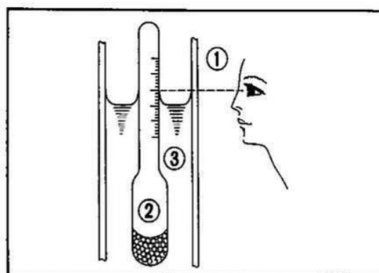
Fig. 5-63 ① Livello dell'occhio. ② Densimetro. ③ Elettrolito.
