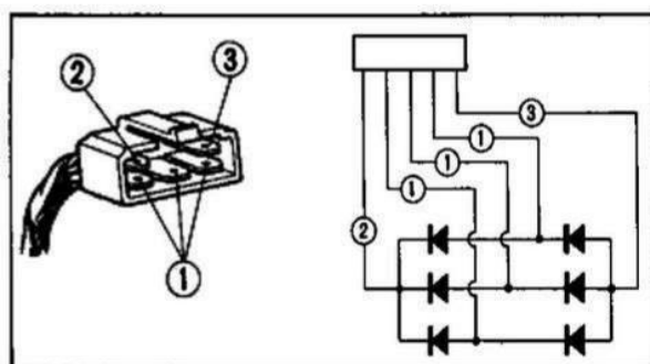
Fig. 5-17 ① Cavetti gialli. ③ Cavetto verde. ② Cavetto rosso/bianco.
