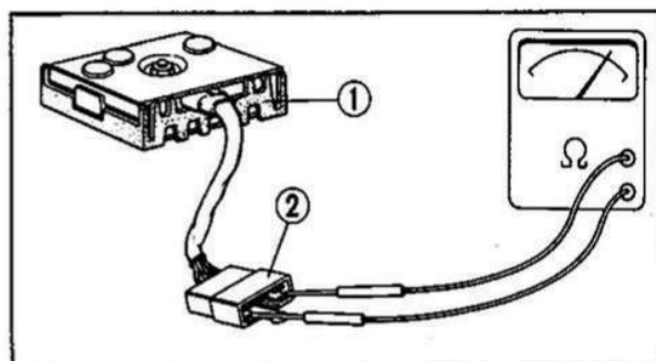
Fig. 5-16 ① Raddrizzatore al silicio. ② Scatola di collegamento.
