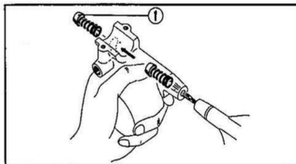
Fig. 4-7 ① Cappellotto.
