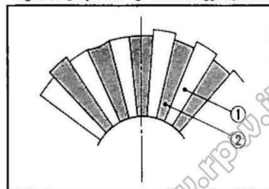
Fig. 5-89 ① Commutatore. ② Mica.
