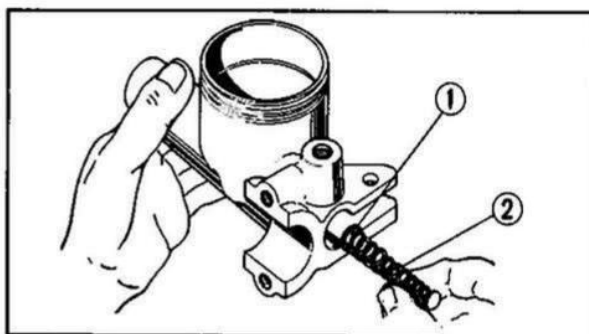
Fig. 4-10 ① Valvola di controllo. ② Molla di ritorno.
