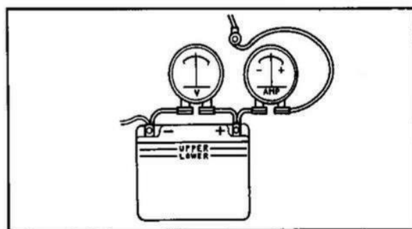
Fig. 5-11 Controllo della produzione di corrente.
