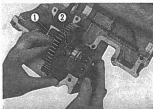
Fig. 3-143 ① Guida dell'olio. ② Complesso dell'alberino del pignone finale.
