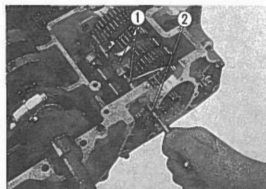
Fig. 3-144 ① Forchetta del cambio. ② Perno delle forchette.
