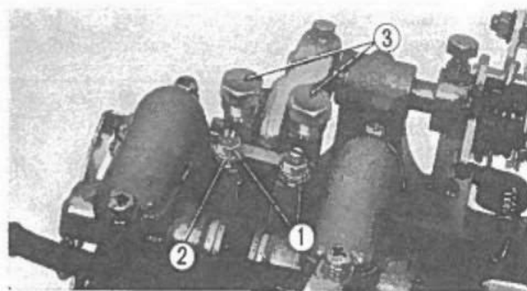
Fig. 3-45 ① Dadi esagonali. ② Piastrina parapolvere B. ③ Dadi a cappellotto.
