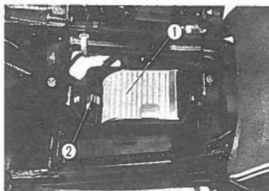
Fig. 2-62 ① Filtro aria. ② Molla di fermo.
