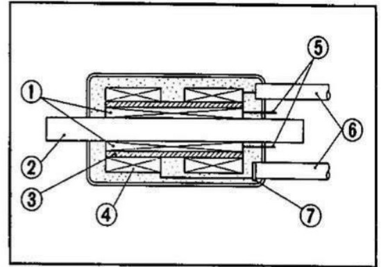
Fig. 5-36 ① Avvolgimento primario. ② Nucleo di ferro. ③ Rocchetto. ④ Avvolgimento secondario. ⑤ Terminali primario. ⑥ Cavetti ad alta tensione. ⑦ Terminali del secondario.
