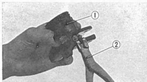
Fig. 4-6 ① Cilindro principale. ② Pinze per l'anello elastico (Seeger).
