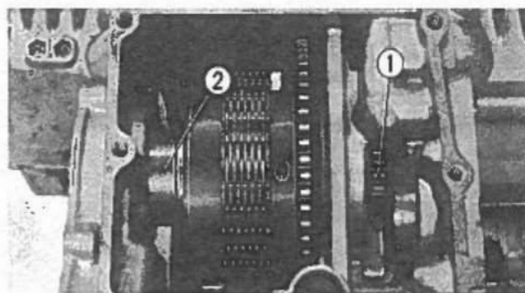
Fig. 3-29 ① Contralbero. ② Distanziale da 25 mm.
