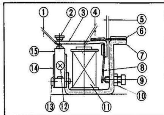
Fig. 5-81 ① Apertura puntine. ② Contatto inferiore. ③ Armatura. ④ Apertura del nucleo. ⑤ " della intelaiatura. ⑥ Molla. ⑦ Intelaiatura. ⑧ Molla di registrazione. ⑨ Vite regolazione voltaggio. ⑩ Controdado. ⑪ Avvolgimento. ⑫ Vite regolazione apertura puntine. ⑬ Vite regolazione apertura nucleo. ⑭ Gruppo di contatto. ⑮ Contatto superiore.
