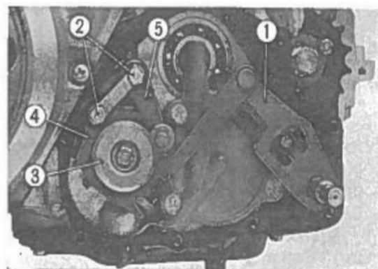
Fig. 3-140 ① Leva di comando del selettore. ② Bulloni da 6 mm. ③ Piastrina laterale del selettore. ④ Braccetto di fermo del tamburo selettore. ⑤ Piastrina del preselettore.
