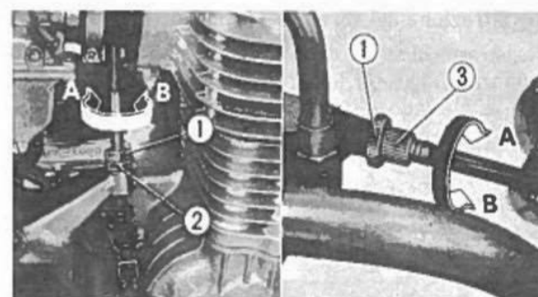
Fig. 2-37 ① Controdado. ② Registro inferiore del cavetto della frizione. ③ Registro superiore del cavetto della frizione.
