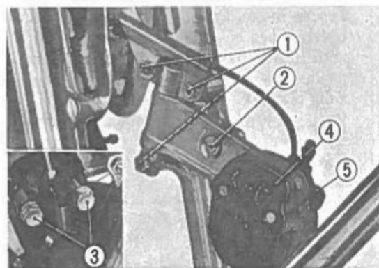
Fig. 4-15 ① Bulloni di montaggio della pinza. ② Bullone di registro. ③ Bulloni di unione della pinza. ④ Pinza B. ⑤ Pinza A.
