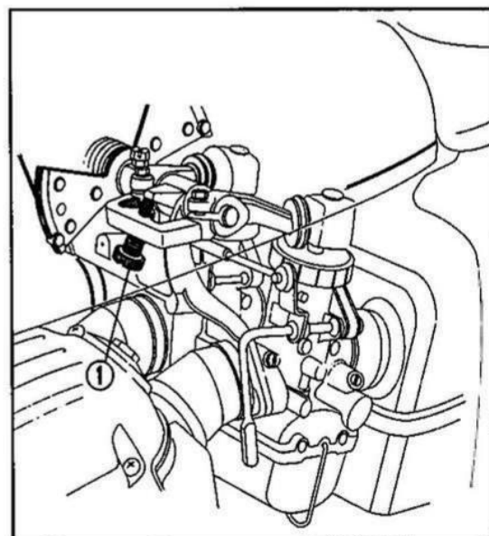
Fig. 2-27 Regolazione del minimo. ① vite di registro del minimo.
