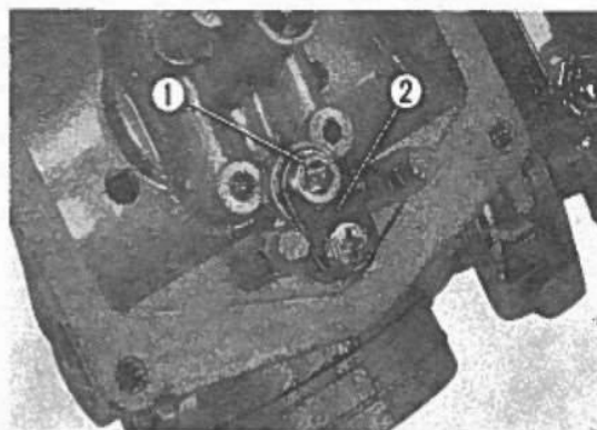
Fig. 3-116 ① Sede della valvola a spillo. ② Piastrina di fermo.
