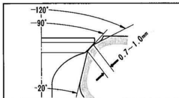
Fig. 3-2 Contatto della sede valvola.
