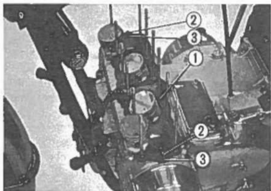
Fig. 3-65 ① Guarnizione base cilindri. ② Boccolette speciali di centraggio. ③ Gommini.
