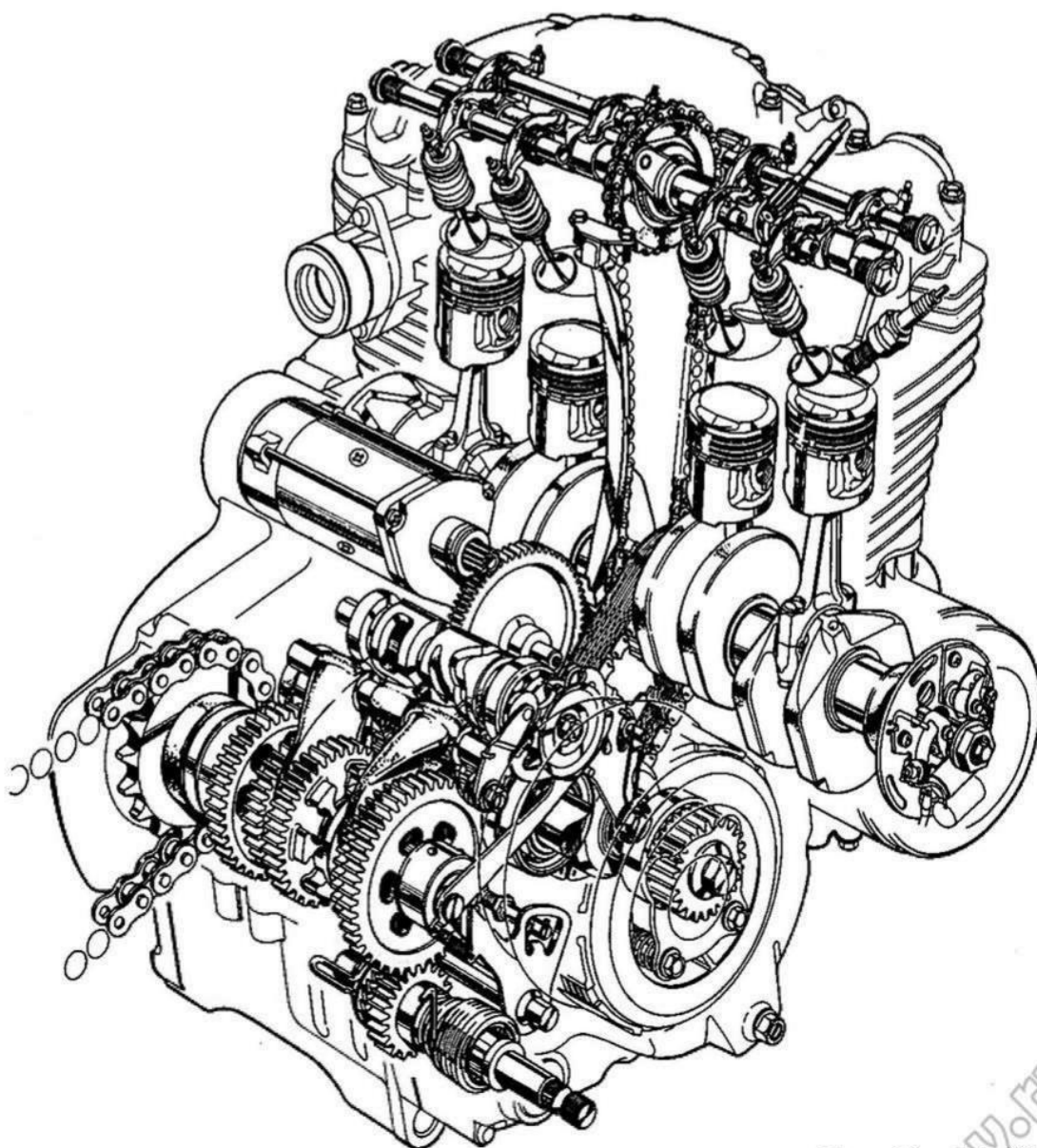
Motore del modello CB 350 F
