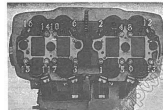
Fig. 3-128 Ordine di serraggio dei dadi della testa.
