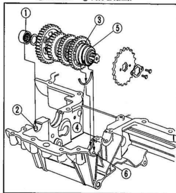
Fig. 3-27 ① Cuscinetto ad aghi da 20 mm. ② Spina di fermo da 6 mm. ③ Cuscinetto a sfera 5205. ④ Semianello di fermo del cuscinetto, da 50 mm. ⑤ Paraolio. ⑥ Foro di fermo.
