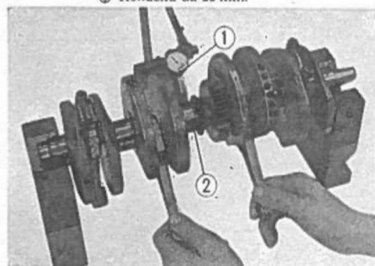
Fig. 3-91 ① Comparatore. ② Albero motore.
