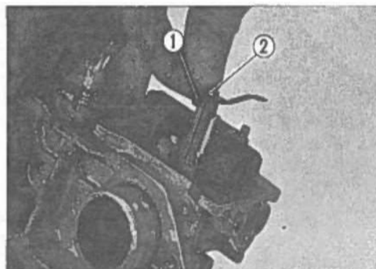
Fig. 3-114 ① Molla a lamella. ② Getto del massimo.
