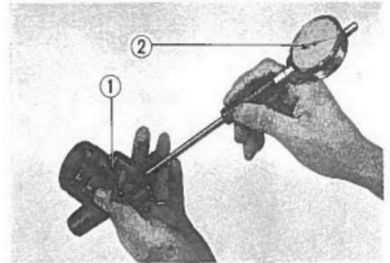
Fig. 4-21 ① Cilindro principale. ② Alesametro.
