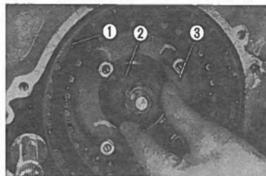
Fig. 3-136 ① Campana frizione. ② Rondella scanalata da 25 mm. ③ Piastra di pressione della frizione.
