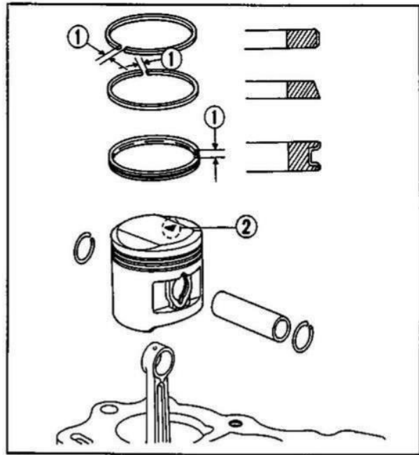
Fig. 3-4 ① Apertura del segmento. ② Segno sul pistone.
