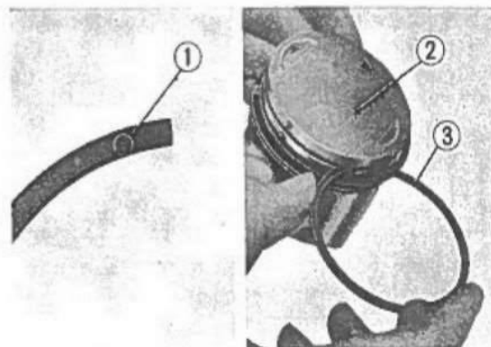
Fig. 3-62 ① Lettera stampigliata.
