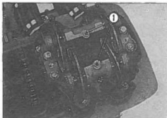
Fig. 3-132 ① Bulloni di fissaggio dei perni dei bilancieri.
