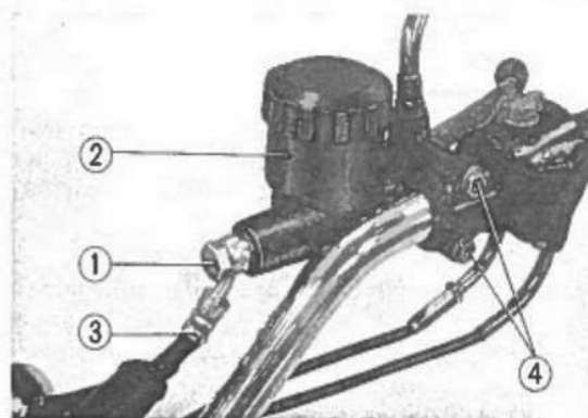
Fig. 4-17 ① Bullone di attacco. ② Complesso del cilindro principale. ③ Cavetto del liquido del freno. ④ Attacco al manubrio.
