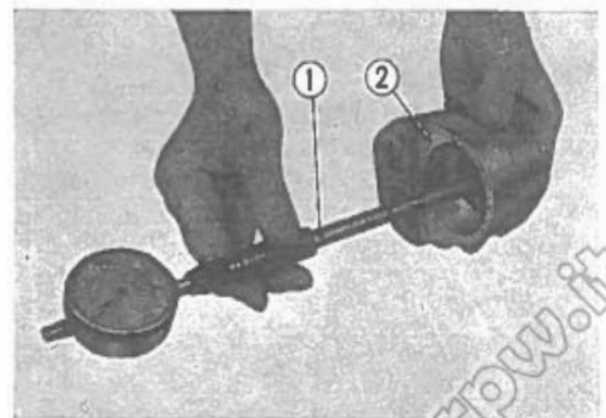
Fig. 4-31 ① Alesametro. ② Cilindro della pinza del freno.
