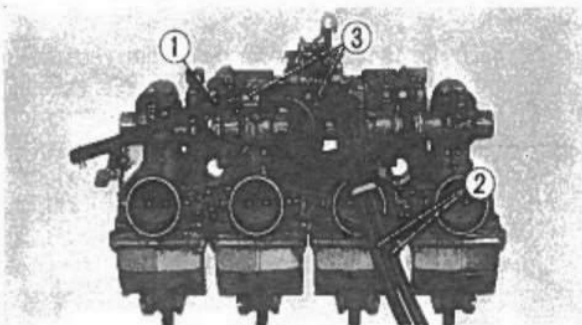
Fig. 3-58 ① Cavo benzina. ② Cavo benzina (3,5×600) ③ Fascette di fissaggio.
