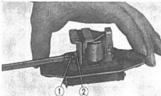
Fig. 5-53 ① Vite registrazione voltaggio. ② Controdado.
