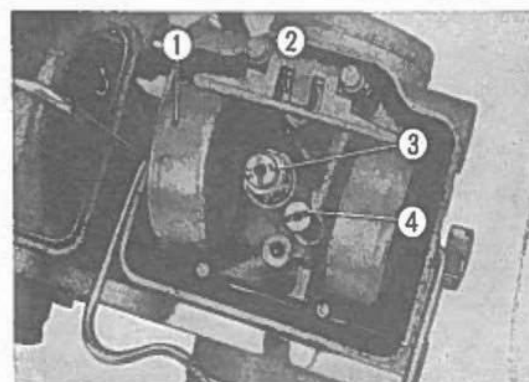
Fig. 3-162 ① Galleggiante. ② Gruppo valvolina a spillo. ③ Getto del massimo. ④ Getto del minimo.
