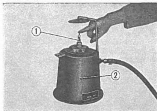
Fig. 5-40 ① Candela. ② Apparecchio per la pulizia delle candele.
