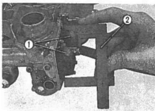
Fig. 3-117 ① Galleggiante. ② Misuratore di livello.
