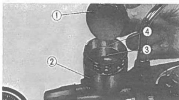
Fig. 4-12 ① Diaframma. ③ Liquido dei freni. ② Cilindro principale. ④ Linea di livello.
