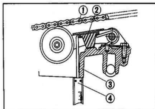
Fig. 3-148 ① Catena primaria. ② Tendicatena. ③ Carter inferiore. ④ Calibro.
