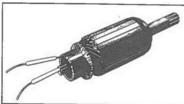
Fig. 5-27 Controllo della continuità dell'avvolgimento dell'armatura.
