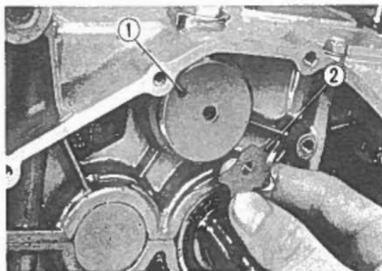
Fig. 3-85 ① Spina. ② Piastrina terminale del tamburo selettore.
