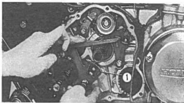
Fig. 3-18 ① Perno di comando del cambio.
