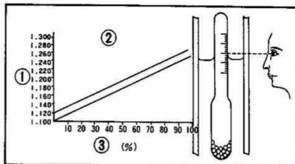
Fig. 5-31 ① Densità. ② Relazione tra densità e carica residua. ③ Carica residua.
