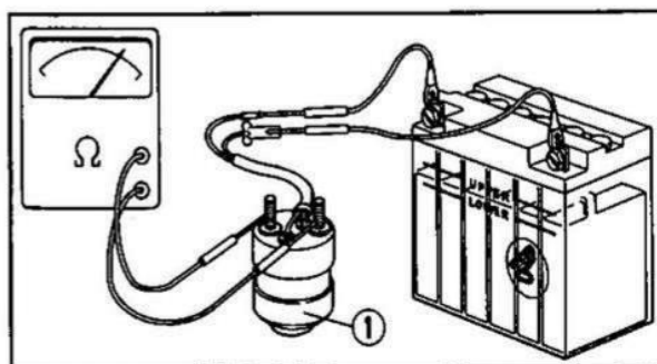
Fig. 5-92 ① Interruttore magnetico di avviamento.
