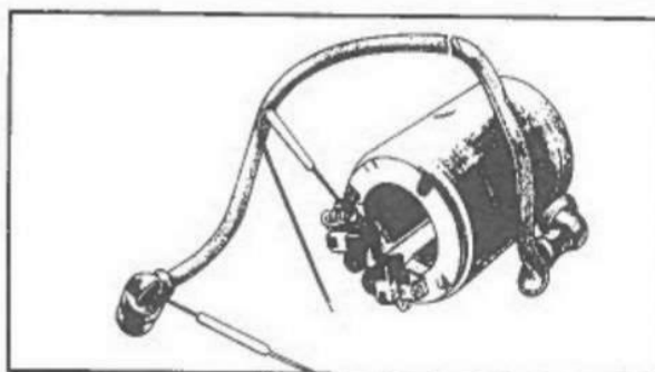
Fig. 5-26 Controllo della continuità dell'avvolgimento di campo.
