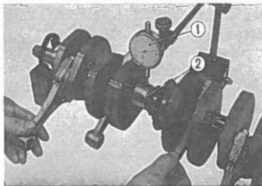
Fig. 3-150 ① Comparatore. ② Albero motore.
