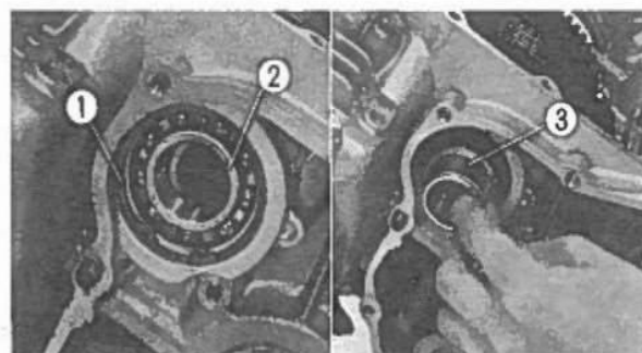
Fig. 3-22 ① Anello interno di fermo da 52 mm. ② Cuscinetto a sfera 6205. ③ Distanziale da 25 mm.
