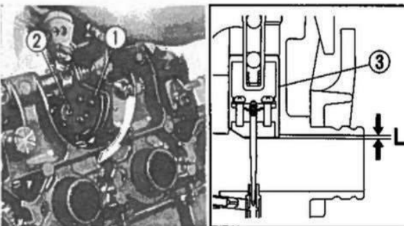
Fig. 3-59 ① Leva della valvola del gas. ② Vite di registro. ③ Valvola del gas.
