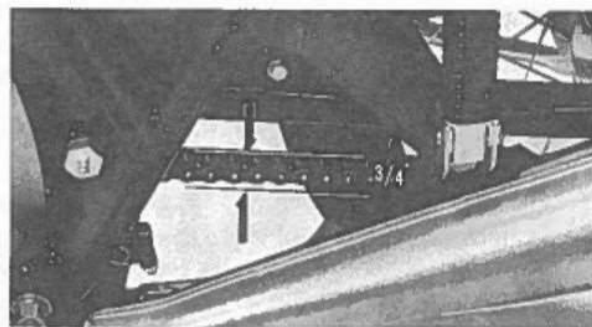
Fig. 2-64 Controllo dell'allentamento della catena.
