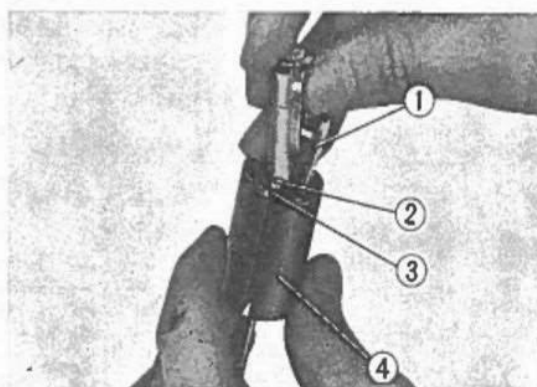
Fig. 3-118 ① Piastrina della valvola. ② Vite da 3 mm. ③ Rondella elastica. ④ Valvola del gas.
