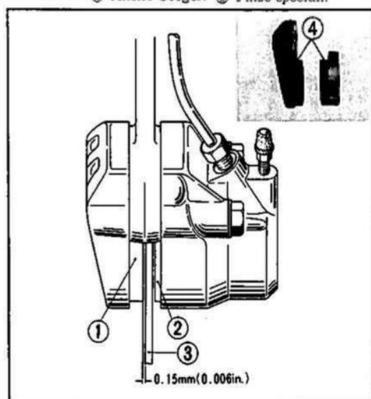
Fig. 4-19 ① Pasticca B. ③ Disco. ② Pasticca A. ④ Indicatore del limite di usura.
