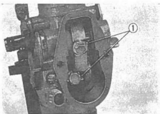
Fig. 3-108 ① Rondella di sicurezza.
