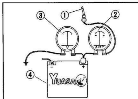
Fig. 5-45, ① Cavetto rosso/bianco. ③ Voltmetro. ② Amperometro. ④ Batteria.
