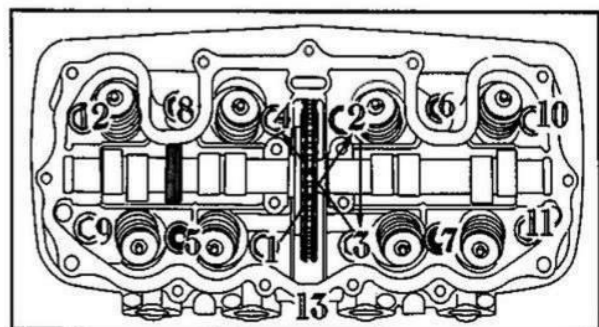
Fig. 3-6 Ordine di serraggio dei dadi della testa.
