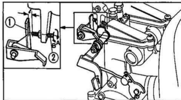
Fig. 2-13 ① Piastrina di fissaggio. ② Vite di registro.
