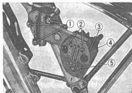
Fig. 4-26 ① Bulloni di fissaggio della pinza. ② Bulloni a brugola. ③ Pinza. ④ Parte A. ⑤ Parte B.
