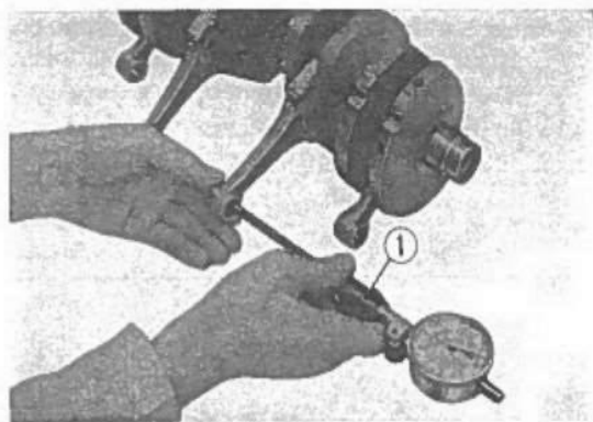
Fig. 3-100 ① Alesametro.
