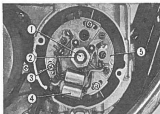
Fig. 5-41 ① Bullone da 6 mm. ② Rondella speciale. ③ Viti. ④ Condensatori. ⑤ Piatto delle puntine.
