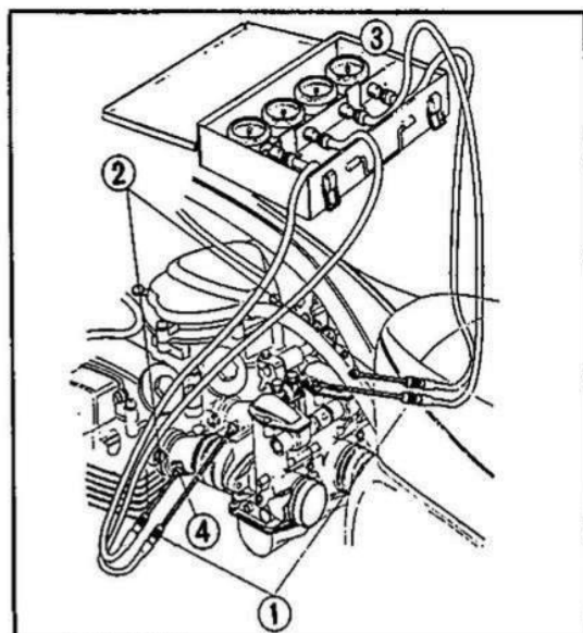
Fig. 2-19 ① Tubicino di raccordo "A". ② Tubicino di raccordo "B". ③ Vacuometro. ④ Foro di attacco.
