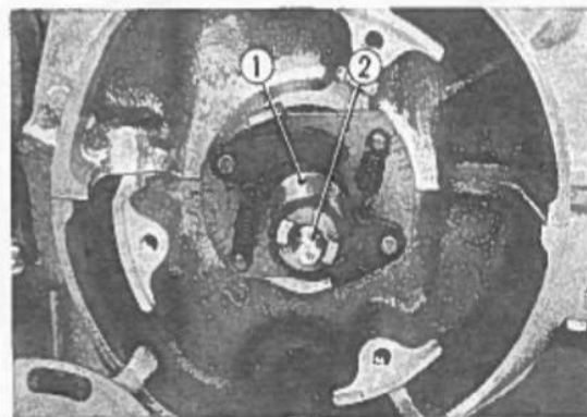
Fig. 5-74. ① Anticipo di accensione. ② Alberino dell'anticipo di accensione.
