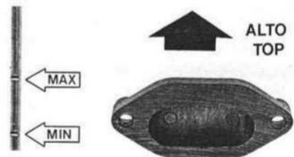
Fig. 8 Tacche livello olio - Dipstick marks Verso di montaggio coperchio filtro Oil filter cover should be fitted this way round
