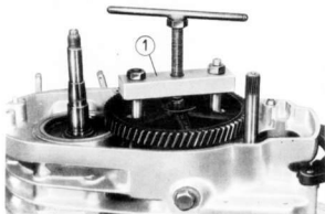
Slika 16. Skidanje pogonskog zupčanika
