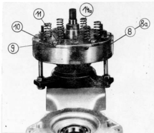
Slika 19a. Montaža spojke - 2. faza
