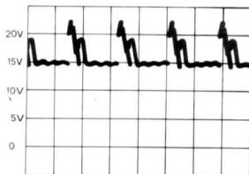
Slika 142. Prekid u pozitivnoj diodi
