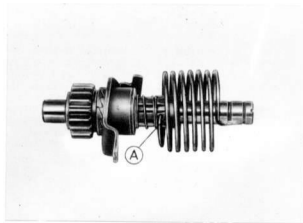
Slika 81. Kompletno vratilo pokretača
