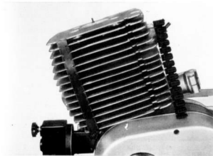
Slika 74. Montirati prigušne češlje Zatim utisnuti četiri prigušna češlja (D) u cilindar i poklopac cilindra.
