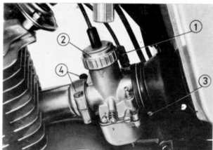
Slika 10. Vадjenje karburatora
