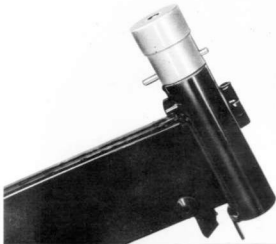
Slika 102. Namestiti gornji deo izvlačača
