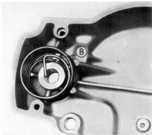
Slika 82. Položaj ugradjivanja opruge spojke
