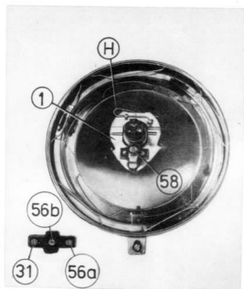
Slika 172. Prednji deo fara sa držačem sijalica
