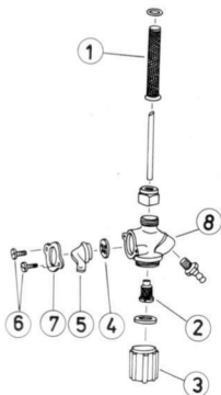
Slika 116. Filterska slavina za gorivo rastavljena
