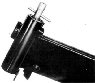
Slika 101. Unutrašnji deo izvlačaka utisnuti u kuglični ležaj
