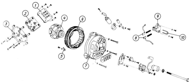
Slika 156. Eksplozivni prikaz alternatora
