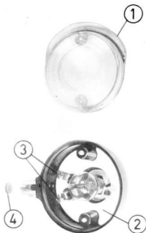
Slika 182. Prednji žmigavac
