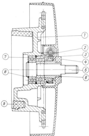
Slika 118. Pogon zadnjeg točka
