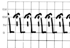
Slika 144. Kratak spoj u pobudnoj diodi
