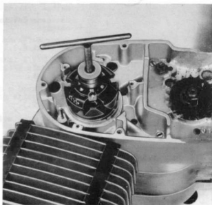
Slika 154. Vajdenje rotora
