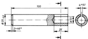
Slika 158. Štap za prešanje okrugli čelik 22 TGL 11 163 St 50 K TGL O-1652
