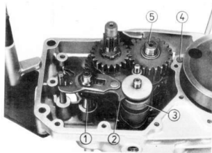
Slika 64. Završena montaža menjača i radilice
