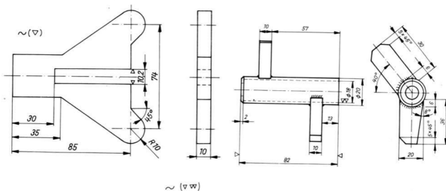
Slika 1c. Priklešni deo, prednji, kompl. 89-99.322
