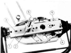
Slika 17. Izvoditi aretiranje komande menjača i uskočnike
