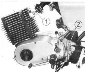
Slika 12. Vадjenje motora ili zamena cilindra
