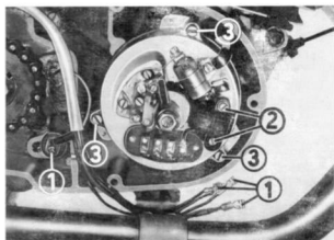
Slika 8. Vadjenje statora iz alternatora
