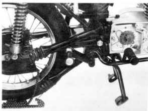
Slika 129. Nameštanje lanca - 2. etapa
