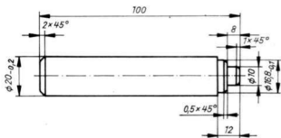
Slika 157. Trn za izbacivanje okrugli čelik 22 TGL 11 163 St 50 K TGL O-1652
