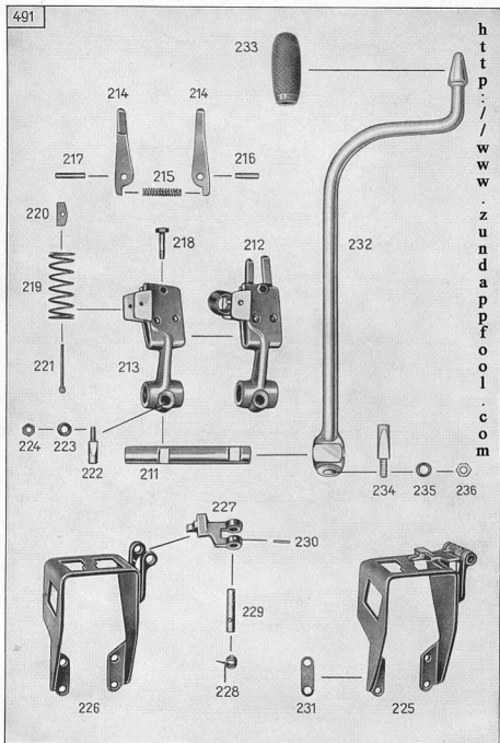
Tafel 10, Gruppe G: d) Fußschaltung
