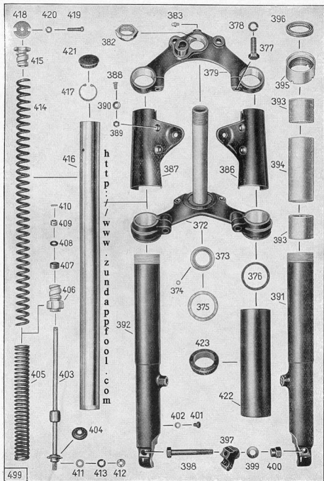
Tafel 20, Gruppe R: i) Federgabel, Zusammenbau Federgabelaufhängung
