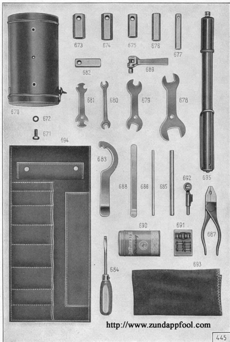
Tafel 29, Gruppe W: a) Werkzeug
