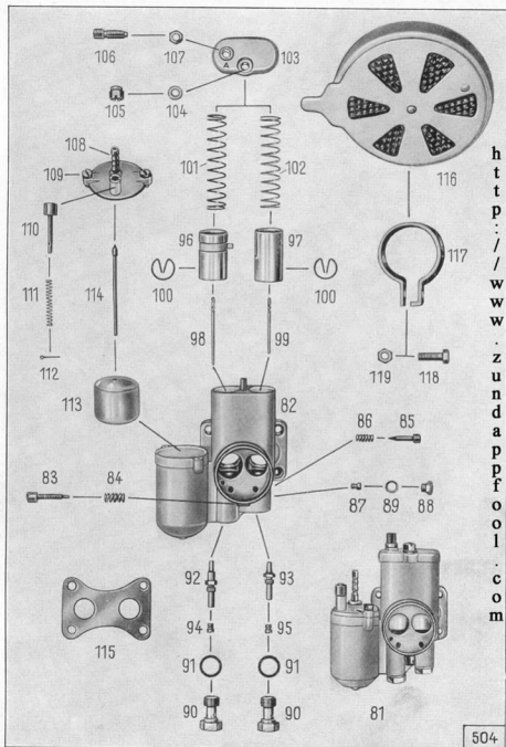
Tafel 6, Gruppe M: f) Vergaser und Filter
