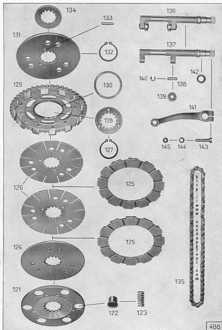
Tafel 7, Gruppe M: g) Kupplung, Kupplung, Kupplungsbetätigung
