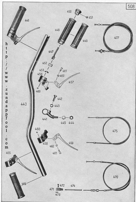
Tafel 22, Gruppe R: k) Lenker u. Handbetätigungen mit Seilzügen
