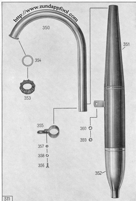
Tafel 19, Gruppe R: h) Auspuffanlage
