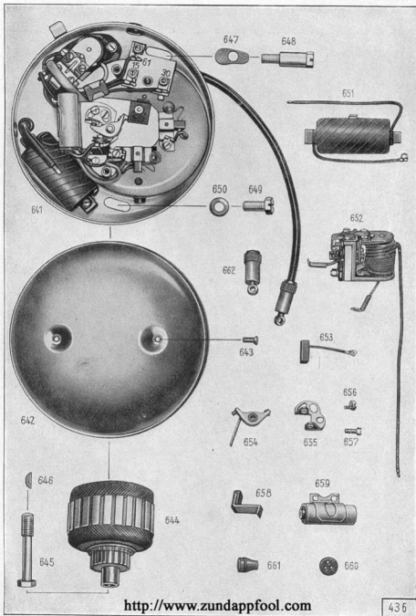
Tafel 28, Gruppe E: a) Elektrische Ausrüstung, Batterie-Lichtzünd-Anlage
