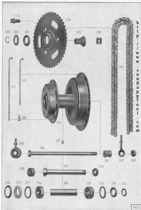
Tafel 26. Gruppe B: b) Räder, Hinterrad
