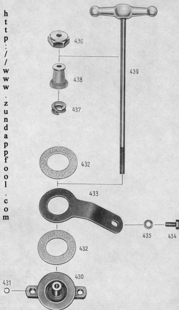
Tafel 21, Gruppe R: i) Federgabel, Steuerungsdämpfer
