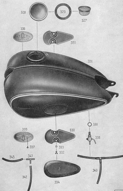
Tafel 18, Gruppe R: f) Kraftstoffbehälter und -leitungen
