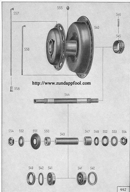
Tafel 25, Gruppe B: b) Räder, Vorderrad
