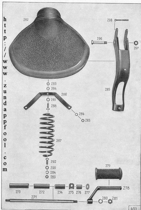
Tafel 14, Gruppe R: b) Fußraster und Sattel
