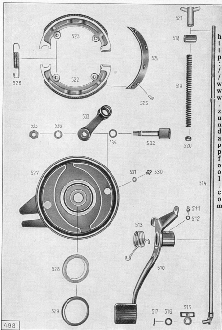
Tafel 24, Gruppe B: a) Bremsen, Fußbremse
