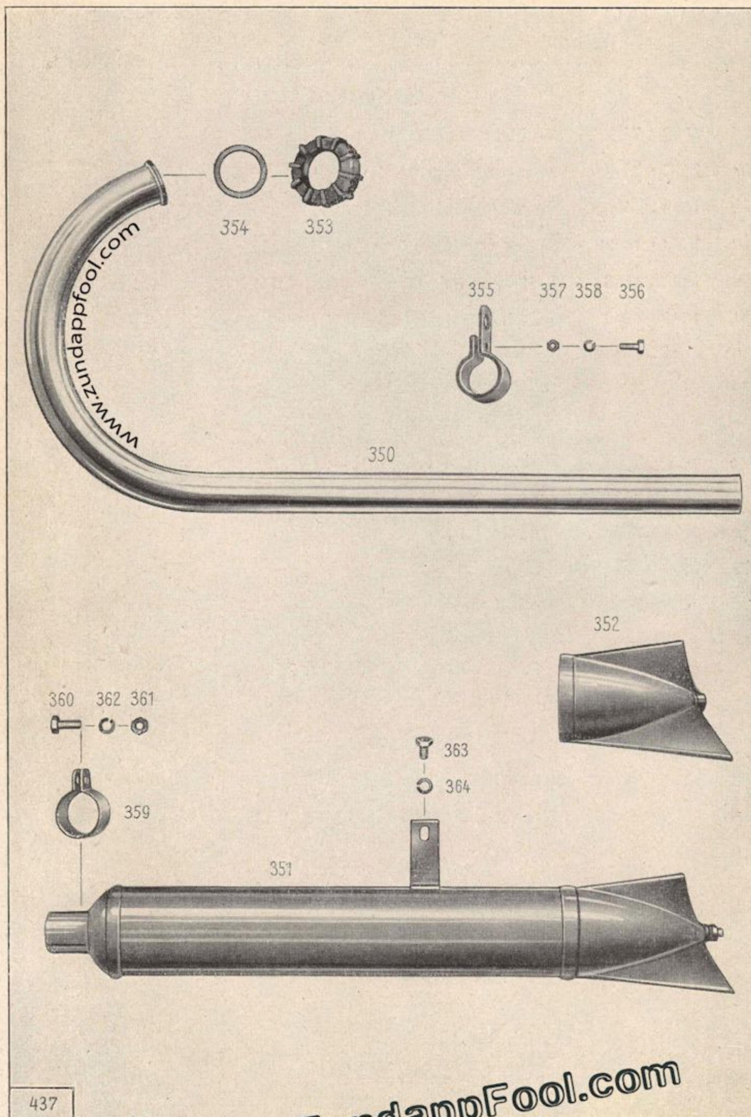
Tafel 17, Gruppe R: h) Auspuffanlage
