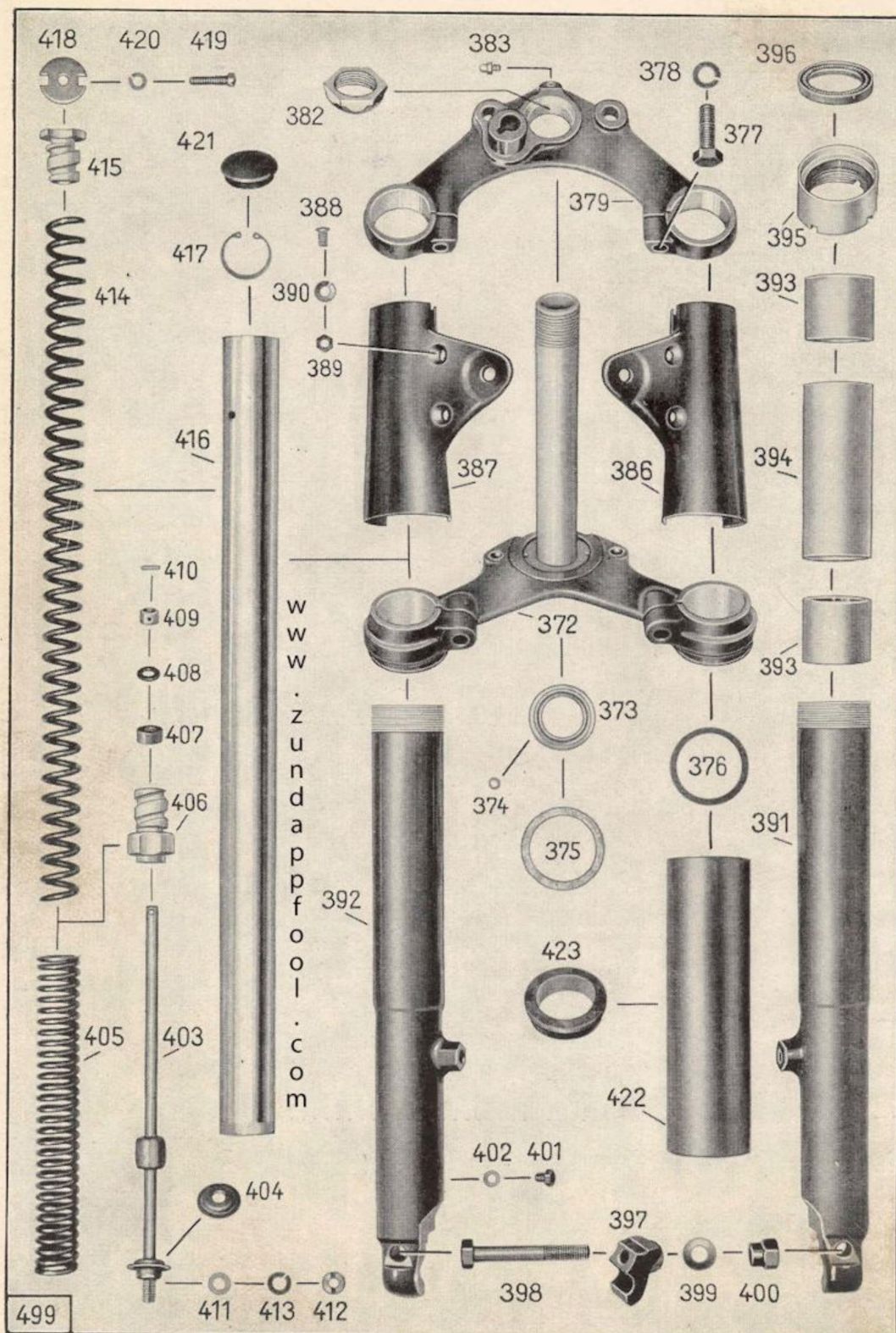
Tafel 18, Gruppe R: i) Federgabel, Zusammenbau Federgabelaufhängung
