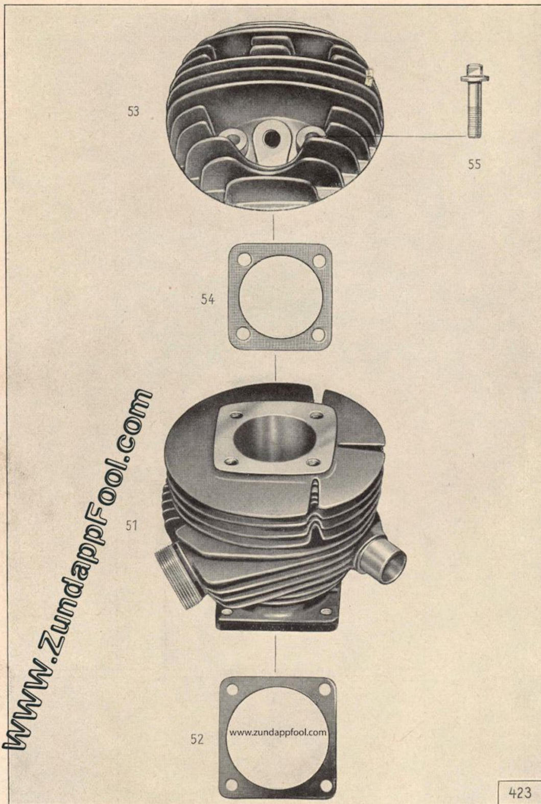
Tafel 4, Gruppe M: b) Gehäuse und Zylinder,
