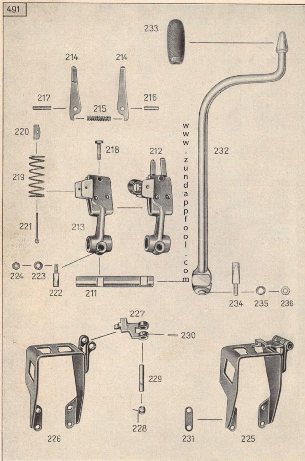
Tafel 10, Gruppe G: d) Fußschaltung
