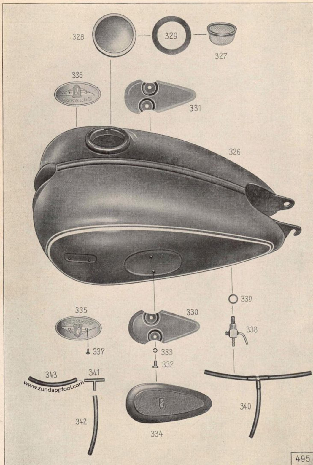
Tafel 16, Gruppe R: f) Kraftstoffbehälter und -leitungen
