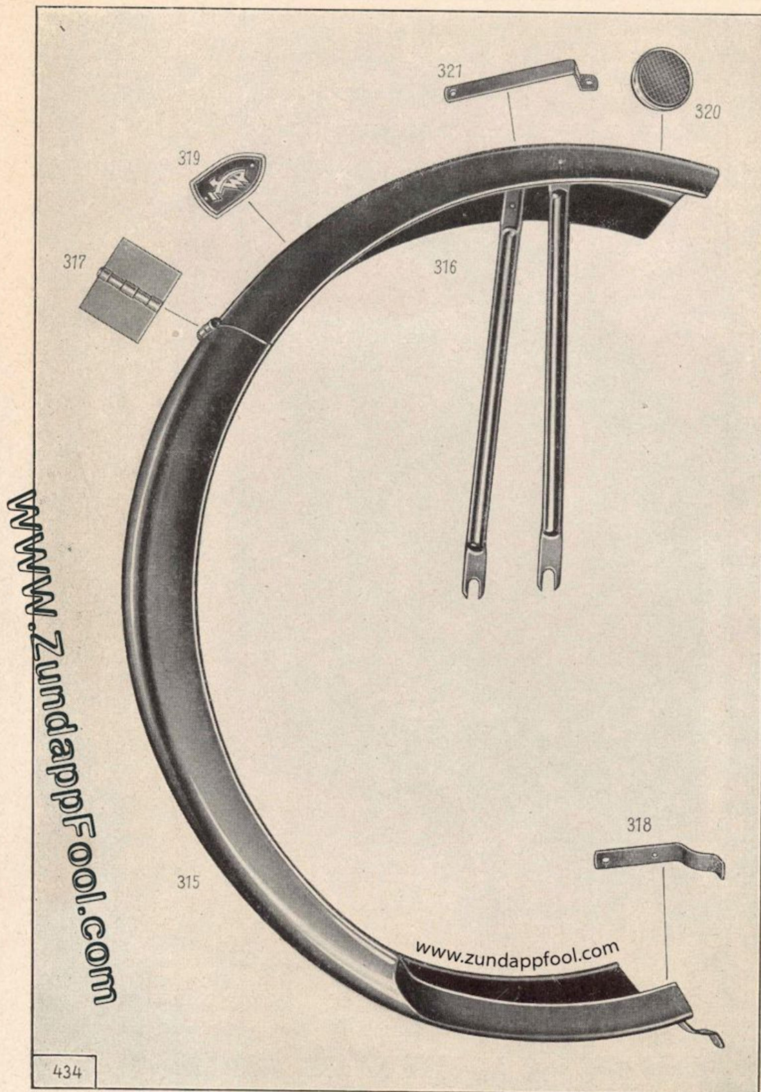
Tafel 15, Gruppe R: d) Schutzbleche, Hinterrad-Schutzblech
