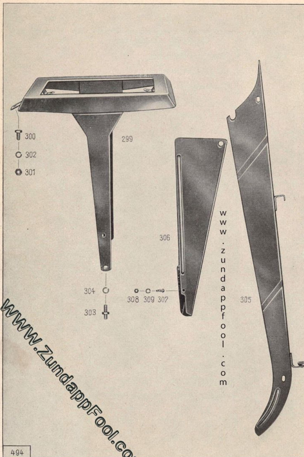
Tafel 13, Gruppe R: c) Gepäckträger und Kettenschutz
