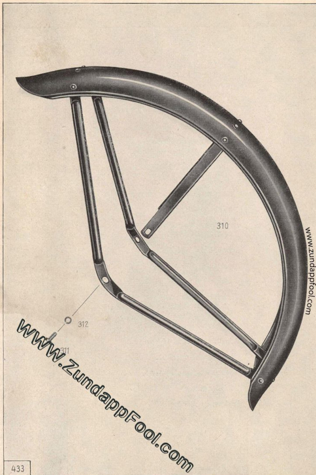
Tafel 14, Gruppe R: d) Schutzbleche, Vorderrad-Schutzblech
