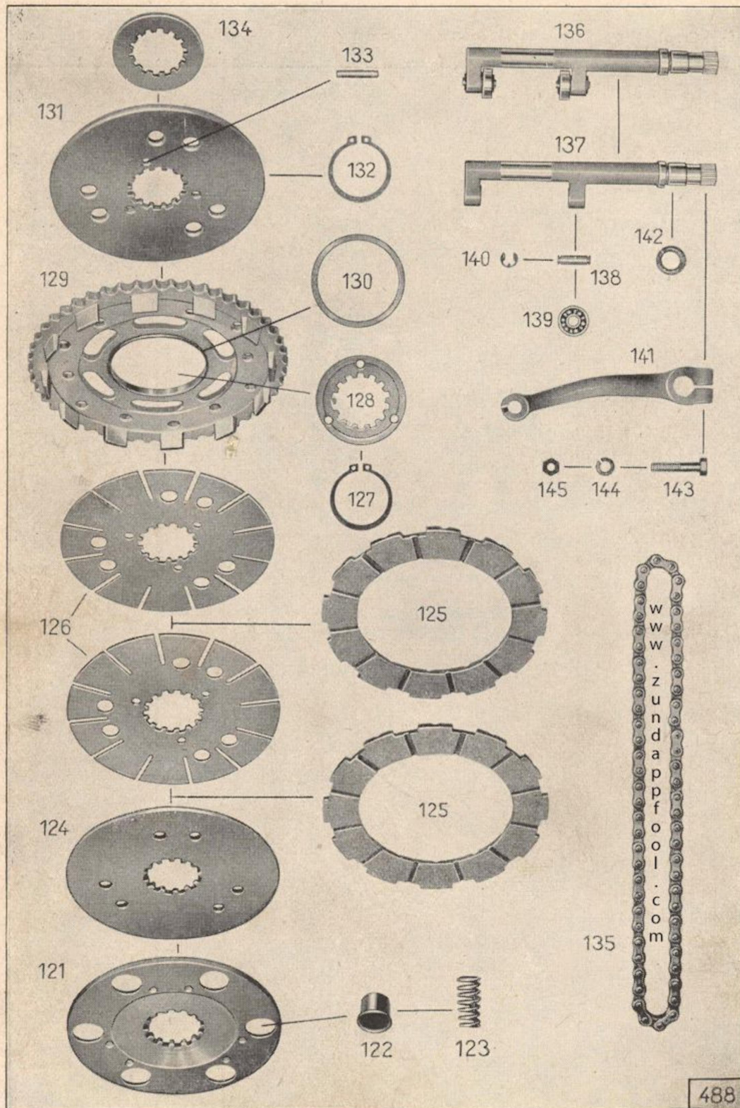
Tafel 7, Gruppe M: g) Kupplung Kupplung, Kupplungsbetätigung
