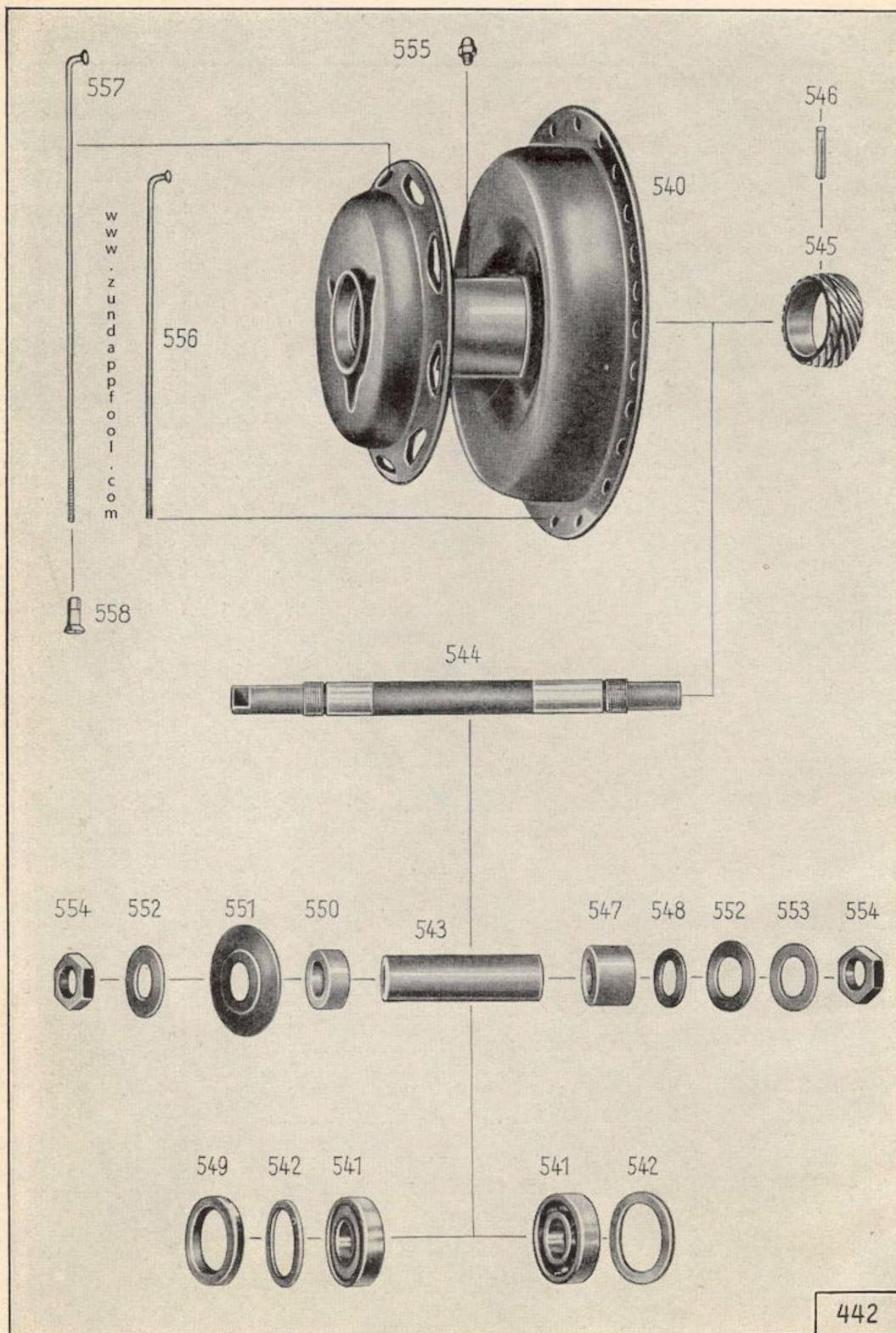
Tafel 23, Gruppe B: b) Räder, Vorderrad
