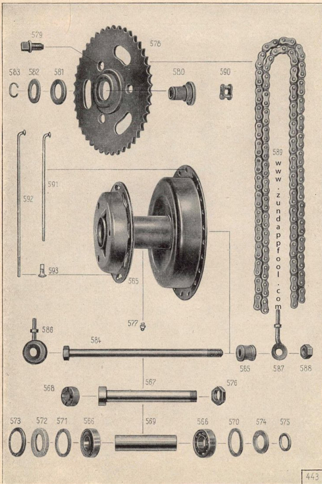
Tafel 24, Gruppe B: b) Räder, Hinterrad
