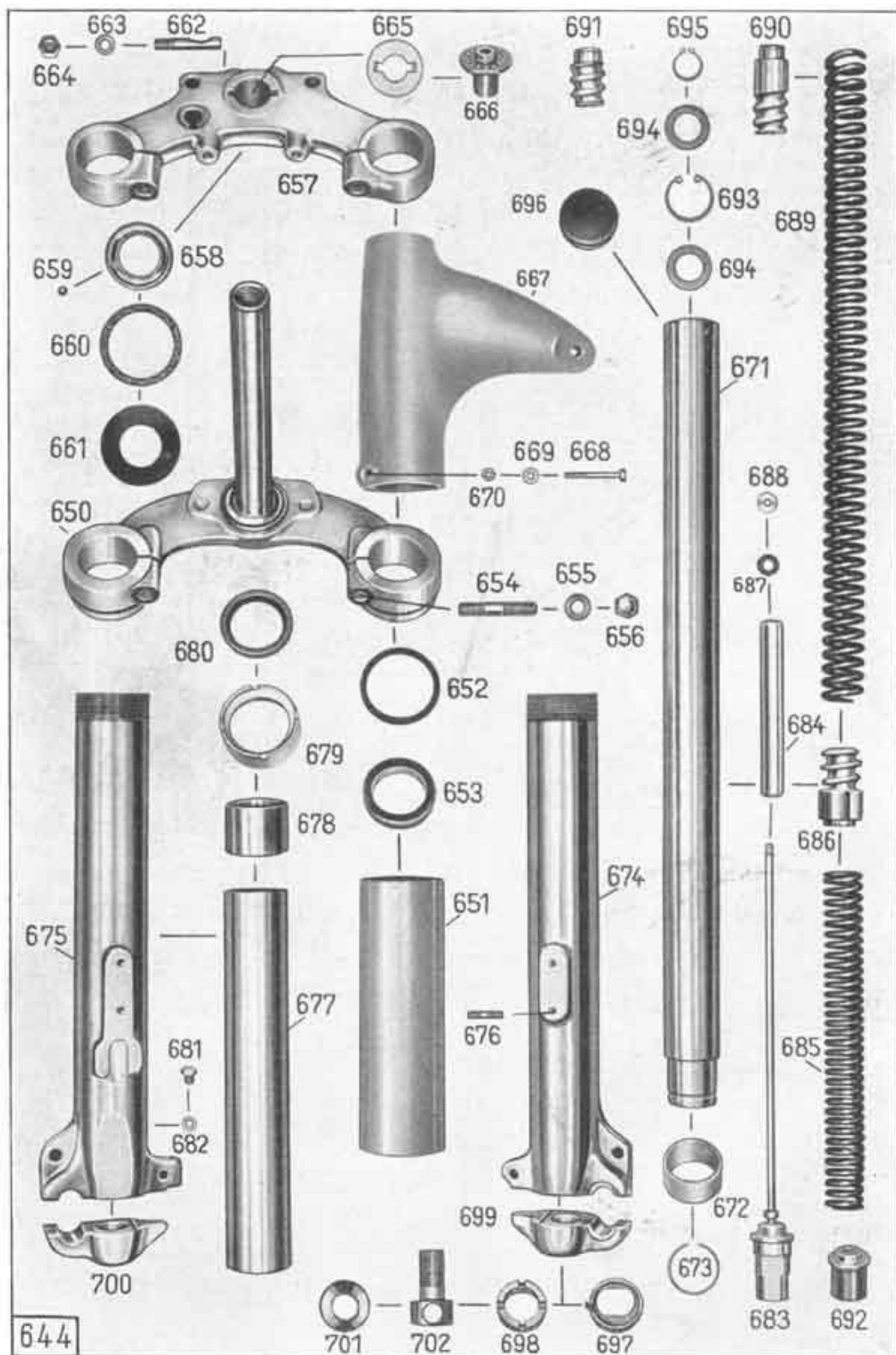
Tafel 25, Gruppe R: f) Vordergabel (Zusammenbau)
