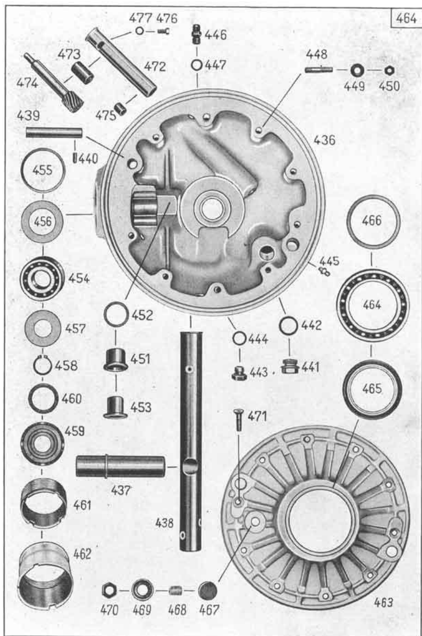
Tafel 16, Gruppe H: a) Hinterachsgetriebe (Zusammenbau)
