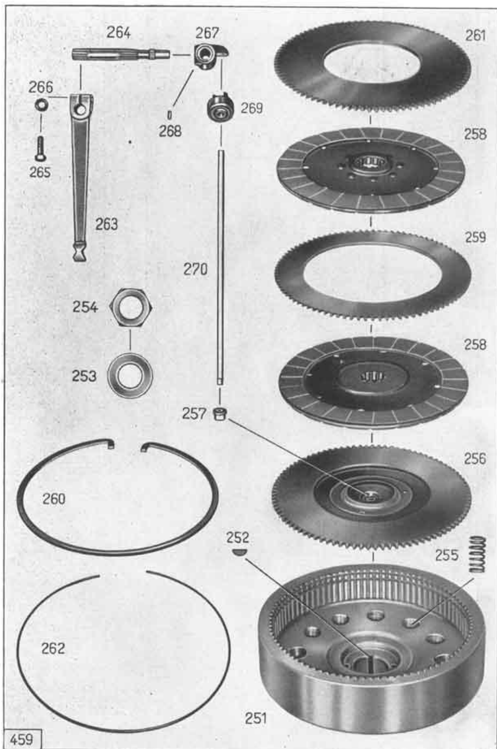
Tafel 11, Gruppe M: g) Kupplung, Kupplung, Kupplungsbetätigung
