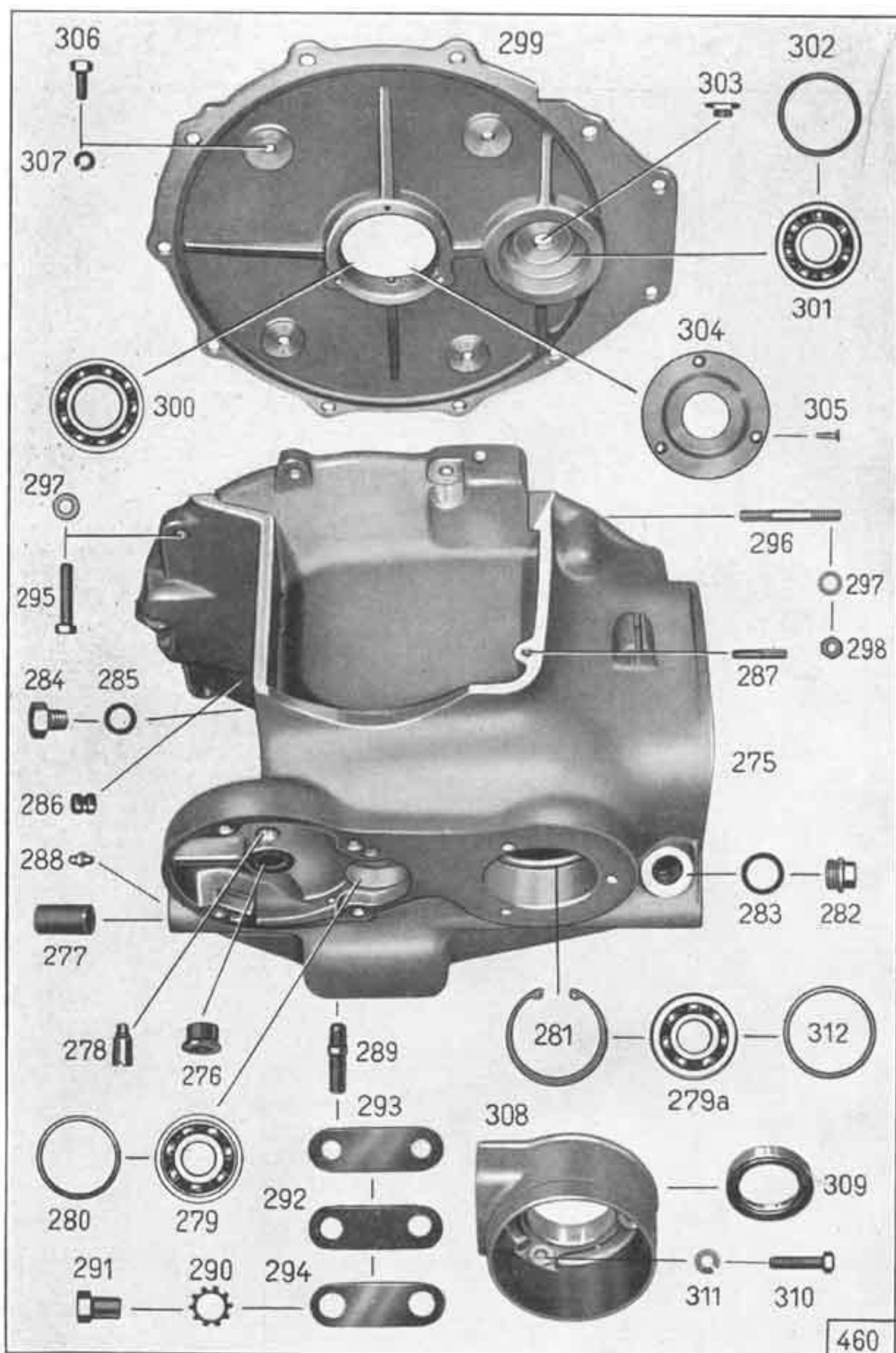
Tafel 12, Gruppe G: a) Wechselgetriebe, b) Getriebegehäuse
