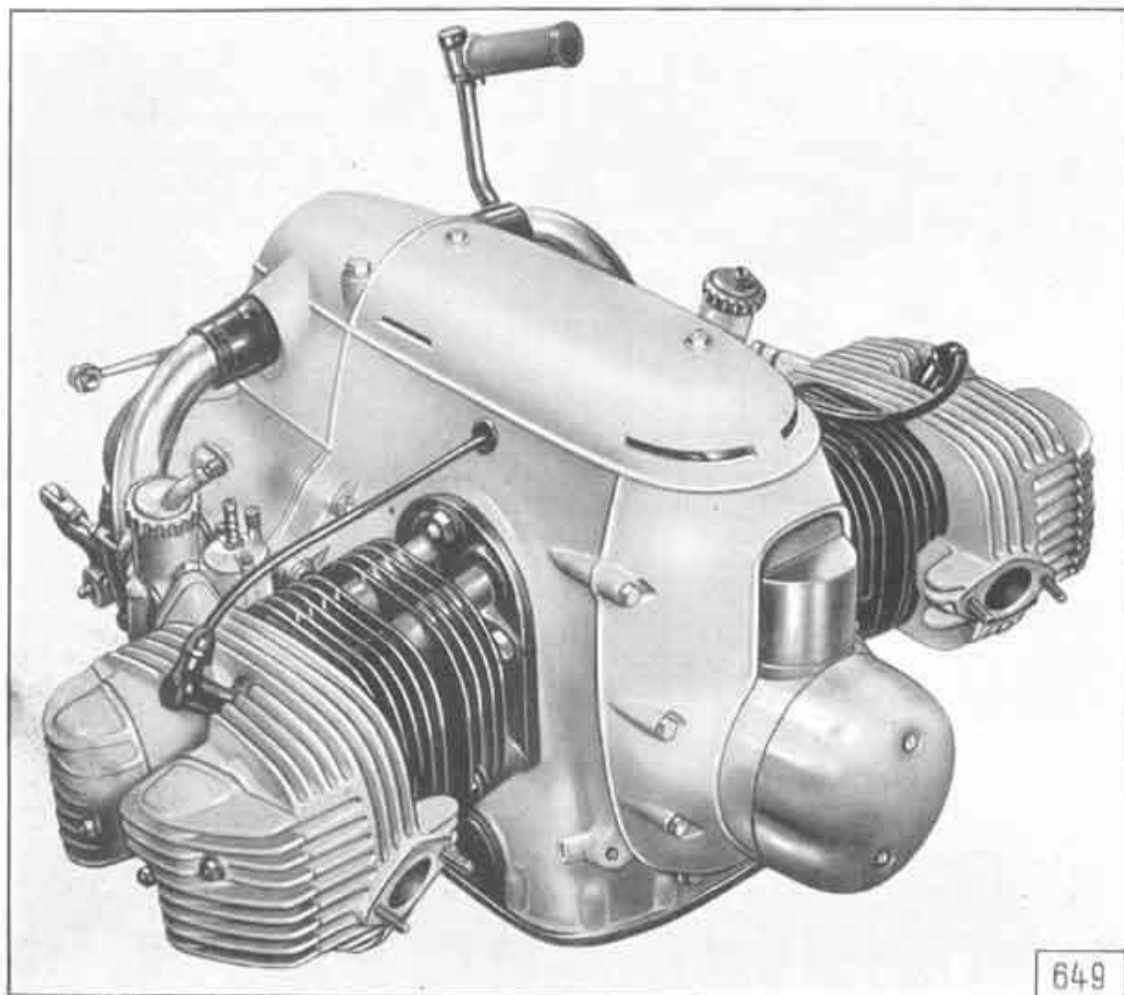
Tafel 1, Gruppe M: a) Motor (Zusammenbau)
