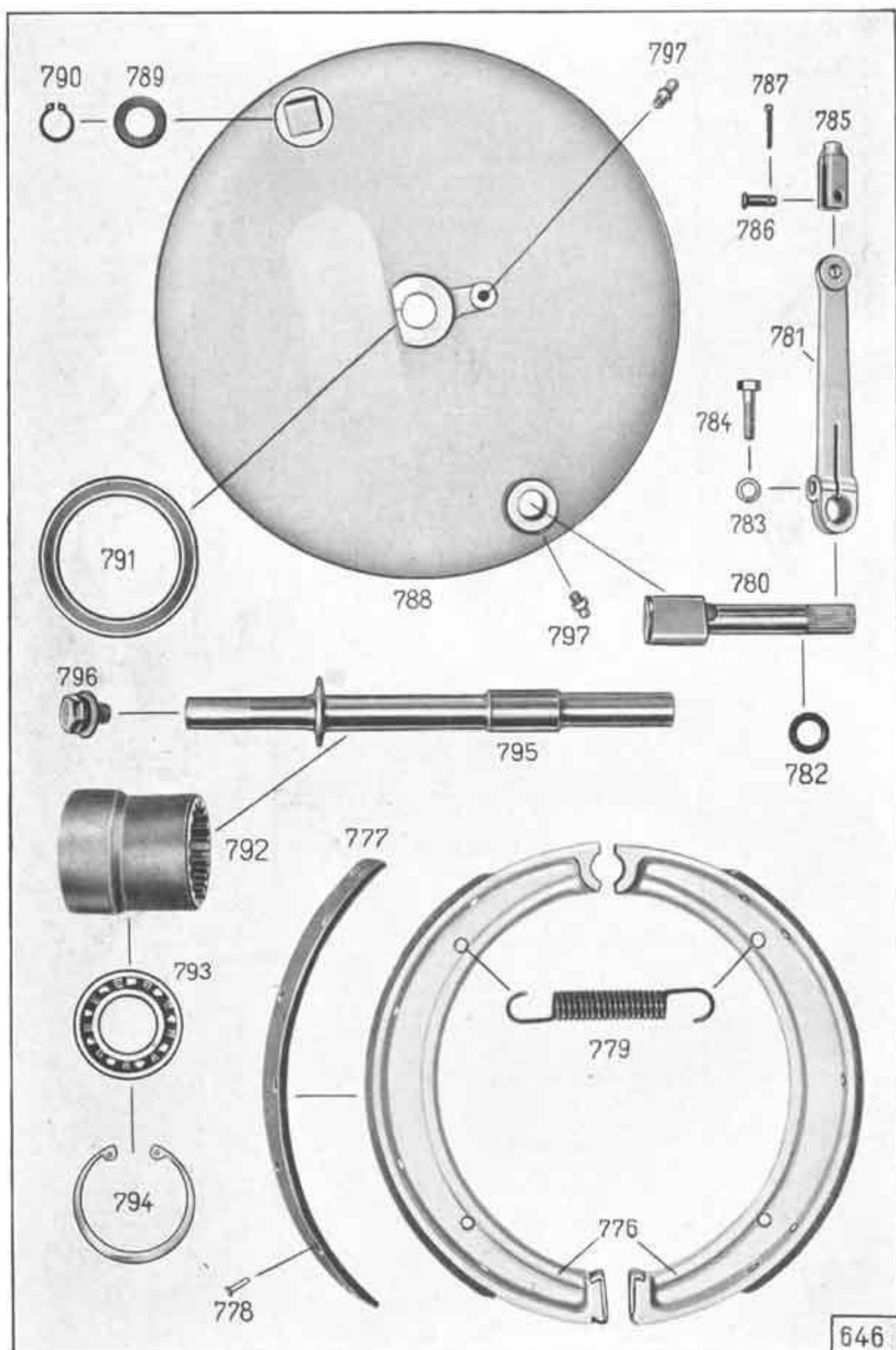
Tafel 28, Gruppe B: a) Bremsen, Handbremse
