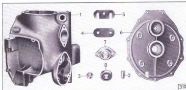
Tafel 11, Gruppe G: a) Wechselgetriebe, b) Getriebegehäuse
