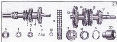
Tafel 12, Gruppe G: c) Wellen und Kettenräder
