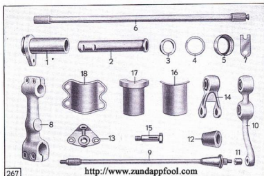
Tafel 34, Gruppe 1: Seitenwagen-Fahrgestell, Radfederung
