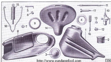
Tafel 21, Gruppe R: f) Kraftstoffbehälter und -leitungen
