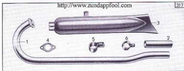
Tafel 22, Gruppe R: h) Auspufftopf und -leitungen
