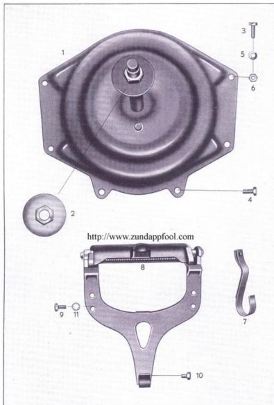
Tafel 35, Gruppe 2: Seitenwagenboot
