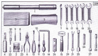
Tafel 30, Gruppe W: a) Werkzeug
