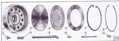
Tafel 10, Gruppe M: g) Kupplung Kupplung Kupplungsbetätigung
