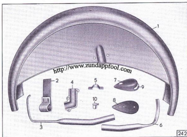
Tafel 33, Gruppe 1: Seitenwagen-Fahrgestell, Schutzblech
