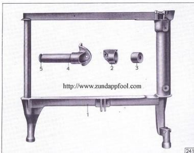
Tafel 31, Gruppe 1: Seitenwagen-Fahrgestell, Rahmen
