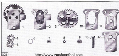
Tafel 7, Gruppe M: e) Ölpumpe
