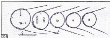
Tafel 26, Gruppe R: k) Lenker, Seilzüge
