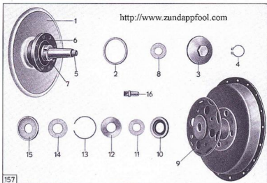
Tafel 36, Gruppe 3: Seitenwagenrad
