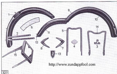
Tafel 20, Gruppe R: d) Schutzbleche, Vorderrad-Schutzblech
