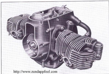
Tafel 1, Gruppe M: a) Motor (Zusammenbau)
