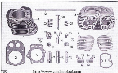
Tafel 5, Gruppe M: b) Gehäuse und Zylinder Zylinder und Zylinderkopf Ventile und Steuerung
