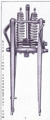
Tafel 23, Gruppe R: i) Vordergabel (Zusammenbau)
