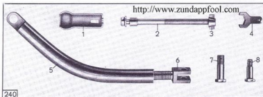
Tafel 32, Gruppe 1: Seitenwagen-Fahrgestell, Anschlußteile
