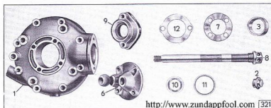
Tafel 16, Gruppe H: b) Gehäuse mit Deckel
