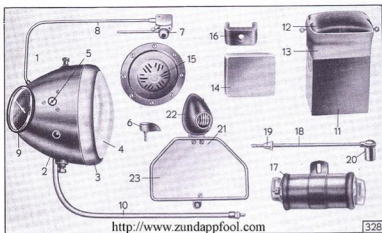
Tafel 28, Gruppe E: a) Elektrische Ausrüstung, Scheinwerfer
