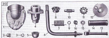
Tafel 14, Gruppe G: e) Anwerfer
