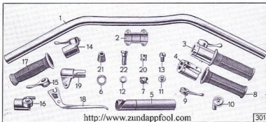
Tafel 25, Gruppe R: k) Lenker
