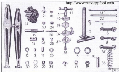
Tafel 24, Gruppe R: i) Vordergabel
