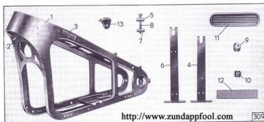
Tafel 18, Gruppe R: a) Rahmen
