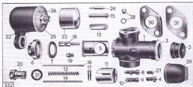
Tafel 8, Gruppe M: f) Vergaser
