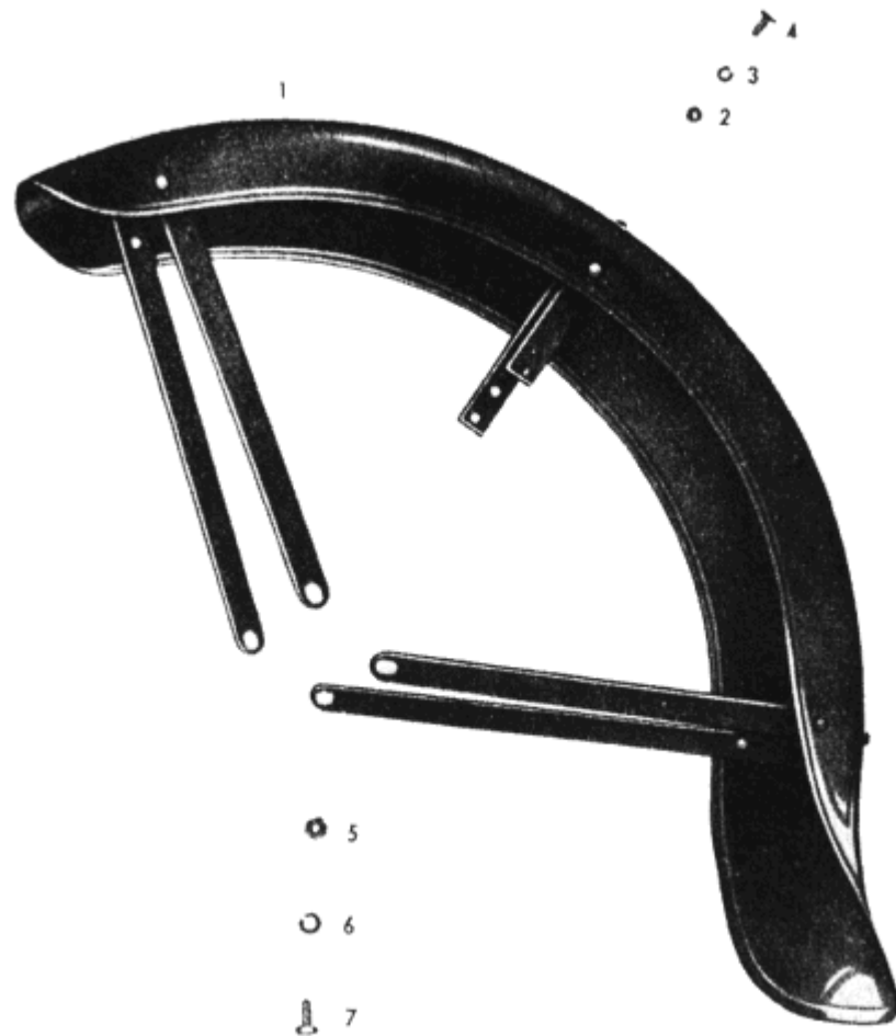
Tafel 7 Schutzblech, vorderes
