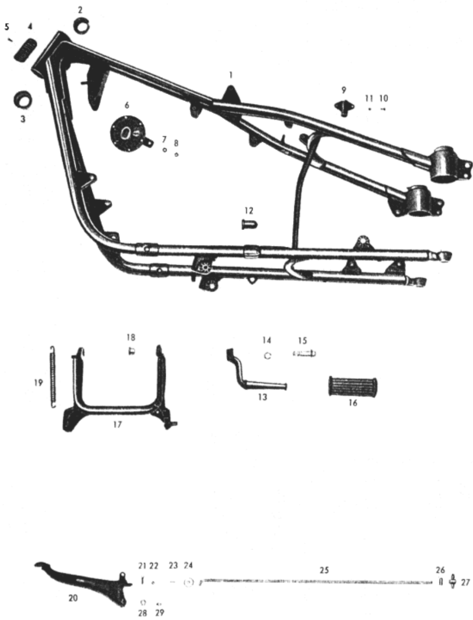
Tafel 2 Rahmen, Fußbremse
