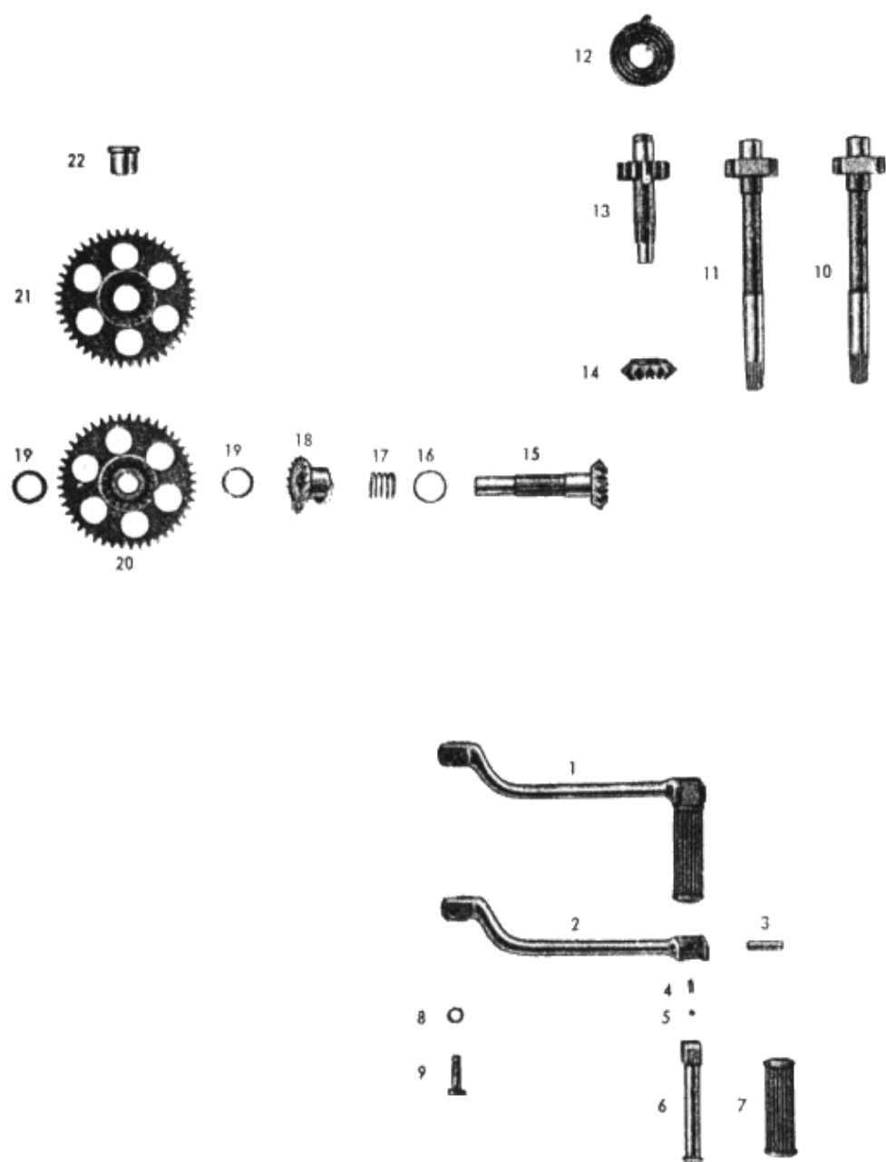
Tafel 26 Kickstarteranlage, Kickstarterhebel
