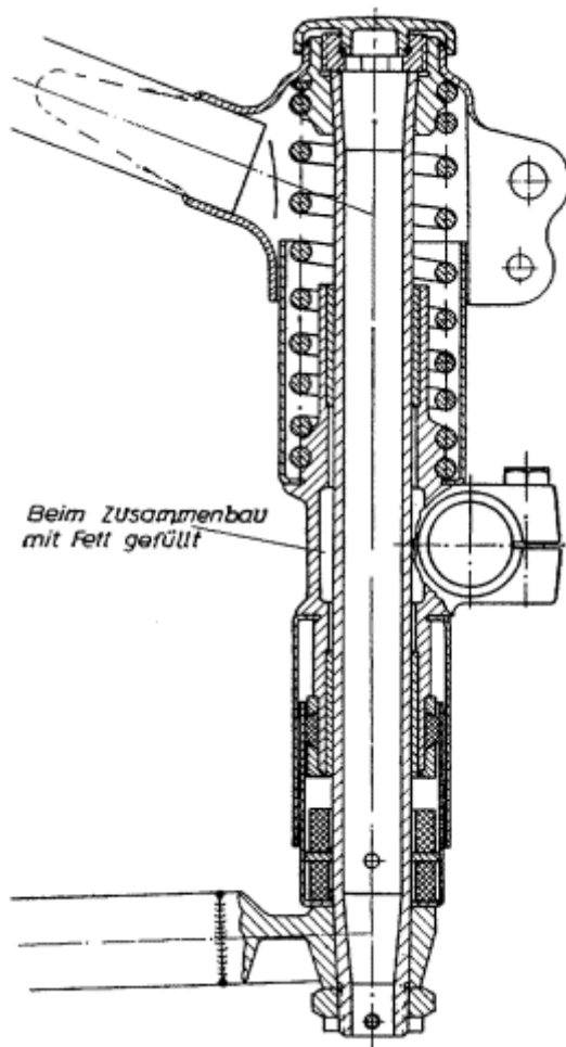
Bild 28. Schnitt durch die Hinterradfederung
