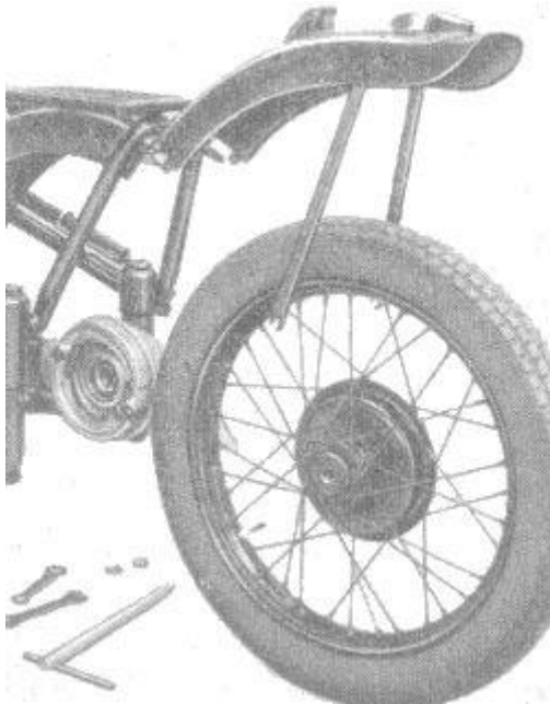
Bild 67. Hinterrad ausbauen
