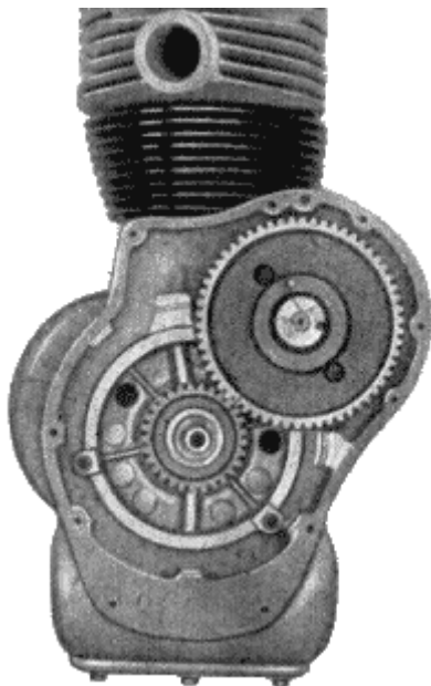
Bild 8. Antrieb der Pleuellnockenwelle
