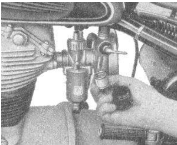
Bild 46. Kraftstofffilter des Benzinahns reinigen
