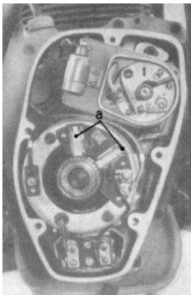
Bild 16. Elektrikgehäuse mit Lichtmaschine und Magnetzylinder
