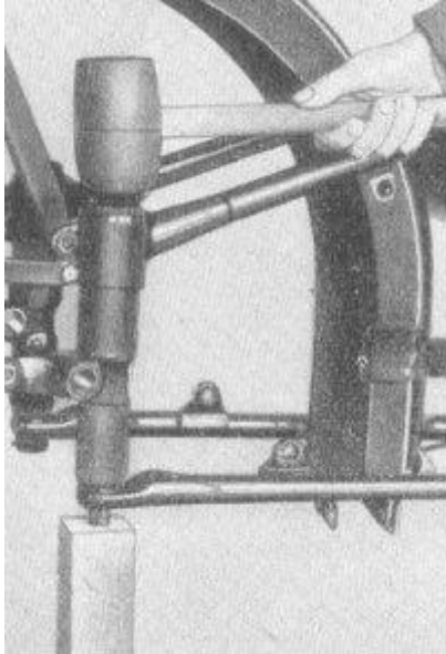
Bild 77. Ausbau der Führungshülse der Hinterradfederung
