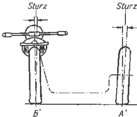
Bild 82. Einstellung des Seitenwagens (Sturz)
