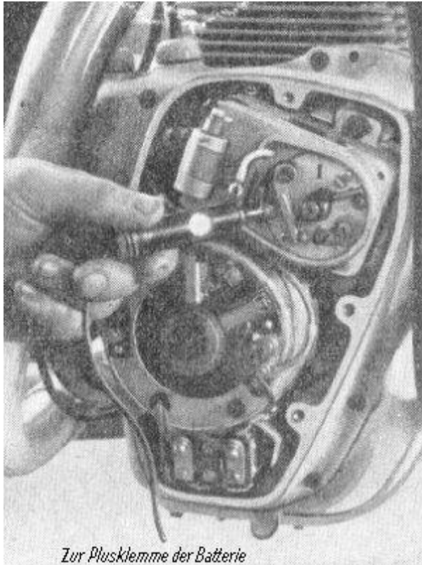
Bild 52. Einstellung der Zündung mittels Prüflampe
