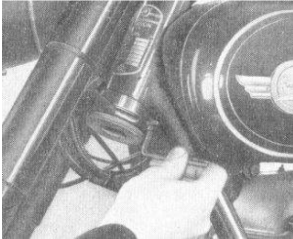
Bild 70. Widerstandsblech des Steuerungs- dämpfers ausbauen (Lösen der Innensechskantschraube)
