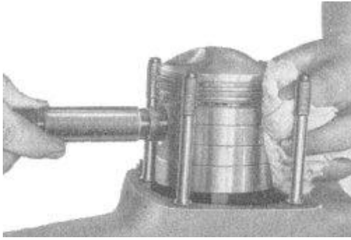
Bild 60. Einbau des Kolbenbolzens mittels Hilfsdorn
