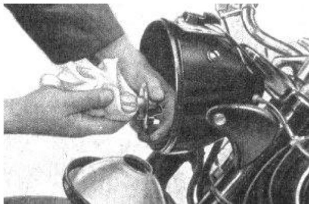
Bild 20. Auswechseln der Biluxlampe
