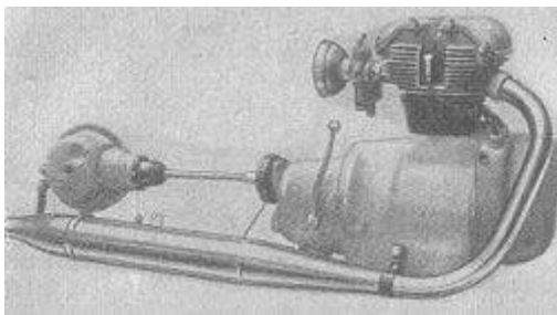
Bild 2. Antriebsblock
