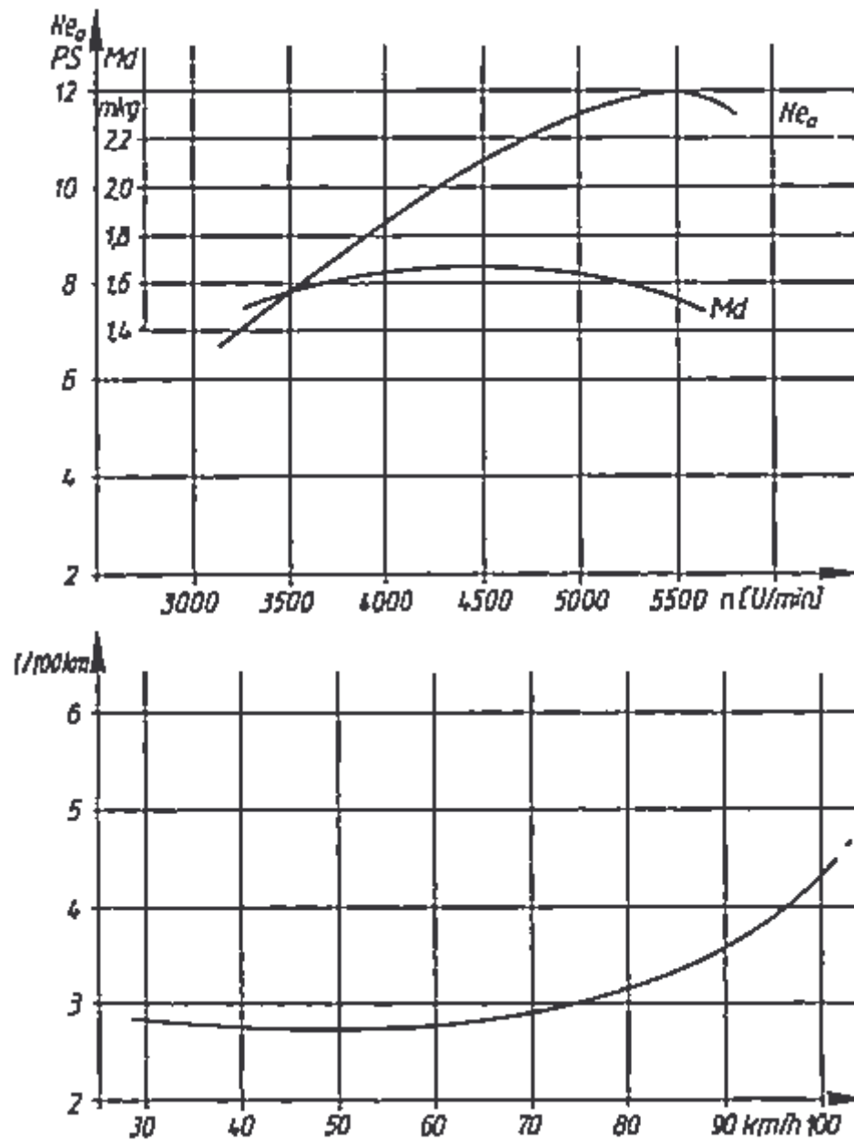
Bild 1. Motorkennlinien
