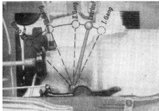
Bild 33. Fußschalthebel
