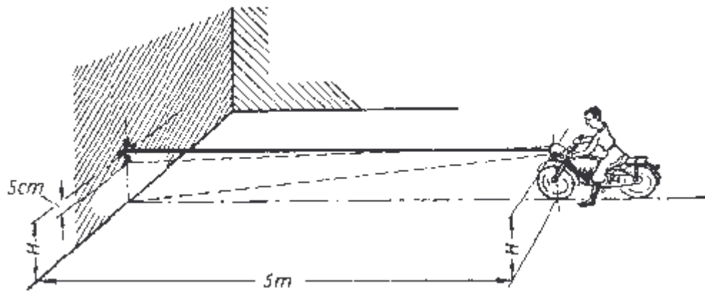
Bild 21. Einstellen des Scheinwerfers
