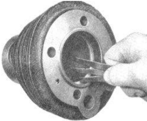
Bild 58. Kolbenringstoß prüfen
