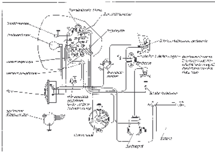
Schaltplan
