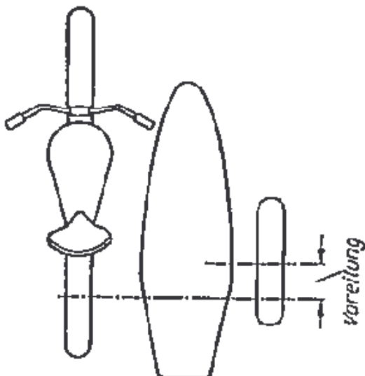
Bild 81. Einstellung des Seitenwagens (Voreilung oder Vorlauf)
