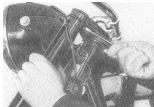
Bild 41. Lösen der Sechskantmuttern für die Lenkerbefestigung
