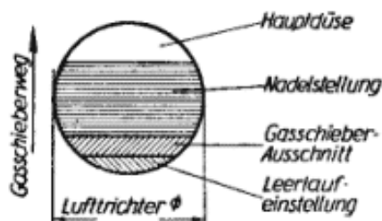
Bild 15. Wirkungsbereiche der verschiedenen Einstellfaktoren beim Vergaser
