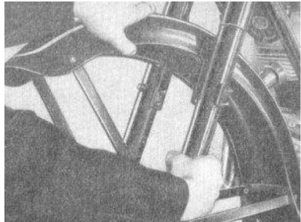
Bild 68. Vorderradschutzblech ausbauen (mittlere Schutzblechstreben aus den Halteschrauben herausheben)
