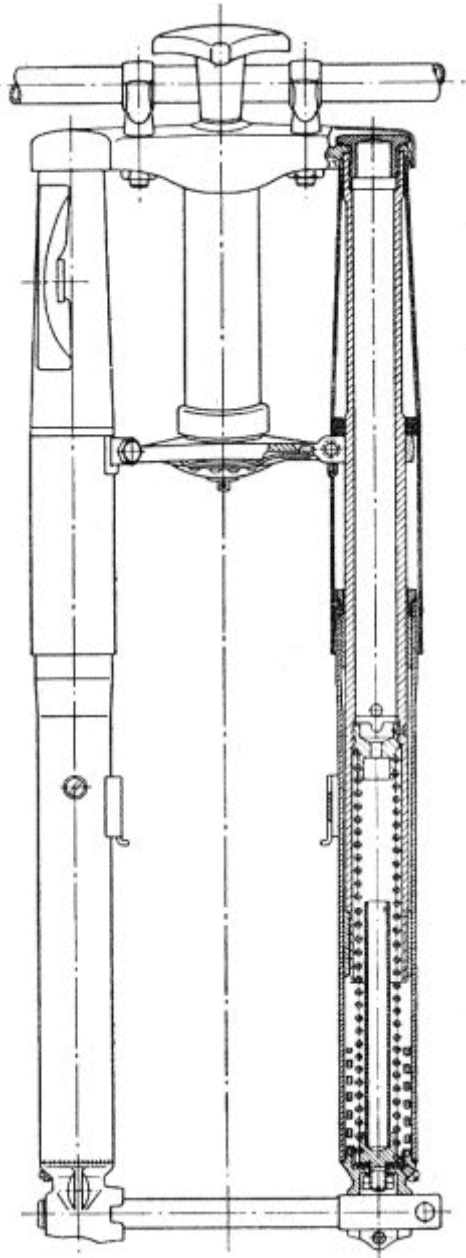
Bild 27. Schnitt durch die Teleskopgabel
