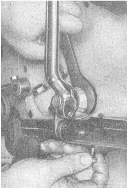
Bild 65. Kickstarterfeder spannen
