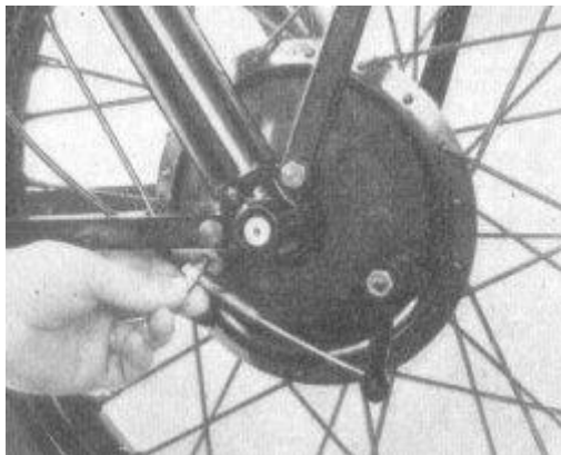
Bild 29. Nachstellen der Vorderradbremse
