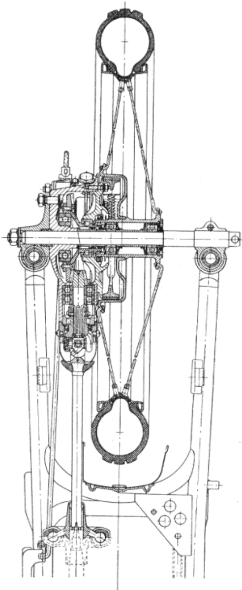
Bild 26. Schnitt durch den Hinterradantrieb
