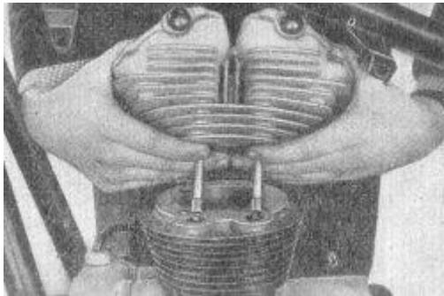
Bild 53. Zylinderkopf abnehmen
