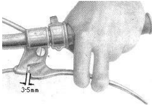
Bild 32. Erforderliches Spiel am Kupplungshebel
