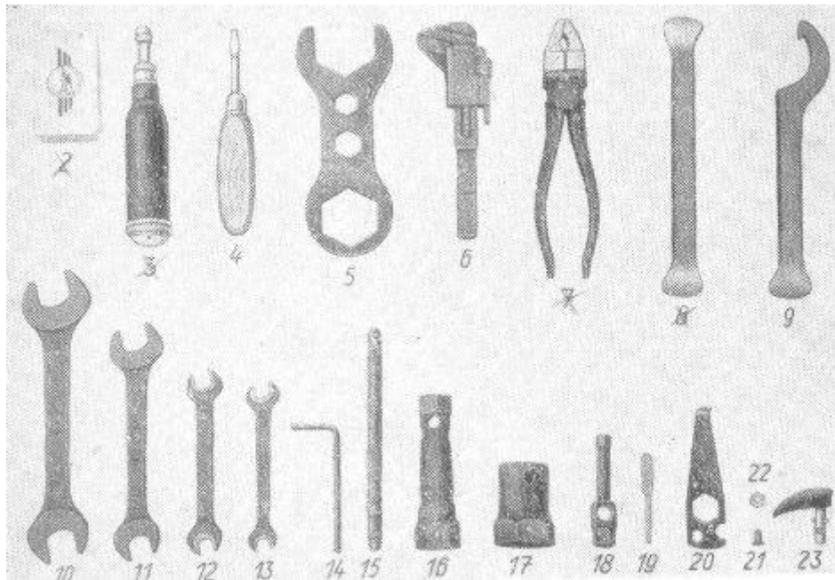
Bild 49a. Bordwerkzeug
