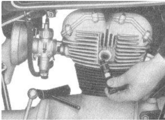
Bild 48. Zündkerze prüfen
