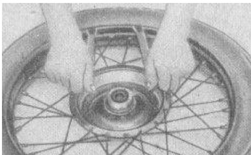
Bild 79. Reifen abnehmen
