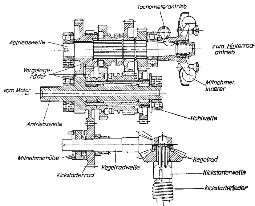
Bild 25. 4-Gang-Getriebe (Schieberäder in Leerlaufstellung)
