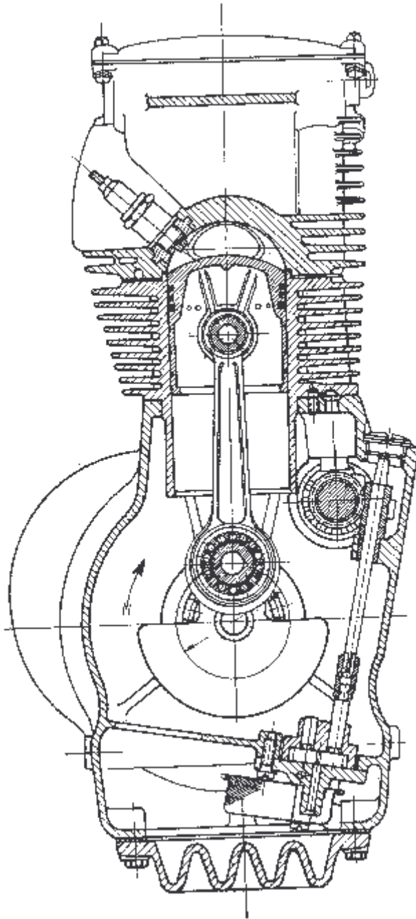
Bild 4. Querschnitt durch den Motor
