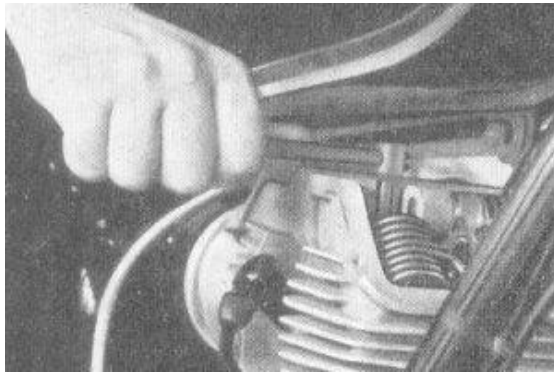
Bild 40. Zuganker für Zylinderkopf nachziehen
