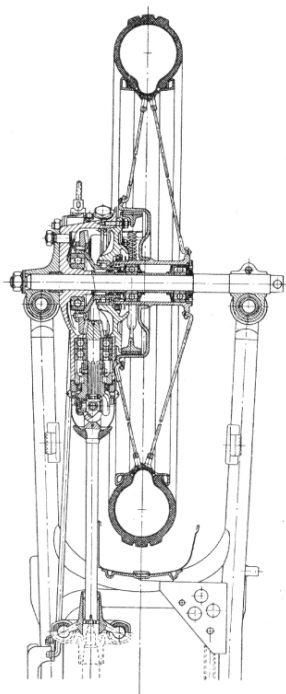
Bild 26. Schnitt durch den Hinterradantrieb
