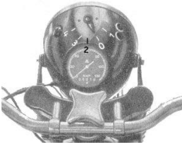
Bild 35. Schalterstellungen des Zünd-Licht-Schalters
