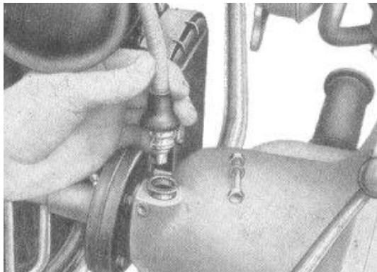
Bild 47. Ausbau der Tachowelle
