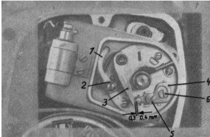
Bild 19. Magnetzünder
