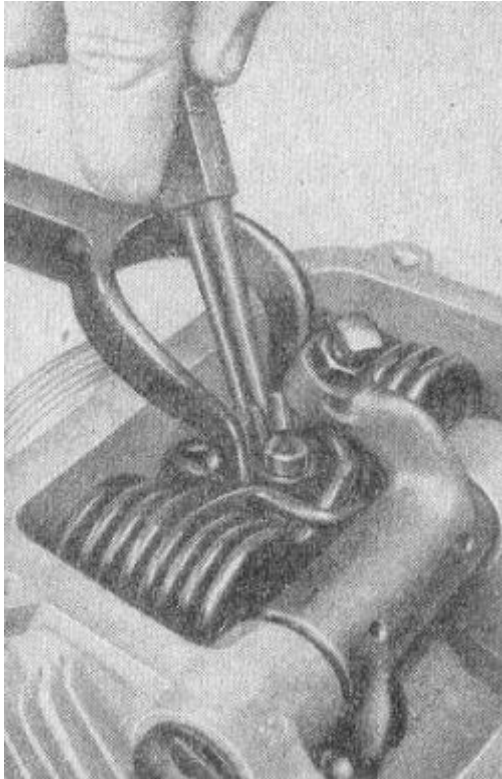
Bild 54. Ventile ausbauen
