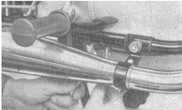
Bild 23. Nachstellen des Kupplungsbowdenzuges
