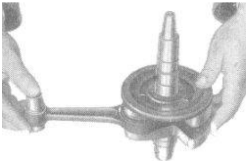
Bild 59. Der Kolbenbolzen darf in dieser Stellung nicht von selber durch sinken, er muss sich aber mit leichtem Fingerdruck durchdrücken lassen
