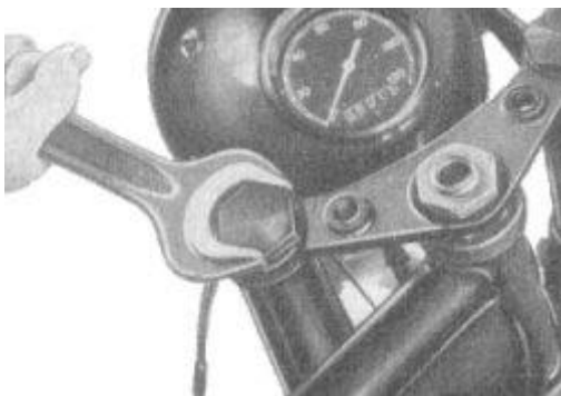
Bild 42. Lösen der Muttern zum Tragrohr
