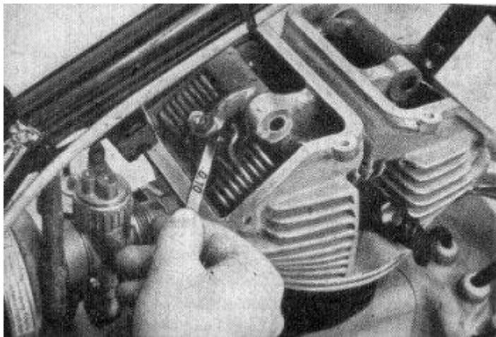
Bild 10. Kontrolle des Ventilspiels mittels Blattlehre
