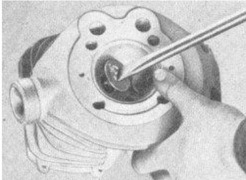
Bild 55. Ventile einschleifen
