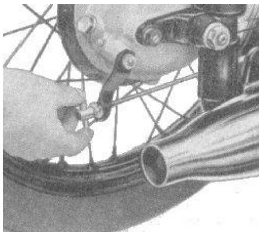
Bild 30. Nachstellen der Hinterradbremse
