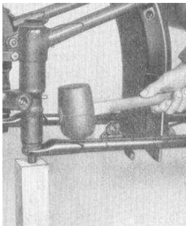
Bild 76. Ausbau der Führungshülse der Hinterradfederung
