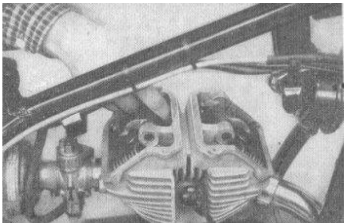
Bild 10. Kontrolle des Ventilspiels mittels Blattlehre
