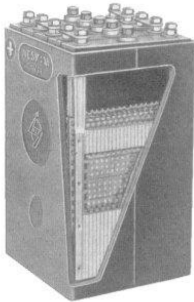
Bild 18. Batterie
