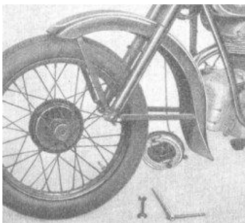
Bild 66. Vorderrad ausbauen
