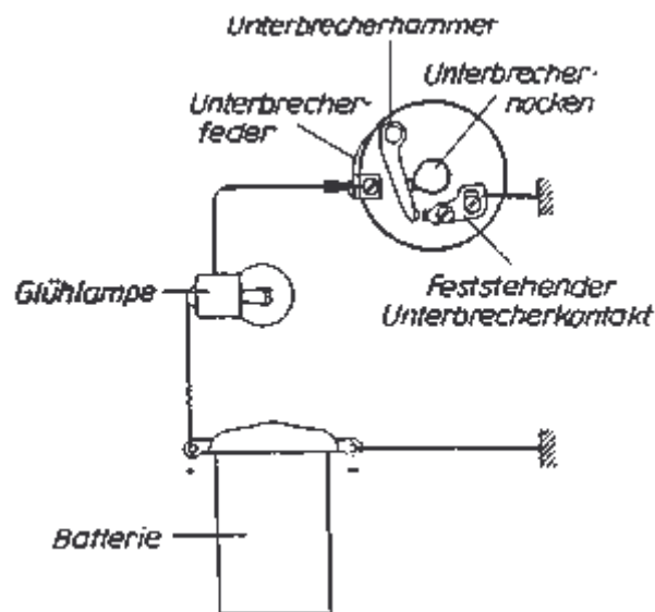
Bild 51. Schaltschema zur Einstellung der Zündung mittels Prüflampe
