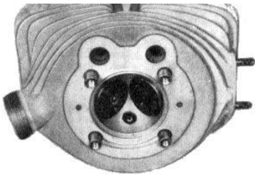
Bild 6. Zylinderkopf (Verbrennungsraum)
