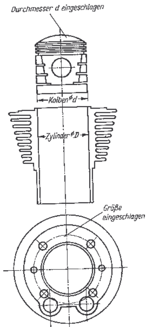
Bild 5. Zusammengehörigkeit von Kolben und Zylinder
