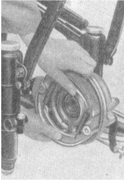
Bild 78. Bremsbacken abnehmen
