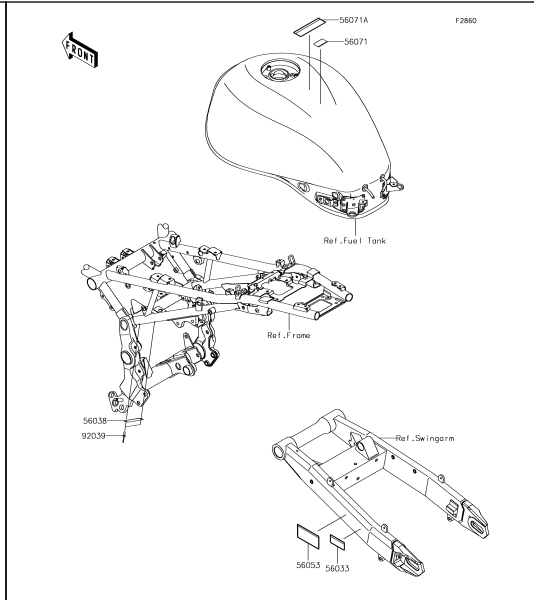
59 Labels
