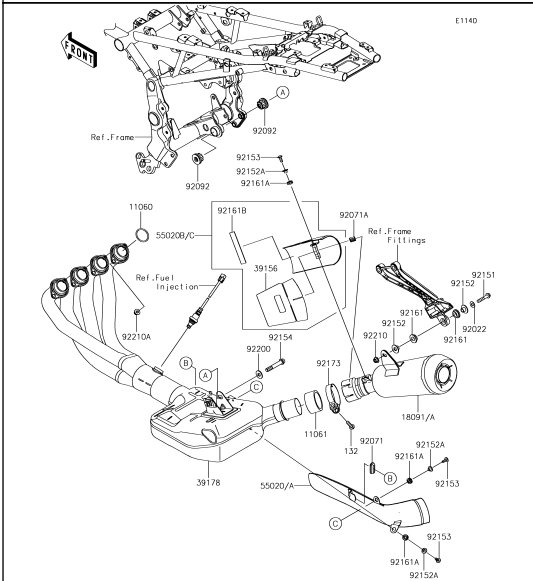
5 Muffler(s)
