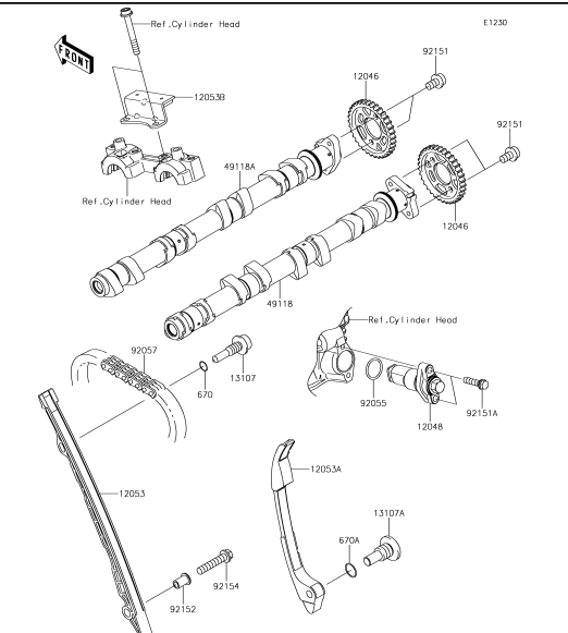
7 Camshaft(s)/Tensioner
