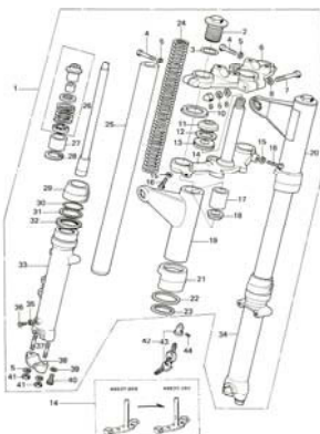
27. Front Fork1/2
