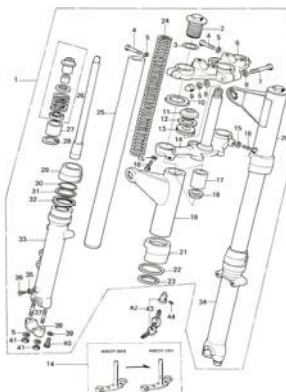
27. Front Fork2/2
