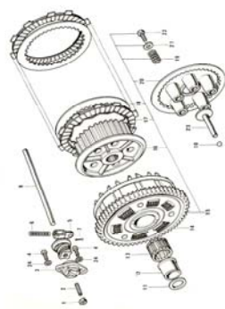
7. Clutch
