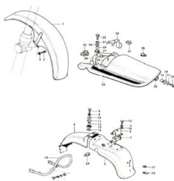
21. Fenders
