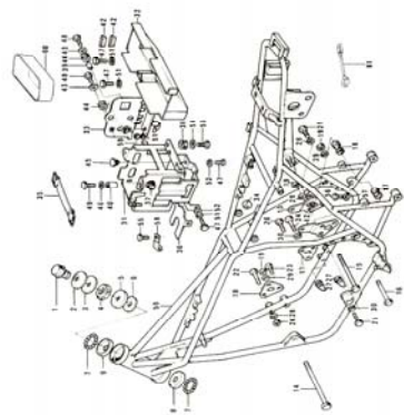
17. Frame 1/2
