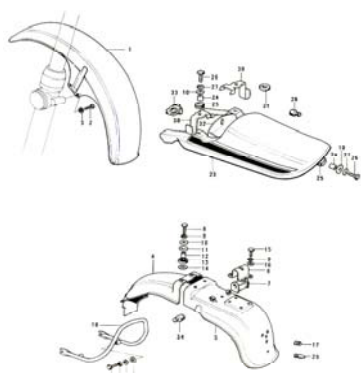
21. Fender
