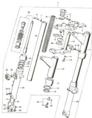
27. Front Fork
