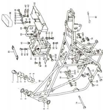
17. Frame 1/2
