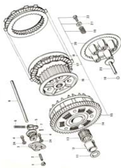
7. Clutch
