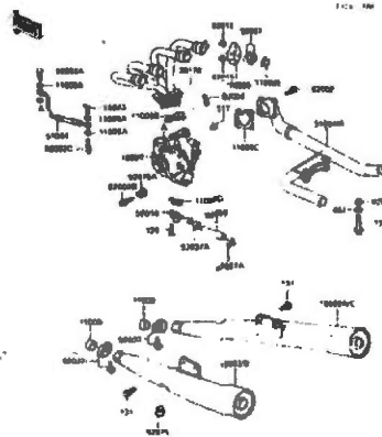
B-7 Muffler
