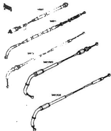
G-3 Cable
